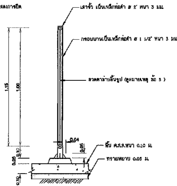
รูปตัด ก-ก ไม่แสดงขนาดราวน
