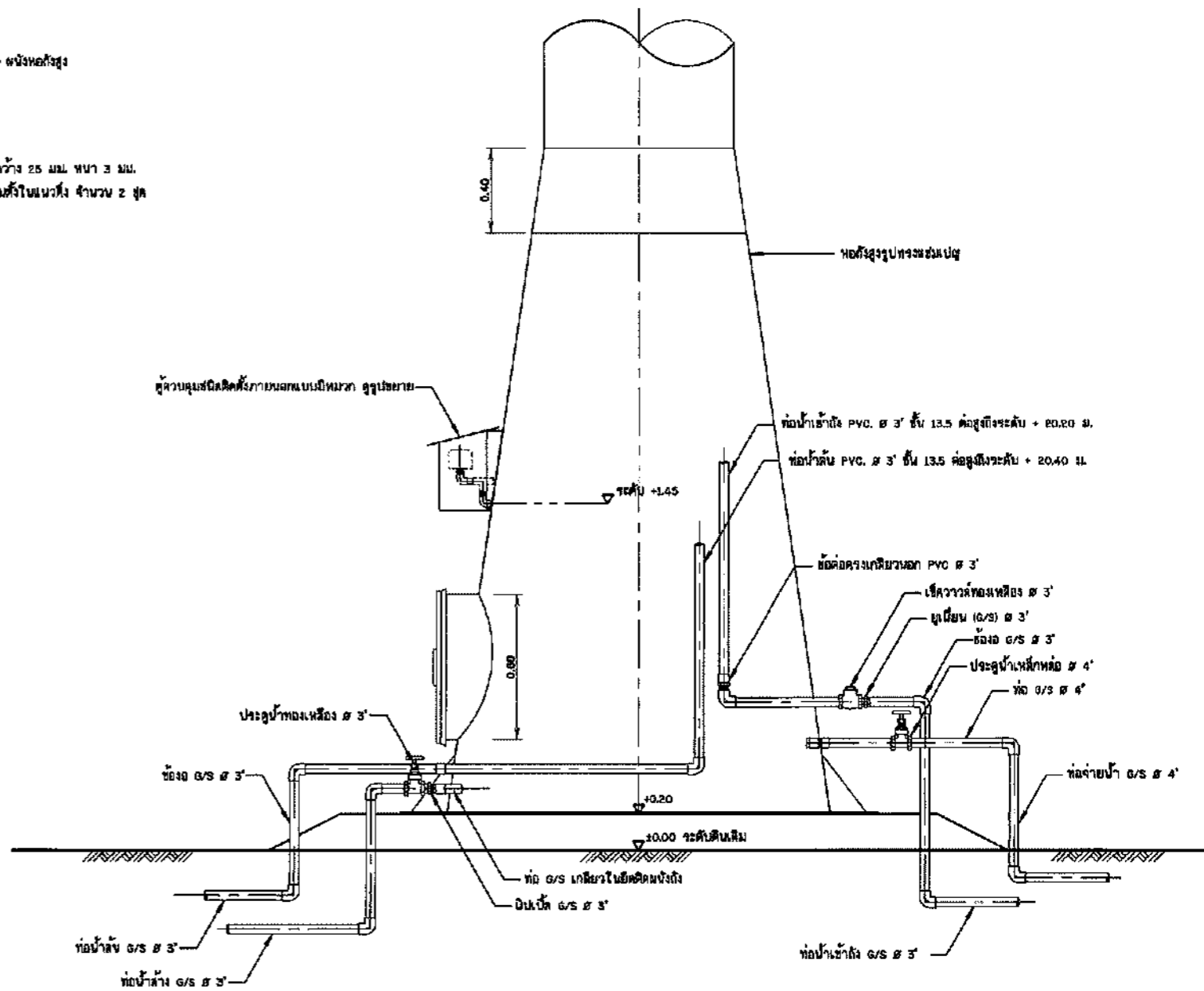
แบบแสดงการเดินทางท่อในห้องถังสูง ไม่แสดงขนาดส่วน
