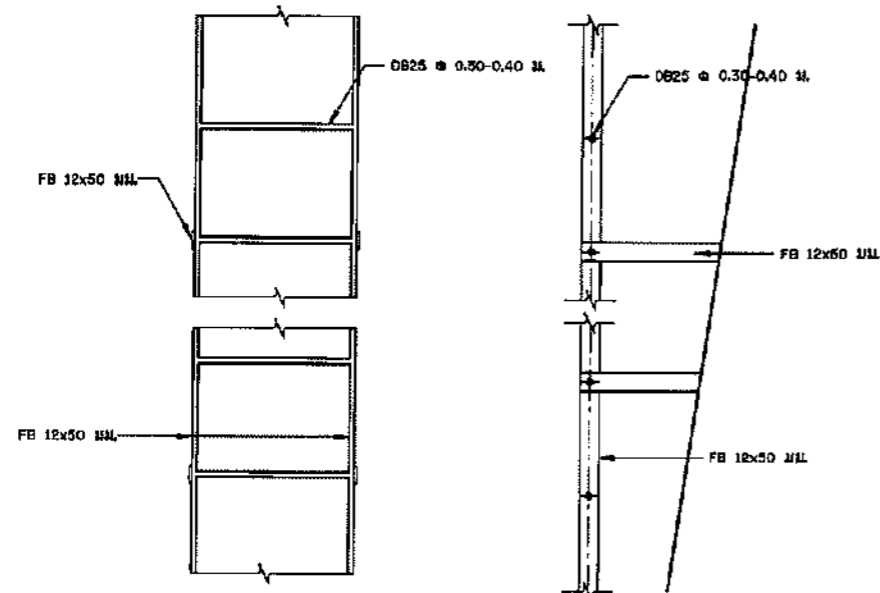
แบบขยายบันได ภายในห้องถังสูง ไม่แสดงขนาดส่วน
