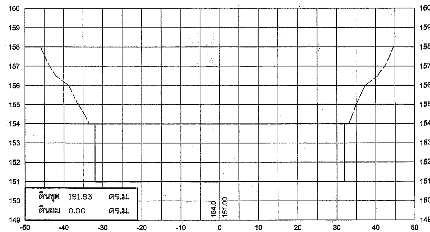
5+150
