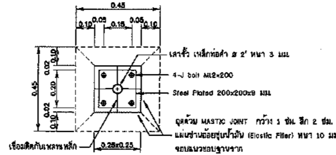
รูปตัด ข-ข ไม่แสดงขนาดราวน
