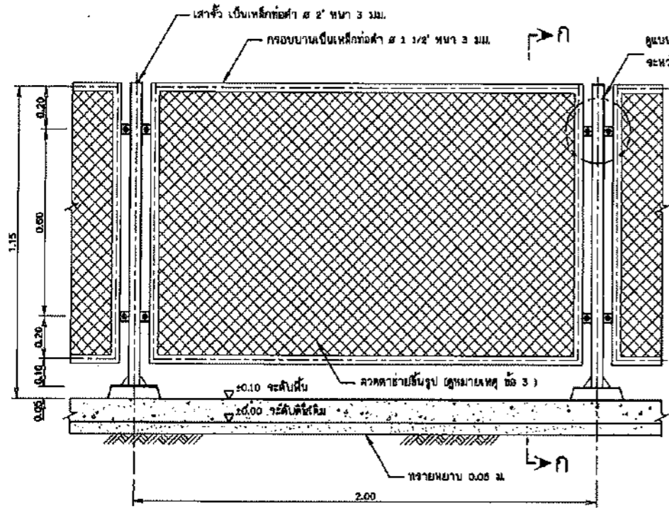
แบบขยายรูปลวดตาข่าย ไม่แสดงขนาดราวน
