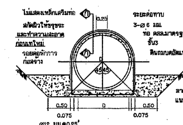
รูปตัดการวางท่อ คลล. ไม่แสดงมาตราส่วน
