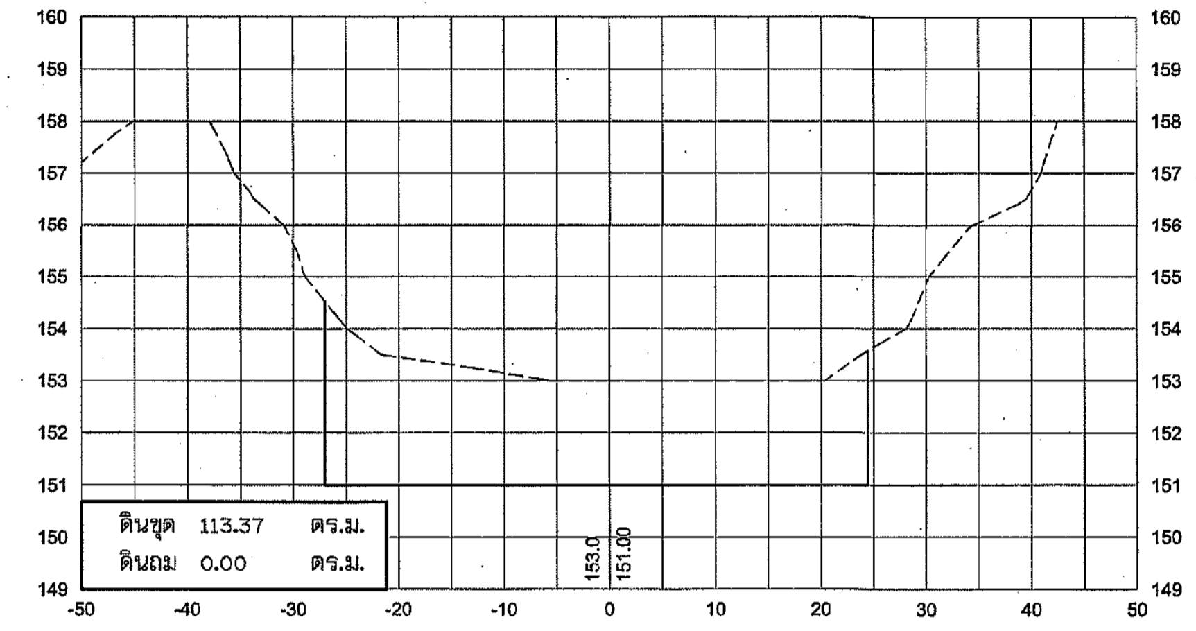
5+303
