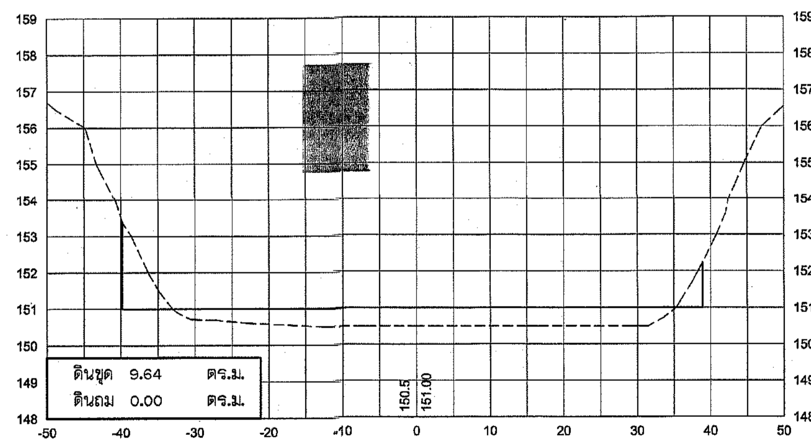
5+000
