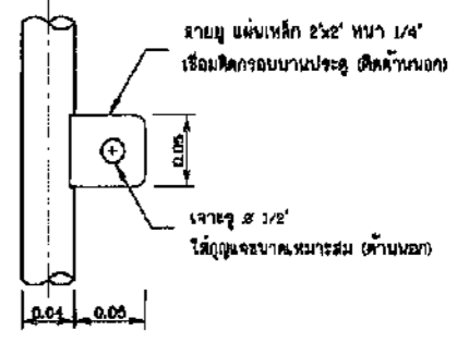
แบบขยายสายยู ไม่แสดงขนาดราวน
