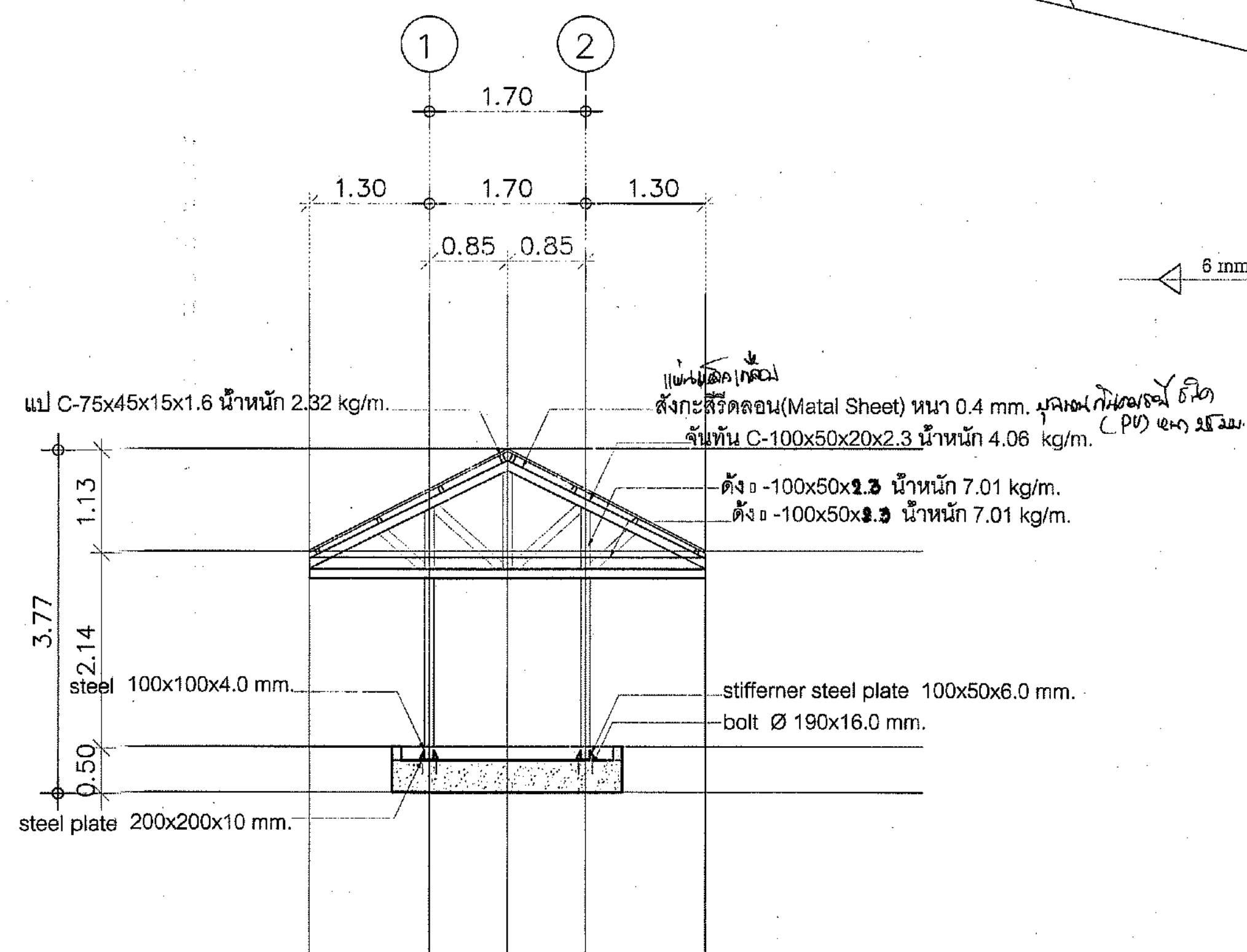
รูปตัด B-B SCALE 1:100
