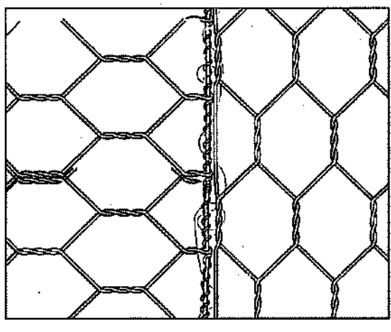
รูปที่ 2 วิธีการผูกยึดกลองลวดตาข่าย
