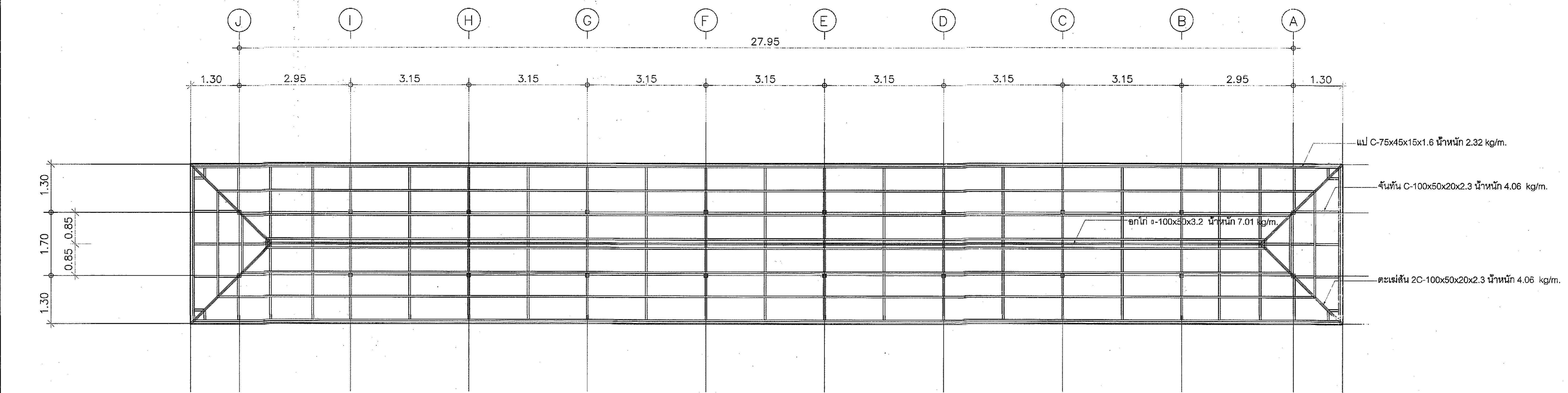
แบบแสดงแปลนโครงสร้างหลังคา SCALE 1:100
