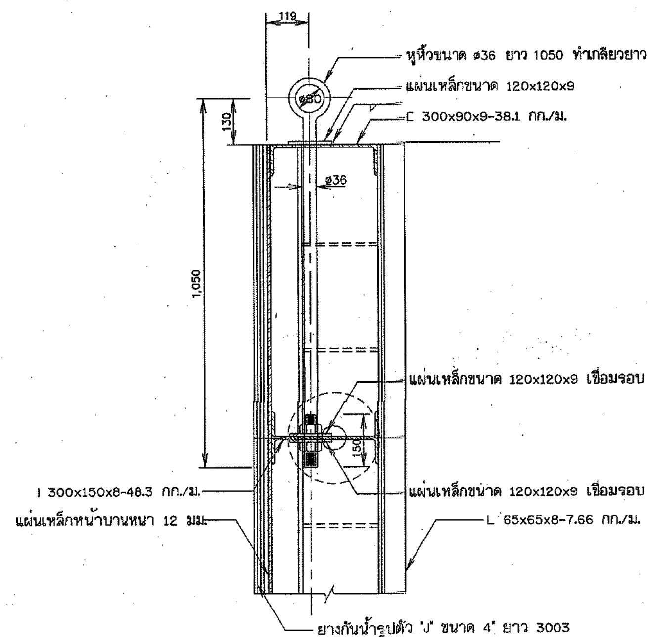
รูปขยาย 1 มาตราส่วน 1:10
