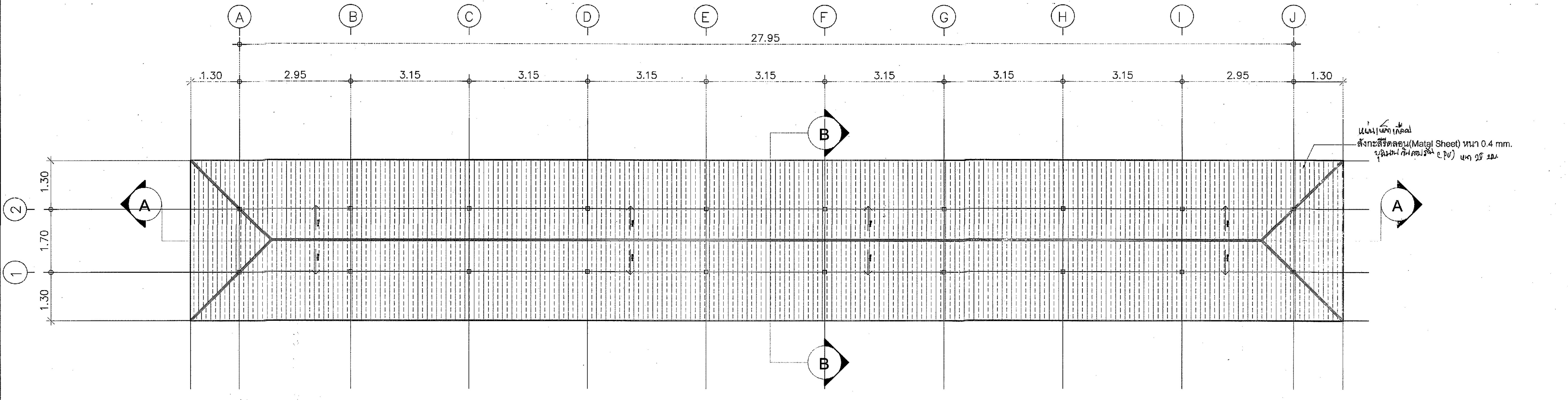
แบบแสดงแปลนหลังคา SCALE 1:100
