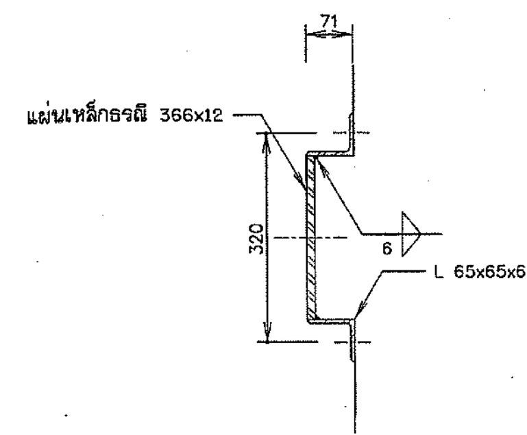
รูปตัด จ - จ มาตราส่วน 1:7.5
