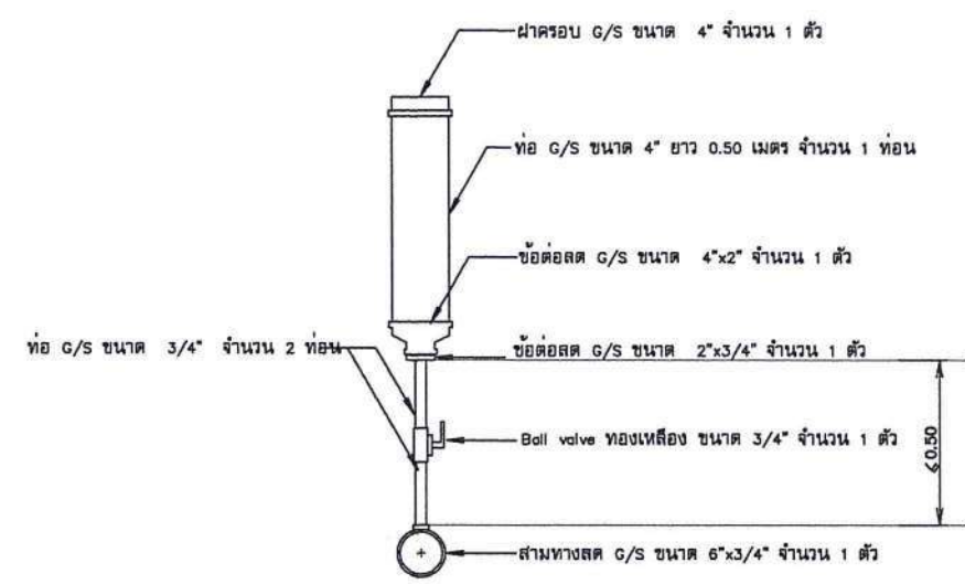
ห้องเติมน้ำ ไม่แสดงมาตราส่วน
