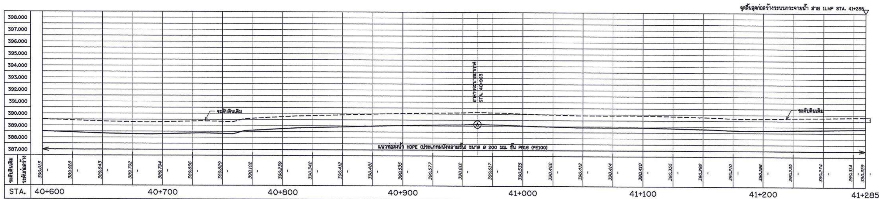
รูปตัดตามแนวยาว สาย 1LMP STA. 40+600 - 41+285
