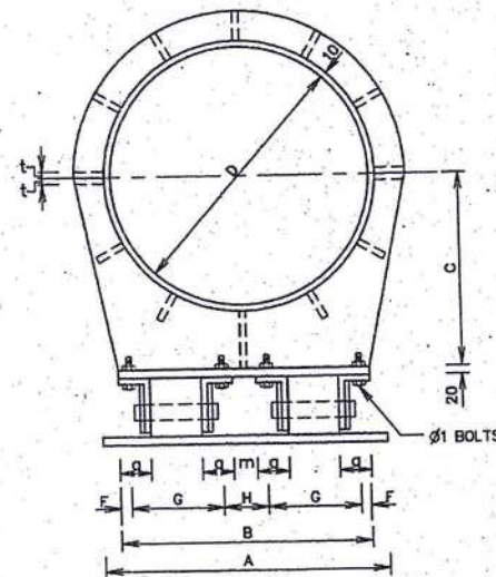
รูปด้านหน้า (สำหรับท่อ Ø400 มม. - Ø1,000 มม.) ไม่แสดงขนาดส่วน
