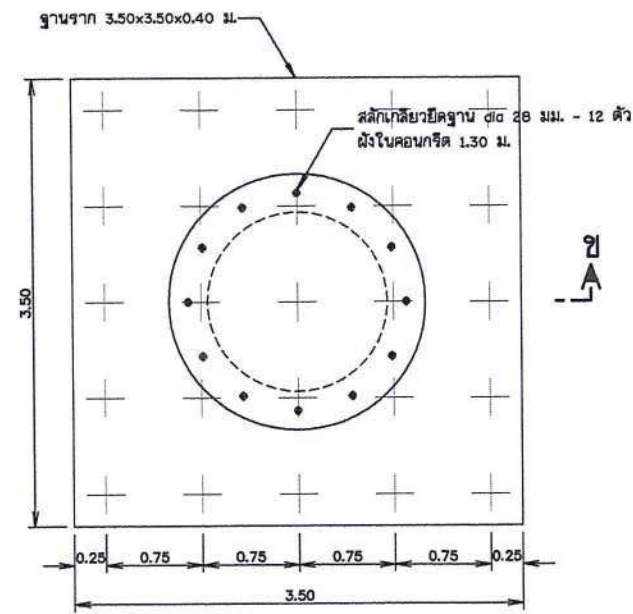
แปลน ฐานรากหอดึงสูง (แบบเสาเข็ม)
