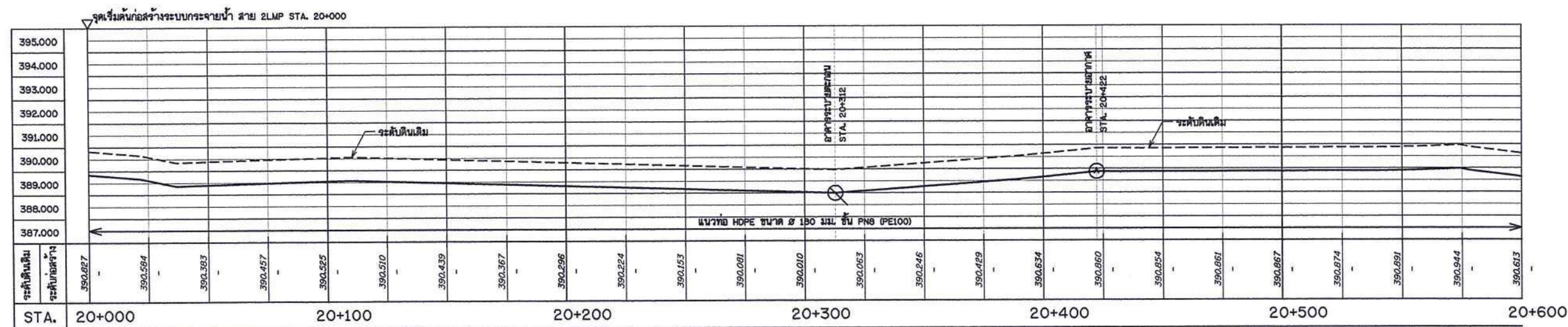
รูปตัดตามแนวยาว สาย 2LMP STA.20+000 - 20+600
