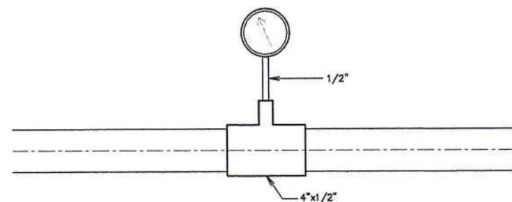
Pressure Gauge Valve ไม่แสดงมาตราส่วน
