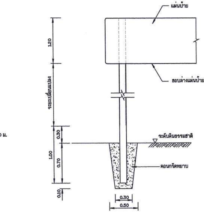
รายละเอียดการติดตั้งเสาป้าย มาตราส่วน 1:20
