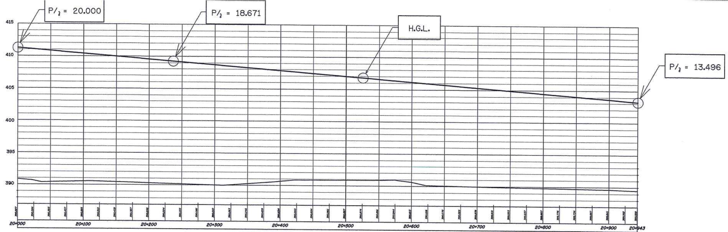
รูปตัดตามแนวยาวแสดง H.G.L. สาย 2LMP STA. 20+000 - 20+943 ไม่แสดงขนาดสวน
