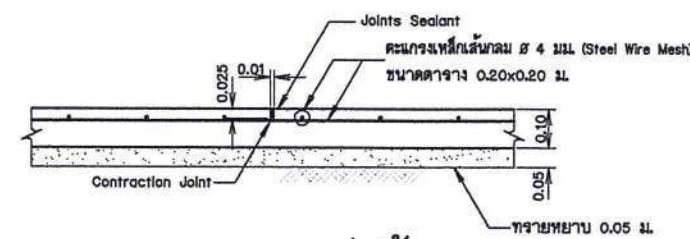
แบบขยายรอยต่อพื้น
