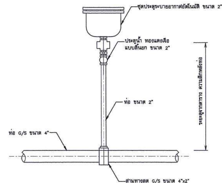
การติดตั้งประตูปะบายอากาศอัตโนมัติ ไม่แสดงมาตราส่วน
