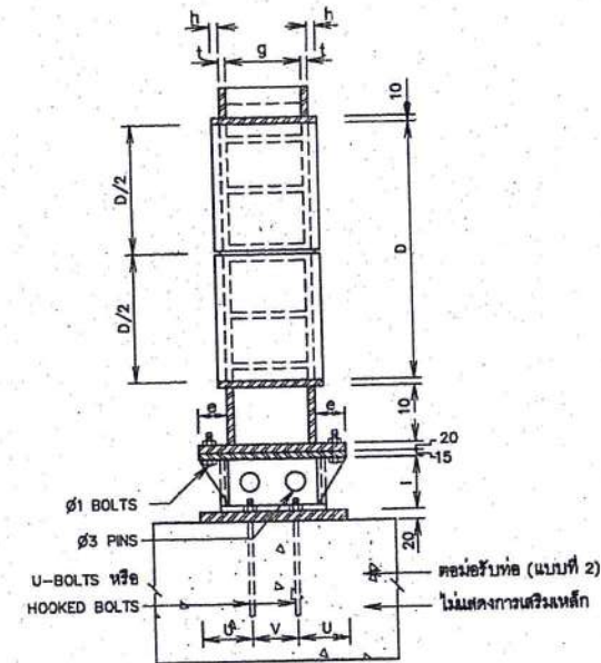
รูปตัด ค-ค ไม่แสดงขนาดส่วน
