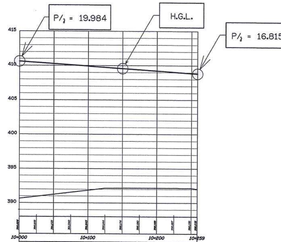
รูปตัดตามแนวยาวแสดง H.G.L. สาย 1R-3LMP STA. 10+000 - 10+259 ไม่แสดงขนาดจั่วหัว
