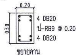
ขยายคาน
