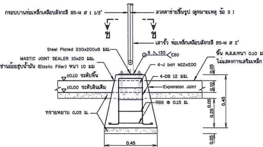
รูปขยายฐานรากโครงสร้างรับแผง F1 (ต่อหน้า คสล. หล่อสำเร็จรูปพร้อมติดตั้ง) ไม่แสดงมาตราส่วน
