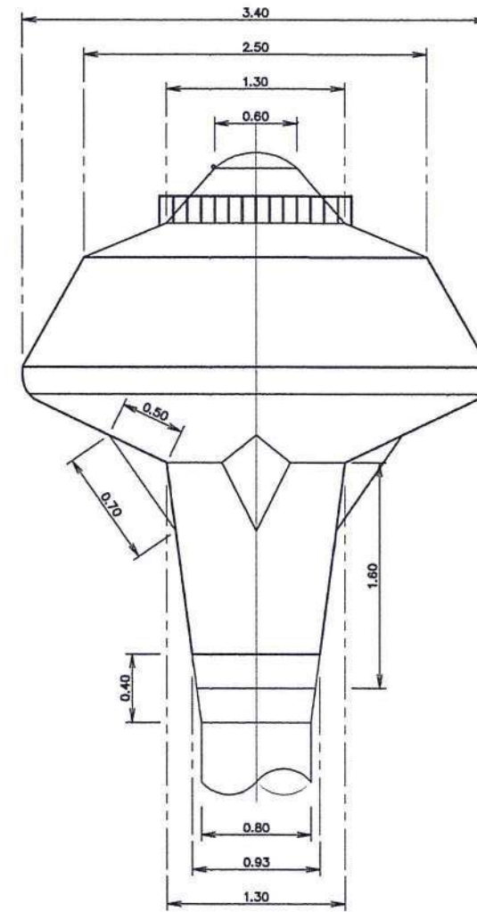
แบบขยายแมนโฮลบนของท่อสูง
