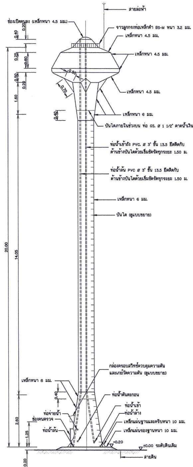
รูปด้านข้างของท่อสูง แบบถังเหล็กทรงกลมแป้น
