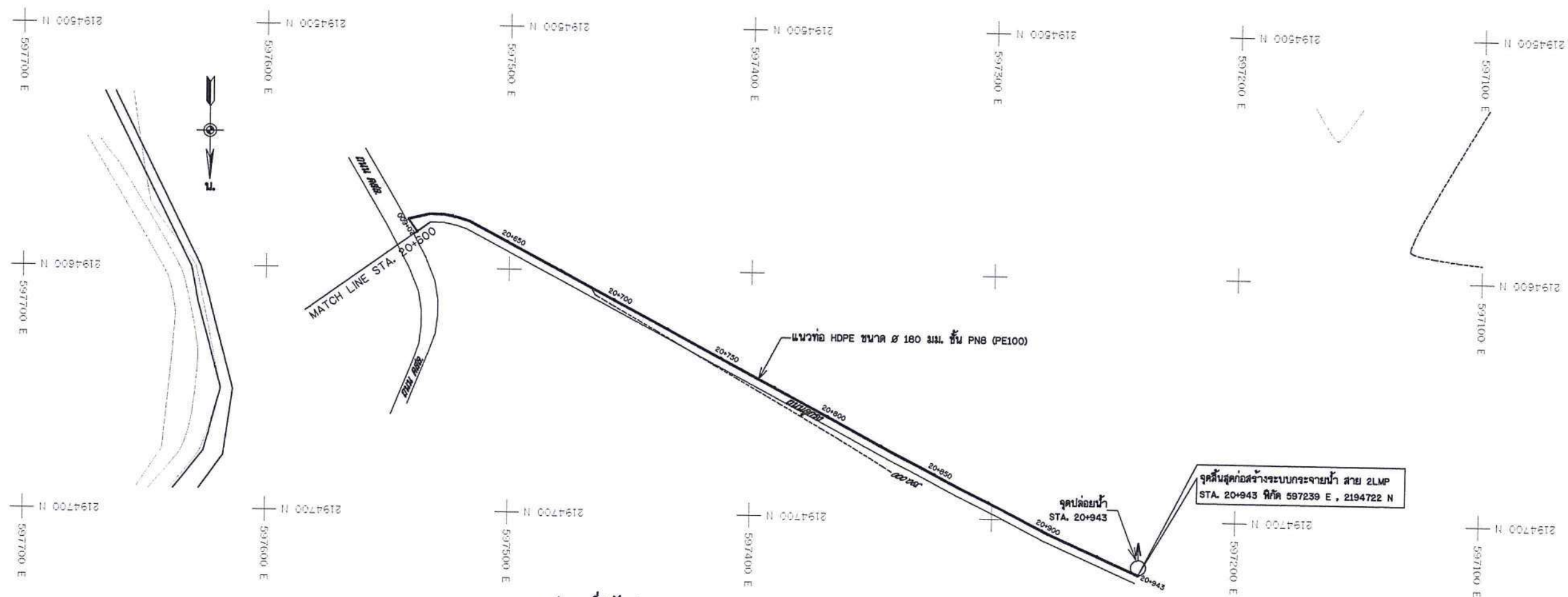
แปลนทั่วไป สาย 2LMP STA.20+600 - 20+943 มาตราส่วน 1:1,000
