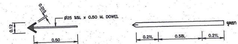
รูปขยาย CASH IRON SHOE
