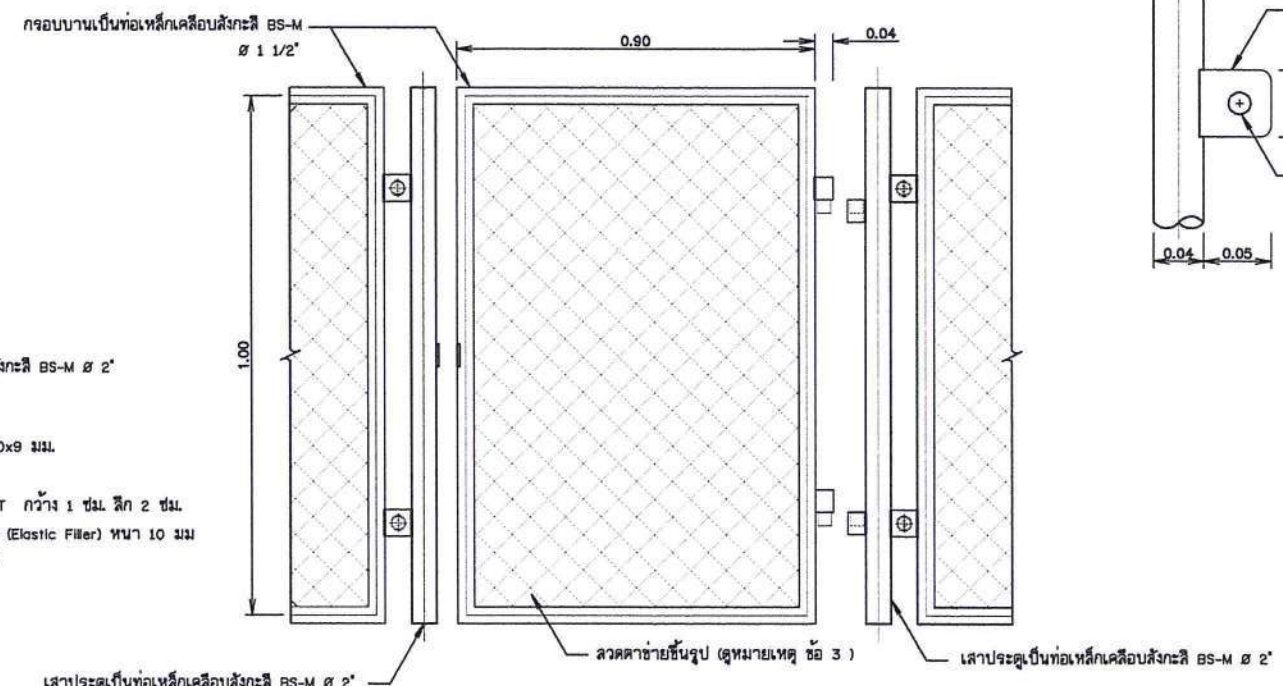
แบบขยายรายละเอียดประตู ไม่แสดงมาตราส่วน
