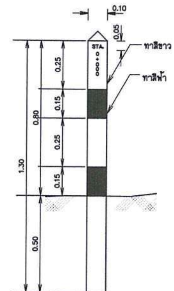
แสดงสัดส่วนหลักบอกแนวท่อ
