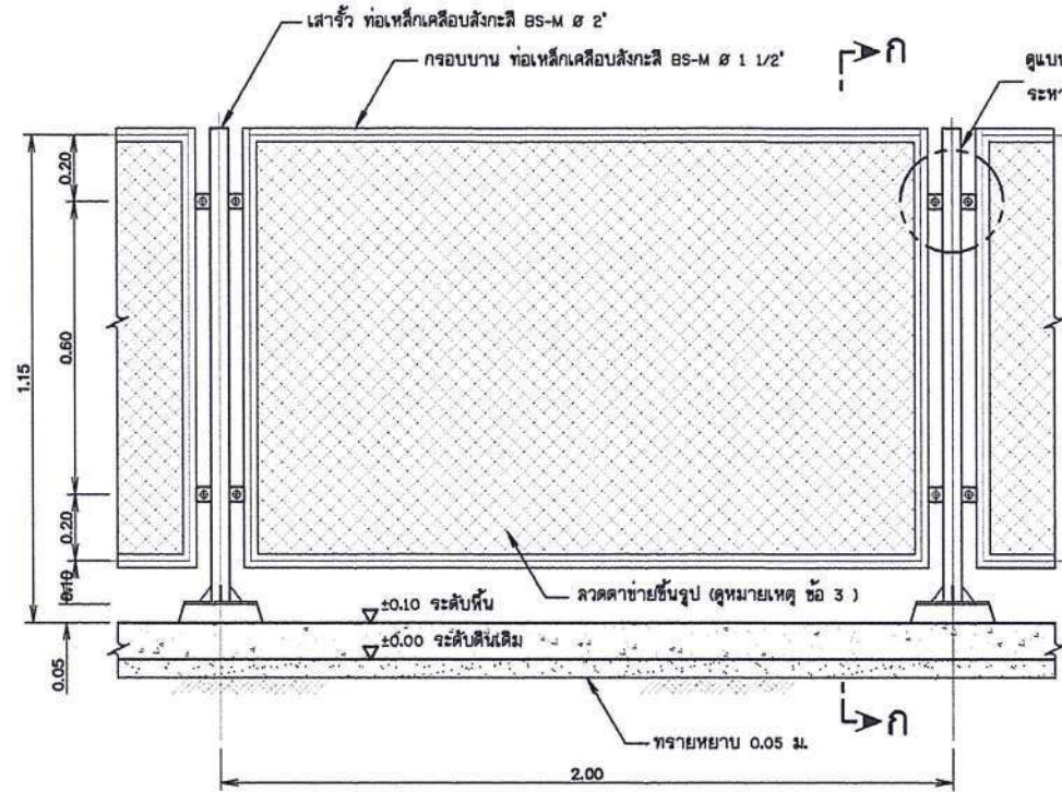
แบบขยายรั้วลวดลาย ไม่แสดงมาตราส่วน
