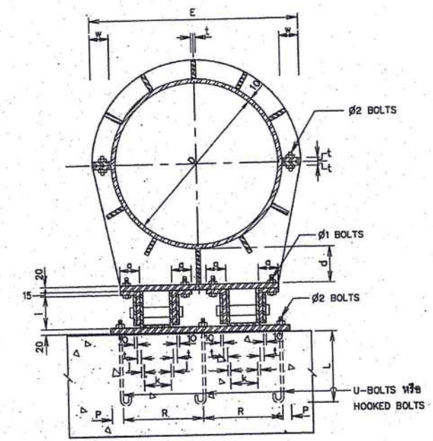
รูปตัด ง-ง ไม่แสดงขนาดส่วน
