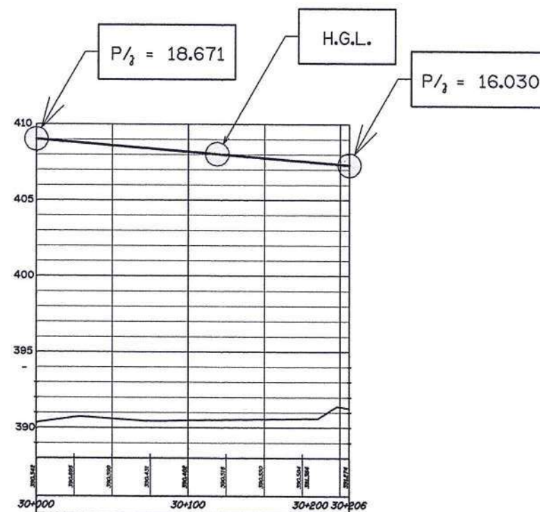
รูปตัดตามแนวยาวแสดง H.G.L. สาย 1R-2LMP STA. 30+000 - 30+206 ไม่แสดงขนาดจั่วหัว
