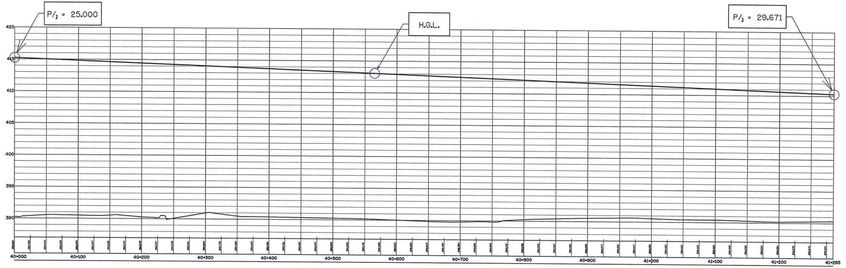
รูปตัดตามแนวยาวแสดง H.G.L. สาย 1LMP STA. 40+000 - 41+285 ไม่แสดงขนาดสวน
