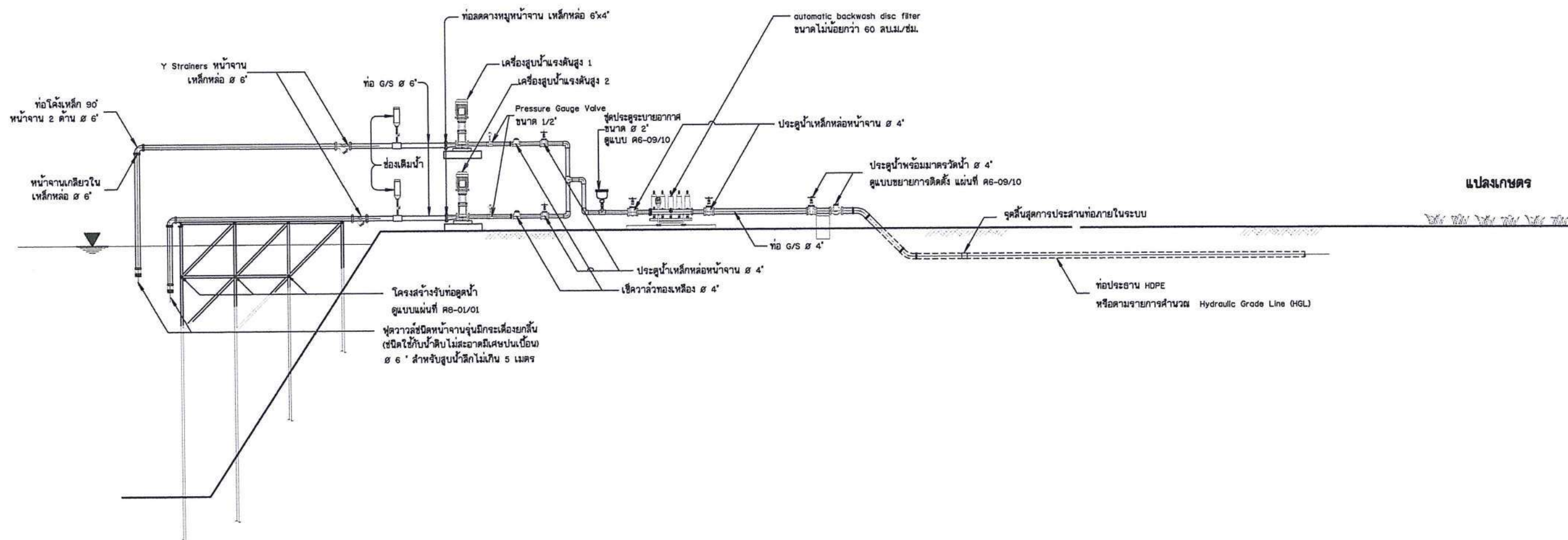
รูปแสดงรายละเอียดท่อและอุปกรณ์ระบบสูบน้ำพลังงานแสงอาทิตย์ ไม่แสดงมาตราส่วน
