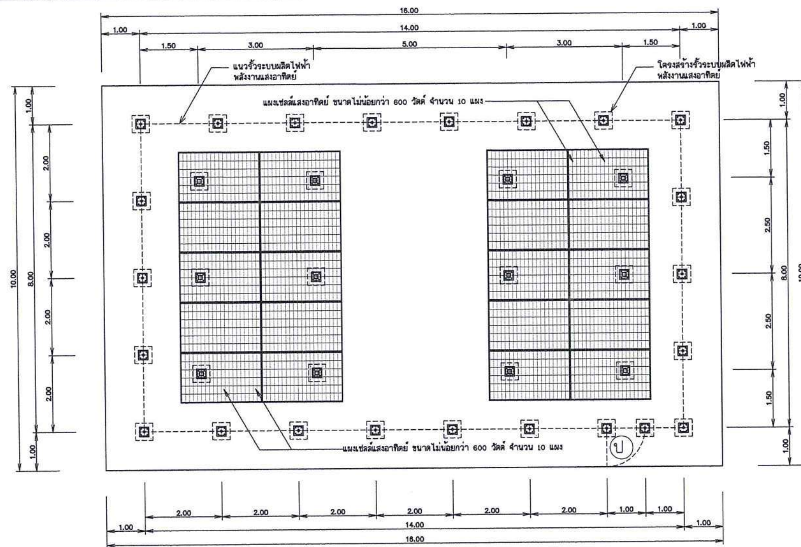
แปลนการติดตั้งแผงเซลล์แสงอาทิตย์ พร้อมรั้ว ไม่มีมาตราส่วน
