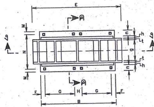
แปลนคูกด้ารับท่อ (สำหรับท่อ Ø400 มม. - Ø1,200 มม.) ไม่แสดงขนาดส่วน
