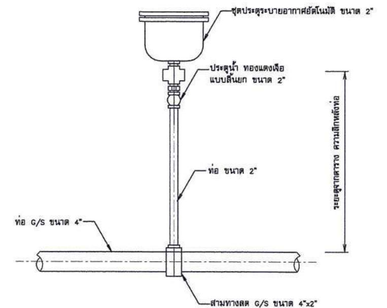
การติดตั้งประตูละบายอากาศอัตโนมัติ ไม่แสดงมาตราส่วน
