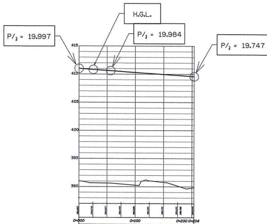
รูปตัดตามแนวยาวแสดง H.G.L. สาย 3LMP STA. 0+000 - 0+204 ไม่แสดงขนาดจั่วหัว
