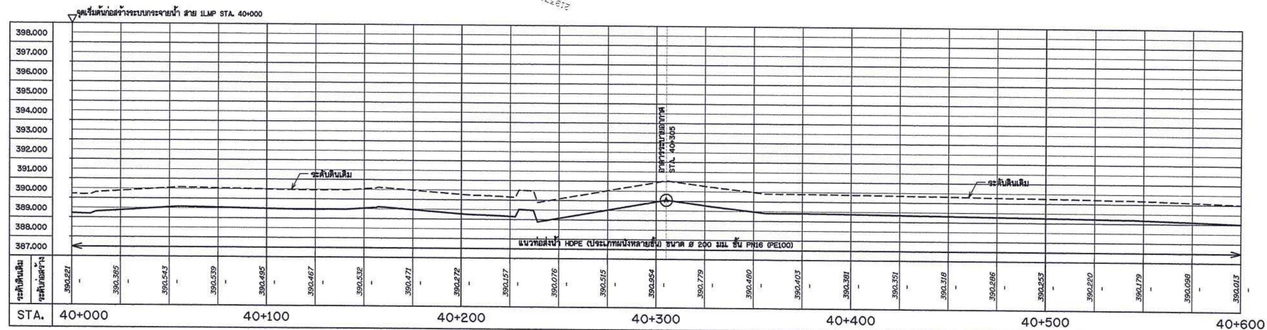
รูปตัดตามแนวยาว สาย 1LMP STA. 40+000 - 40+600
