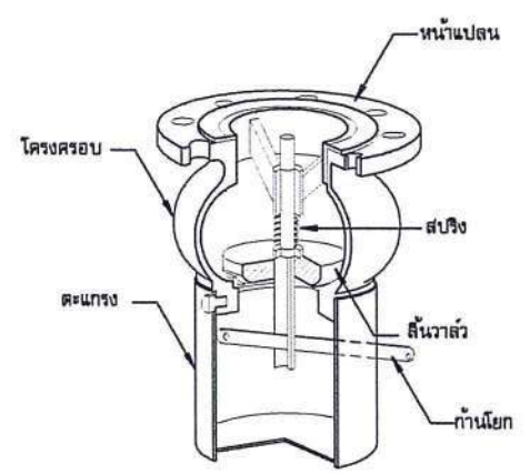
ฟลวาล์ว แบบก้านโยก ไม่แสดงมาตราส่วน
