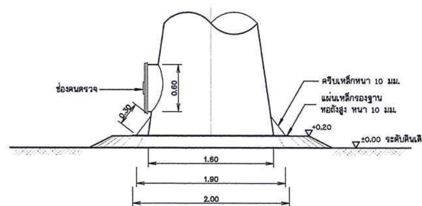
แบบขยายแมนโฮลล่างของท่อสูง
