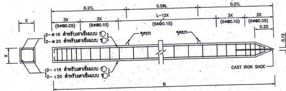
เสาเข็ม ค.ส.ล. ไม่แสดงขนาดบางส่วน
