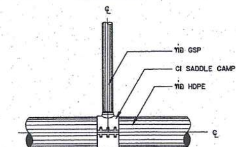
การบรรจุบ่อสามทาง HDPE กับท่อ GSP
