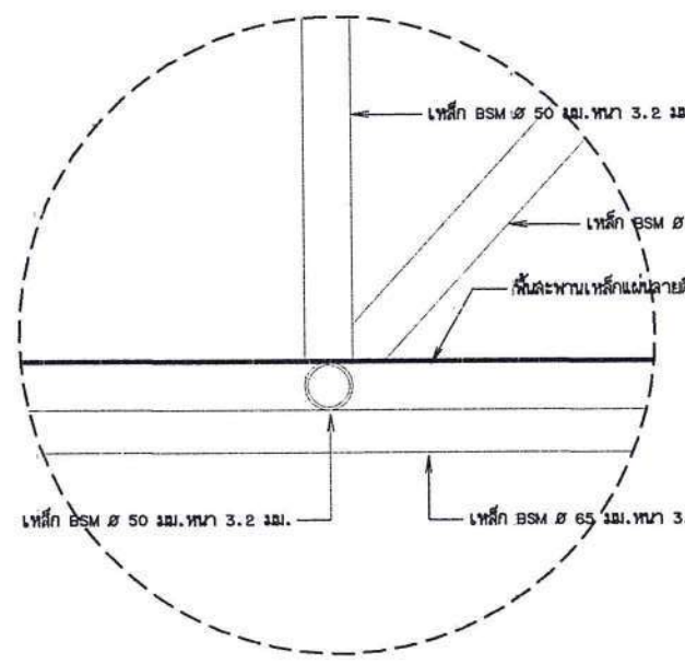
รูปขยาย 3
