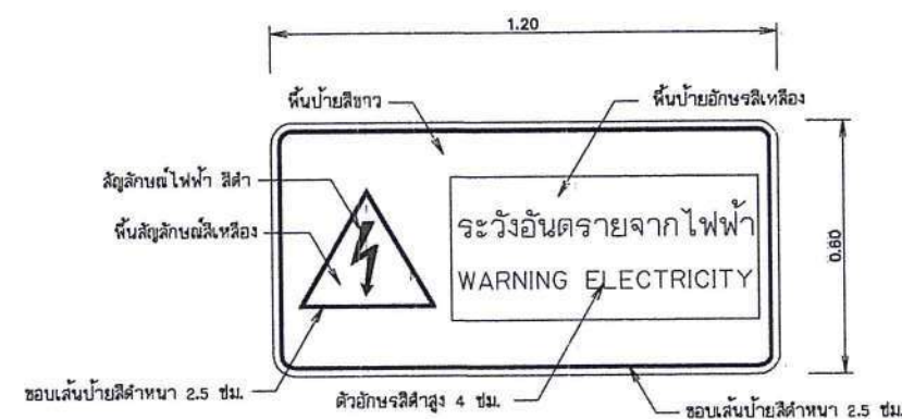
ป้ายเตือนกระแสไฟฟ้า ไม่แสดงมาตราส่วน
