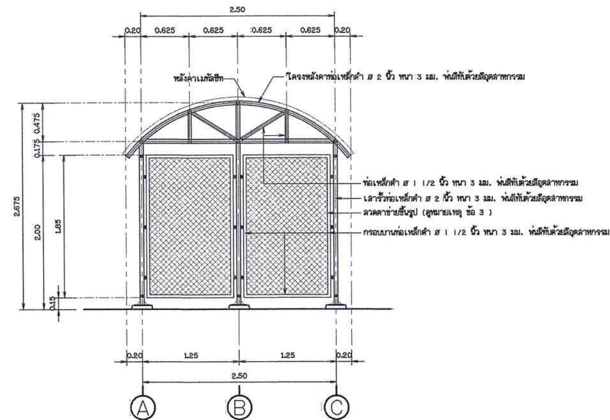
รูปตัด ข - ข (อาคารโรงสูบน้ำ) ไม่แสดงขนาดราวล้วน
