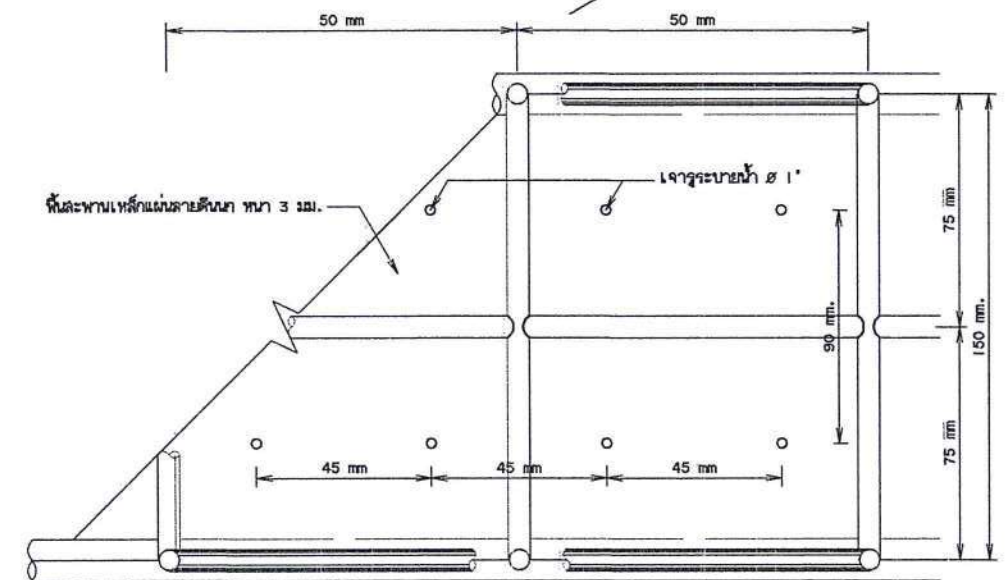
แบบขยายโครง พื้นสะพาน มาตรฐาน 1:10
