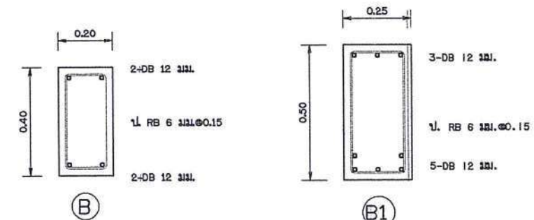
แบบขยายคาน คสล.
