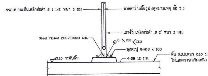
รูปขยายฐานรากโครงสร้างอาคารโรงสูบน้ำ (ต่อหน้า คสล. หล่อสำเร็จรูปพร้อมติดตั้ง) ไม่แสดงมาตราส่วน
