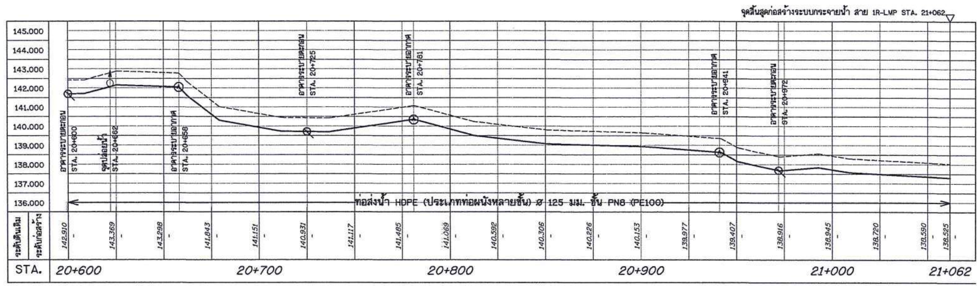
รูปตัดตามแนวยาวระบบกระจายน้ำ สาย 1R-LMP มาตราส่วน 1:1,000
