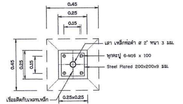
ฐานรากโครงสร้างอาคารโรงสูบน้ำ ไม่แสดงมาตราส่วน
