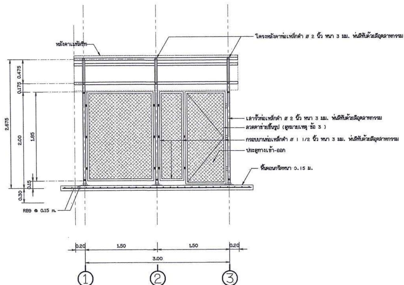
รูปตัด ก - ก (อาคารคลุมตู้ควบคุมเครื่องสูบน้ำ , กรองเกษตร) ไม่แสดงขนาดราวล้วน
