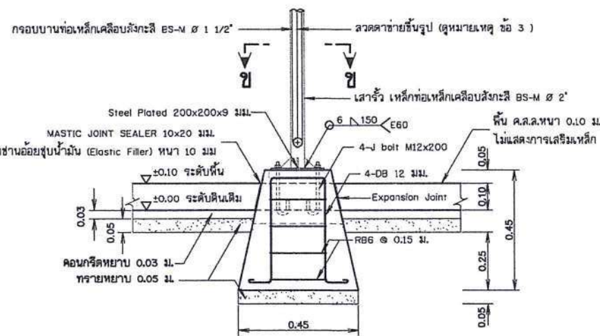
รูปขยายฐานรากโครงสร้างรับแผง F1 (คอม่อ คสส. หล่อสำเร็จรูปพร้อมติดตั้ง) ไม่แสดงมาตราส่วน
