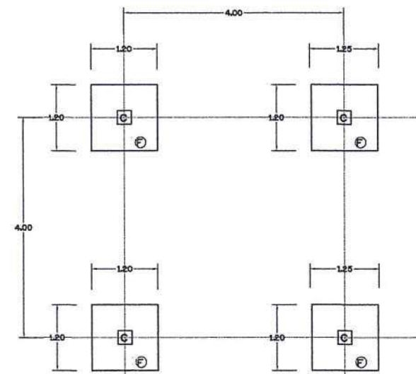
แปลนแสดงฐานราก , เสา คสล.
