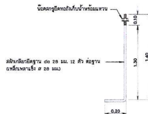
แบบขยายหลักเหล็กรายยัดฐาน
