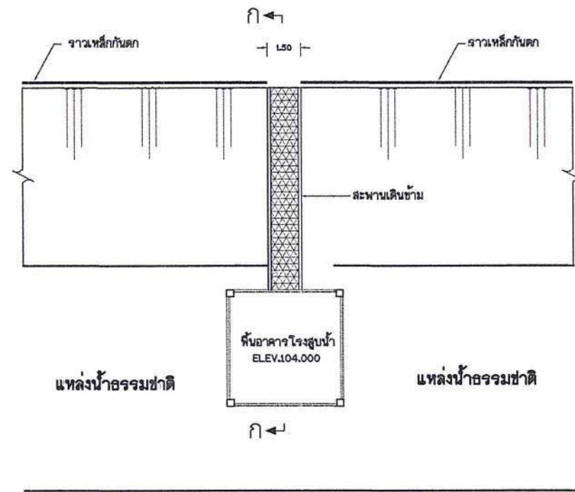
แปลนแสดงอาคารโรงสูบน้ำ
