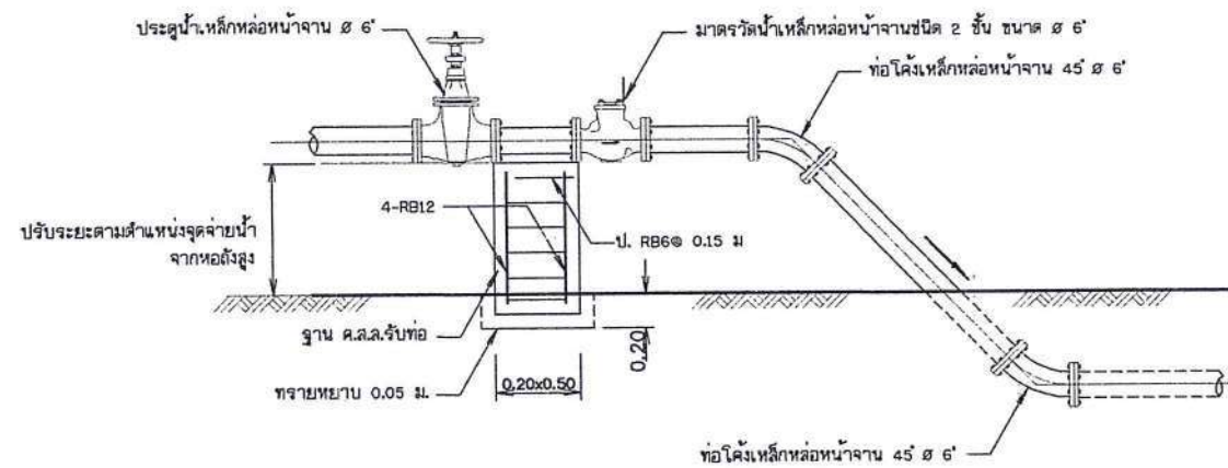
13. การติดตั้งมาตรวัดน้ำบนพื้นดิน ๕ ๖' ไม่แสดงมาตราส่วน
