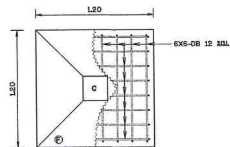
แบบขยายฐานราก F
