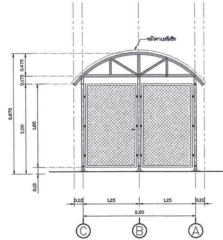
รูปด้าน 2 โมเดลขนาดจริง
