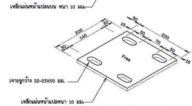
แบบขยายแผ่นเหล็กโครงหัวเสา
