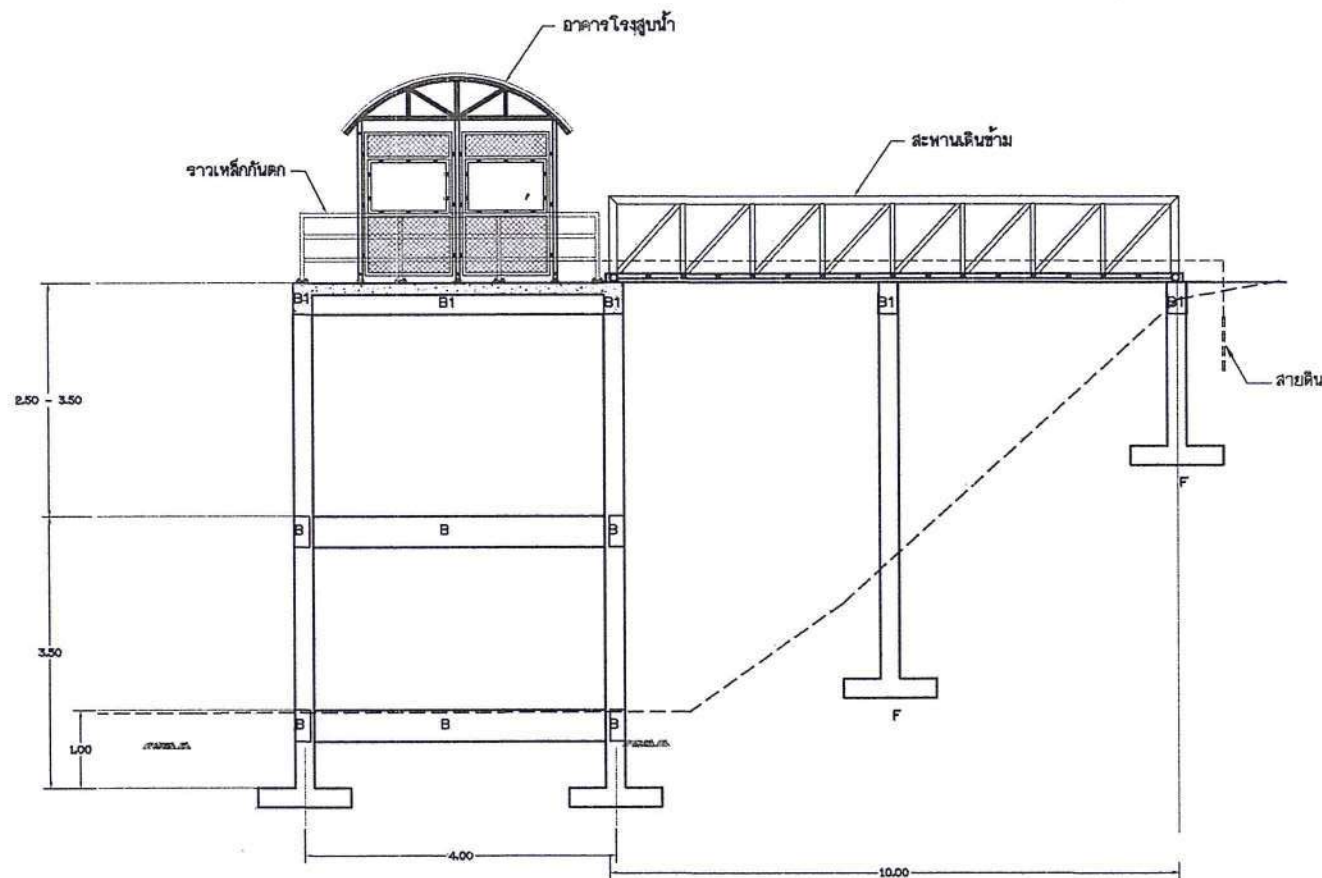
รูปตัดแนว ก - ก
