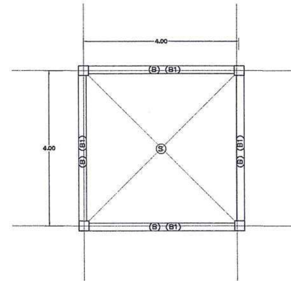
แปลนแสดง คาน เสา พื้น คสล.
