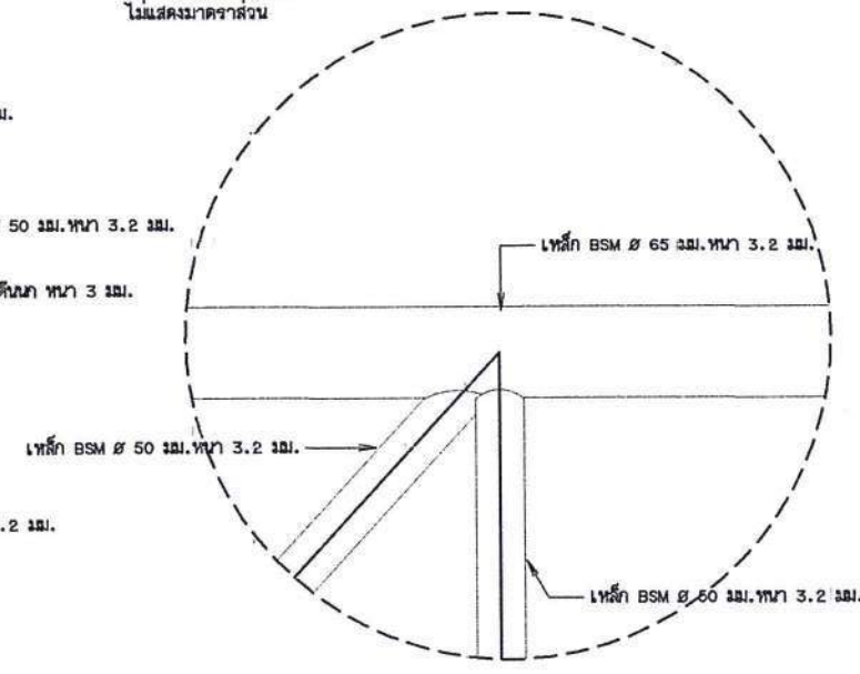
รูปขยาย 2
