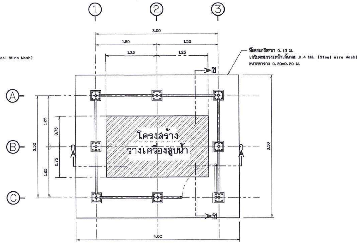
แปลนเสาและรั้ว ไม่แสดงขนาดราส่วน
