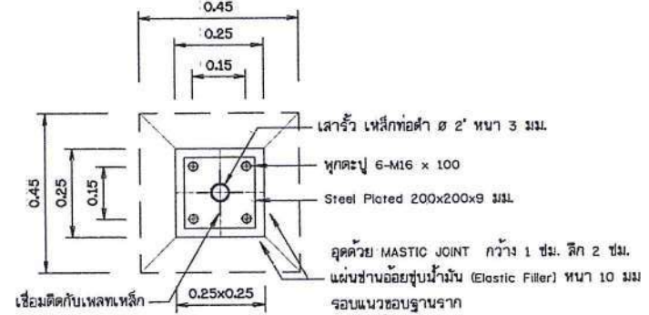
ฐานรากโครงสร้าง อาคารคลุมตู้ควบคุมเครื่องสูบน้ำ , กรองเกษตร ไม่แสดงมาตราส่วน
