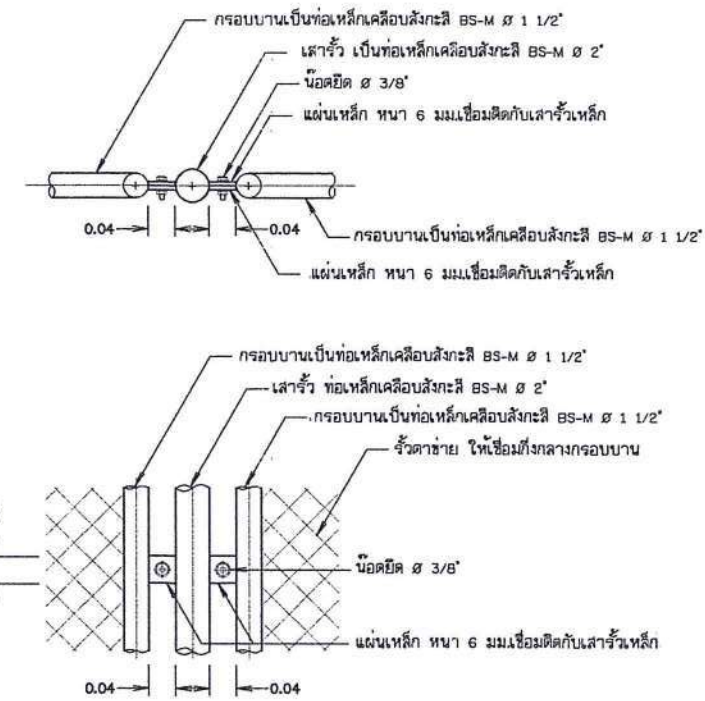
แบบขยายรายละเอียดแสดงการยึดระหว่างจั่วกับเล้า ไม่แสดงมาตราส่วน
