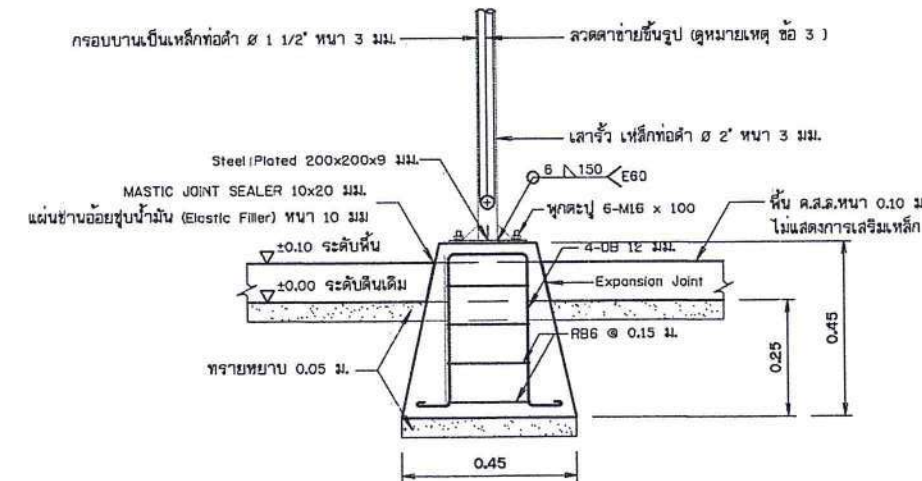
รูปขยายฐานรากโครงสร้างอาคารคลุมตู้ควบคุมเครื่องสูบน้ำ , กรองเกษตร (ต่อหน้า คสล. หล่อสำเร็จรูปพร้อมติดตั้ง) ไม่แสดงมาตราส่วน
