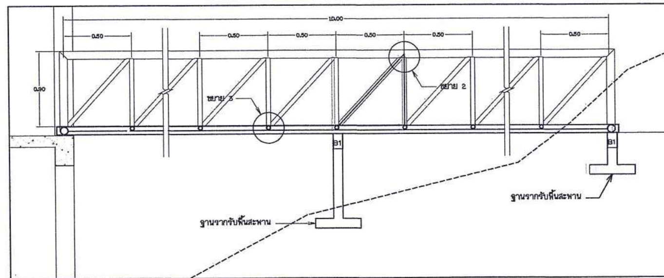
รูปตัดแนว A - A ไม่แสดงขนาดจั่วส่วน
