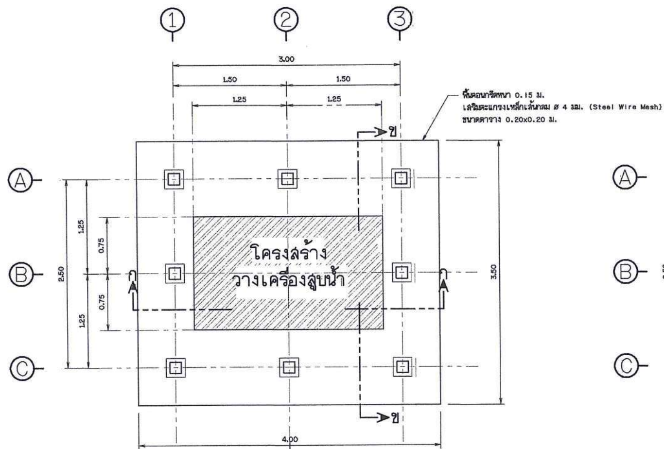
แบบแปลน ไม่แสดงขนาดราส่วน
