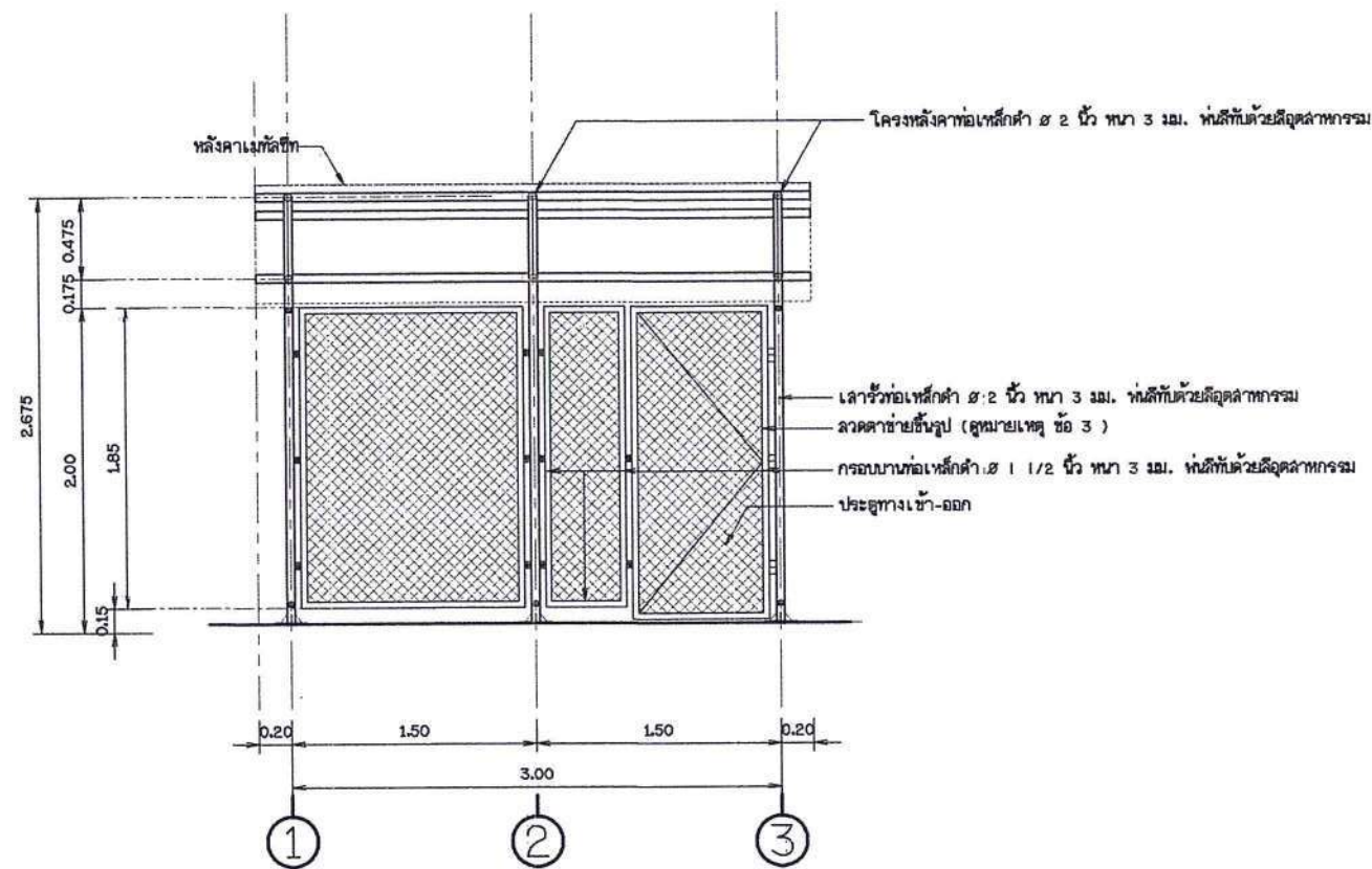
รูปตัด ก - ก (อาคารโรงสูบน้ำ) ไม่แสดงขนาดราวล้วน
