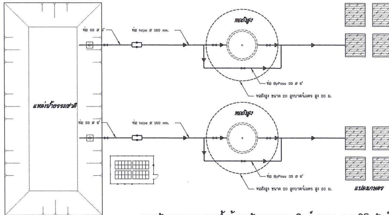
แผนผังระบบกระจายน้ำด้วยพลังงานแสงอาทิตย์ ขนาด 7.5 กิโลวัตต์
