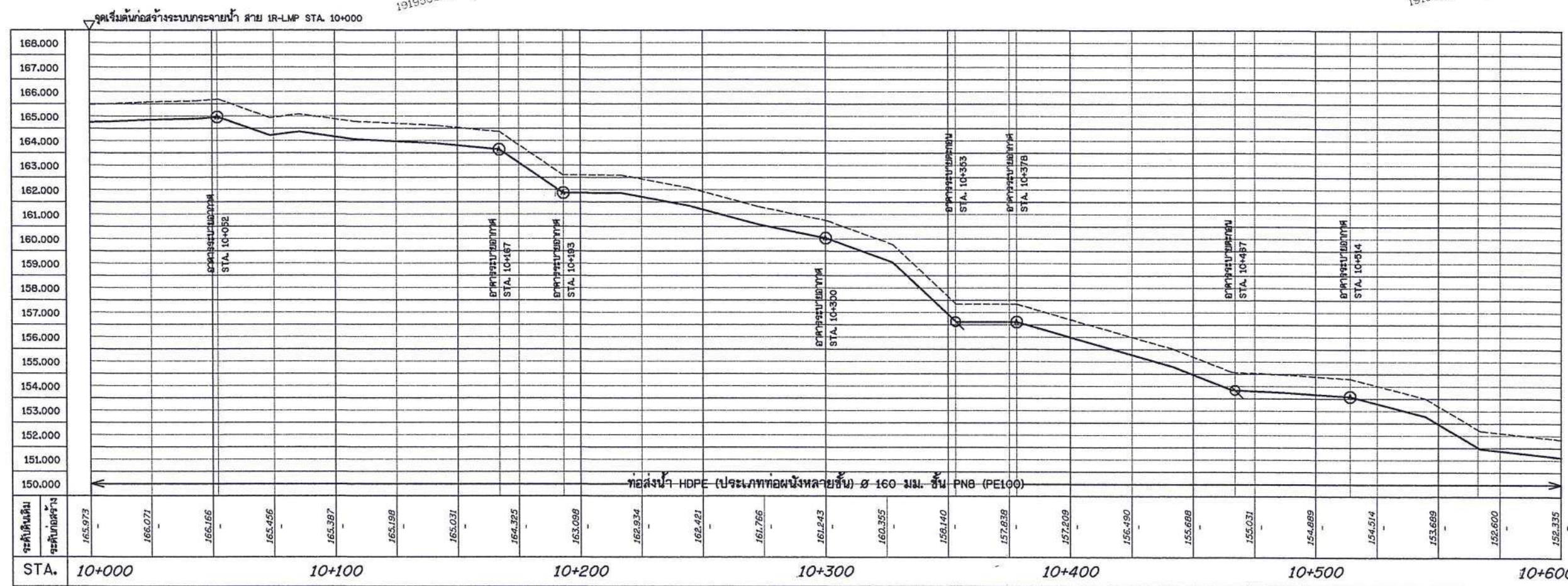
รูปตัดตามแนวยาวระบบกระจายน้ำ สาย RMP
