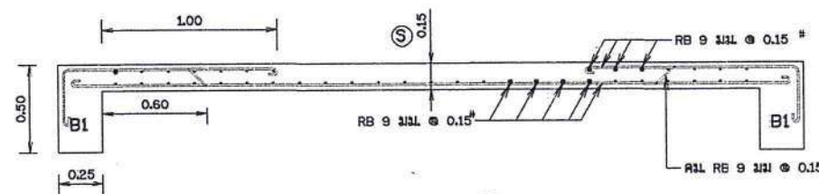
แบบขยายพื้น คสล.
