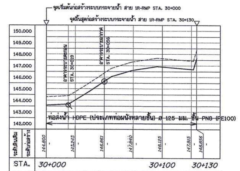
รูปตัดตามแนวยาวระบบกระจายน้ำ สาย 1R-RMP มาตราส่วน 1:1,000
