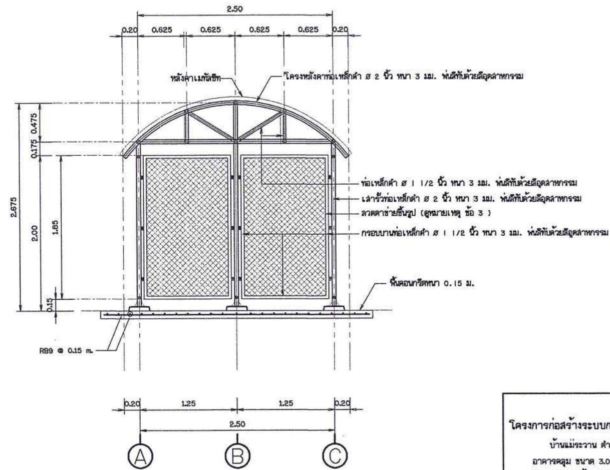
รูปตัด ข - ข (อาคารคลุมตู้ควบคุมเครื่องสูบน้ำ , กรองเกษตร) ไม่แสดงขนาดราวล้วน
