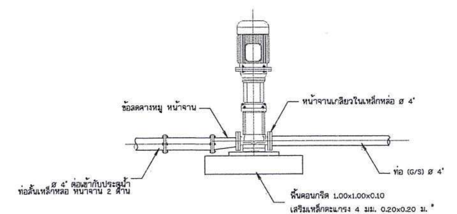
15. การต่อท่อเครื่องสูบน้ำ ไม่แสดงมาตราส่วน
