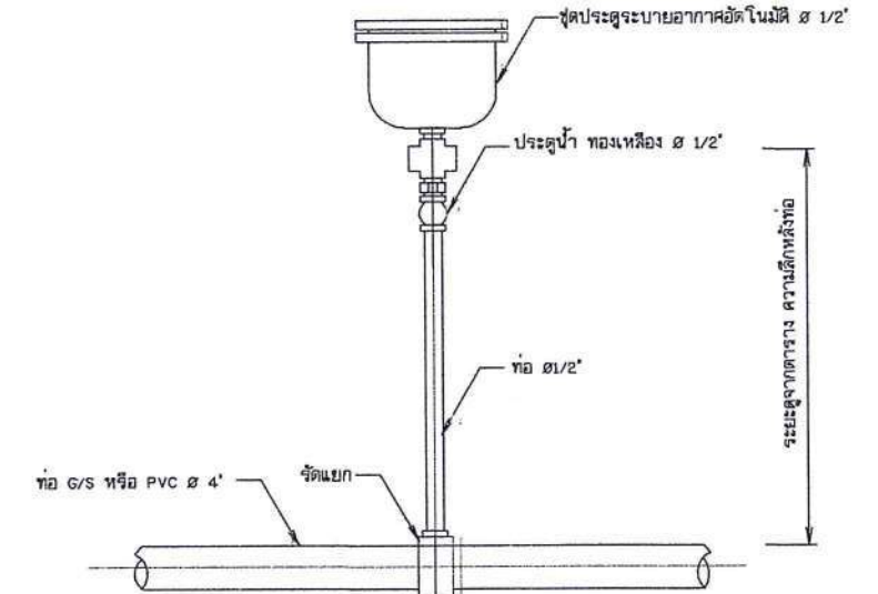
12. การติดตั้งประตูละบายอากาศอัด โนมิต ไม่แสดงมาตราส่วน
