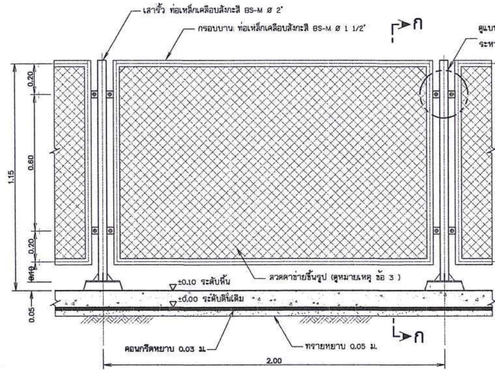
แบบขยายจั่วลวดตาข่าย ไม่แสดงมาตราส่วน
