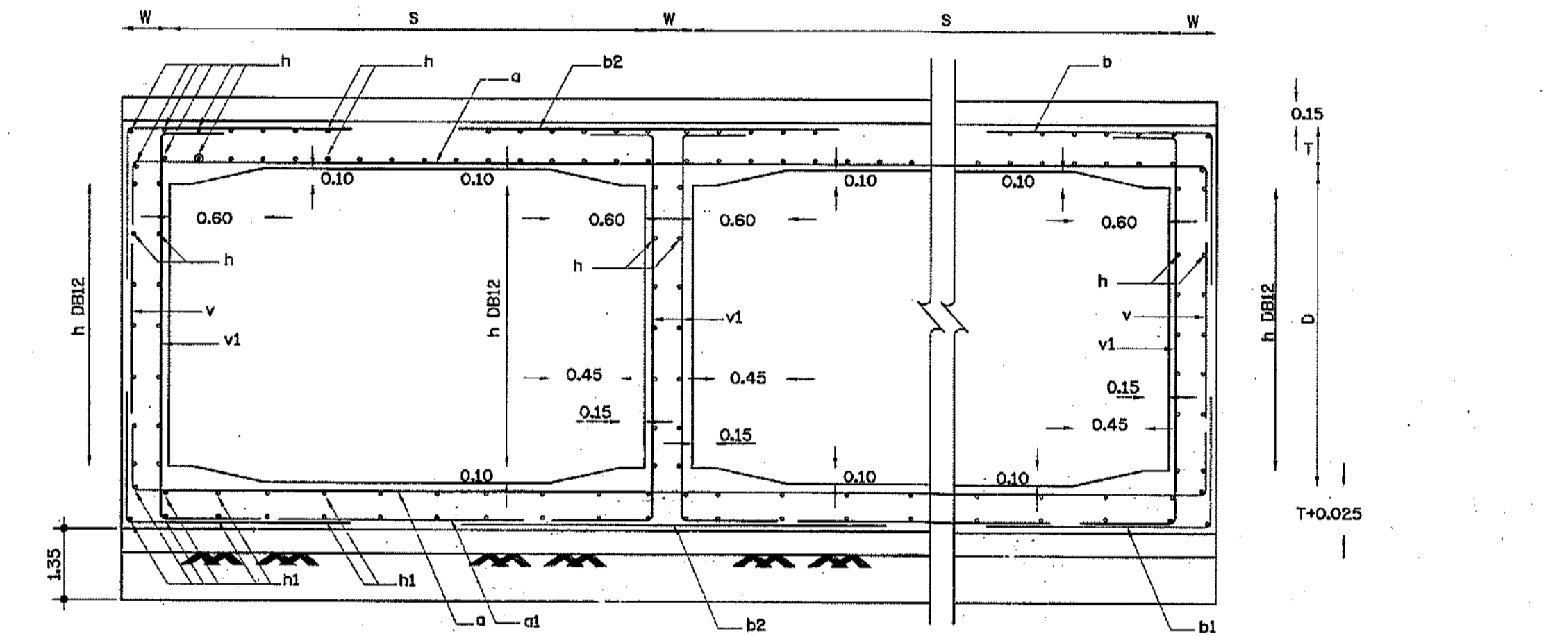
รูปตัด (1)-(1) NOT TO SCALE
