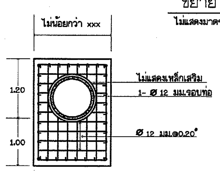
ขยายการเสริมเหล็กกำแพงปากท่อและท้ายท่อ (HEAD WALLS) ไม่แสดงขนาดจาล้วน
