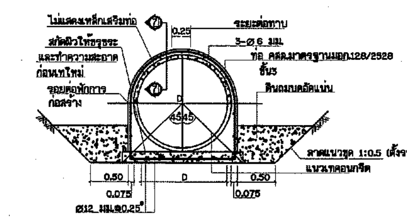
รูปตัดการวางท่อ คสล. ไม่แสดงขนาดจาล้วน
