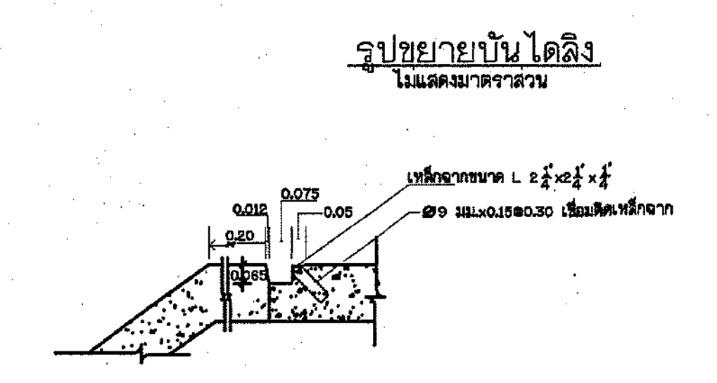
ขยายร่องใส่บานประตูไม้ ไม่แสดงขนาดจาล้วน
