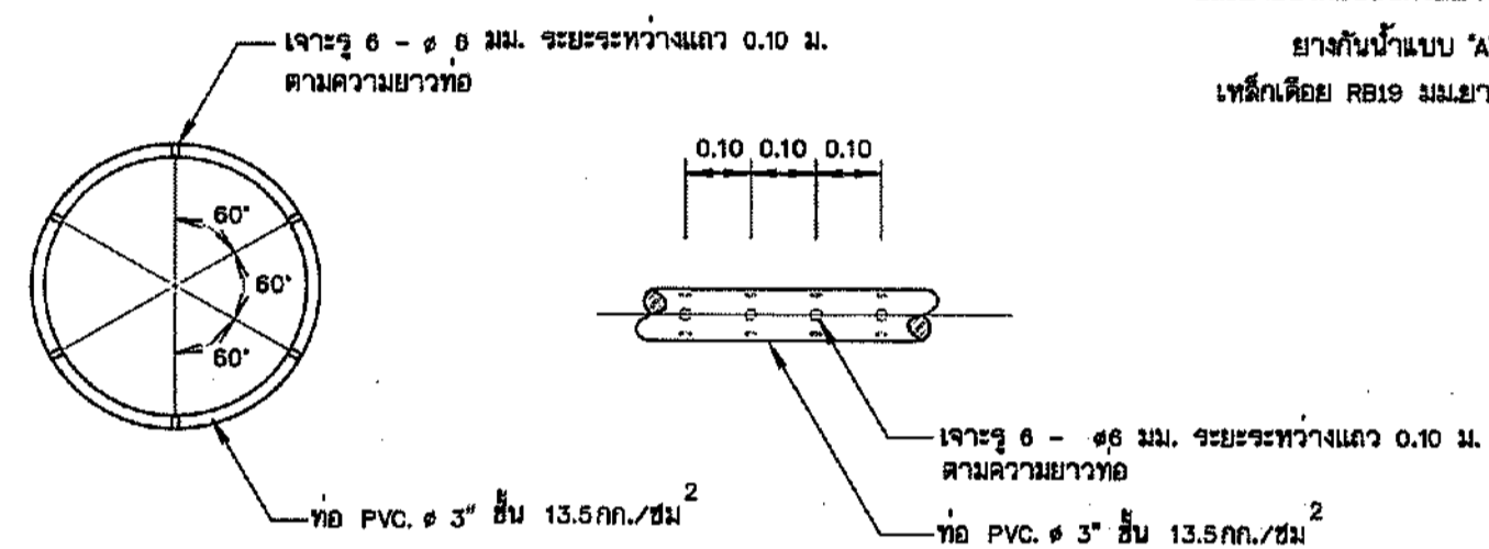
รูปขยายเจาะรูท่อ
