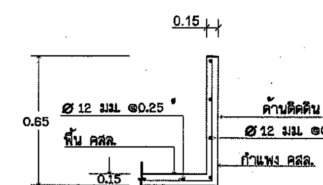
รูปตัด ๑-๑ (ความหนาพื้น 0.15 ม.) ไม่แสดงขนาดจาล้วน
