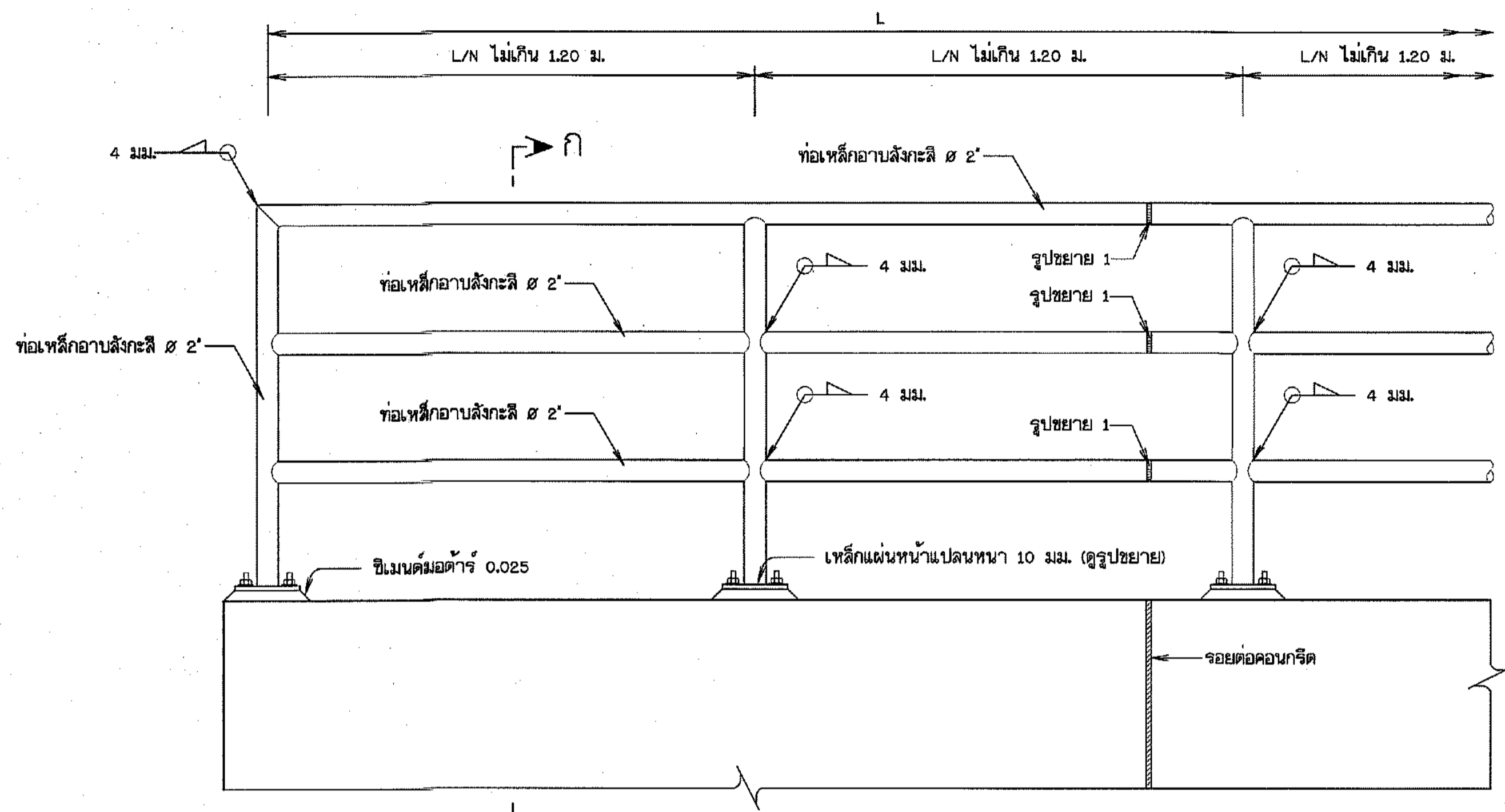
รูปขยายราวเหล็กกันดก
