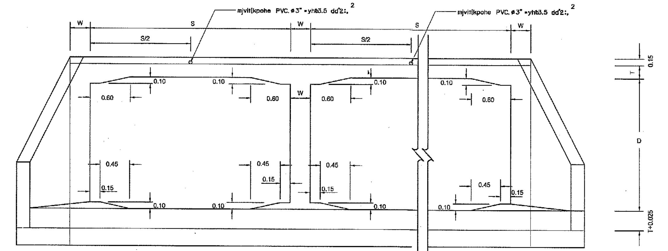
รูปตัดด้านหน้า NOT TO SCALE
