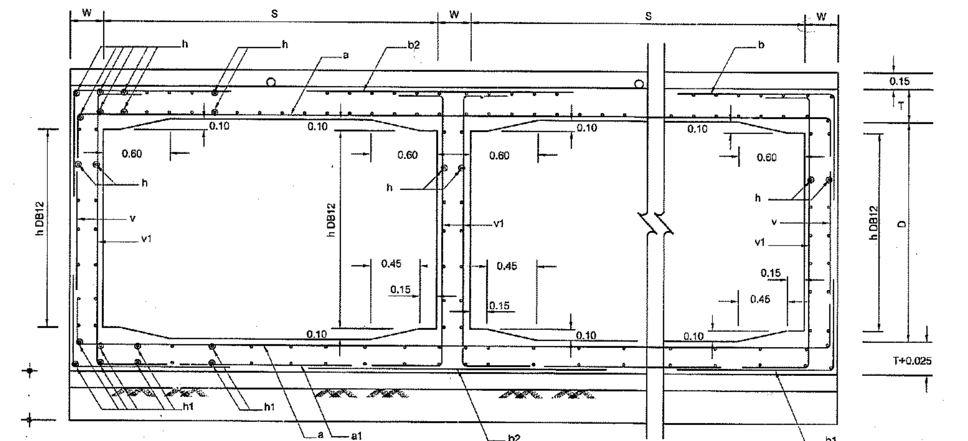
รูปตัด (1)-(1) NOT TO SCALE
