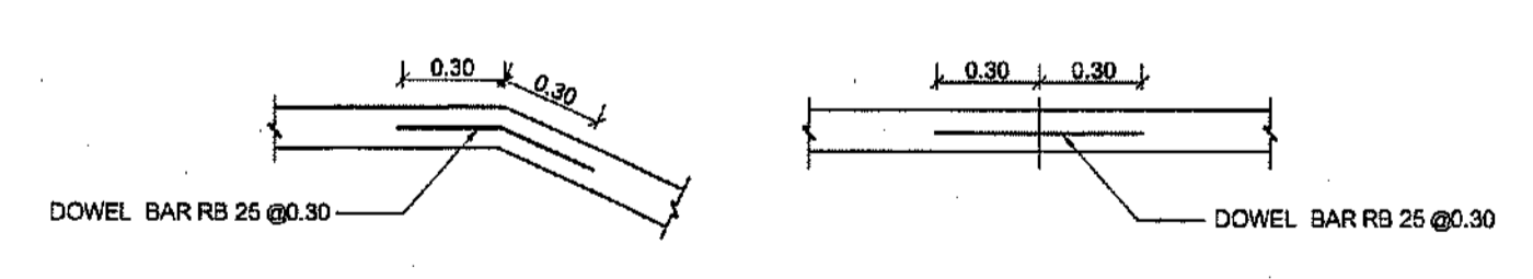
รายละเอียด (ด) ไม่แสดงมาตราส่วน
