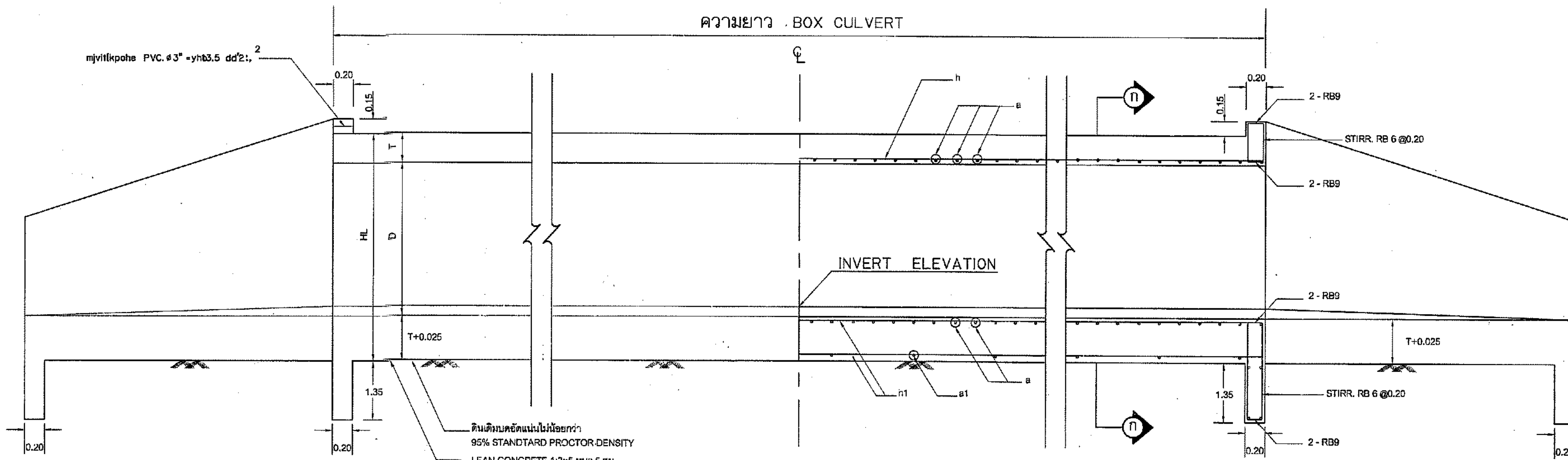
ความยาว BOX CULVERT
