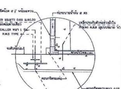
รูปขยาย '3'
