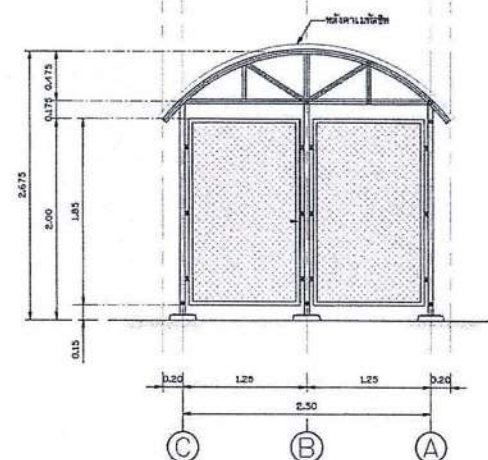
รูปด้าน 4 ไม่แสดงขนาดฐาน
