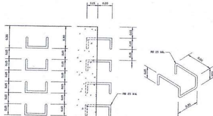
รูปขยายบันไดลง
