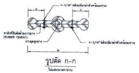
รูปตัด ก-ก ไม่ลดขนาดส่วน
