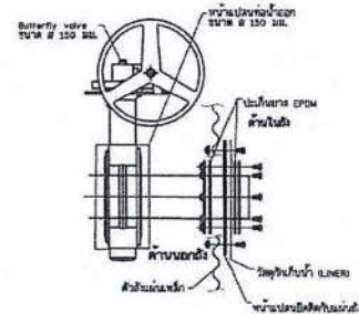
แบบขยาย 7 Scale NTC
