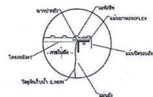
แบบขยาย 3-จุดยึดหลังคาแบบไม้ Scale NTC
