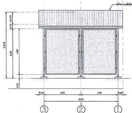
รูปด้าน 3 ไม่แสดงขนาดฐาน
