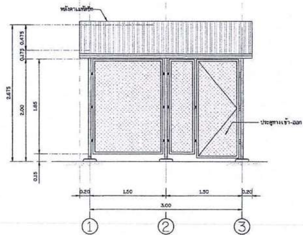
รูปด้าน 1 ไม่แสดงขนาดฐาน
