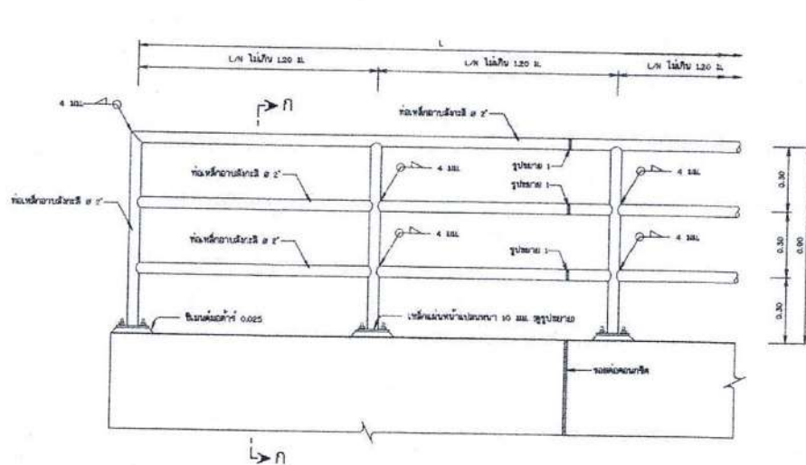
รูปขยายจาวหลักกันตก
