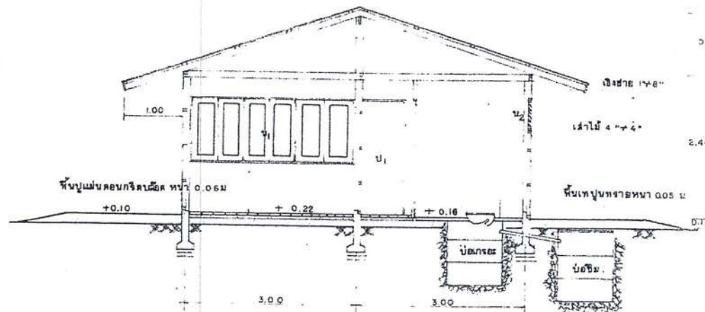
รูปตัด 1850
