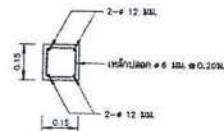
รูปตัด ก - ก
