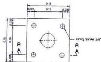
รูปขยายแผ่นหลักหน้าแปลน
