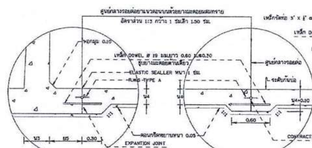
รูปขยาย '1'
