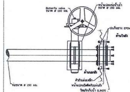
แบบขยาย 4 Scale NTC
