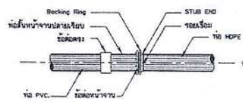
การบรรจุท่อพีวีซี (PVC) กับท่อ HDPE.
