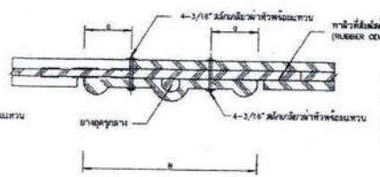
รูปตัด จ-จ ไม่ลดขนาดส่วน
