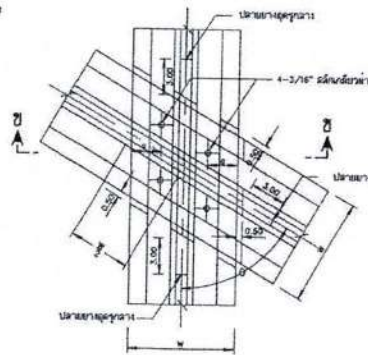
การต่อพาดทับกันไม่ทำมุมฉาก ไม่ลดขนาดส่วน
