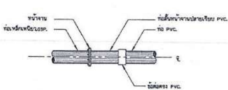
การบรรจุท่อเหล็กเหนียวหรือ GSP. กับท่อ PVC.
