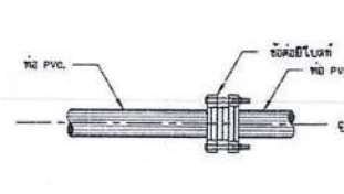
การบรรจุท่อ PVC. กับท่อ PVC.
