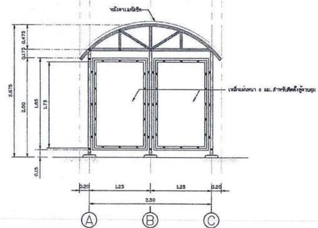
รูปด้าน 2 ไม่แสดงขนาดฐาน
