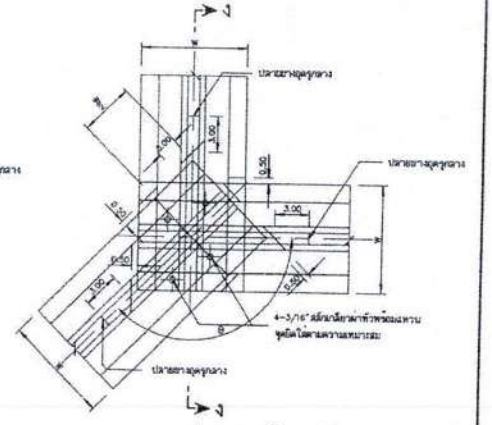
การต่อมุมกันทั้ง 3 ชั้น ไม่ลดขนาดส่วน
