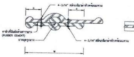
รูปตัด ข-ข ไม่ลดขนาดส่วน
