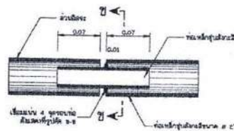
รูปขยาย 1
