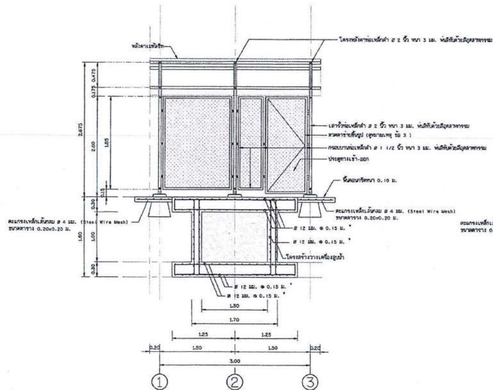
รูปตัด ก - ก ไม่แสดงขนาดส่วน
