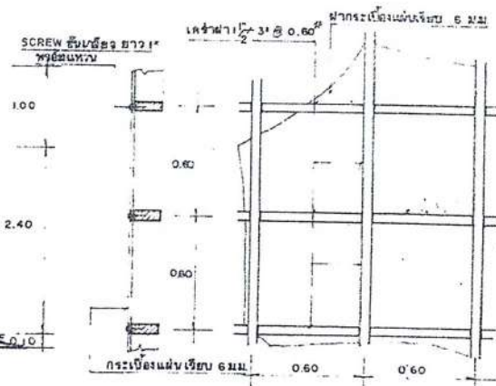
รูปขยายโครง, ฝา 1820
