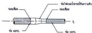
การบรรจุท่อ HDPE. กับข้อต่อ HDPE.
