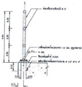
รูปตัด ก-ก
