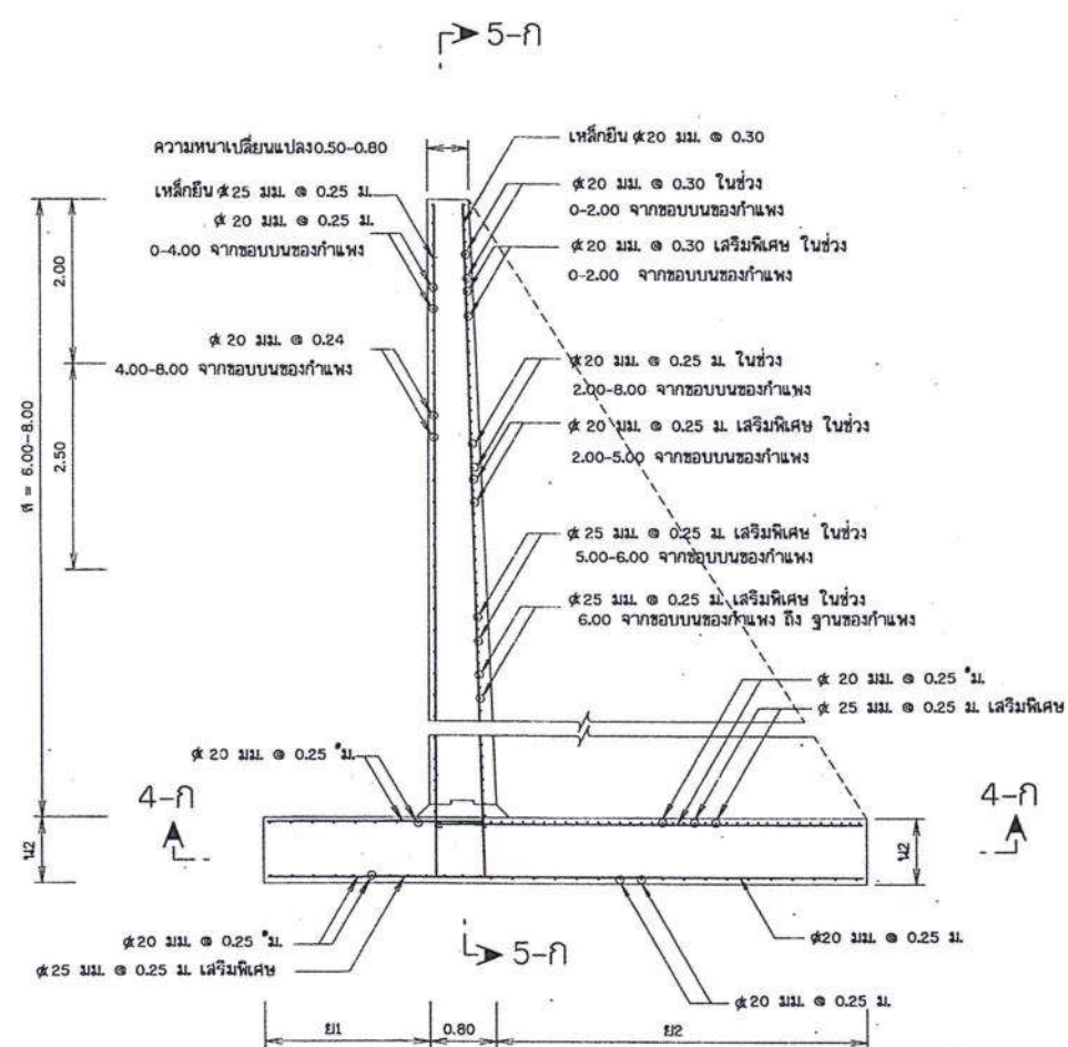
รูปตัด ก-ก (ใกล้ค่ายัน)
