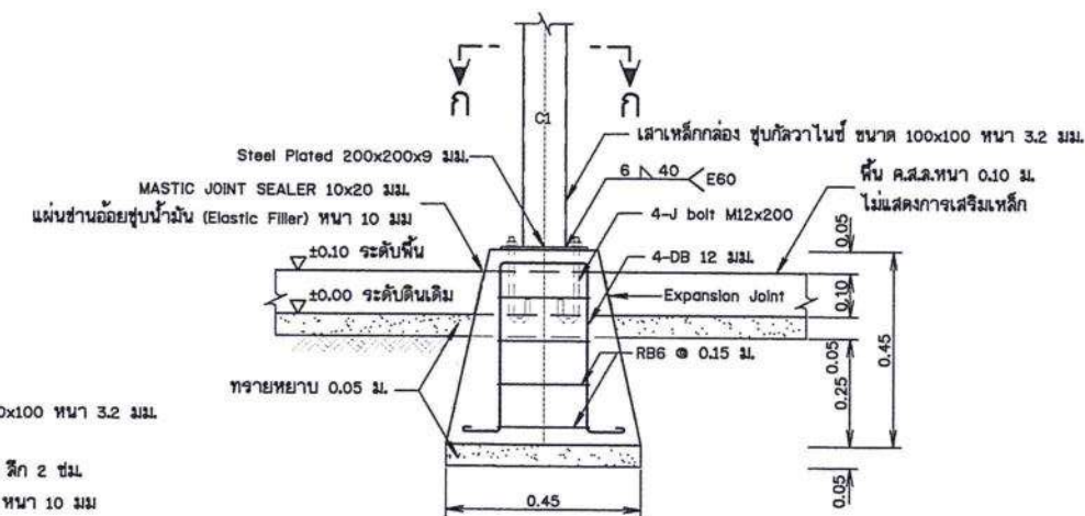
รูปขยายฐานรากโครงสร้างรับแรง F1
