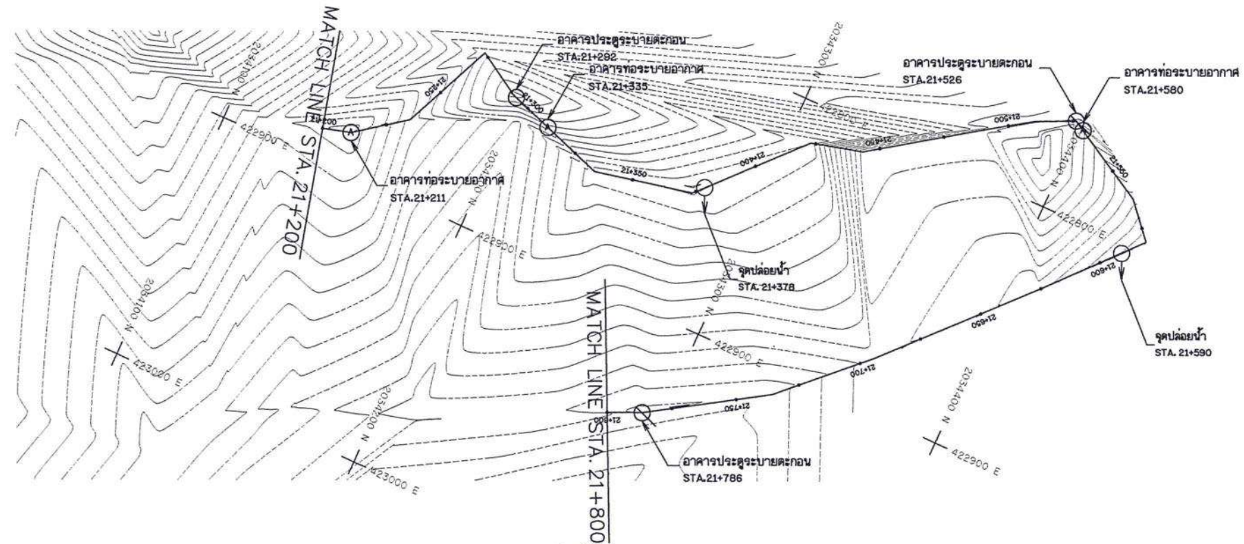
แปลนระบบส่งน้ำ
