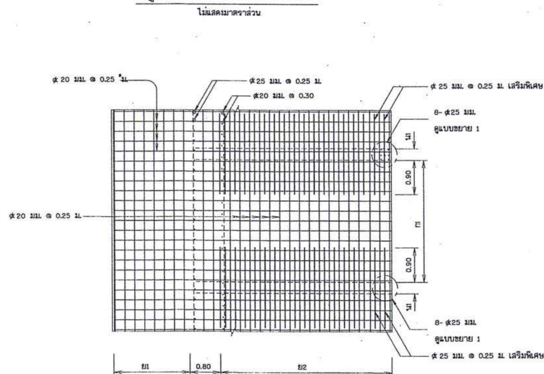
รูปตัด ก-ก (ใกล้ค่ายัน)
