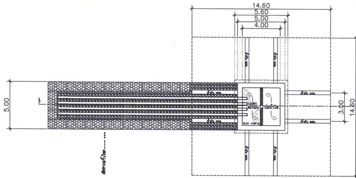
แปลนแสดงทางน้ำเข้าสู่อาคารบ่อสูบ
