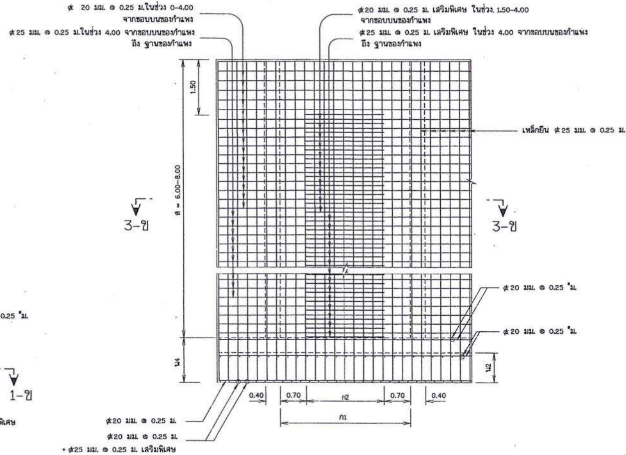
รูปตัด 2-ข (ด้านไม่ติดดิน) ไม่แสดงขนาดราส่วน
