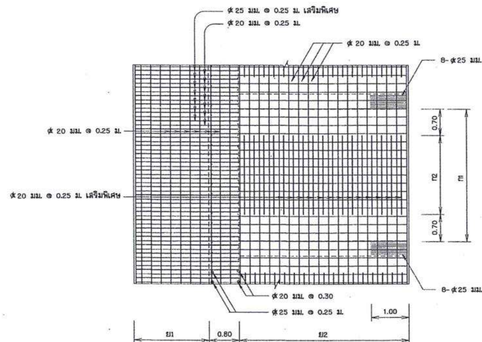
รูปตัด 1-ข (พื้นด้านล่าง) ไม่แสดงขนาดราส่วน
