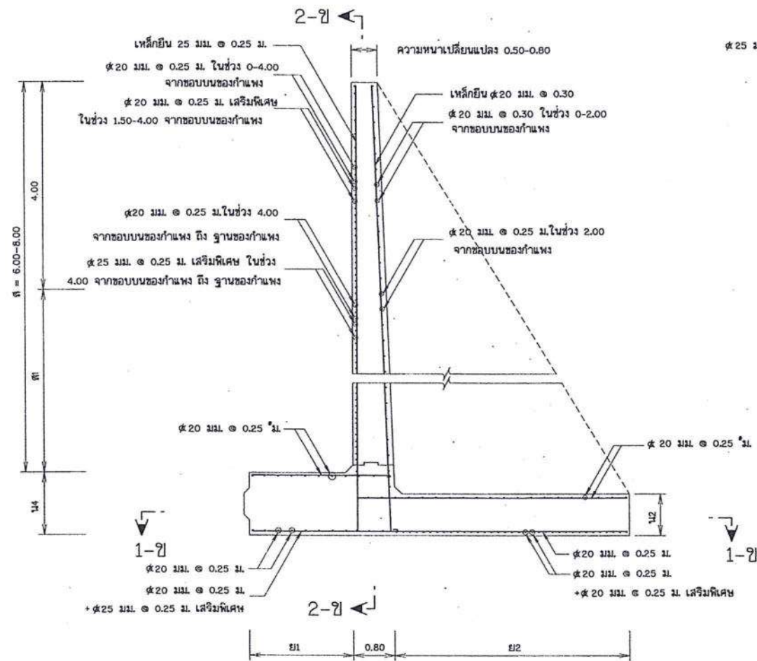
รูปตัด 2-ข (ที่กึ่งกลางช่วง) ไม่แสดงขนาดราส่วน
