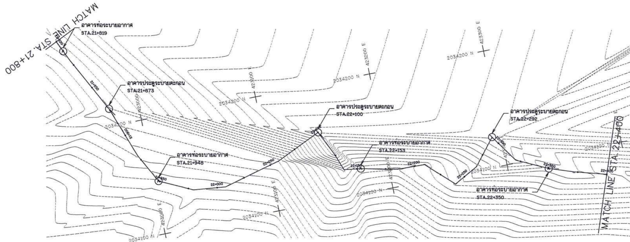
แปลนระบบส่งน้ำ
