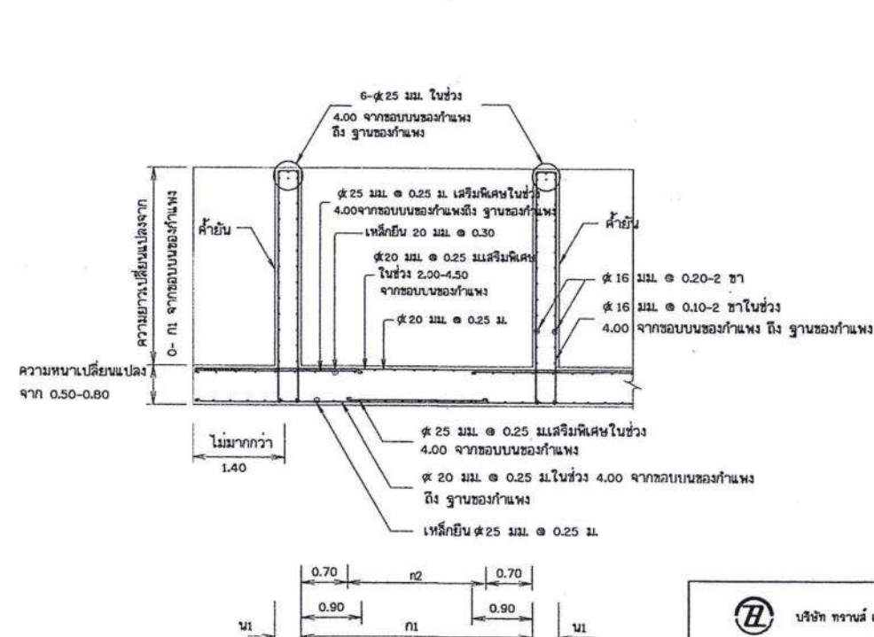
รูปตัด 3-ก
