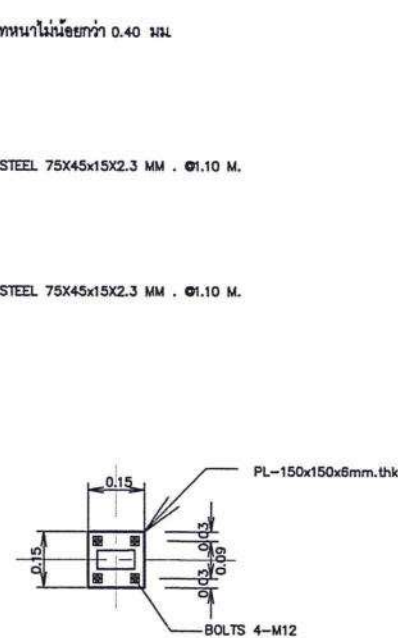
รูปด้าน 1
