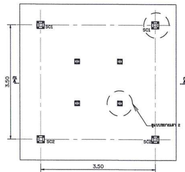
แปลนเสาอาคารโรงสูบน้ำ
