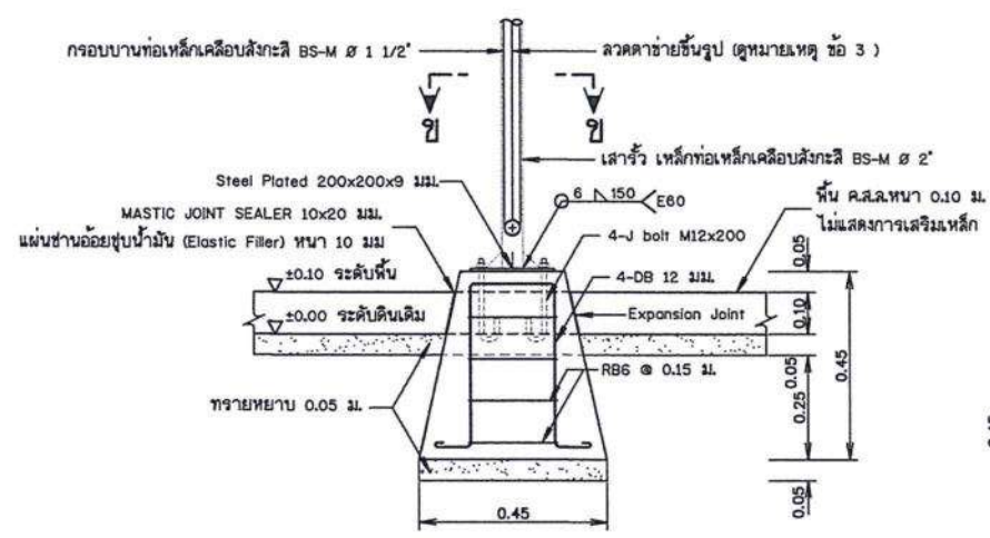
รูปขยายฐานรากโครงสร้างรับแผง F1 (เดมอ คสล. หล่อสำเร็จรูปพร้อมติดตั้ง) ไม่แสดงมาตราส่วน
