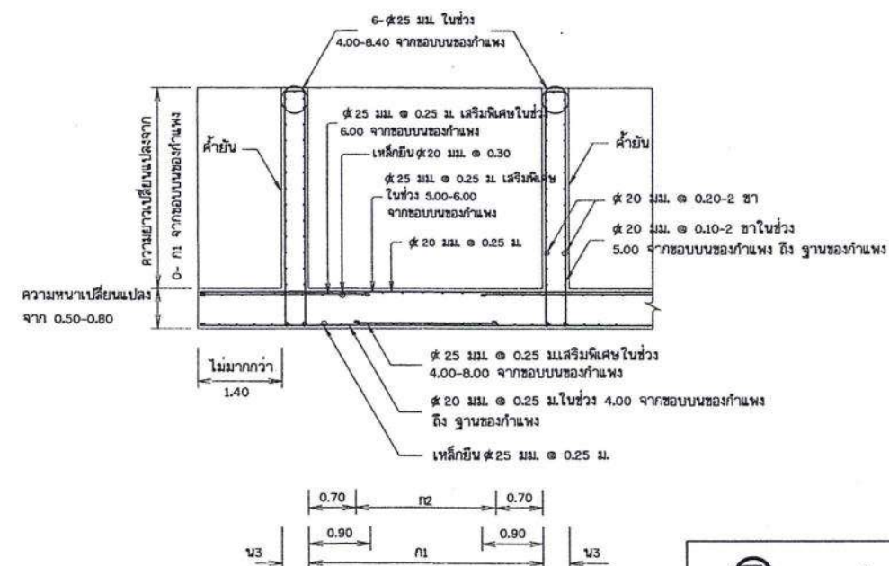
รูปตัด 3-ข ไม่แสดงขนาดราส่วน
