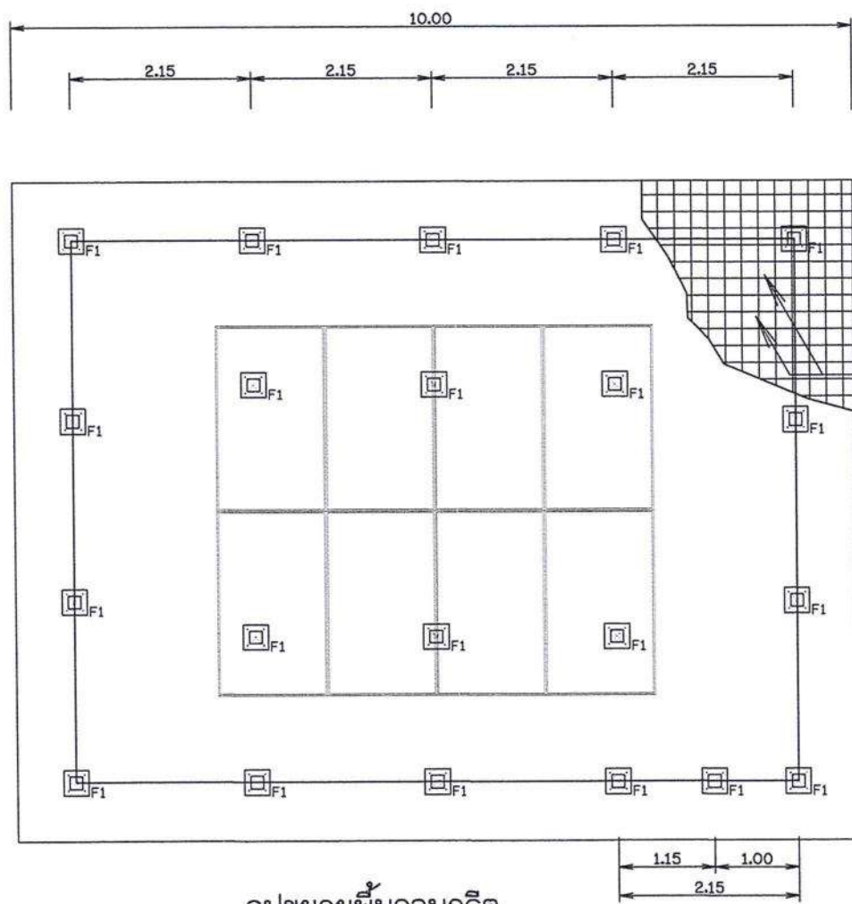
แปลนฐานรากและโครงหลังคา ไม่แสดงขนาดจั่วส่วน
