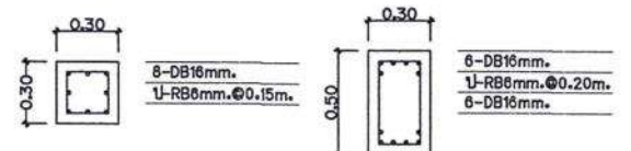
รูปตัดเสา CW
