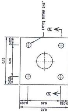
รูปขยายแผนเหล็กหน้าแปลน
