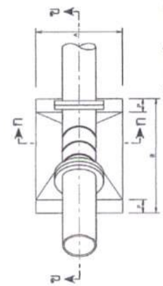
แปลน THRUST BLOCK รับข้อต่อโค้งแนวตั้ง
