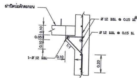
ขยาย 1 มาตราส่วน 1 : 10
