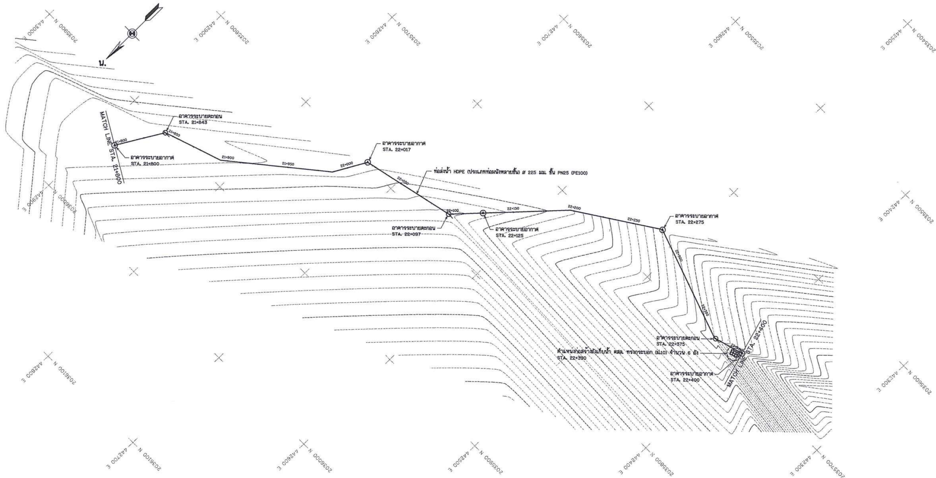
แปลนทั่วไประบบกระจายน้ำ สายที่ 1 มาตราส่วน 1:1,000
