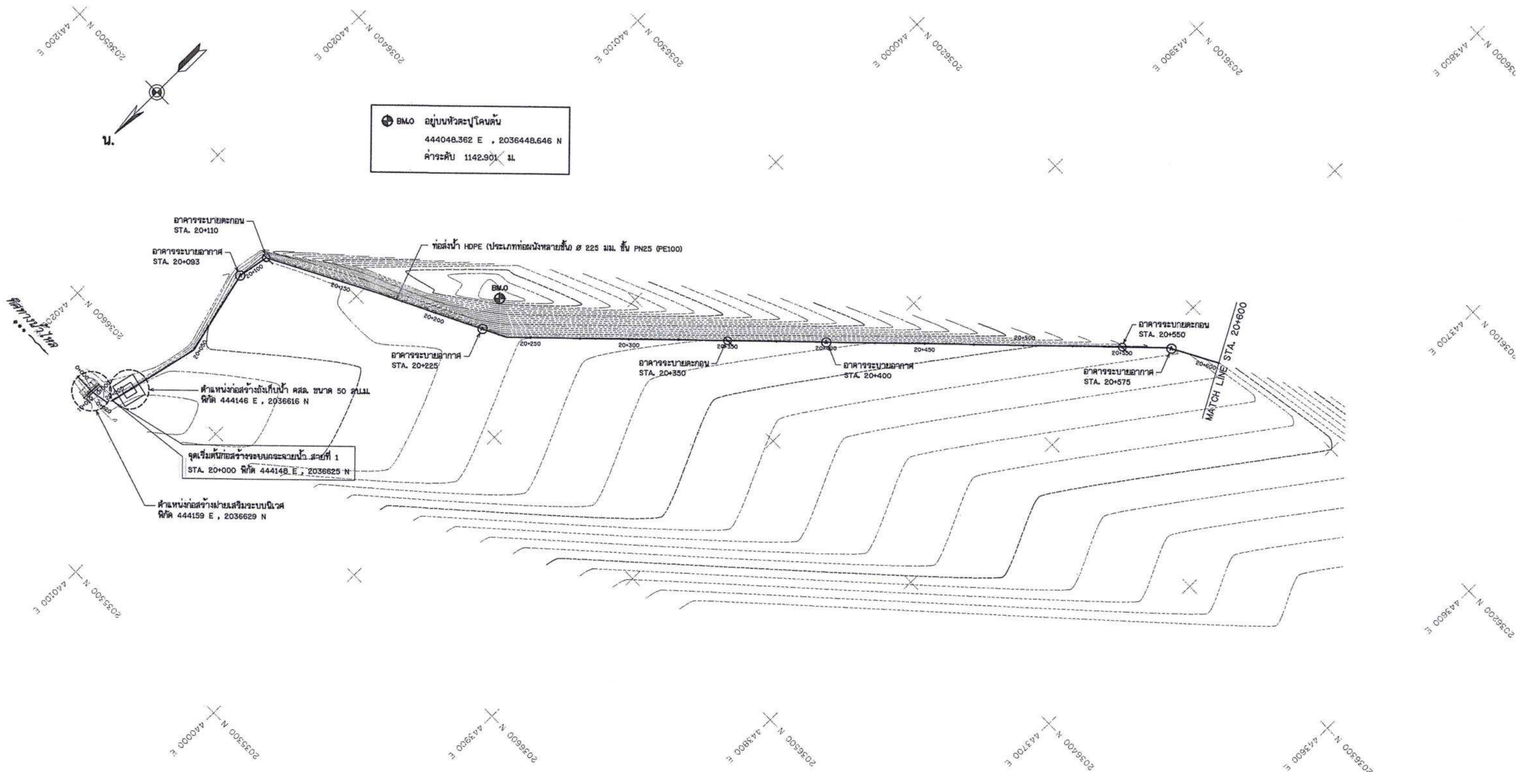
แปลนทั่วไประบบกระจายน้ำ สายที่ 1 มาตรฐาน 1:1,000
