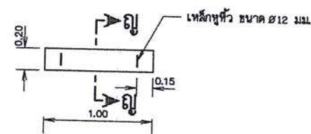
แปลนฝาบ่อตกตะกอน มาตราส่วน 1 : 10
