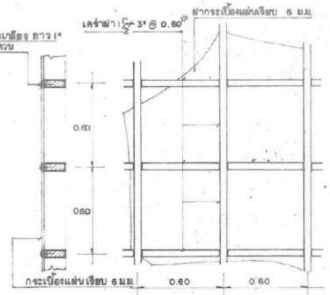
รูปขยายโครง, ฝา 1820
