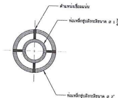
รูปตัด ย-ย
