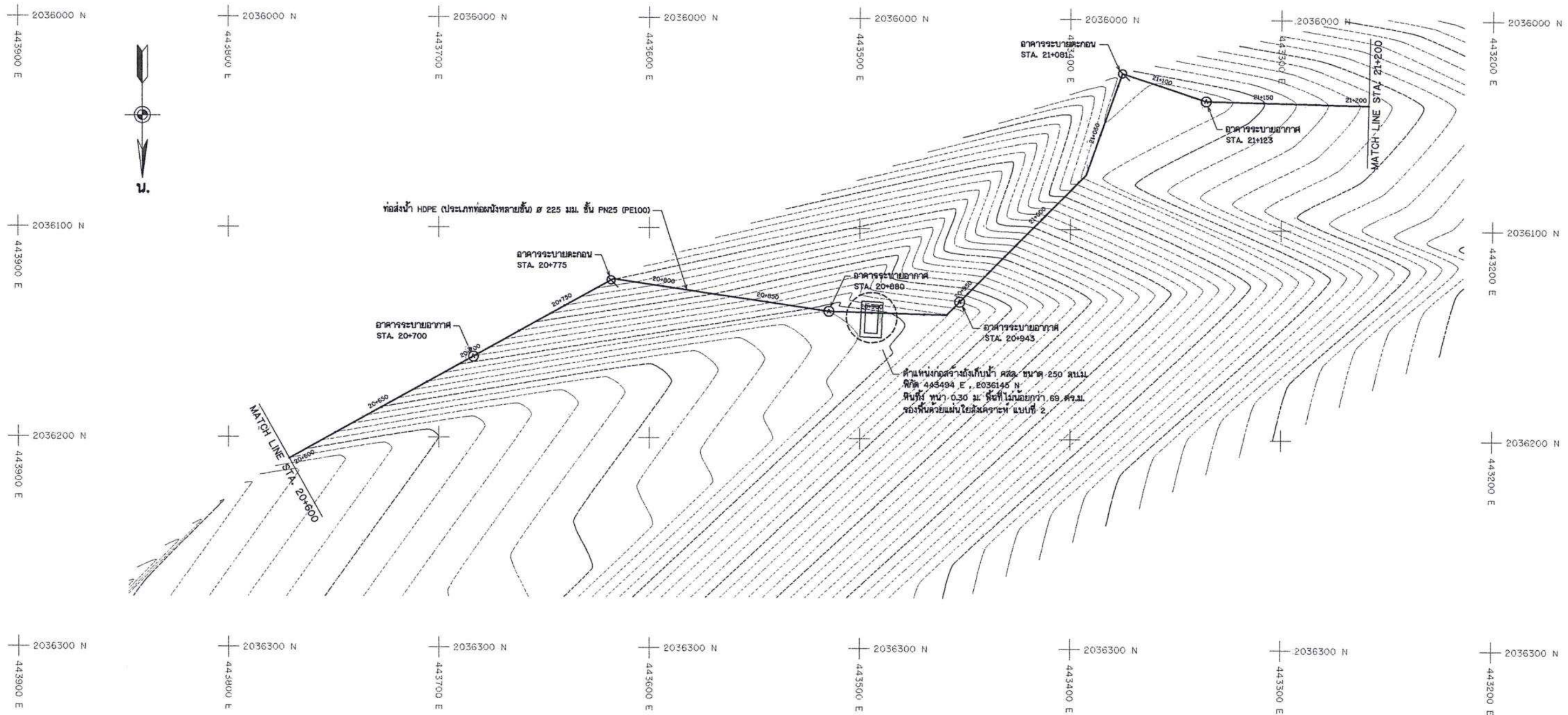
แปลนทั่วไประบบกระจายน้ำ สายที่ 1 มาตราส่วน 1:1,000
