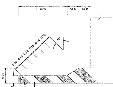
รูปแสดงการทาสี หั้ว , ท้าย ท่อเหลี่ยม คลส.
