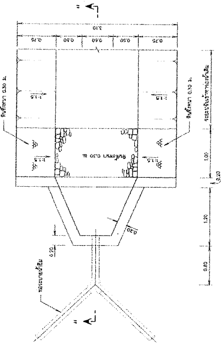
แผนอาคารระบายน้ำซึมท้ายเขื่อน
