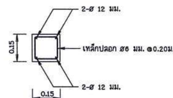
รูปตัด ก - ก k9ikij:o 1:10
