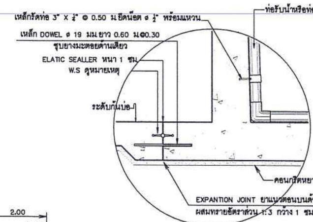
รูปขยาย "3"
