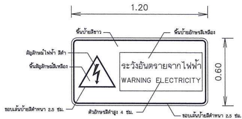
ป้ายเตือนกระแสไฟฟ้า
