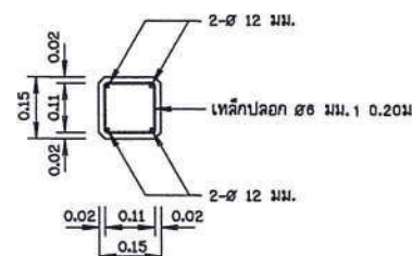
รูปตัด ข - ข k9ikij:o 1:10
