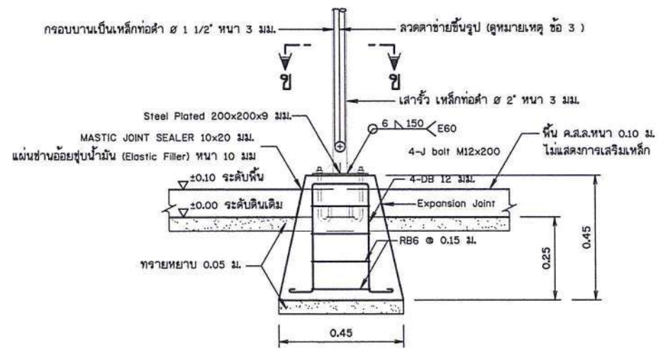
รูปขยายฐานรากโครงสร้างรับแผง F2 (ต่อมอ คสล. หล่อสำเร็จรูปพร้อมติดตั้ง) ไม่แสดงมาตราส่วน
