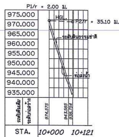
รูปตัดตามแนวยาวแสดง H.G.L. กม. 10+000
