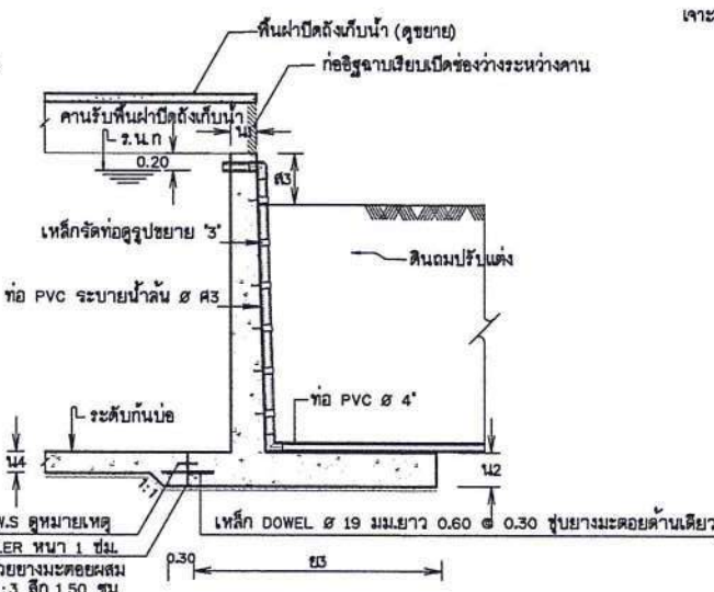
รูปตัดท่อรับน้ำหรือท่อระบายน้ำ
