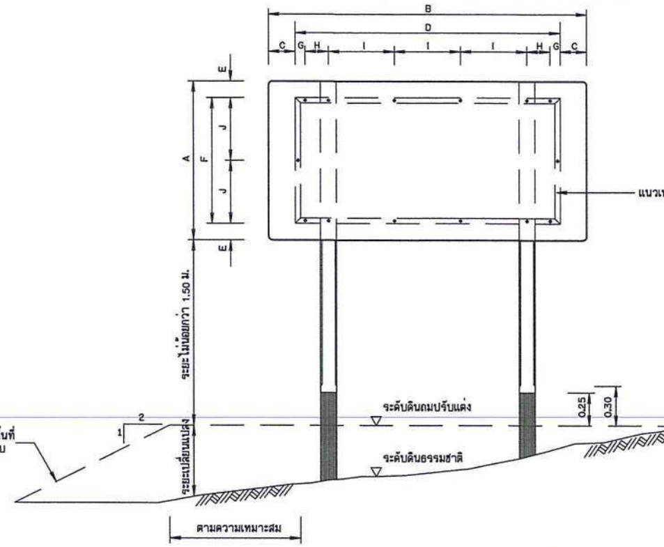
รูปแสดงการประกอบแผ่นป้าย k9ikij:o 1:20
