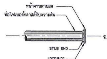
การปิดปลายท่อ
