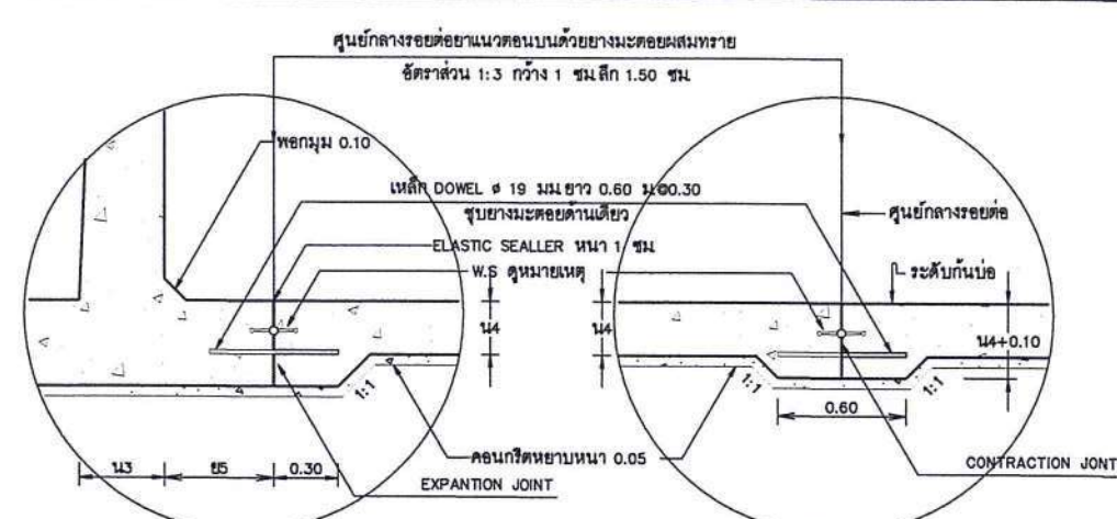
รูปขยาย "1"
