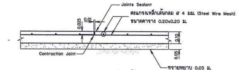
แบบขยายรอยต่อพื้น
