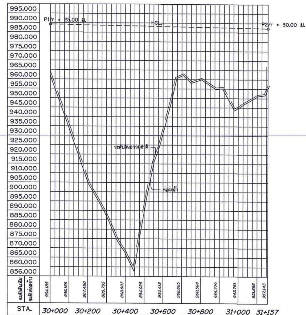
รูปตัดตามแนวยาวแสดง H.G.L. กม. 30+000
