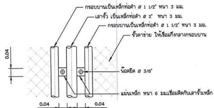
แบบขยายรายละเอียดแสดงการยึดระหว่างหัวกับเสา ไม่แสดงมาตราส่วน
