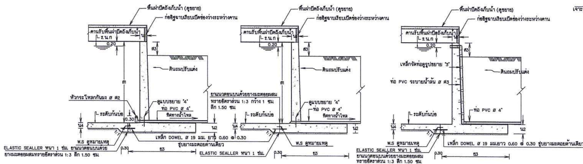
รูปตัดท่อส่งน้ำ มาตราส่วน 1:50
