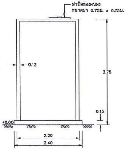
ด้านข้าง มาตราส่วน 1:40
