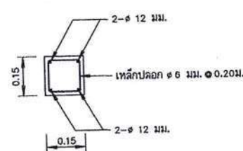
รายละเอียดส่าย คสล.
