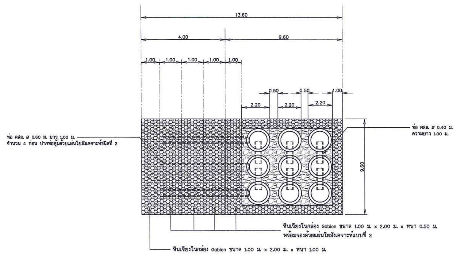
แปลนอาคารบ่อสูบน้ำ มาตราส่วน No scale
