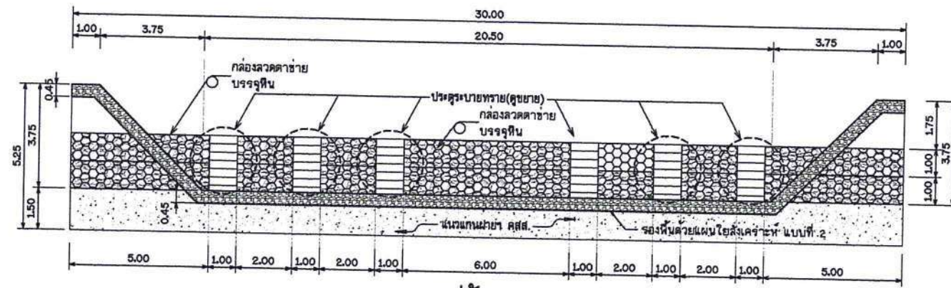
รูปตัด ข-ข
