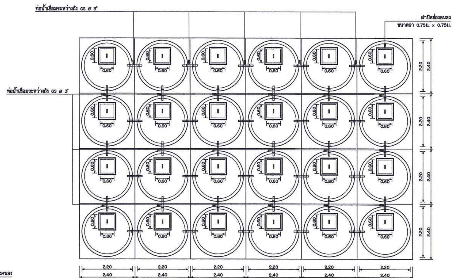
แปลนแบบ 24 ถัง ไม่แสดงมาตราส่วน
