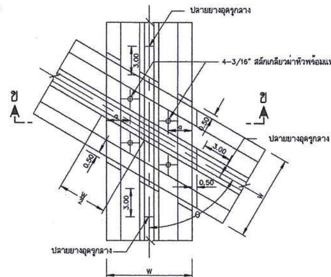
การตอขาดทับกันไม่ทำมุมฉาก ไม่แสดงมาตราส่วน
