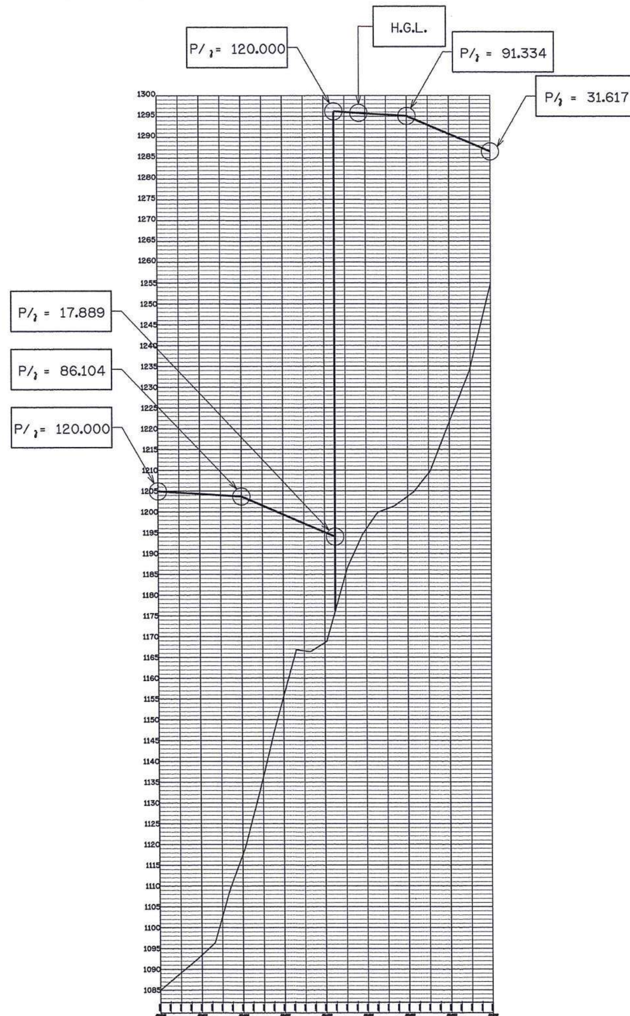
รูปตัดตามแนวยาวแสดง H.G.L. สาย 2RMP STA. 30+000 - 30+799 ไม่แสดงขนาดราดวัน
