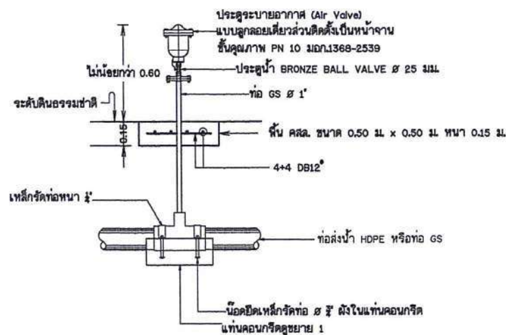
รูปตัดอาคารประตูปะบายอากาศ (Air Valve)
