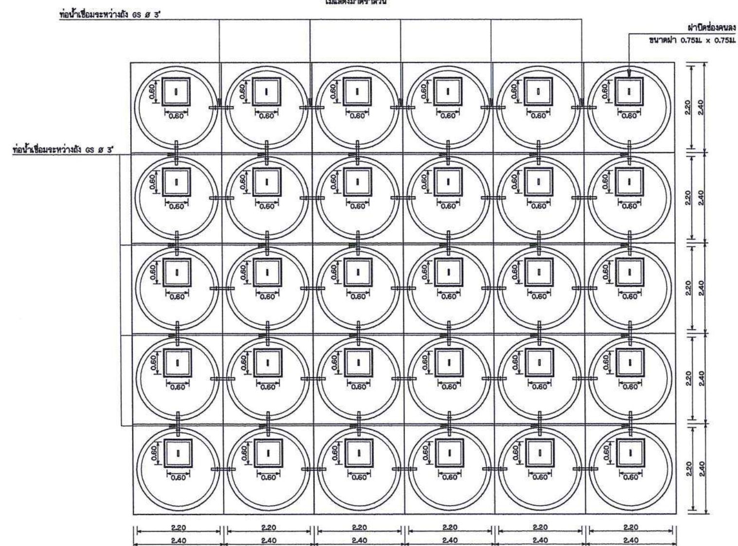
แปลนแบบ 30 ถัง ไม่แสดงมาตราส่วน
