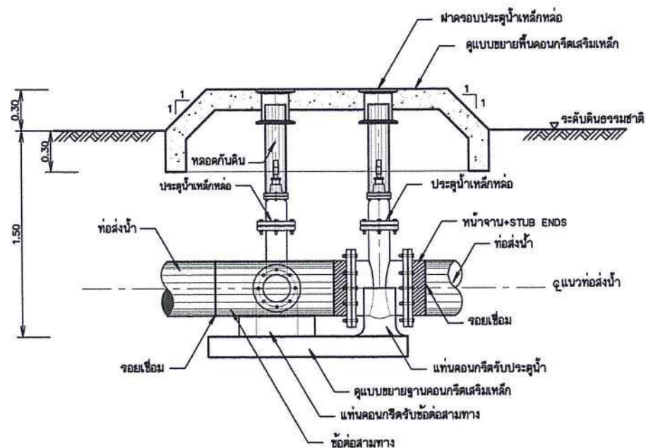
รูปตัดอาคารจตุรแฉก
