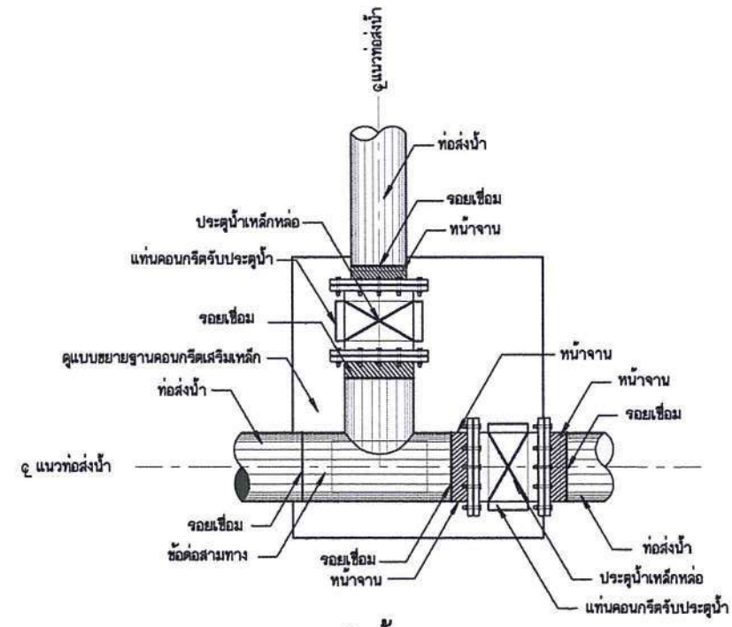
รูปขยายการติดตั้งอาคารจตุรแฉก
