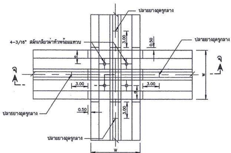
การตอขาดทับกันทำมุมฉาก ไม่แสดงมาตราส่วน
