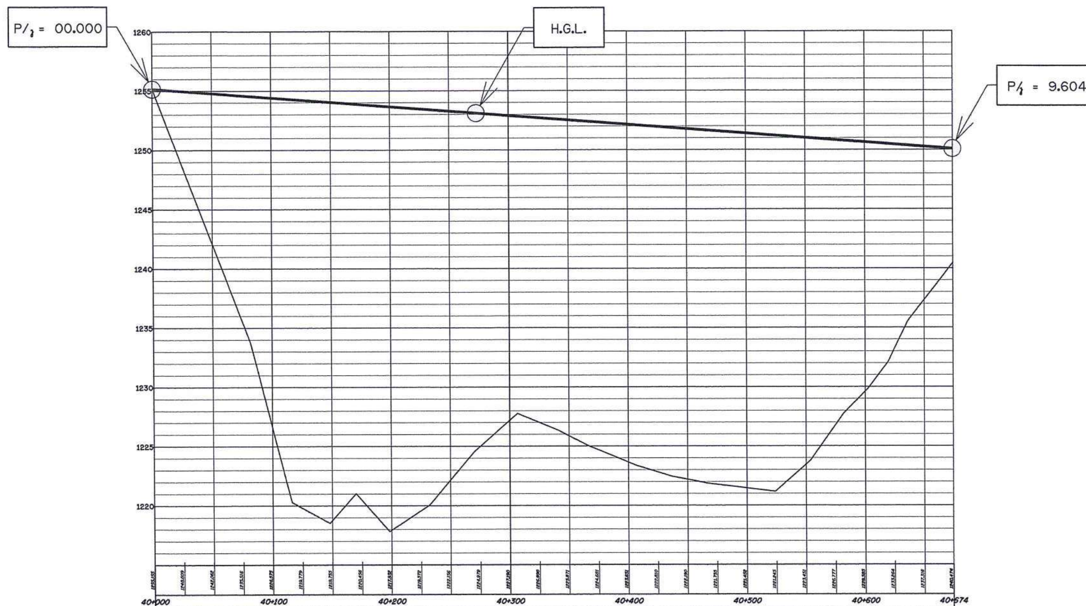
รูปตัดตามแนวยาวแสดง H.G.L. สาย 3RMP STA. 40+000 - 40+674 ไม่แสดงขนาดลำน้ำ
