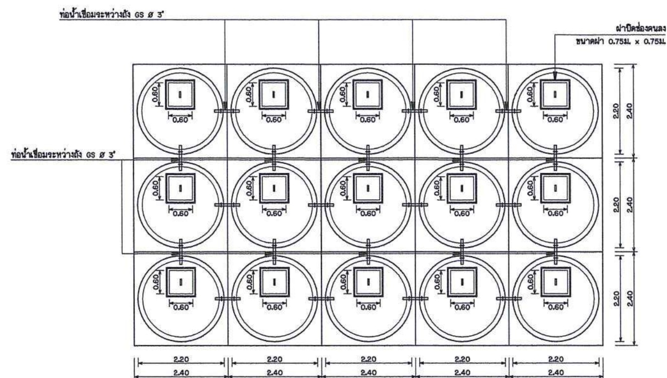
แปลนแบบ 15 ถัง ไม่แสดงมาตราส่วน
