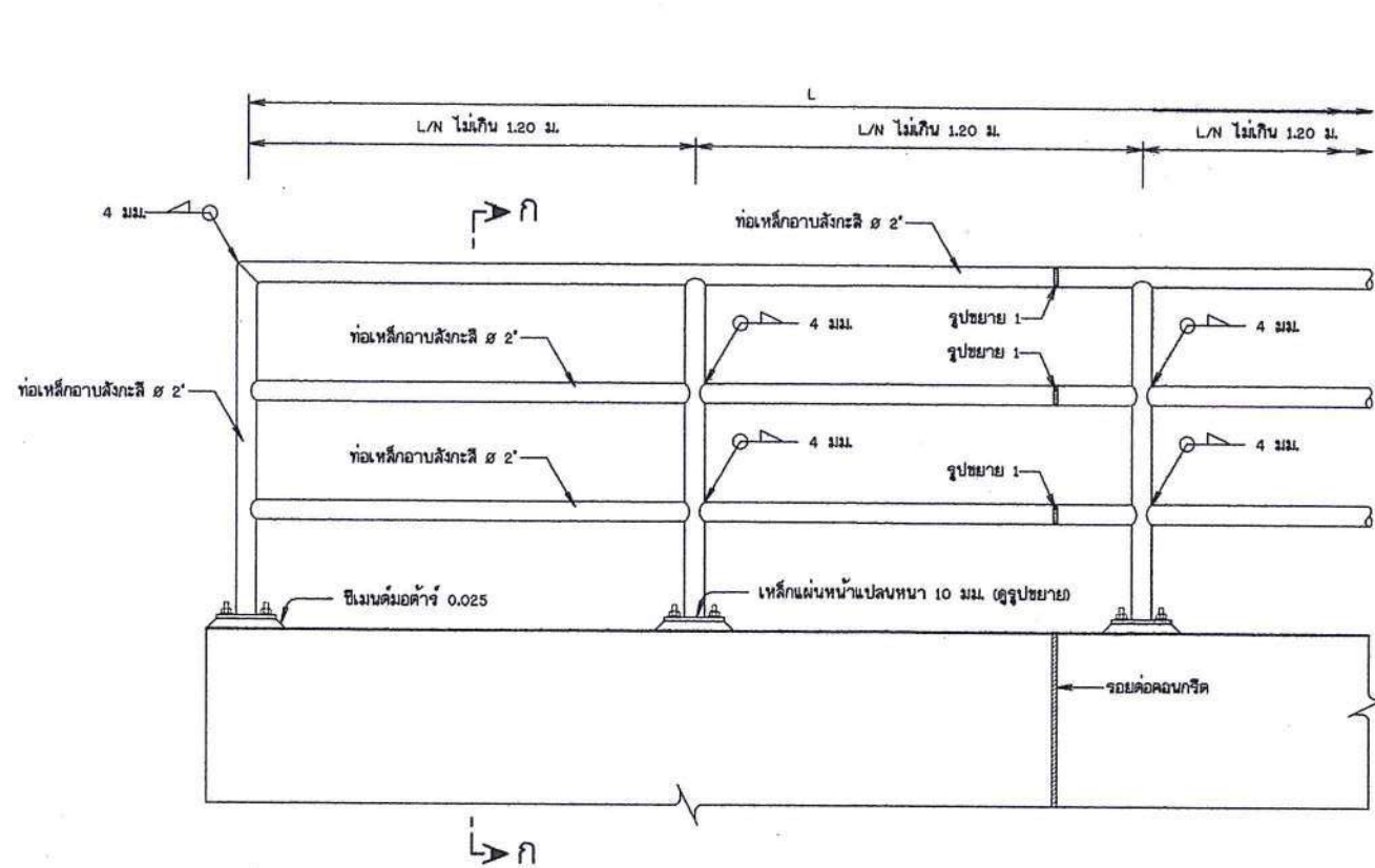
รูปขยายจาวเหล็กกันดก มาตราส่วน 1:10
