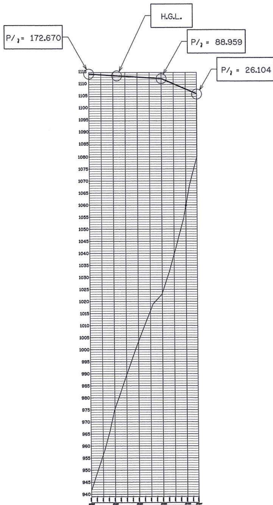
รูปตัดตามแนวยาวแสดง H.G.L. สาย 1RMP STA. 20+000 - 20+447 ไม่แสดงขนาดราดวัน
