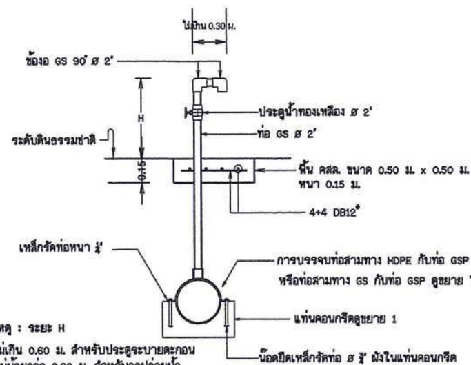
รูปตัดอาคารประตูปะบายตะกอนและอาคารจุดปล่อยน้ำ
