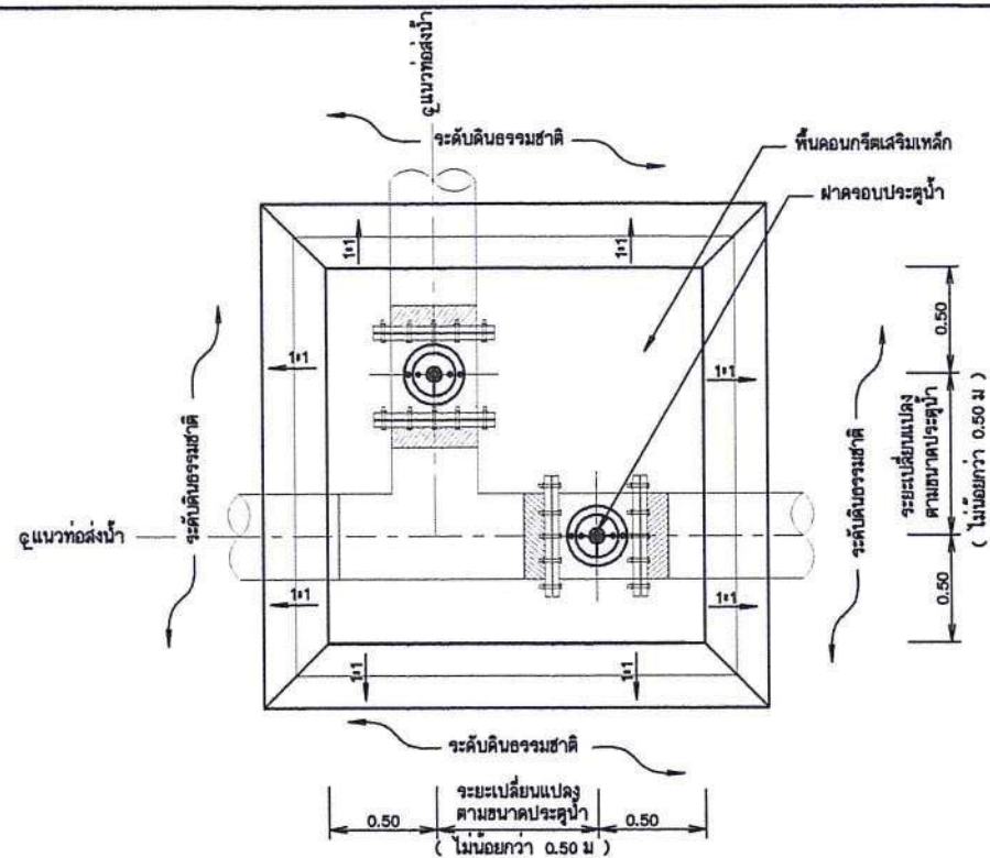
แปลนอาคารจตุรแฉก
