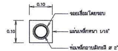
ขยายท่อผ่านผนัง
