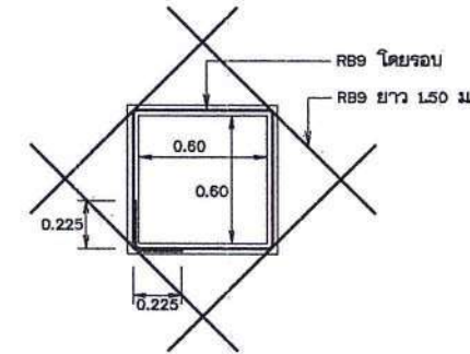
ขยายการเสริมเหล็กช่องคนลง
