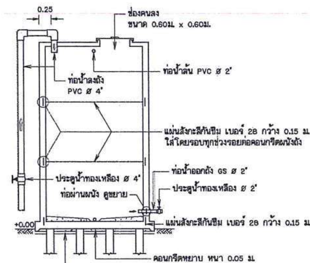
รูปตัด (1)
