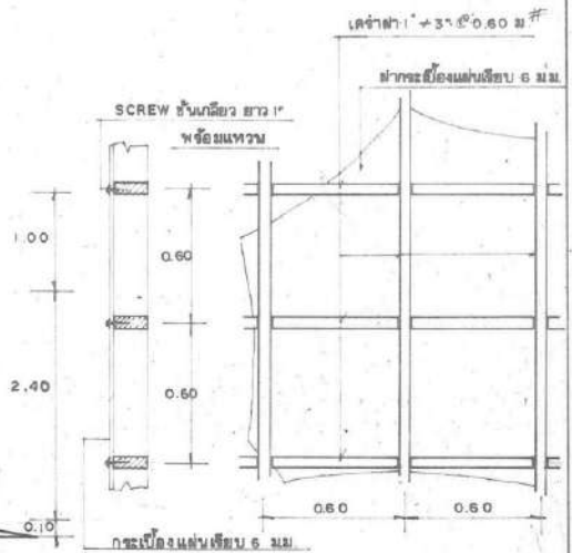
รูปขยายเคาะ, ฝา 1820
