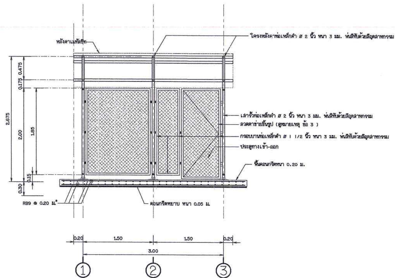
รูปตัด ก - ก ไม่แสดงขนาดจั่ว
