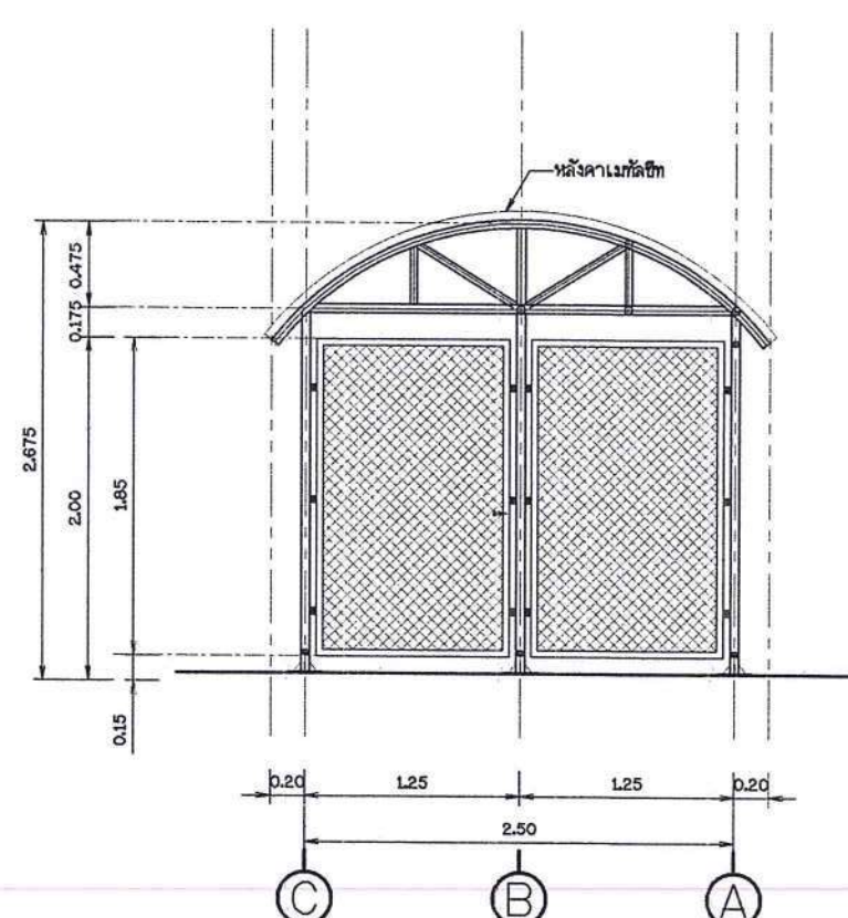
รูปด้าน 2 โมเดลคงภาคกลาง
