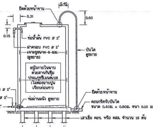
รูปตัด (2)
