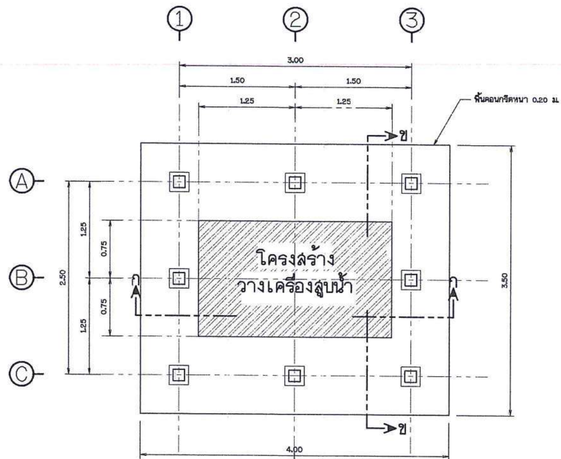
แบบแปลน ไม่แสดงขนาดรา้ว
