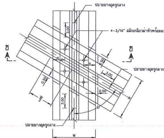
การต่อทำมุมกันไม่ทำมุมฉาก ไม่แสดงมาตราส่วน
