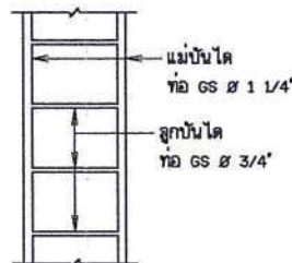
ขยายบันได
