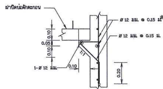
รูปตัด ค - ค
