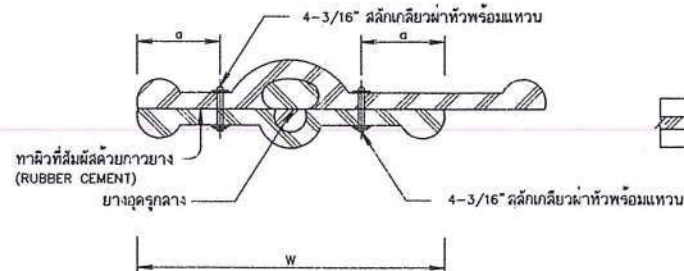
รูปตัด ข-ข ไม่แสดงมาตราส่วน
