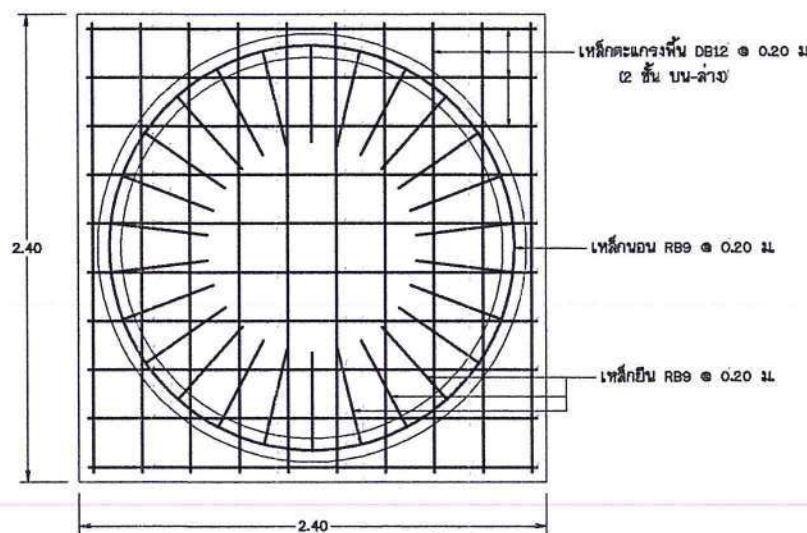
แสดงการเสริมเหล็กพื้นถึง
