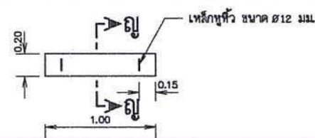
แปลนฝาบ่อตกตะกอน
