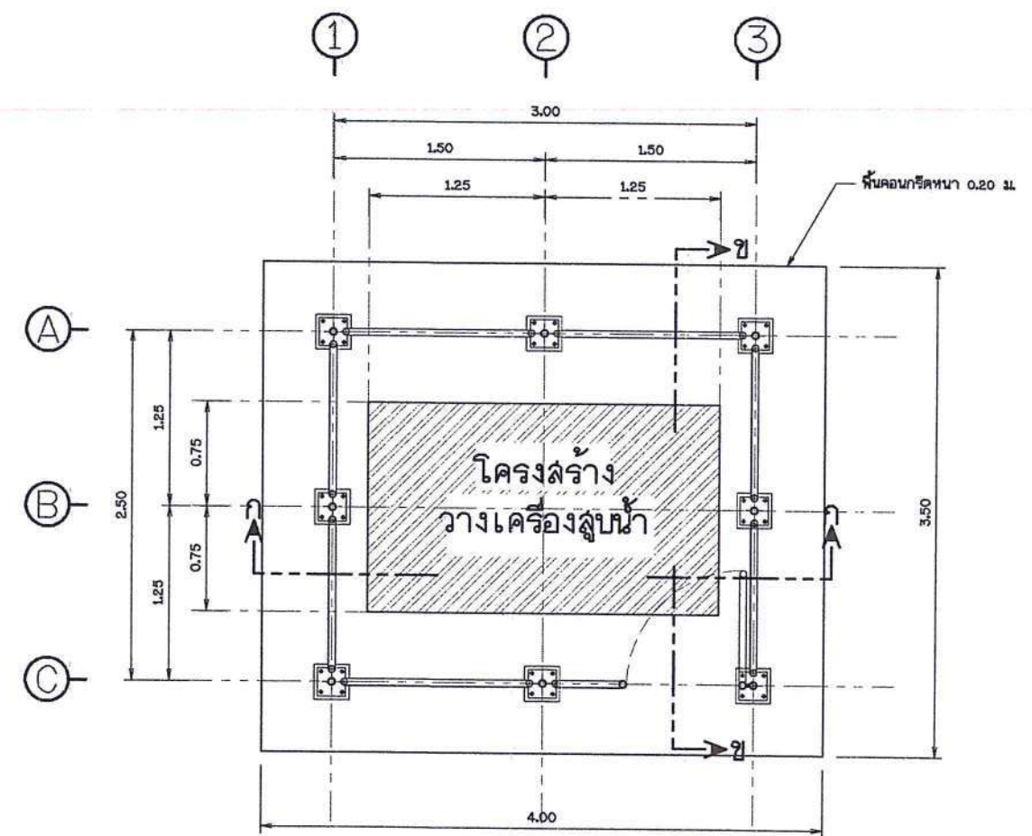
แปลนเสาและรั้ว ไม่แสดงขนาดรา้ว
