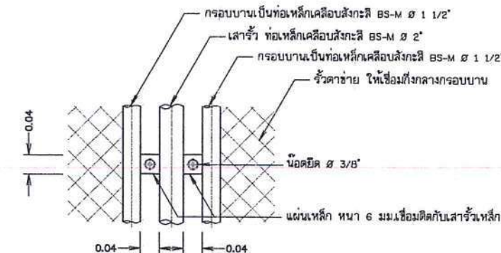
แบบขยายรายละเอียดแสดงการยึดระหว่างรั้วกับเสา
