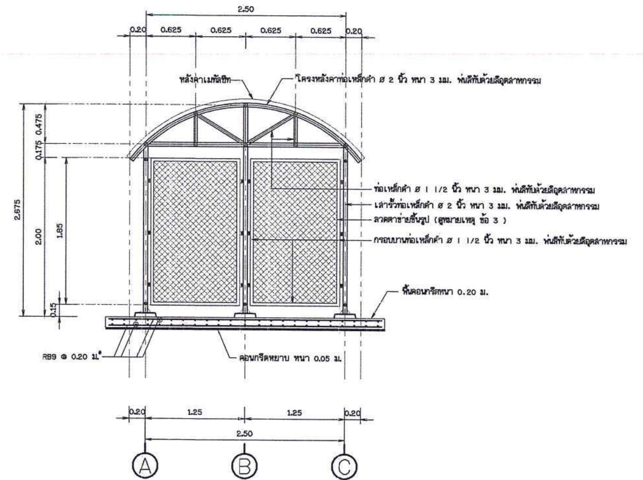
รูปตัด ข - ข ไม่แสดงขนาดจั่ว
