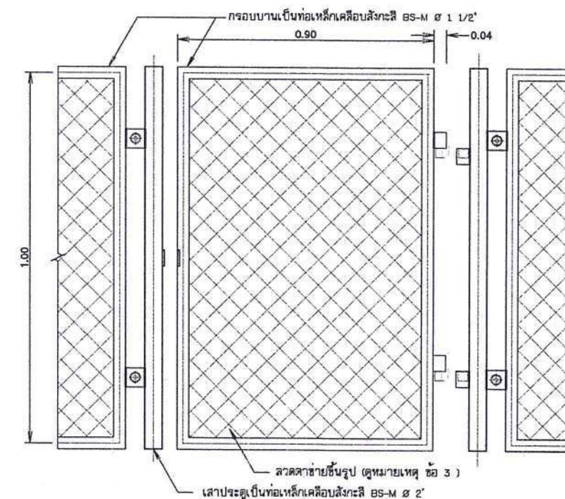
แบบขยายรายละเอียดประตู
