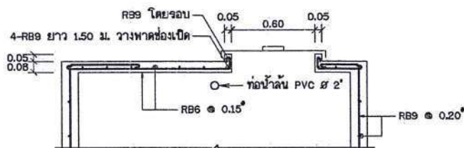
แสดงการเสริมเหล็กฟาดถึง
