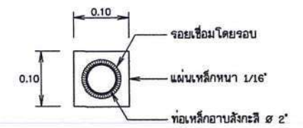
ขยายท่อผ่านผนัง
