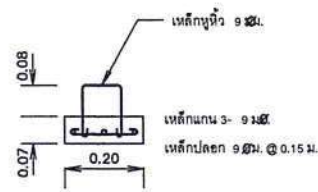
รูปตัด ฅ - ฅ
