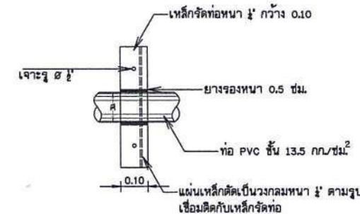
รูปขยาย "4" มาตราส่วน 1:10
