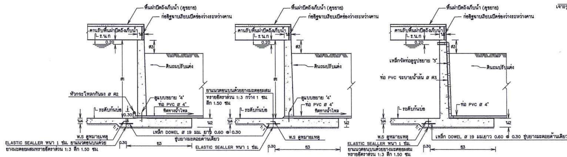
รูปตัดท่อส่งน้ำ มาตราส่วน 1:50
