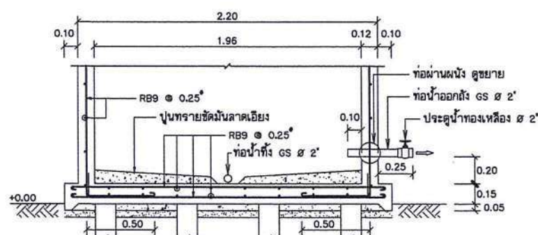
แสดงการเสริมเหล็กพื้นถัง
