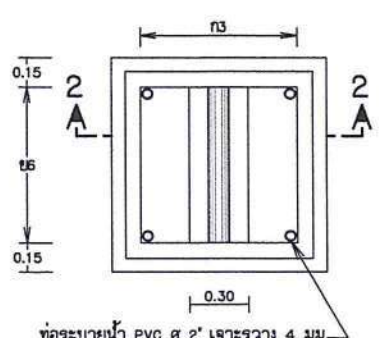
แปลนบ่อประจุบึงค้ำน้ำ มาตราส่วน 1:20
