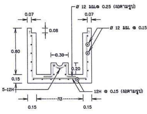
เหล็กเสริมบ่อประจุน้ำ มาตราส่วน 1:20
