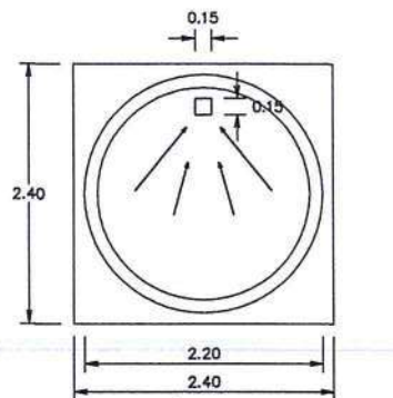
แสดงมิติบ่อรวมตะกอน
