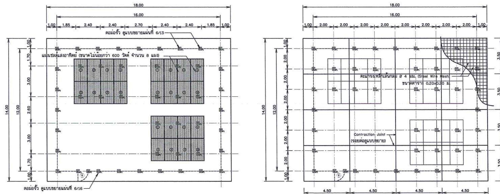
แปลนการติดตั้งแผงเซลล์แสงอาทิตย์ พร้อมรั้ว
