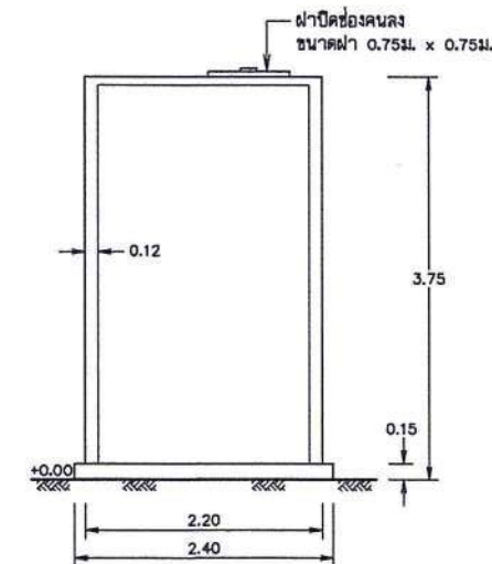
ด้านข้าง
