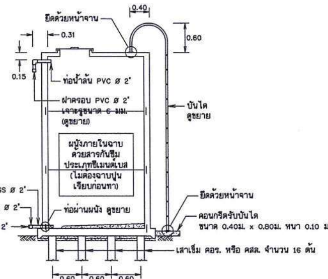
รูปตัด (2)
