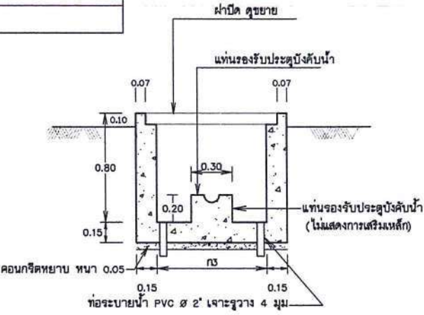
รูปตัด 2 - 2 มาตราส่วน 1:20
