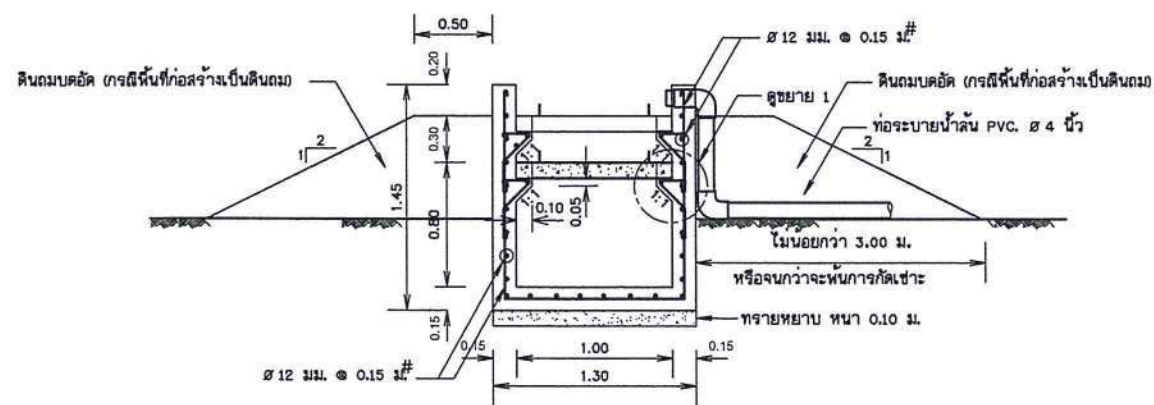
รูปตัด ฅ - ฅ
