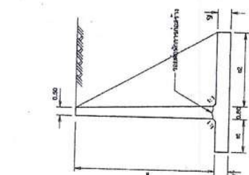
รูปตัด ก-ก โมเดลมาตรฐาน
