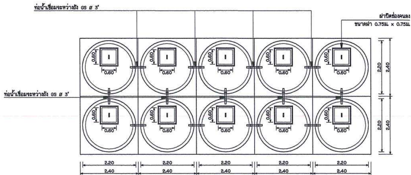
แปลนแบบ 10 ถัง
