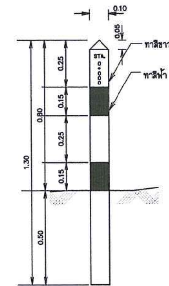
แสดงสัดส่วนหลักบ่อแนวท่อ
