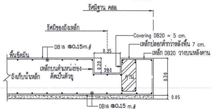
แบบขยายฐานรับถังเก็บน้ำ คสล. SCALE A3 1:50
