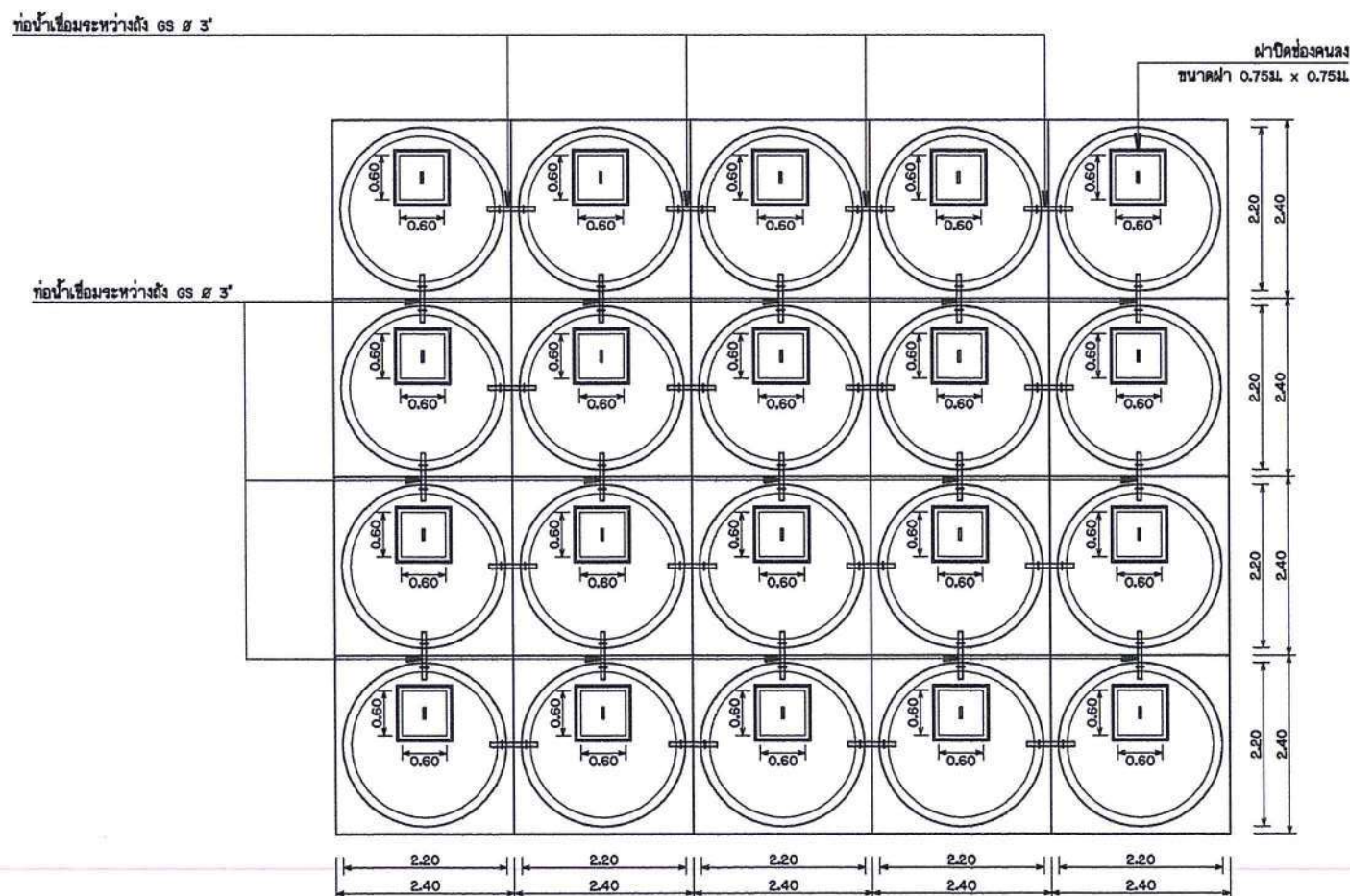
แปลนแบบ 20 ถัง
