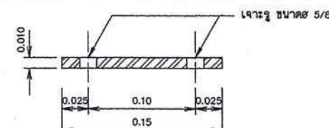
รูปตัด ค-ค
