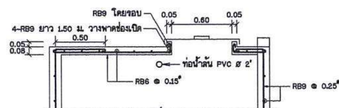
แสดงการเสริมเหล็กฟุตบาท มาตราส่วน 1:20
