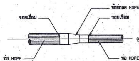
การบรรจุบ่อ HDPE กับข้อคดท่อ HDPE
