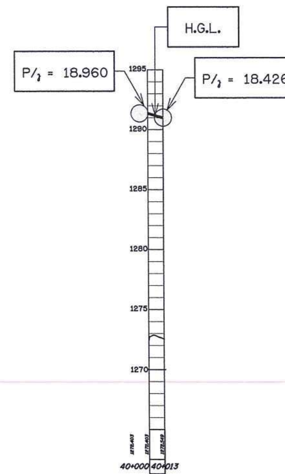
รูปตัดตามแนวยาวแสดง H.G.L. สาย 1R-1L-3RMP STA. 40+000 - 40+013 ไม่แสดงขนาดราวล้วน
