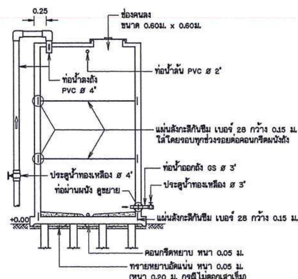
รูปตัด (1) มาตราส่วน 1:40
