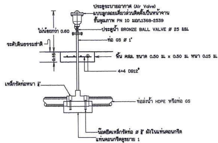
รูปตัดอาคารประตูลูกบอลอากาศ (Air Valve)
