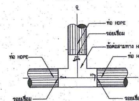
การบรรจุบ่อสามทาง HDPE กับท่อ HDPE
