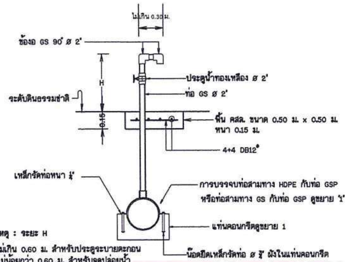
รูปตัดอาคารประตูลูกบอลตะกอนและอาคารจุดปล่อยน้ำ
