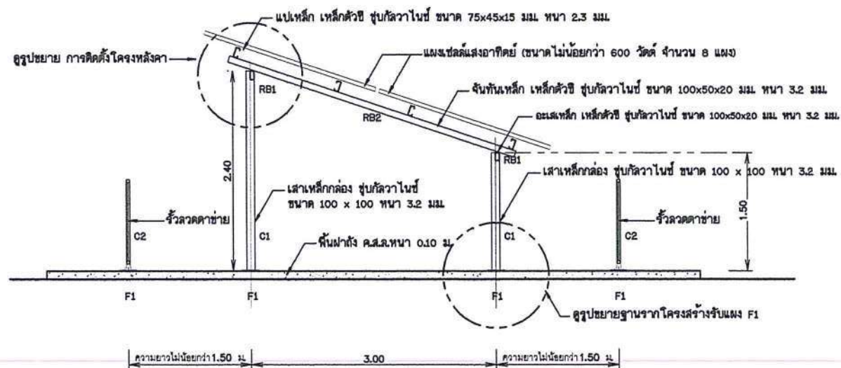
รูปด้านข้าง ไม่แสดงขนาดจาล้วน
