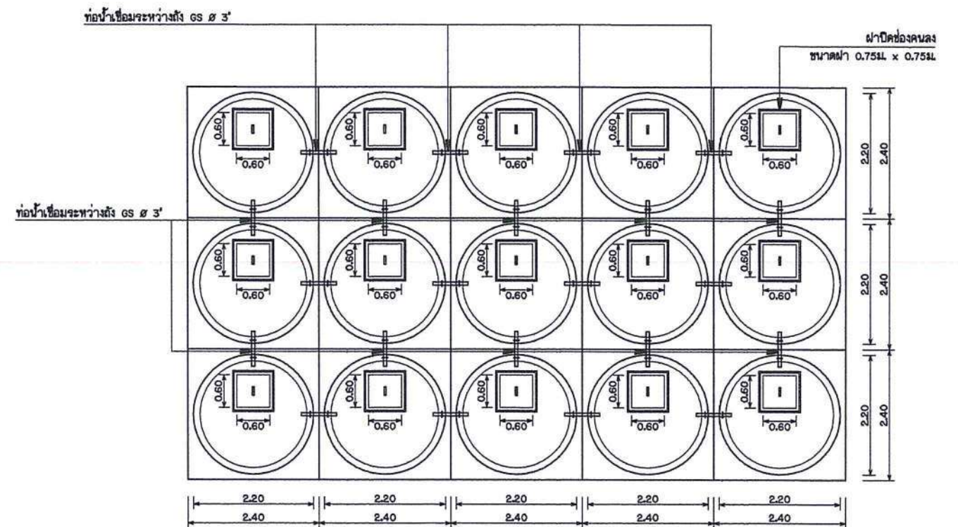
แปลนแบบ 15 ถัง
