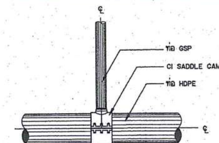
การบรรจุบ่อสามทาง HDPE กับท่อ GSP แบบ CI SADDLE CLAMP
