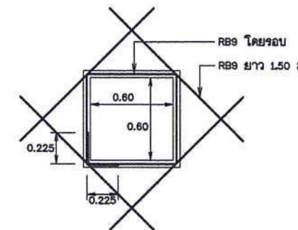
ขยายการเสริมเหล็กฟุตบาทคอนกรีต มาตราส่วน 1:20
