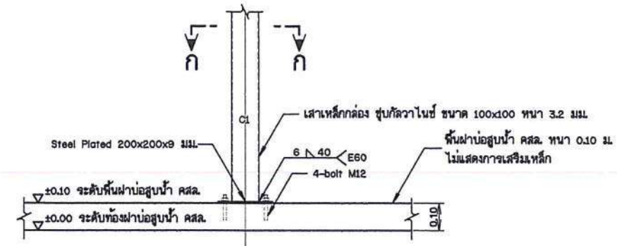
รูปขยายฐานรากโครงสร้างรับแผง F1 (ต่อม่อ คสล. หล่อสำเร็จรูปพร้อมติดตั้ง) ไม่แสดงขนาดจาล้วน
