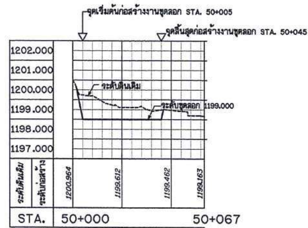
รูปตัดตามแนวยาว งานขุดลอก ไม่แสดงมาตราส่วน
