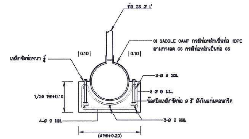
รูปตัดขยาย 1"
