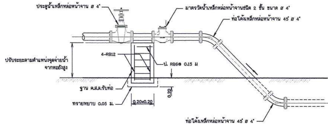
การติดตั้งมาตรวัดน้ำบนพื้นดิน ๕ ๔" ไม่แสดงมาตราส่วน
