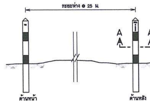
แสดงการวางหลักบ่อแนวท่อ
