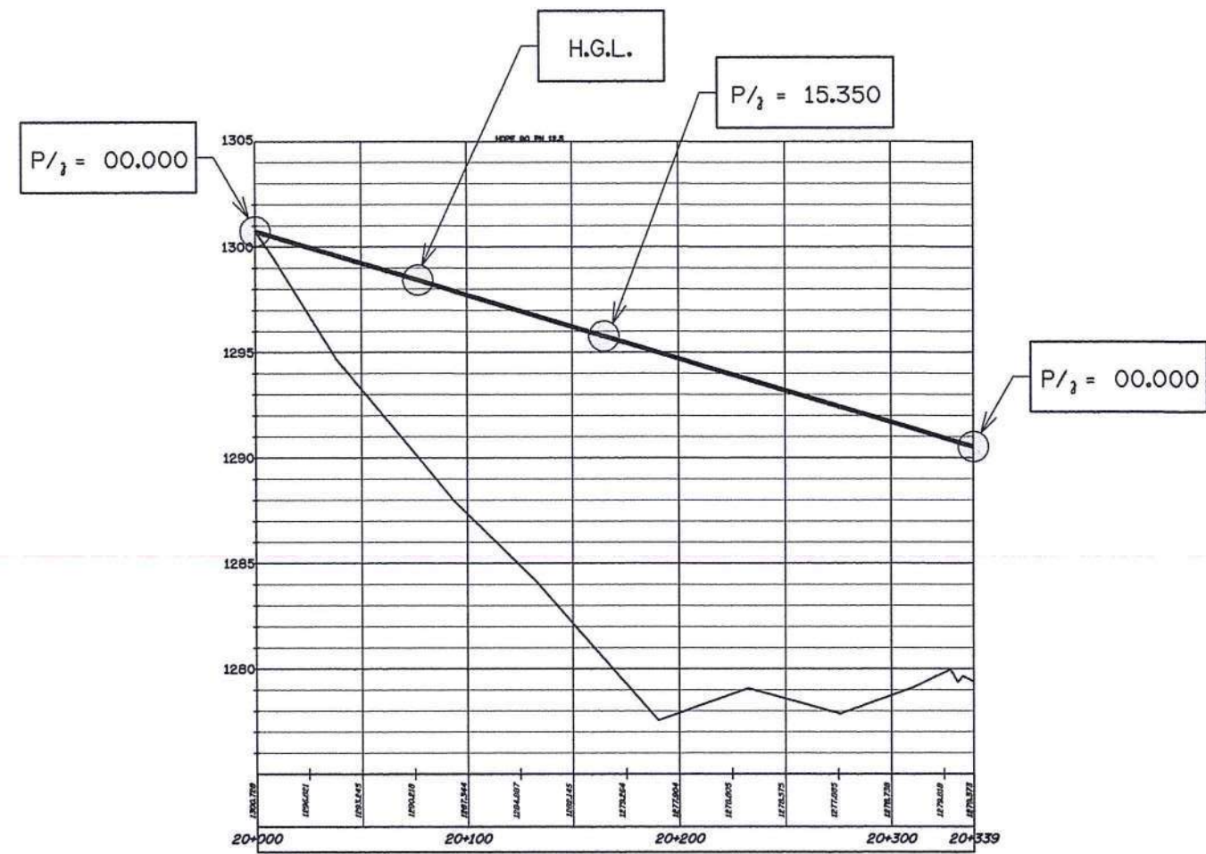
รูปตัดตามแนวยาวแสดง H.G.L. สาย 3RMP STA. 20+000 - 20+339 ไม่แสดงขนาดราวล้วน
