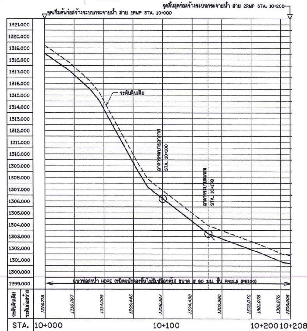
รูปตัดตามแนวยาว สาย 2RMP STA. 10+000 - 10+208
