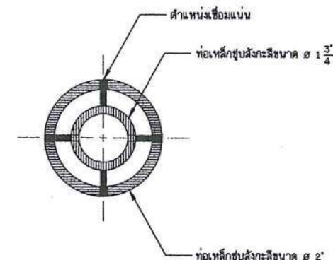
รูปตัด ข-ข
