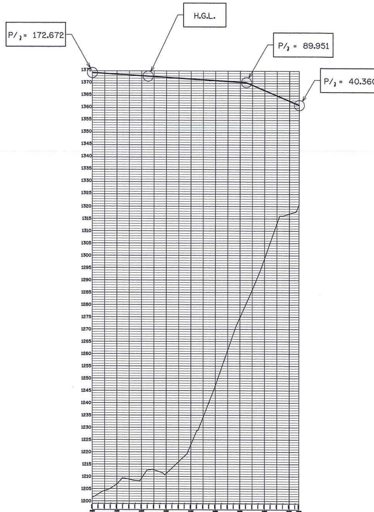
รูปตัดตามแนวยาวแสดง H.G.L. สาย 1RMP STA. 0+000 - 0+840 โมเดลตามค่าจริง
