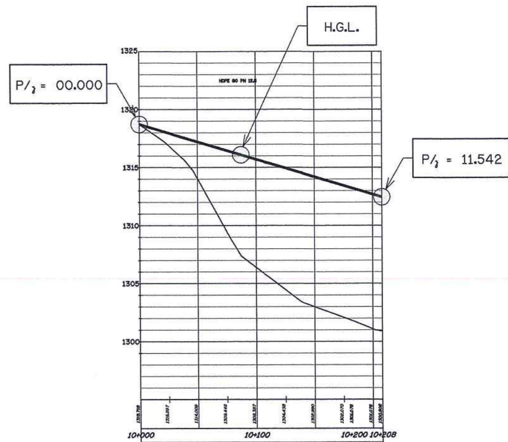
รูปตัดตามแนวยาวแสดง H.G.L. สาย 2RMP STA. 10+000 - 10+208 ไม่แสดงขนาดราวล้วน
