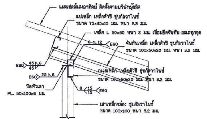
รูปขยาย การติดตั้งโครงหลังคา ไม่แสดงขนาดจาล้วน
