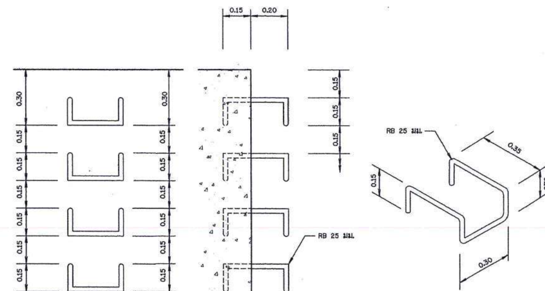
รูปขยายบันไดลิง
