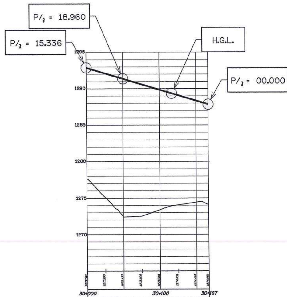
รูปตัดตามแนวยาวแสดง H.G.L. สาย 1L-3RMP STA. 30+000 - 30+167 ไม่แสดงขนาดราวล้วน
