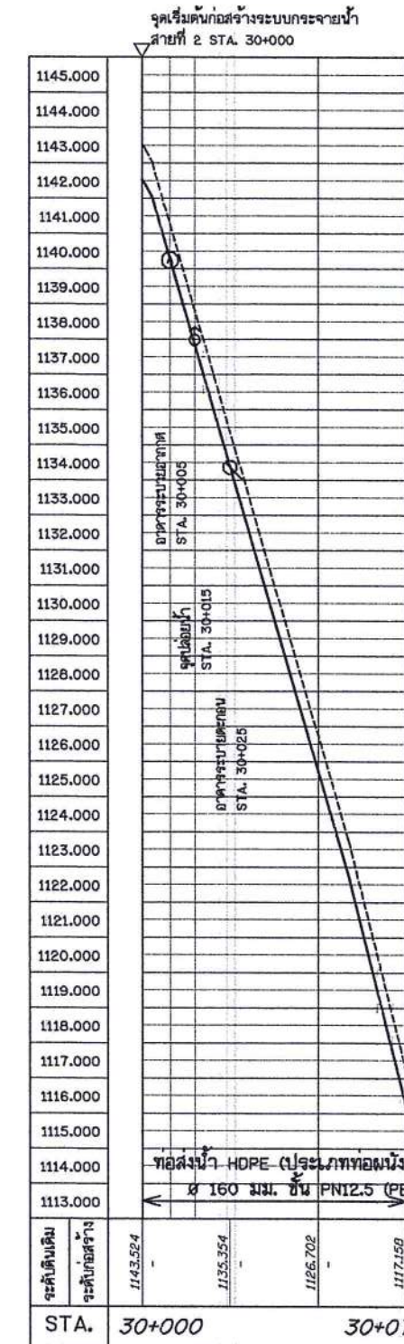
รูปตัดตามแนวยาวระบบกระจายน้ำ สายที่ 2
