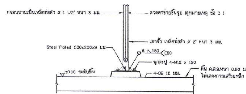
แบบขยายรายละเอียดแสดงการยึด ไม่แสดงมาตราส่วน
