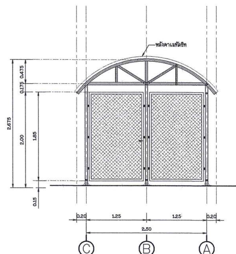
รูปด้าน 2 ไม่แสดงขนาดจาล้วน
