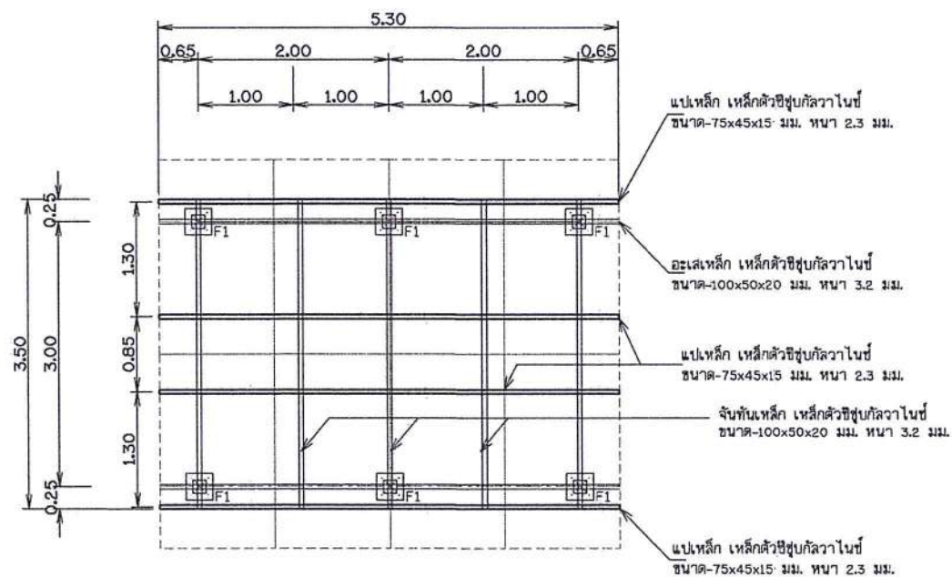
แปลนฐานรากและโครงหลังคารับแผง จำนวน 8 แผง
