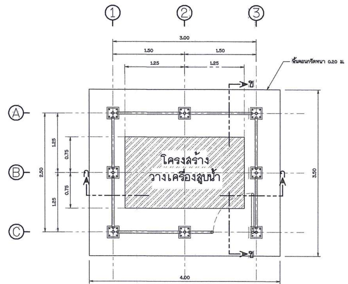
แปลนเสาและรั้ว ไม่แสดงขนาดราวล้วน
