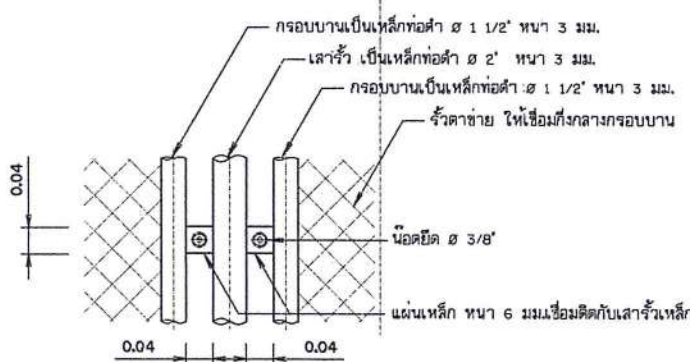
แบบขยายรายละเอียดแสดงการยึดระหว่างรั้วกับเล้า ไม่แสดงมาตราส่วน
