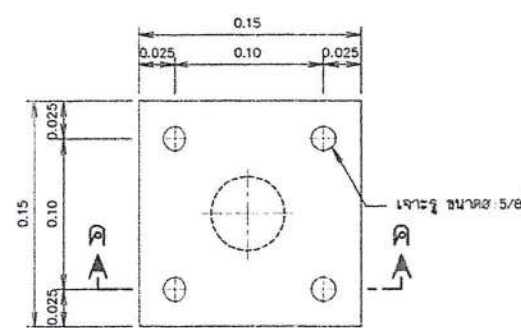
รูปขยายแผ่นเหล็กหน้าแปลน
