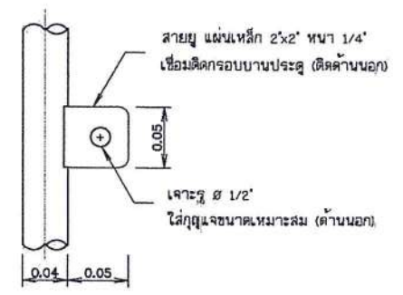
แบบขยายสายยู ไม่แสดงขนาดจริง
