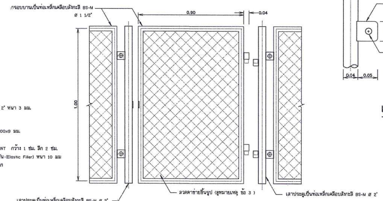
แบบขยายรายละเอียดประตู ไม่แสดงขนาดจริง
