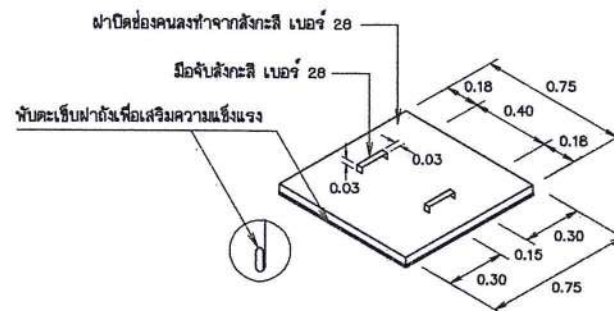
ขยายฟาดช่องคนลง มาตราส่วน not to scale
