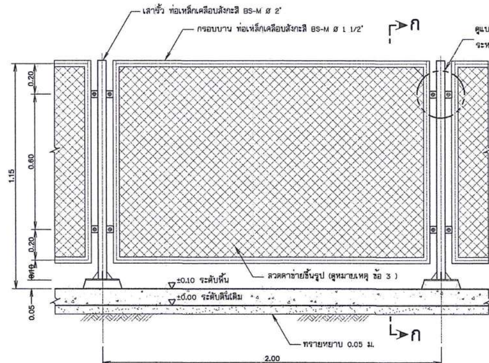
แบบขยายรายละเอียดแสดงการยึดระหว่างรั้วกับเสา ไม่แสดงขนาดจริง
