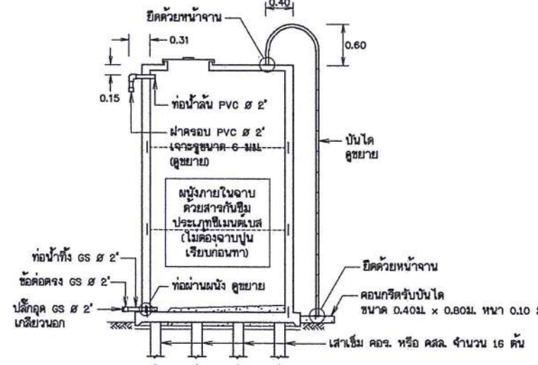
รูปตัด (2) มาตราส่วน 1:40
