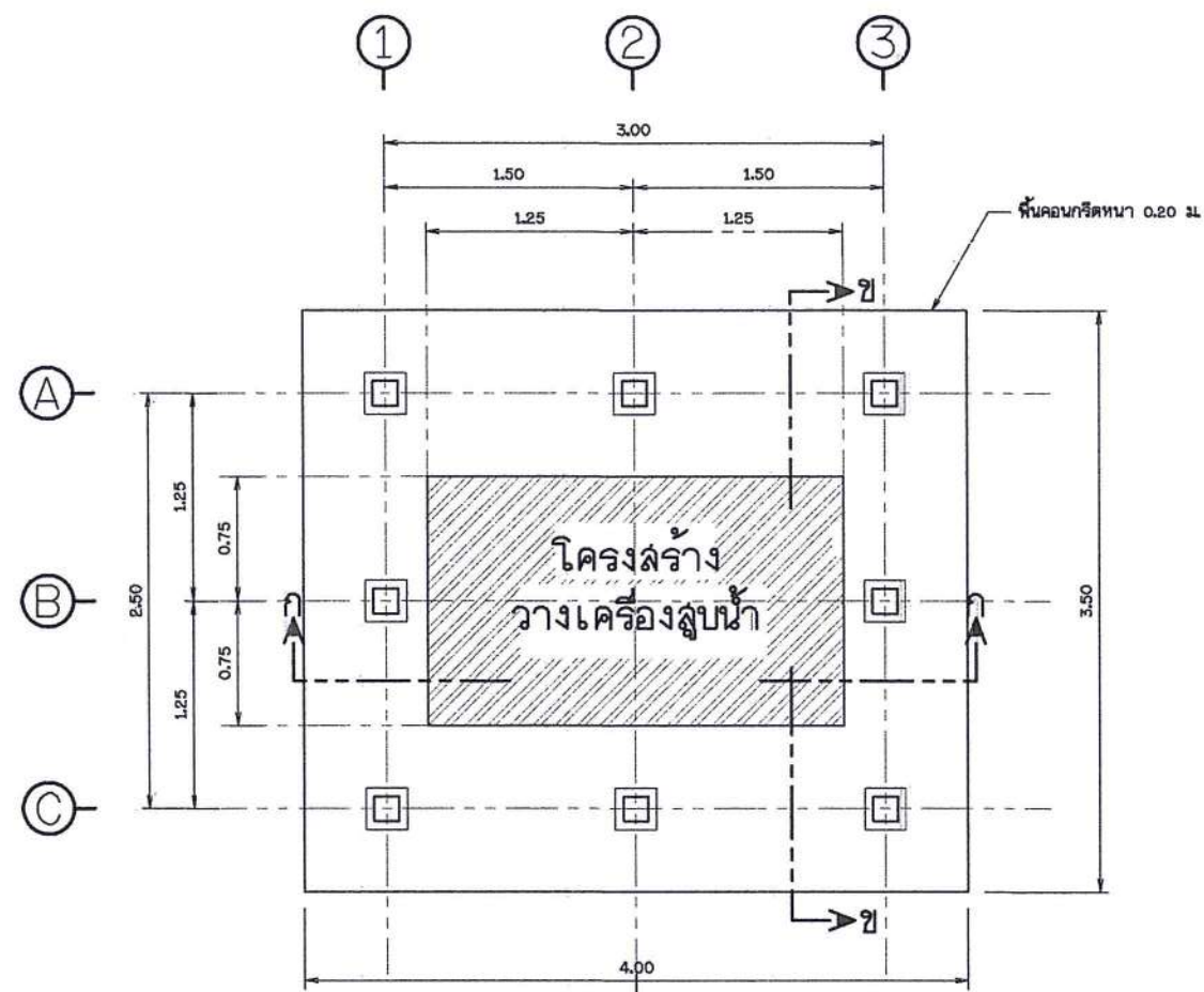
แบบแปลน ไม่แสดงขนาดราวล้วน
