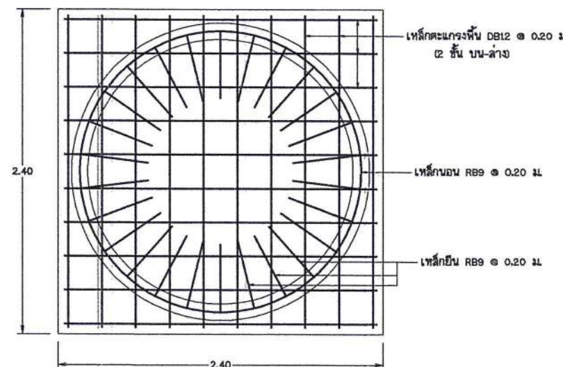
แสดงการเสริมเหล็กพื้นถึง มาตราส่วน 1:20
