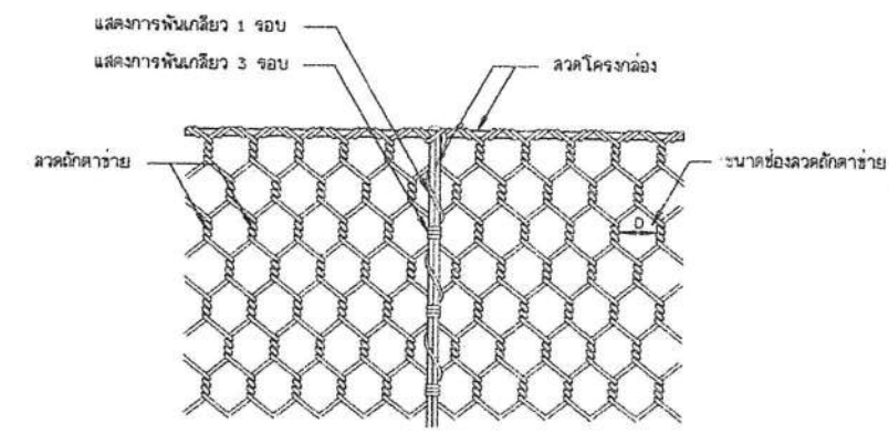
รูปแสดงการผันลดระหว่างกล่องลดตาซ้ายและฝาปิด
