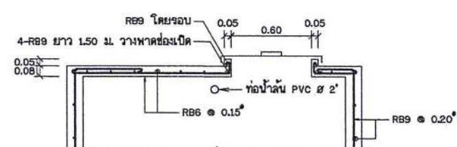
แสดงการเสริมเหล็กฟาดถึง มาตราส่วน 1:20
