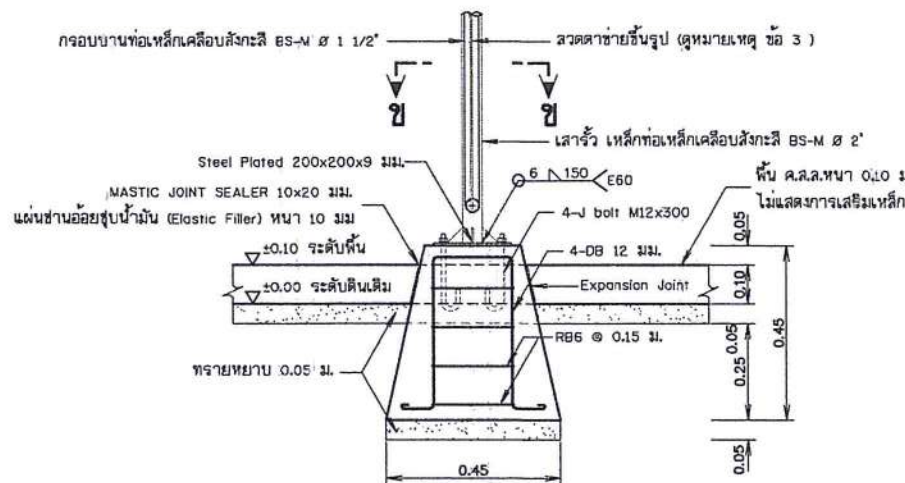
รูปขยายฐานรากโครงสร้างรับแผง F1 (ต่อม่อ คสล. หล่อสำเร็จรูปพร้อมติดตั้ง) ไม่แสดงขนาดจริง
