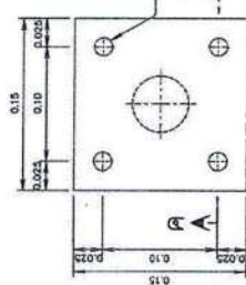
รูปขยายแผนเหล็กหน้าแปลน
