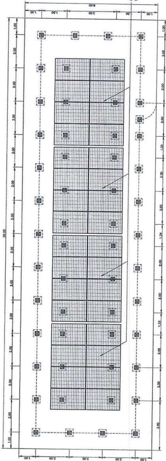
แปลนการติดตั้งแผงเซลล์แสงอาทิตย์ พร้อมรั้ว
