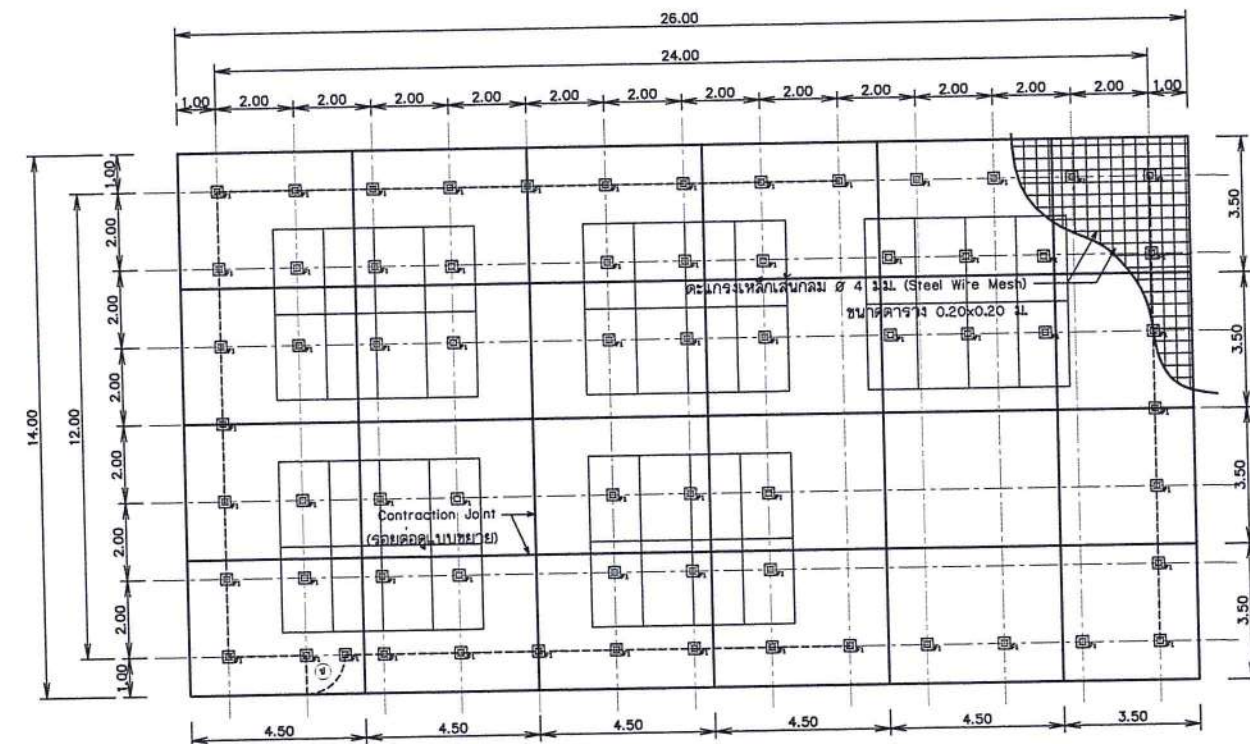
แปลนการติดตั้งแผงเซลล์แสงอาทิตย์ พร้อมรั้ว
