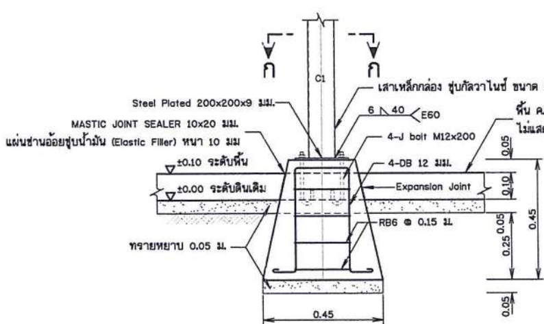
รูปขยายฐานรากโครงสร้างรับแผง F1 (ต่อม่อ คสล. ท่อผ่านรูรูปทรงสี่เหลี่ยม) ไม่แสดงมาตราส่วน
