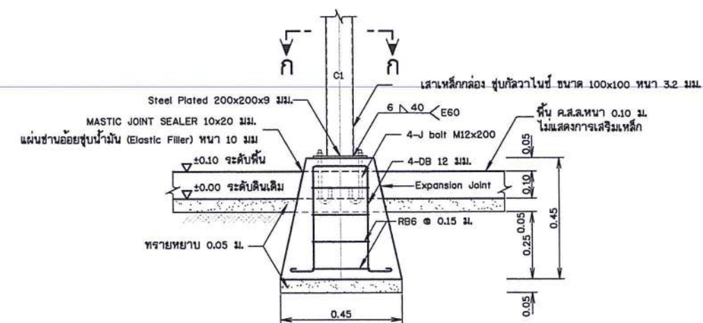
รูปขยายฐานรากโครงสร้างรับแผง F1 (ต่อม่อ คสล. ทล่อสำร็จรูปพร้อมติดตั้ง) ไม่แสดงมาตราส่วน
