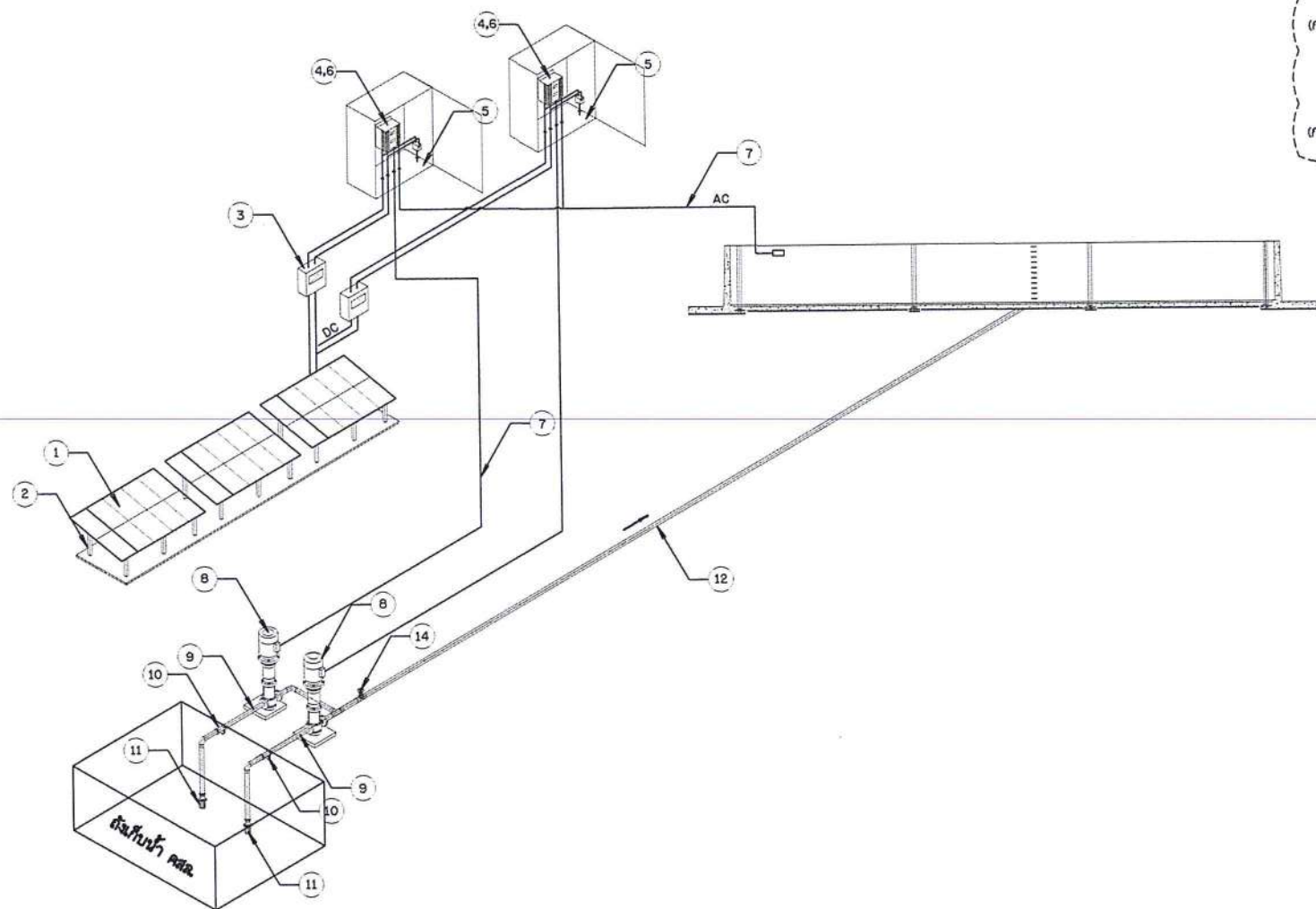
แผนผังระบบไฟฟ้า และไดอะแกรมไฟฟ้า ระบบกระจายน้ำด้วยพลังงานแสงอาทิตย์ ขนาด 15 กิโลวัตต์
