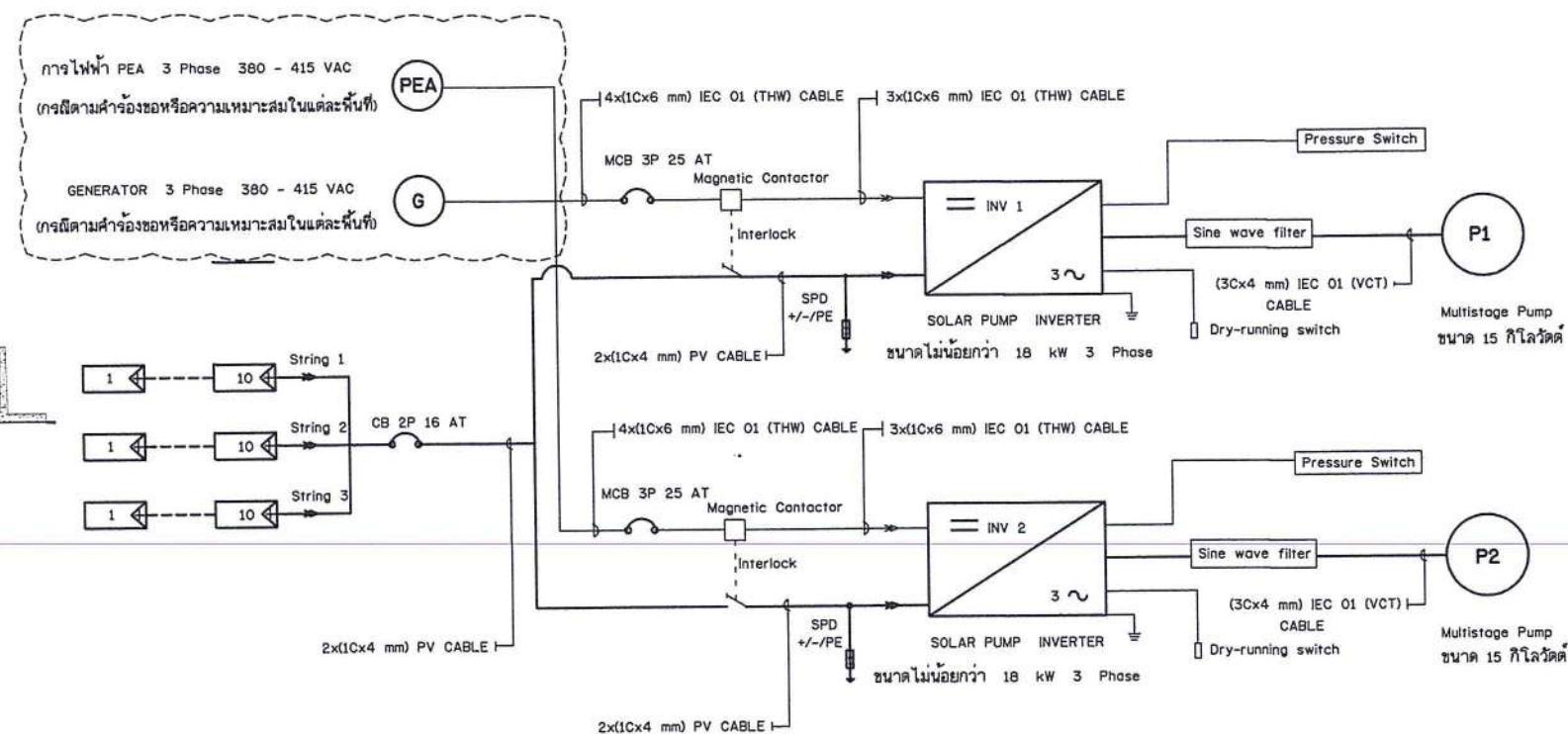
แผนผังระบบไฟฟ้า และไดอะแกรมไฟฟ้า ระบบกระจายน้ำด้วยพลังงานแสงอาทิตย์ ขนาด 15 กิโลวัตต์
