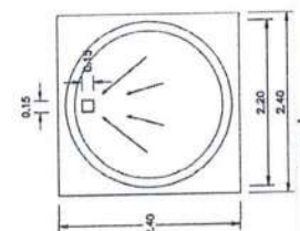
แสดงมิติโดยรวมตะกอน มาตราส่วน 1:40
