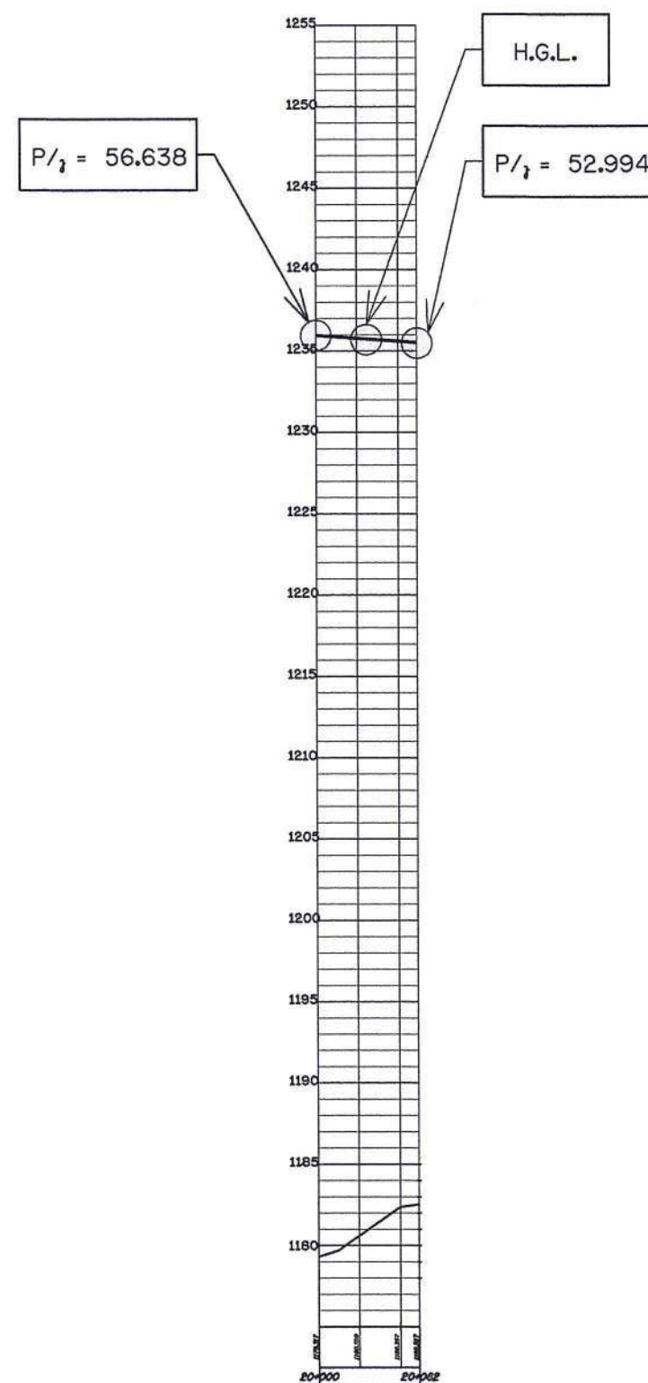
รูปตัดตามแนวยาวแสดง H.G.L. สาย 1L-2LMP STA. 20+000 - 20+062 โมเลกุลขนาดตัว
