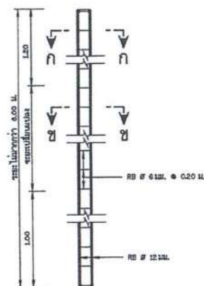
รายละเอียดส่้าบาย คสล.
