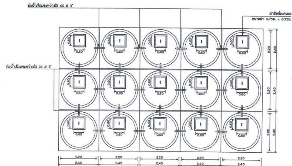
แปลนแบบ 15 ถัง ไม่แสดงขนาดราส่วน
