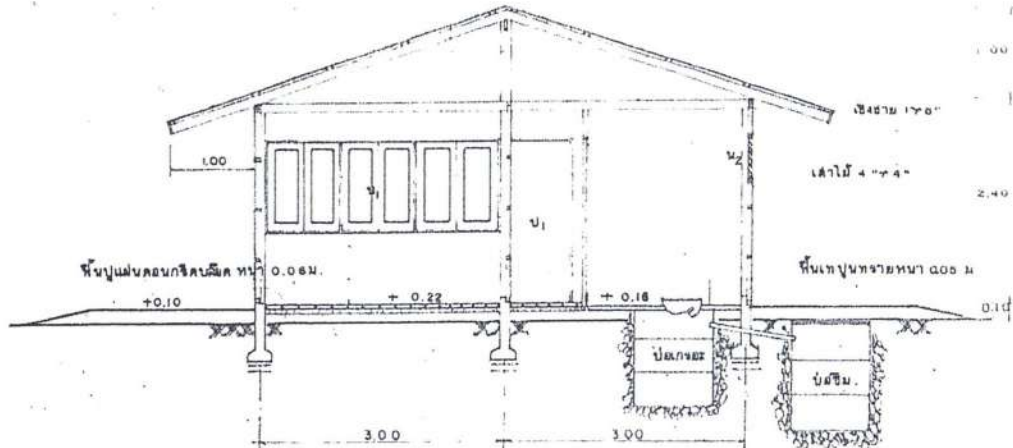
รูปตัด 1850
