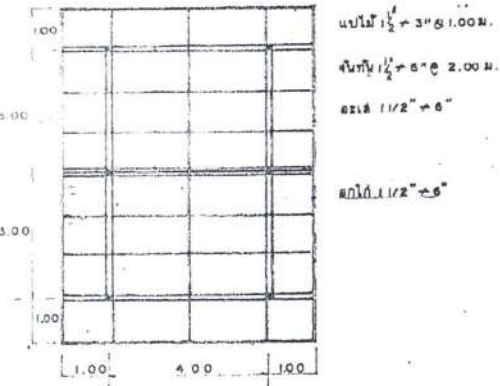
แปลนโครงหลังคา 18100
