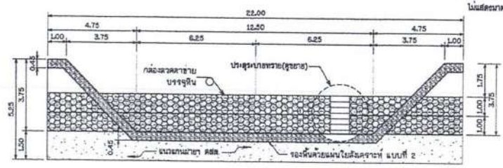
รูปตัด ข-ข ไม้เสริมหน้ากว้าง
