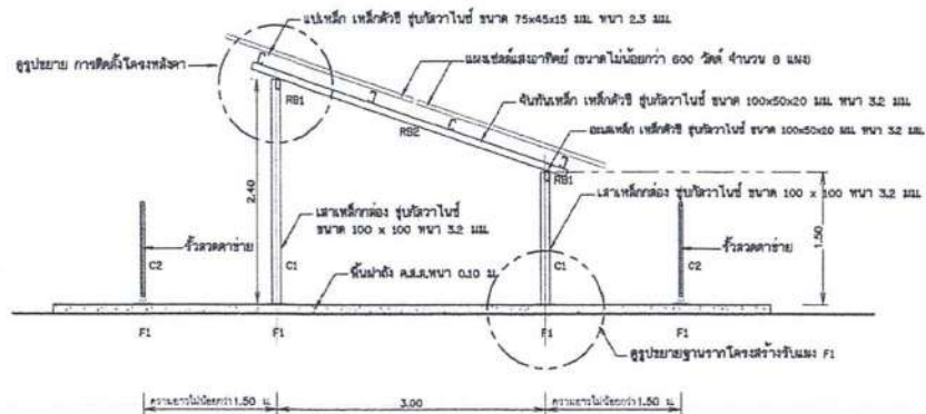
รูปด้านข้าง
