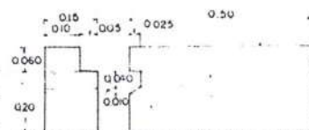
ขยายค้ำยันคอนกรีต 1810
