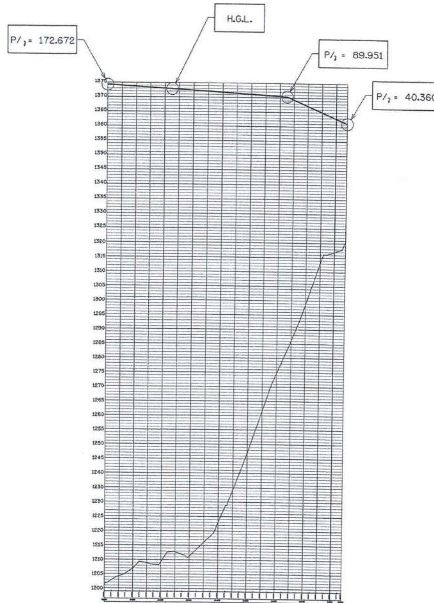
รูปตัดตามแนวยาวแสดง H.G.L. สาย 1RMP STA. 0+000 - 0+840
