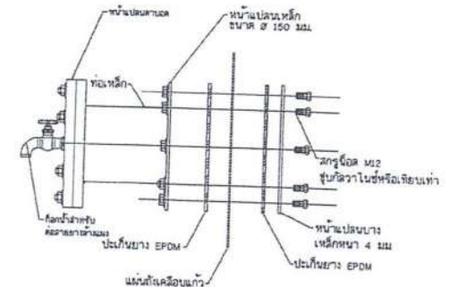
แบบขยายหน้าต่างปลดดาบอด scale NTC.
