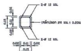
รูปตัด ข - ข
