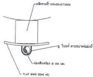
แบบขยาย 6 scale NTC.
