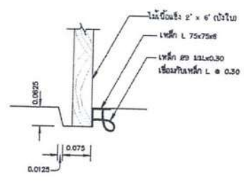
รูปขยาย 1 ขนาดจริง 1:5
