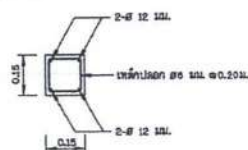
รูปตัด ก - ก
