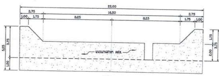
รูปตัด ค-ค ไม้เสริมหน้ากว้าง
