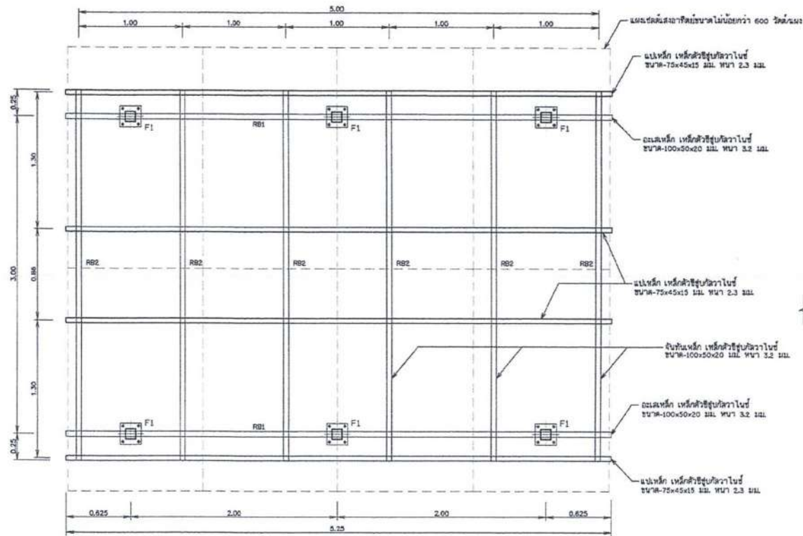
รูปขยายฐานรากโครงสร้างรับแผง F1 (ต่อหน้า คสล. หลังสร้างจุดปัดน้ำฝน)
