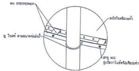
แบบขยาย 2 scale NTC.
