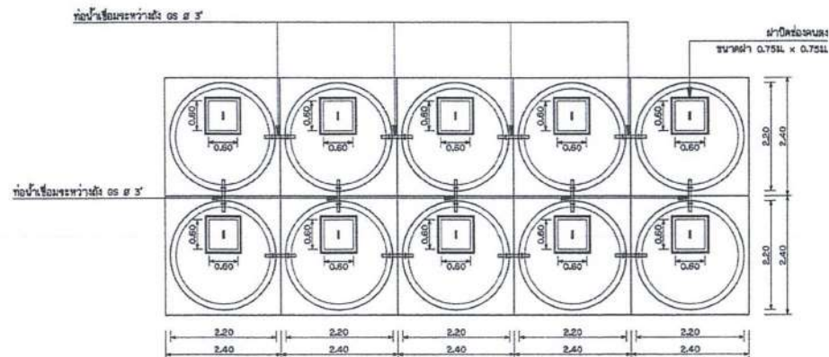
แปลนแบบ 10 ถัง ไม่แสดงขนาดราส่วน
