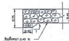
รูปขยาย 1 ไม่แสดงค่า
