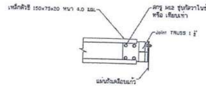
แบบขยาย 3 scale NTC.
