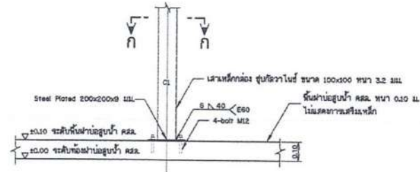
รูปขยายฐานรากโครงสร้างรับแผง F1 (ต่อหน้า คสล. หลังสร้างจุดปัดน้ำฝน)
