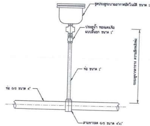
การติดตั้งประตูปะบายอากาศอัตโนมัติ โมเดลมาตรฐาน
