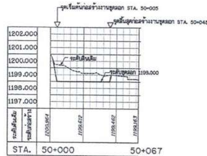
รูปตัดตามแนวยาว งานขุดลอก โมดูลมาตรฐาน
