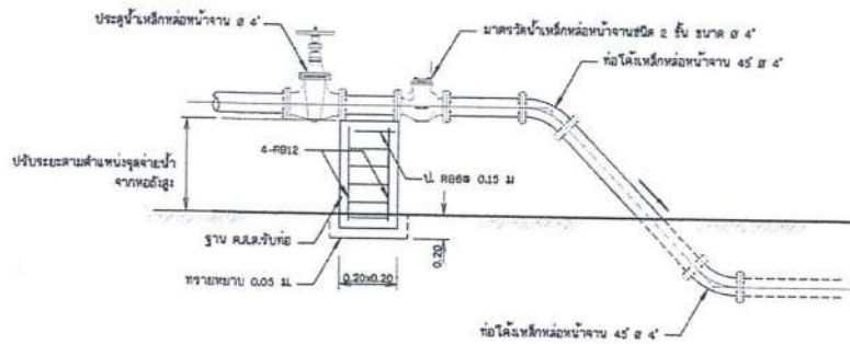
การติดตั้งมาตรวัดน้ำบนพื้นดิน ๔ ๔ โมเดลมาตรฐาน
