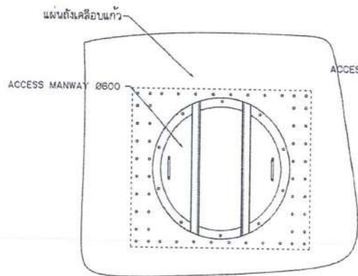
แบบขยาย 5 scale NTC.
