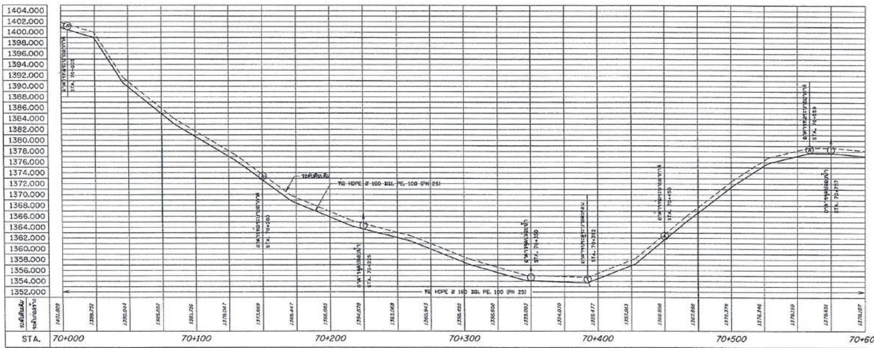
ตัดตามแนวยาว STA. 70+000 - 70+600
