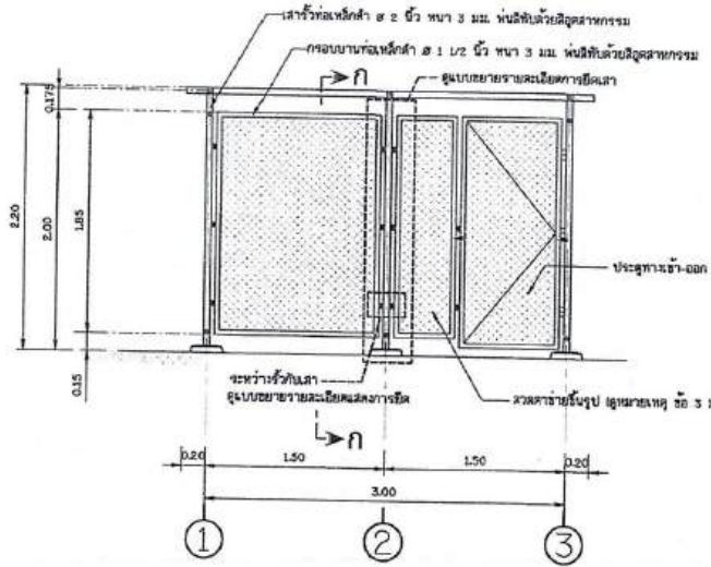
แบบขยายรั้ว 1 ไม่ลดขนาดส่วน
