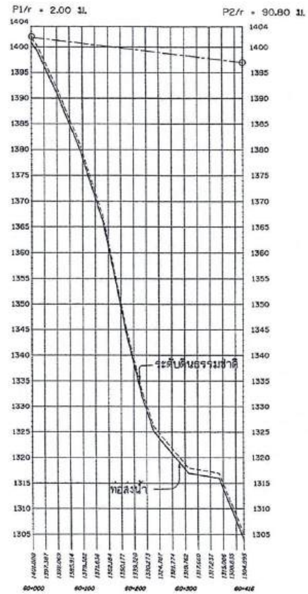
รูปตัดตามแนวยาวแสดง H.G.L. 60+000 - 60+416
