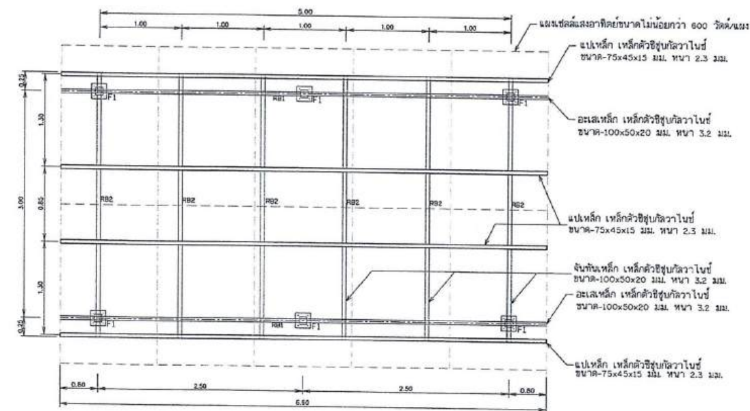
แปลนฐานรากและโครงหลังคา โมเดลมาตรฐาน
