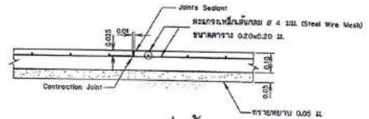
แบบขยายรอยต่อพื้น โมเดลมาตรฐาน
