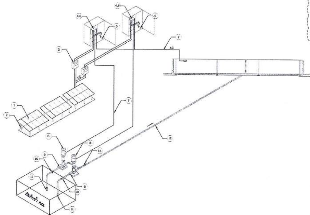
แผนผังระบบไฟฟ้า และ ไดอะแกรมไฟฟ้า ระบบกระจายน้ำด้วยพลังงานแสงอาทิตย์ ขนาด 11 กิโลวัตต์
