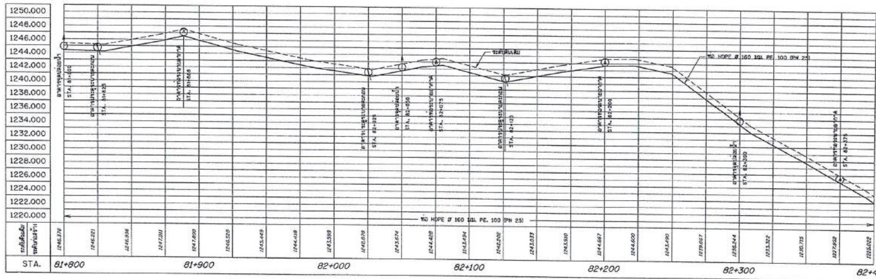
รูปตัดตามแนวยาว STA. 81+800 - 82+400
