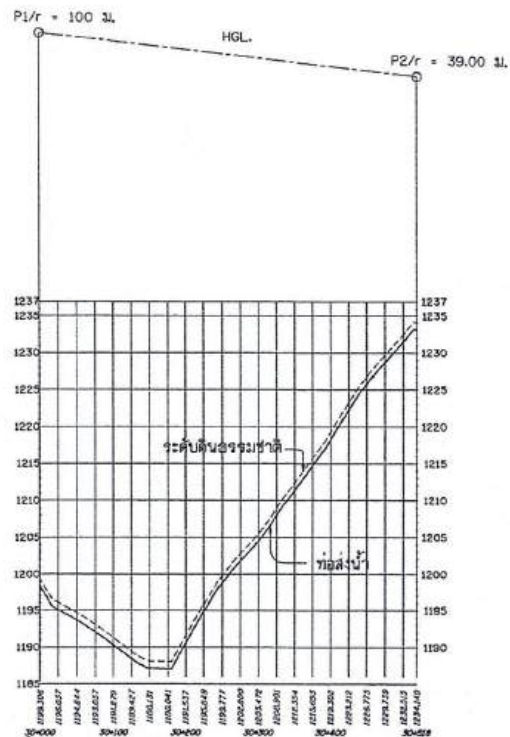
รูปตัดตามแนวยาวแสดง H.G.L. 30+000 - 30+518
