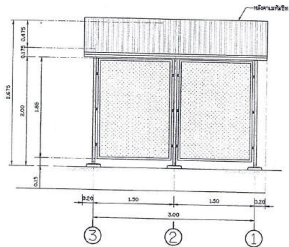
รูปด้าน 3 โมเดลมาตรฐาน
