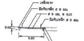
รูปตัดแนว 4 - 4
