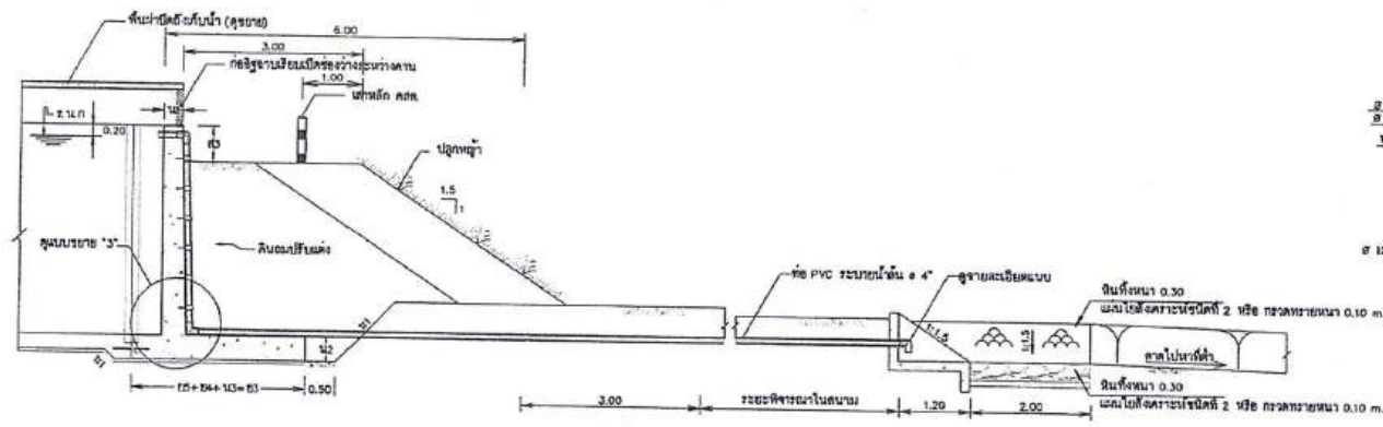
รูปตัด ข - ข
