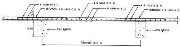
ขยายการเสริมเหล็กพื้นผาปิดถึงเก็บน้ำ
