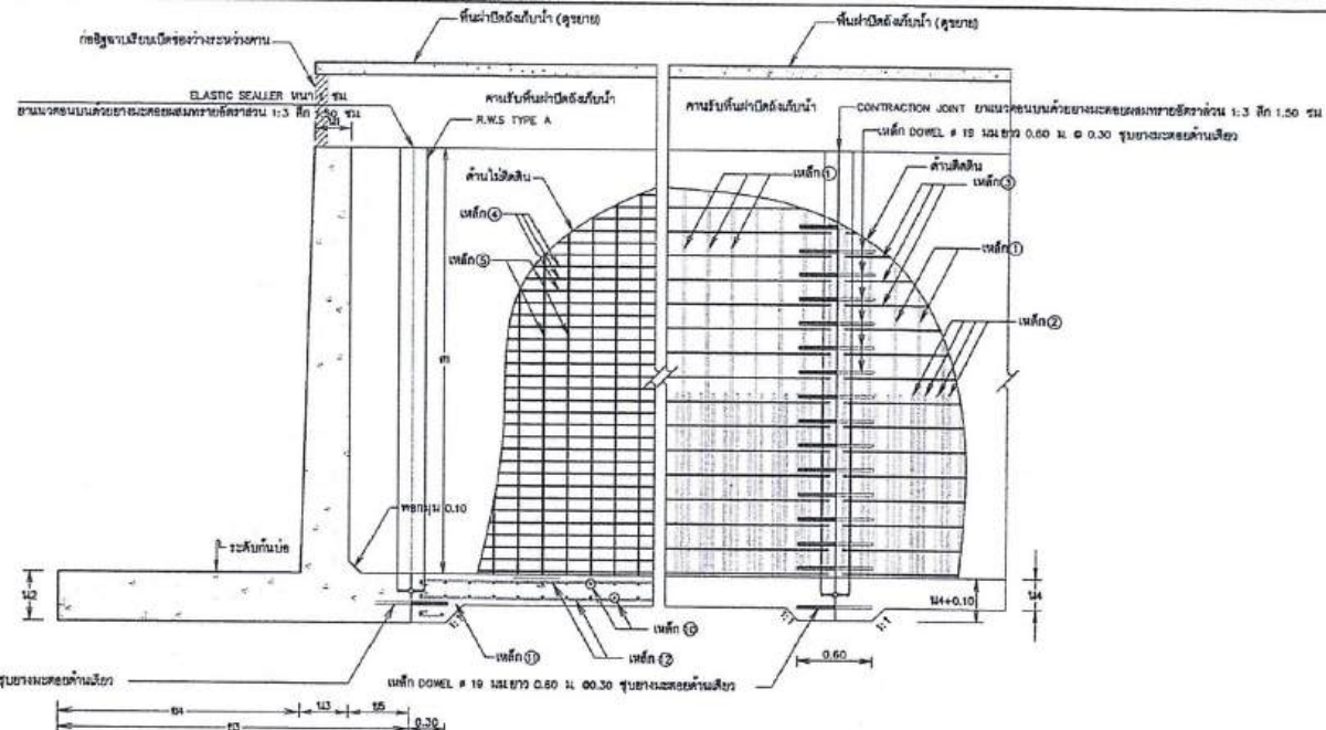
รูปตัดแนว ง - ง
