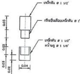
แบบขยายบานพับเหล็ก ไม่ลดขนาดส่วน
