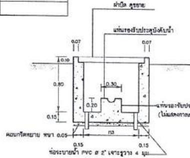
รูปตัด 2 - 2
