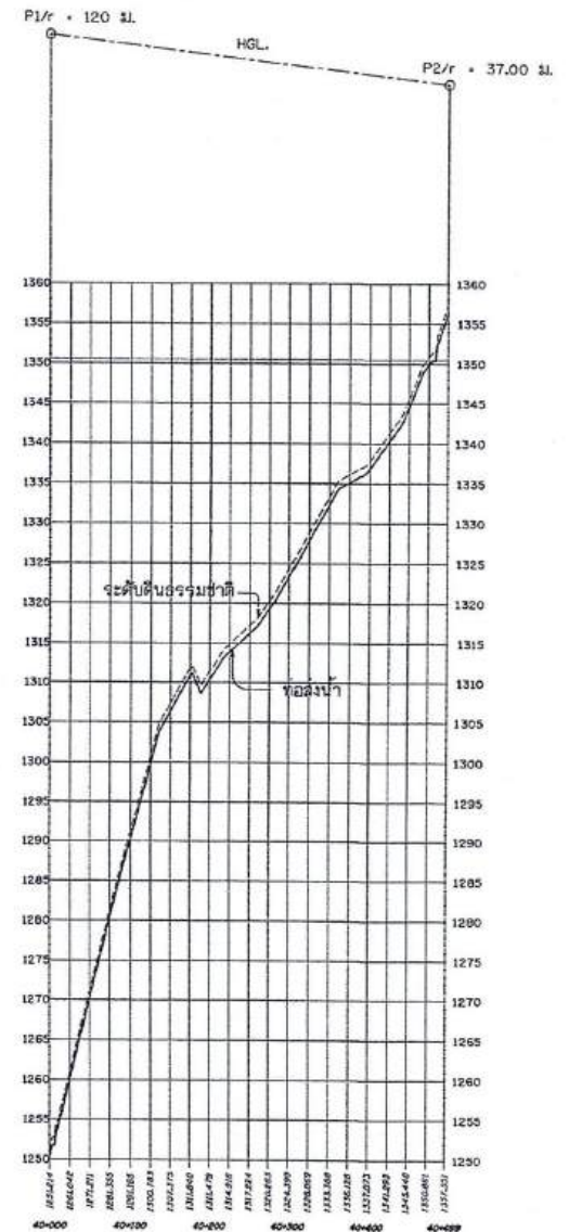
รูปตัดตามแนวยาวแสดง H.G.L. 40+000 - 40+499
