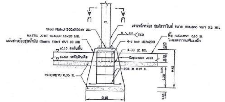
รูปขยายฐานรากโครงสร้างรับแผง F1 (ต่อหน้า คส.ล. ท่อสำหรับรูปพรรณสเปก) โมเดลมาตรฐาน
