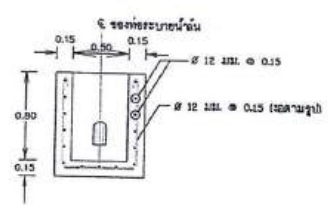
รูปตัดแนว 1 - 1
