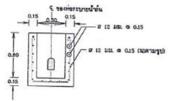
รูปตัดแนว 1 - 1
