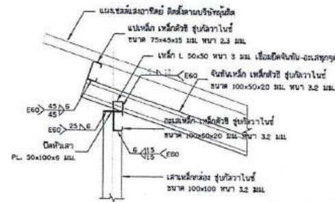
รูปขยาย การติดตั้งโครงหลังคา โมเดลมาตรฐาน
