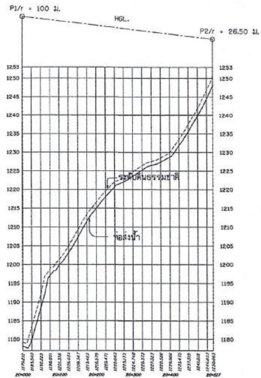
รูปตัดตามแนวยาวแสดง H.G.L. 20+000 - 20+518
