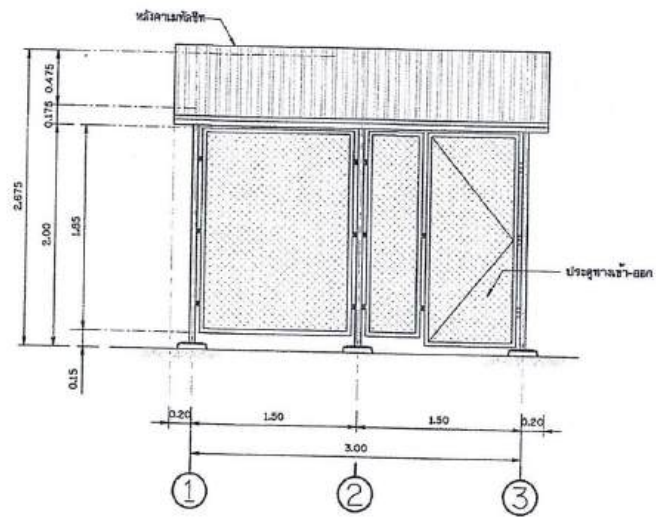
รูปด้าน 1 โมเดลมาตรฐาน
