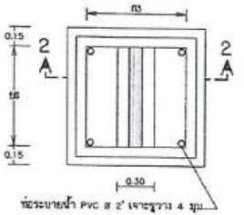
แปลนบ่อประจุถังเก็บน้ำ
