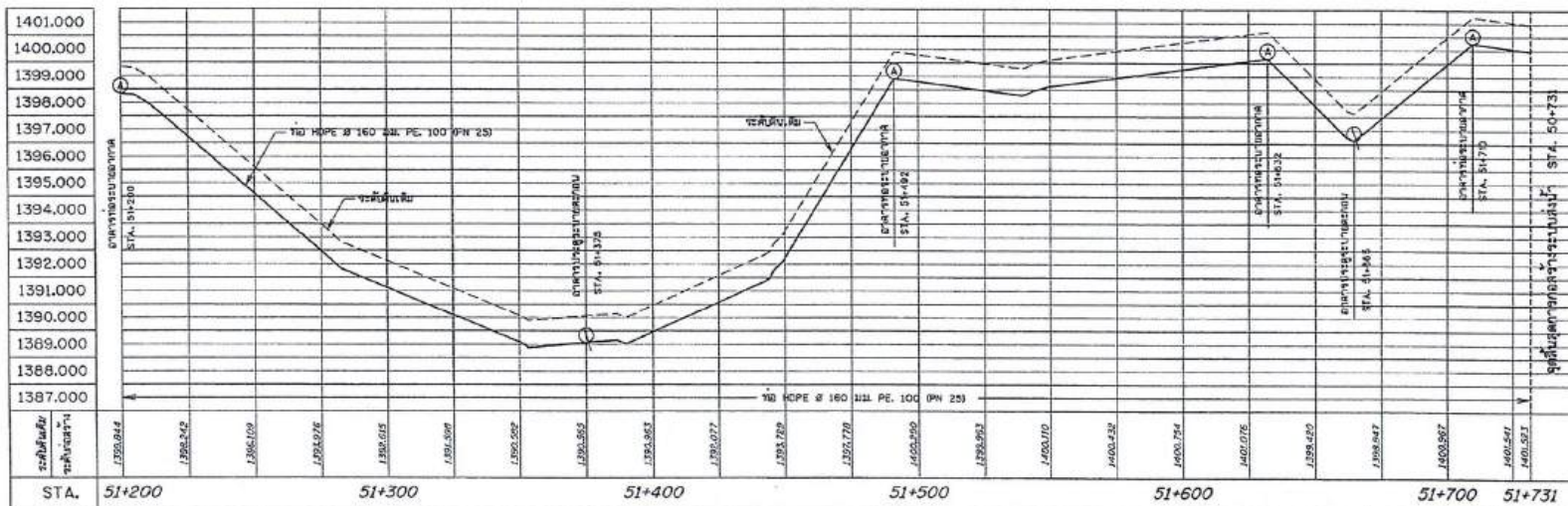
รูปตัดตามแนวยาว STA. 51+200 - 51+731
