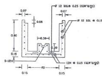
เหล็กเสริมบ่อประจุบึงค้ำน้ำ
