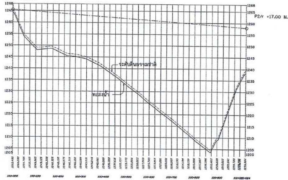
รูปตัดตามแนวยาวแสดง H.G.L. 100+000 - 101+024
