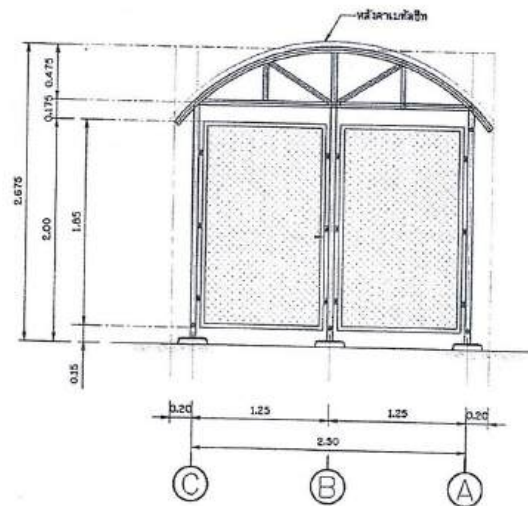
รูปด้าน 4 โมเดลมาตรฐาน
