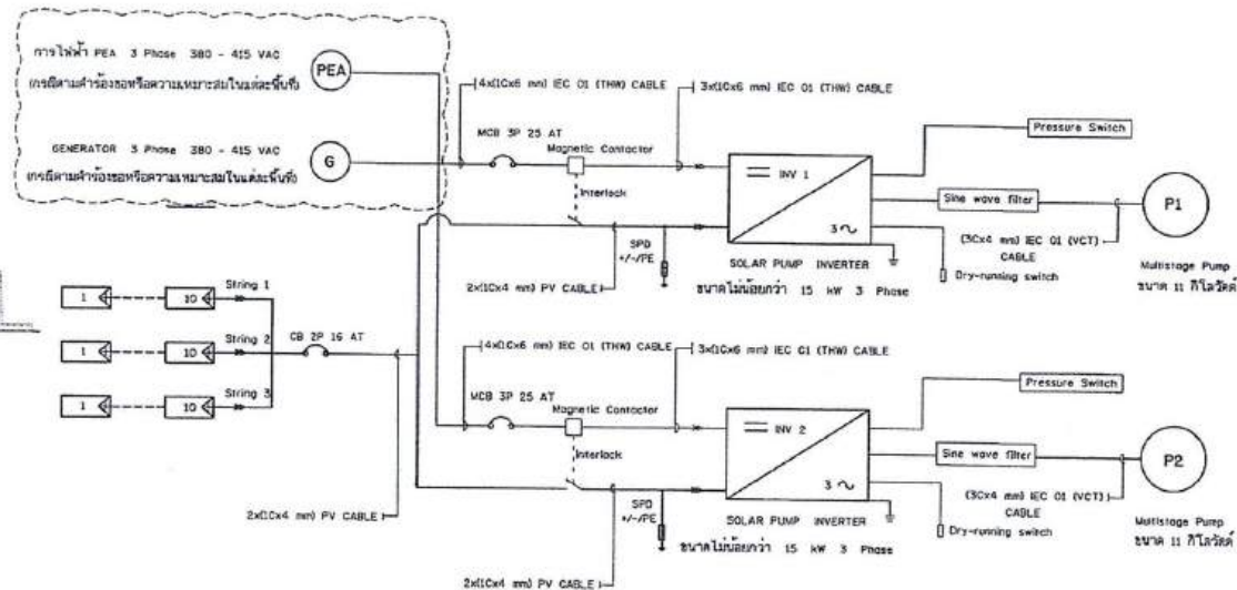
แผนผังระบบไฟฟ้า และ ไดอะแกรมไฟฟ้า ระบบกระจายน้ำด้วยพลังงานแสงอาทิตย์ ขนาด 11 กิโลวัตต์
