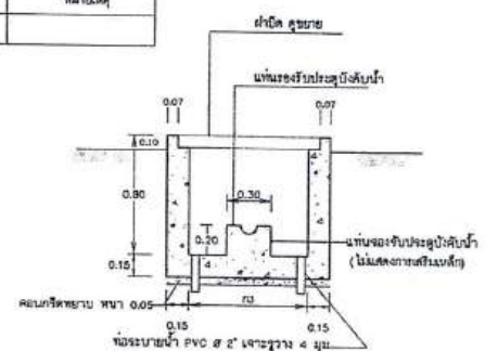
รูปตัด 2 - 2
