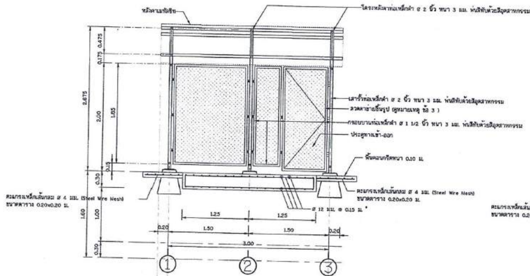
รูปตัด ก - ก ไม่แสดงขนาดส่วน
