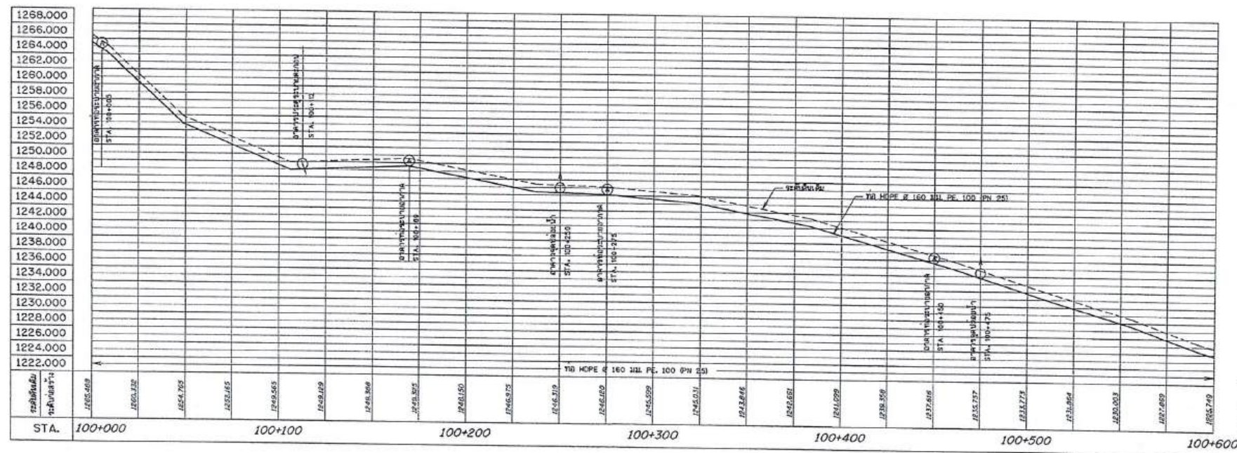
รูปตัดตามแนวยาว STA. 100+000 - 100+600 มาตราส่วน 1:200 แนวตั้ง 1:1,000
