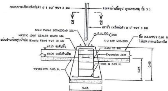
รูปขยายฐานรากโครงสร้างรับแผง F2 ต่อแนว คสล. ท่อใส่ไฟรูปหม้อต้มน้ำ
