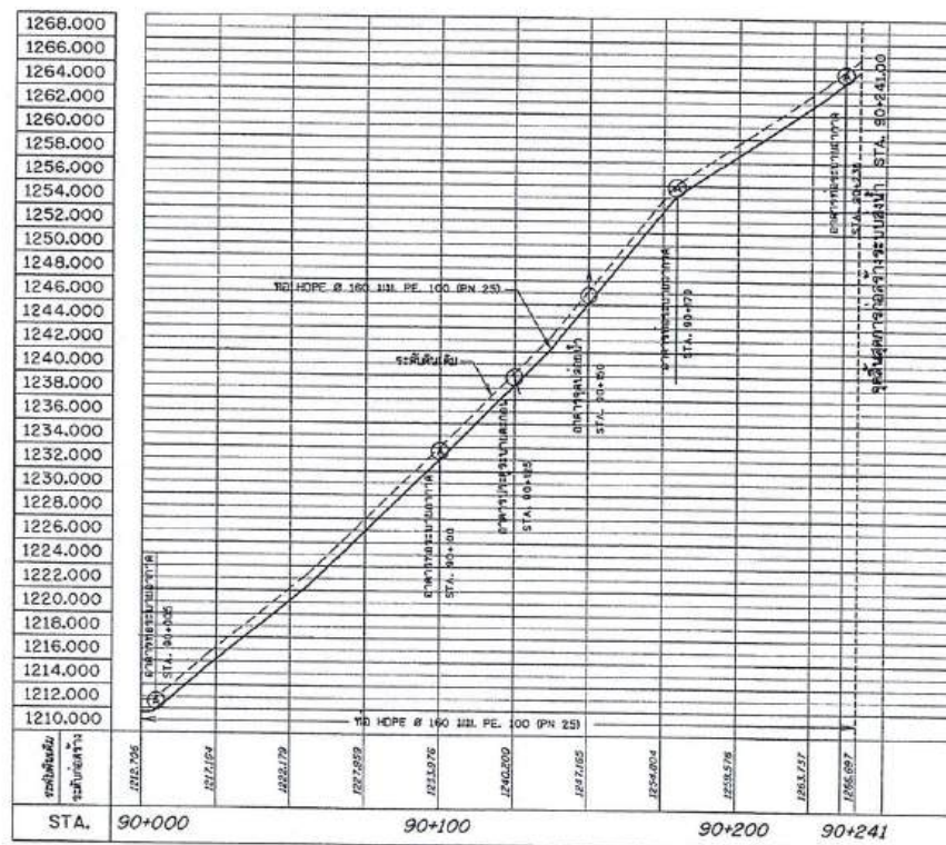
รูปตัดตามแนวยาว STA. 90+000 - 90+241
