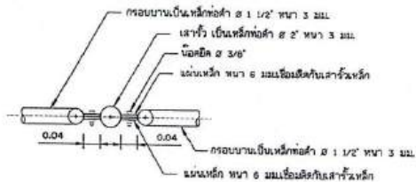
แบบขยายรั้ว 1 ไม่ลดขนาดส่วน
