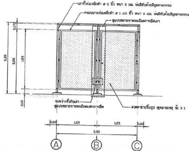
แบบขยายรั้ว 2 ไม่ลดขนาดส่วน
