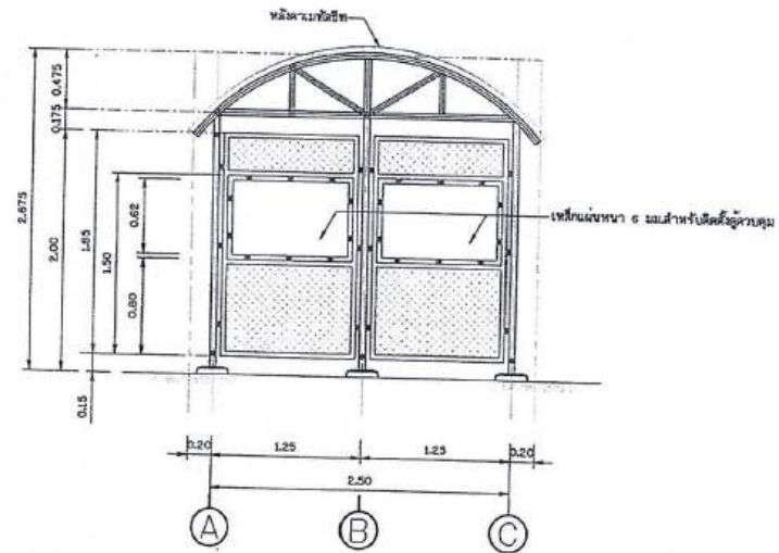
รูปด้าน 2 โมเดลมาตรฐาน
