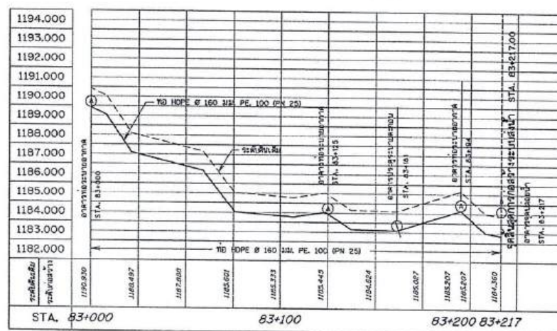
แปลนระบบส่งน้ำ STA. 83+000 - 83+217
