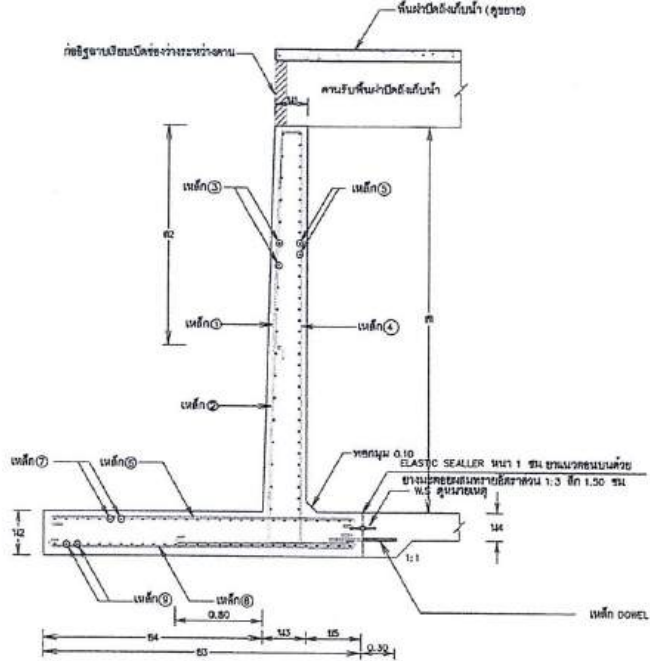
รูปตัดแนว ค - ค
