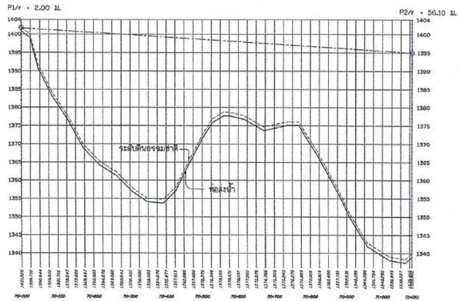
รูปตัดตามแนวยาวแสดง H.G.L. 70+000 - 71+081
