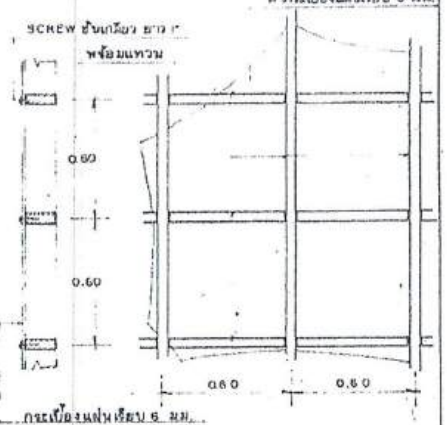
รูปขยายเคาะ ฝา 1:820
