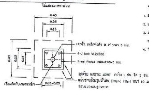
รูปขยายฐานรากโครงสร้างรับแผง F2 ต่อแนว คสล. ท่อใส่ไฟรูปหม้อต้มน้ำ
