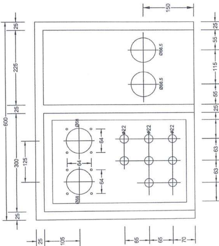
๓ ดานหนา แสดงการเจาะรูเพื่อติดตั้งอุปกรณ์
