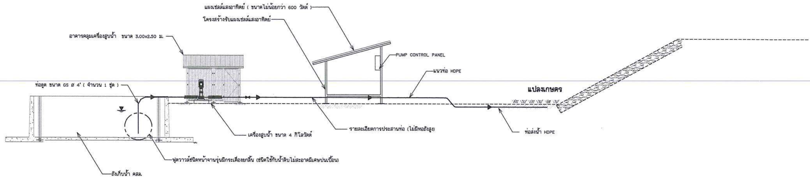
รูปด้านแผนผังระบบกระจายน้ำด้วยพลังงานแสงอาทิตย์ ขนาด 4 กิโลวัตต์ ไม่แสดงขนาดบางส่วน
