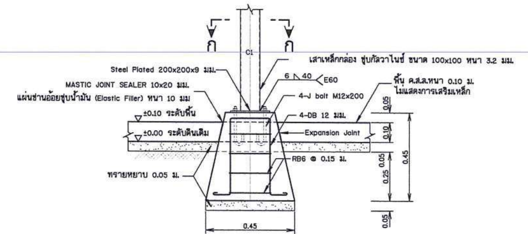
รูปขยายฐานรากโครงสร้างรับแผง F1
