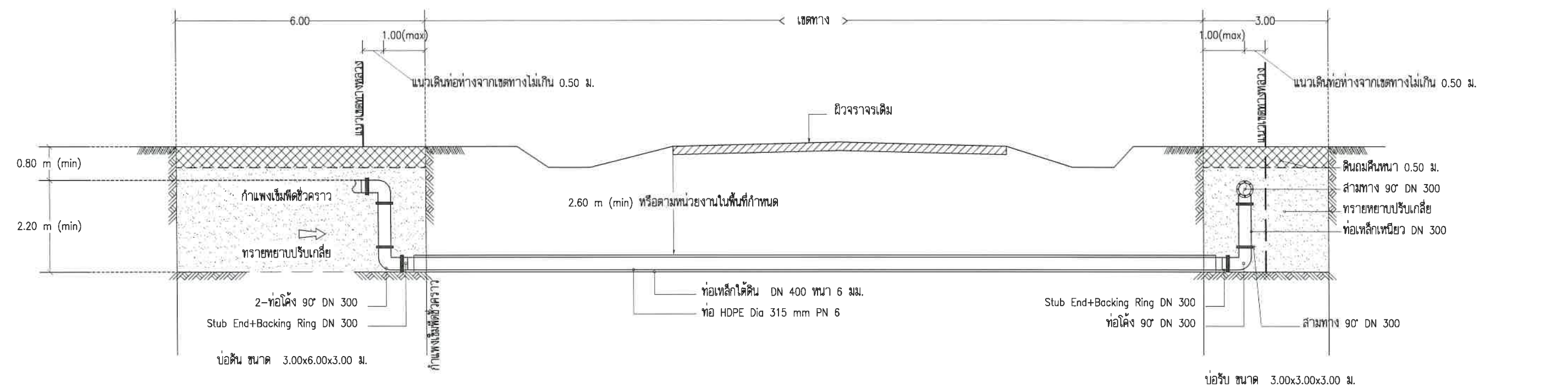
งานดันท่อปลอกลอดถนน (pipe jacking) SCALE 1:100
