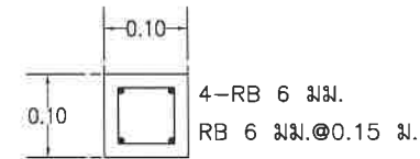
แบบขยายเหล็กเสริมหลักบ่อแกวท่อ มาตราส่วน 1:15
