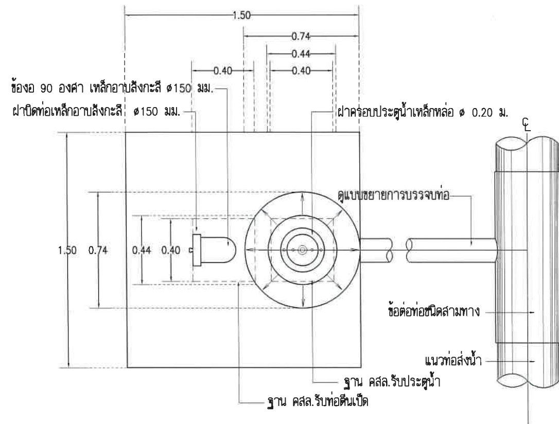
แปลนอาคารระบายตะกอน 1:25
