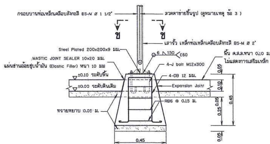
รูปขยายฐานรากโครงสร้างรับแผง F1 (ต่อม่อ คสล. หล่อสำเร็จรูปพร้อมติดตั้ง) ไม่แสดงขนาดจาล้วน
