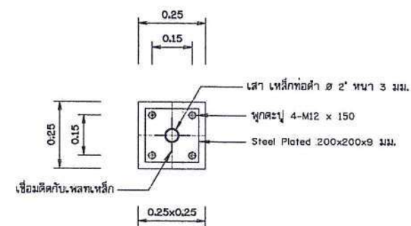
ฐานรากโครงสร้างอาคารคลุม ไม่แสดงขนาดราส่วน
