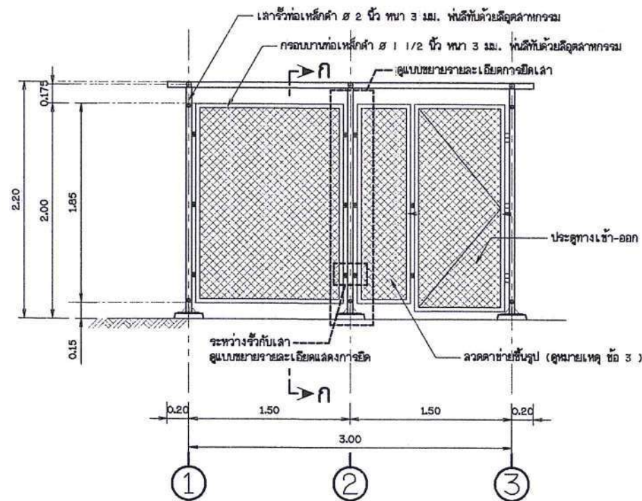
แบบขยายรั้ว 1 ไม่แสดงขนาดราส่วน
