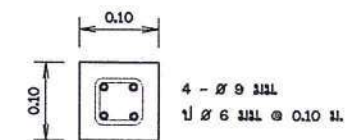
รูปตัดหลักบอกแนวท่อ
