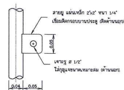
แบบขยายสายยู่ ไม่แสดงขนาดจาล้วน
