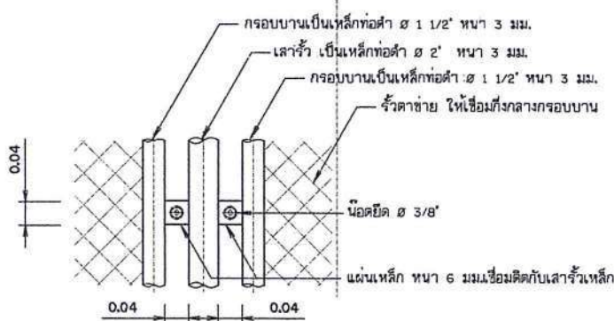
แบบขยายรายละเอียดแสดงการยึดระหว่างรั้วกับเล้า ไม่แสดงขนาดราส่วน
