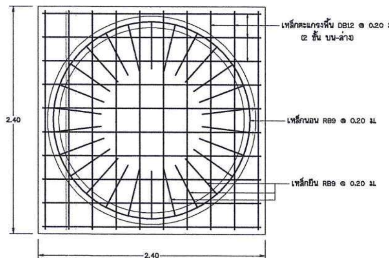
แสดงการเสริมเหล็กพื้นถึง มาตราส่วน 1:20
