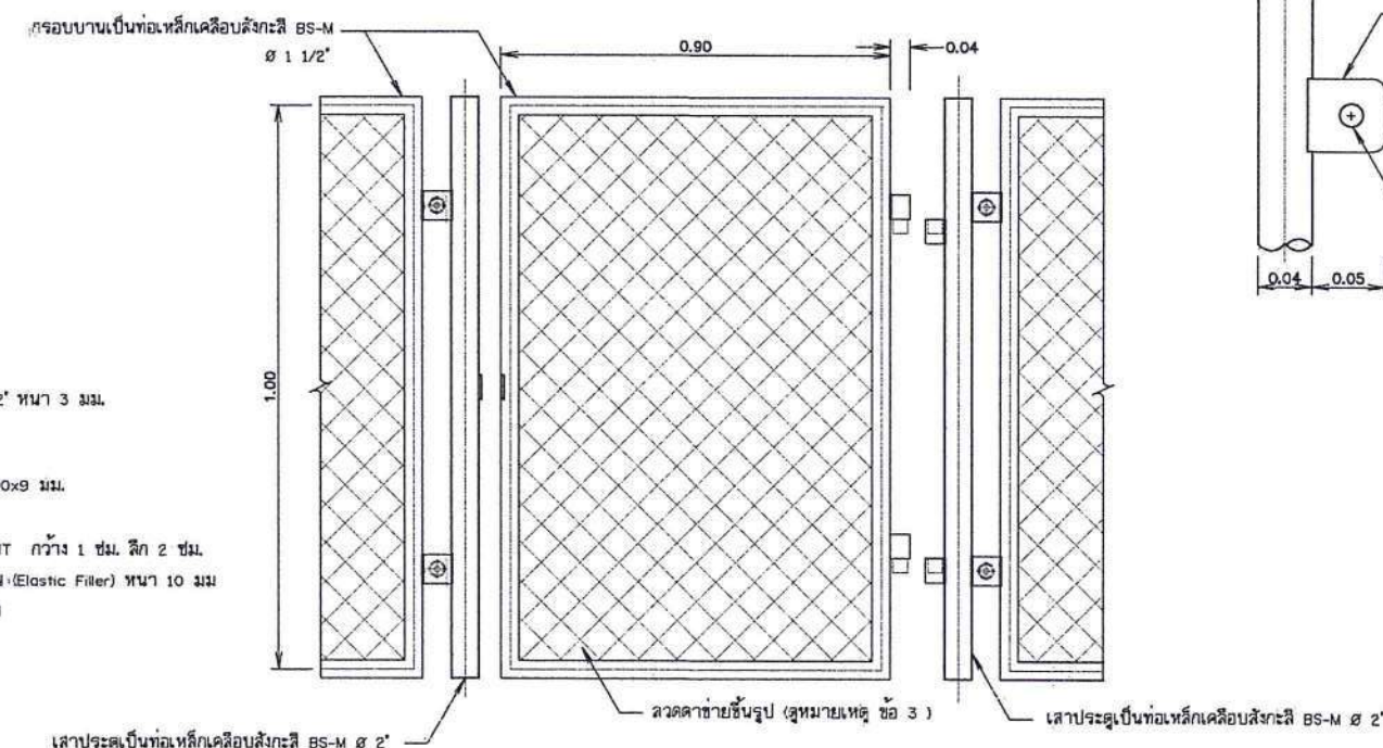
แบบขยายรายละเอียดประตู ไม่แสดงขนาดจาล้วน
