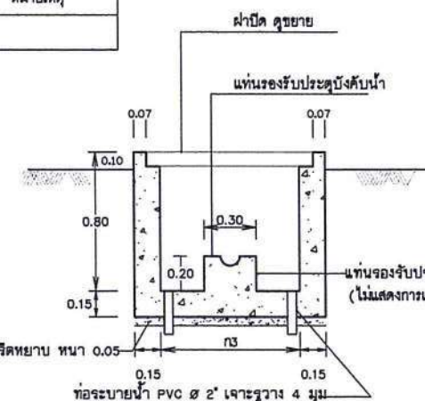
รูปตัด 2 - 2 มาตราส่วน 1:20
