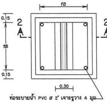
แปลนบ่อประจุบึงค้ำน้ำ มาตราส่วน 1:20
