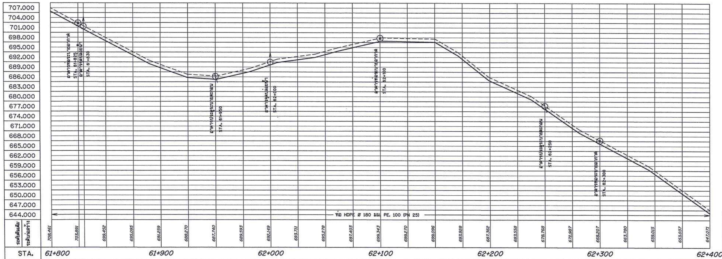
รูปตัดตามแนวยาว STA. 61+800 - 62+400
