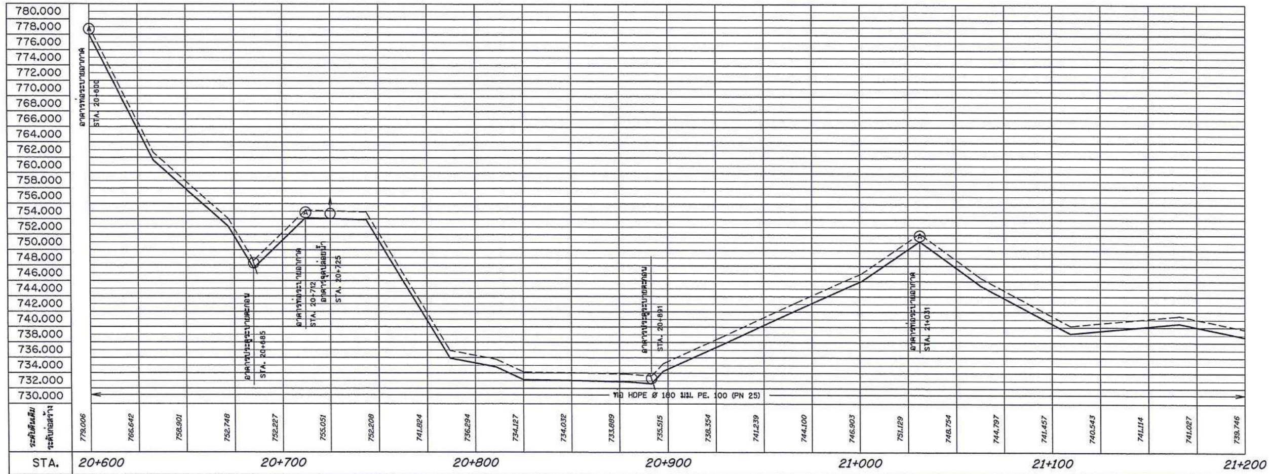
รูปตัดตามแนวยาว STA. 20+600 - 21+200
