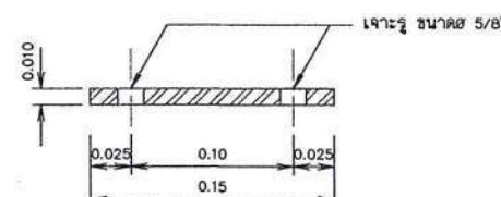
รูปตัด C-C มาตราส่วน 1:10
