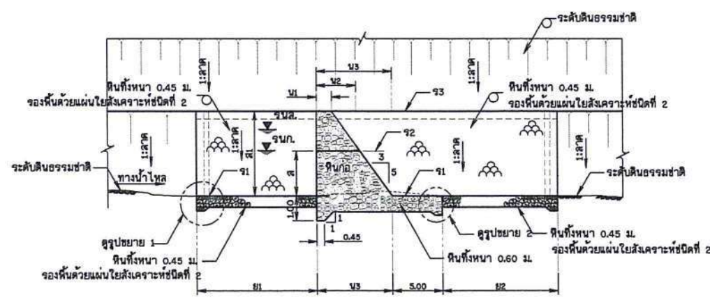
รูปตัด ก - ก
