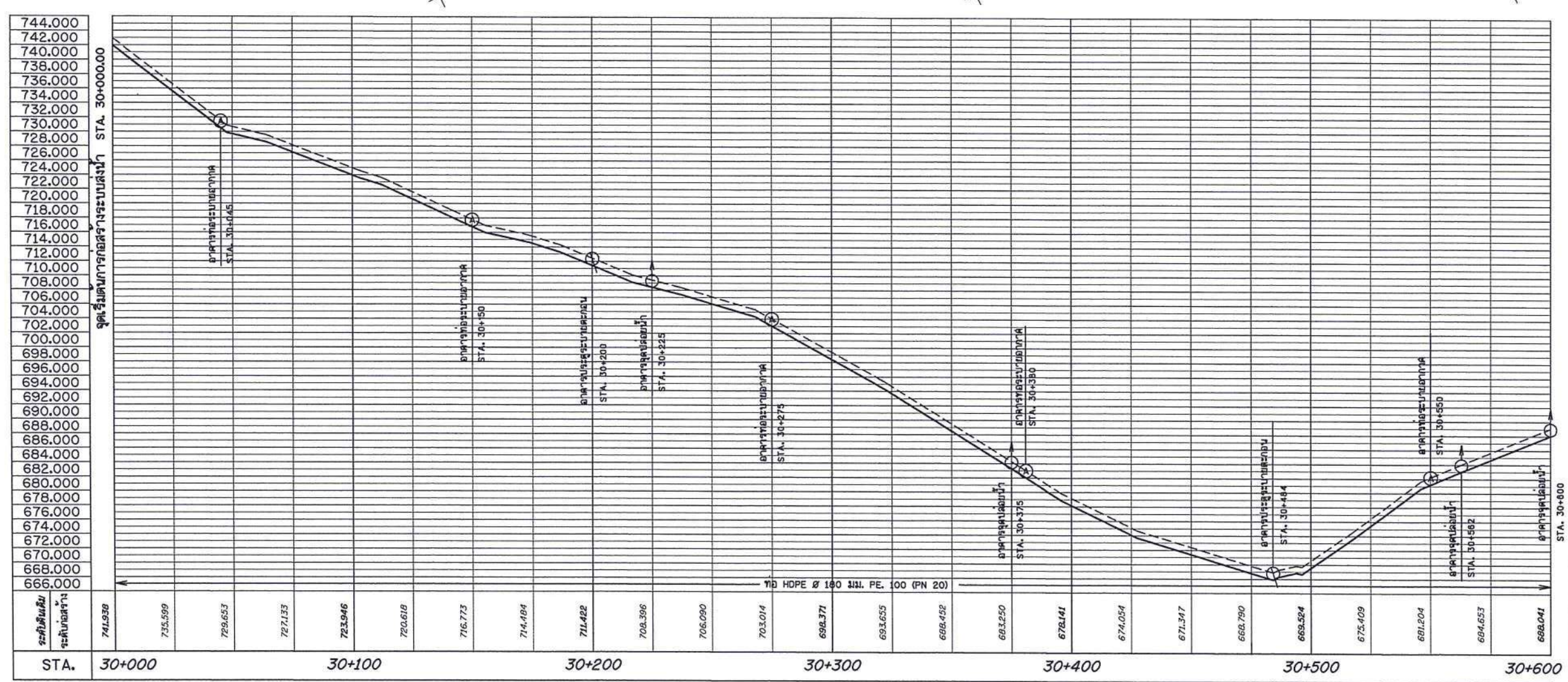
รูปตัดตามแนวยาว STA. 30+000 - 30+600 มาตราส่วน 1:200 แนวตั้ง 1:200 แนวนอน 1:1,000
