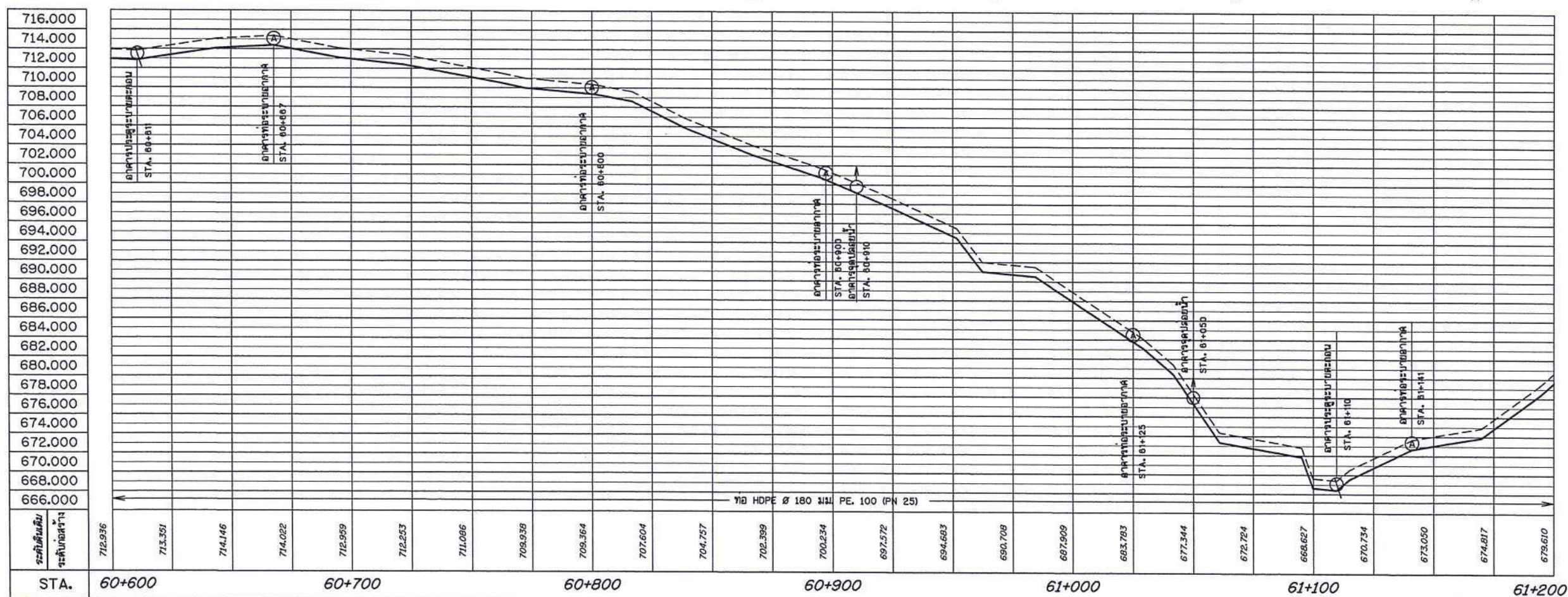
รูปตัดตามแนวยาว STA. 60+600 - 61+200
