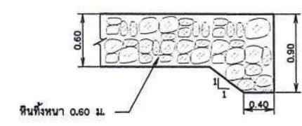
รูปขยาย 2
