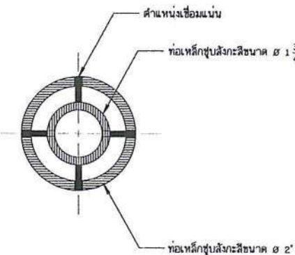
รูปตัด Y-Y มาตราส่วน 1:2.5
