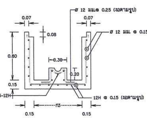
เหล็กเสริมบ่อประจุน้ำ มาตราส่วน 1:20
