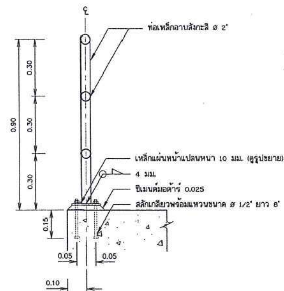
รูปตัด G-G มาตราส่วน 1:10
