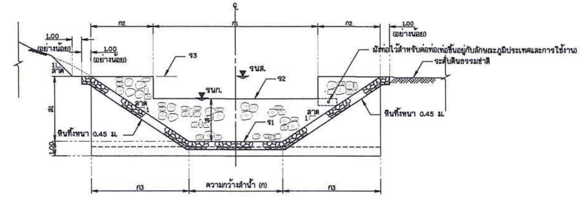
รูปตัด ข - ข
