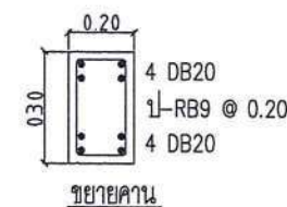
ขยายคาน
