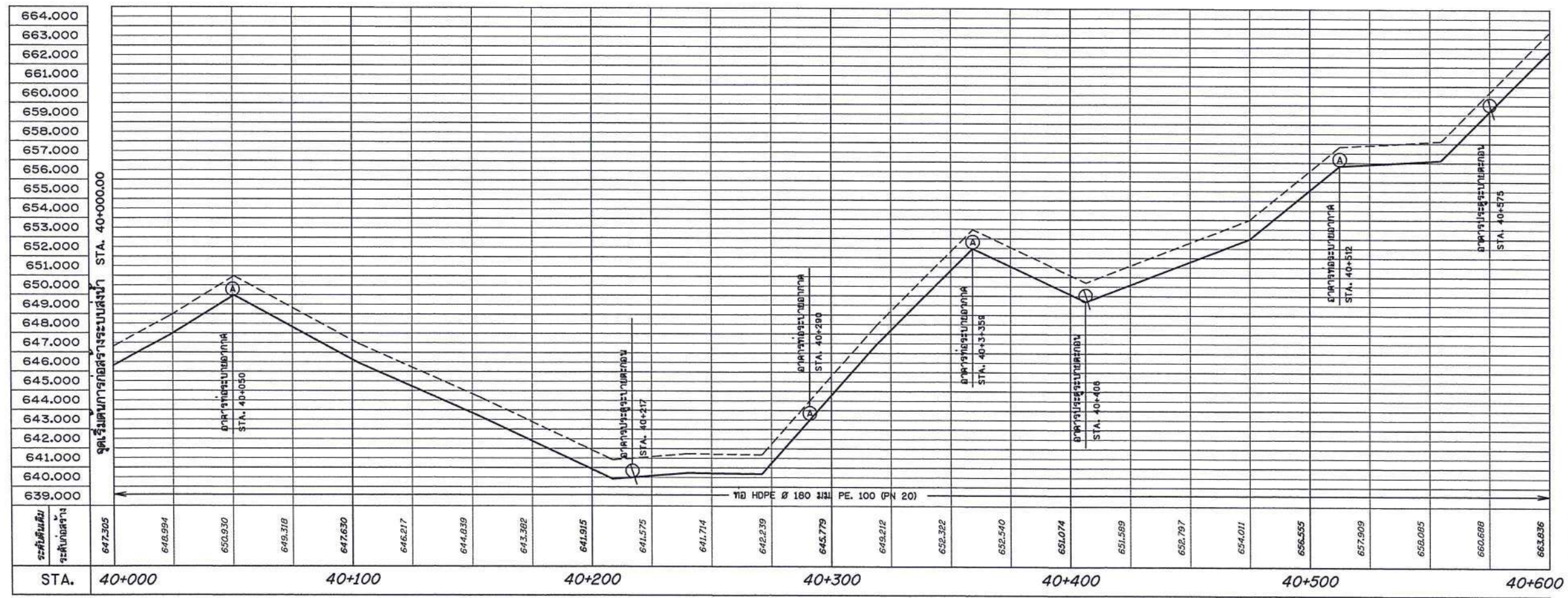
รูปตัดตามแนวยาว STA. 40+000 - 40+600
