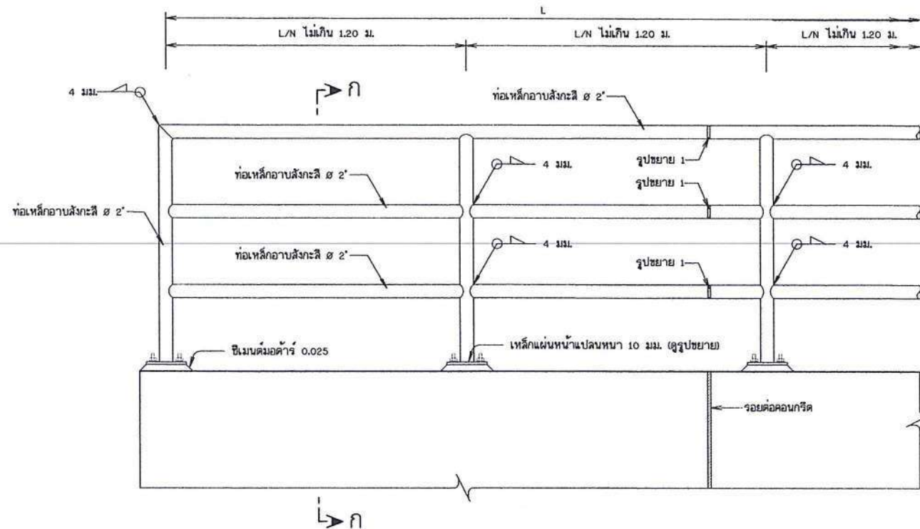
รูปขยายราวเหล็กกันดก มาตราส่วน 1:10
