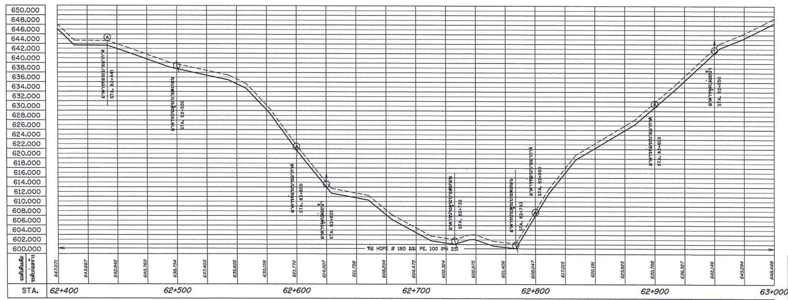
รูปตัดตามแนวยาว STA. 62+400 - 63+000
