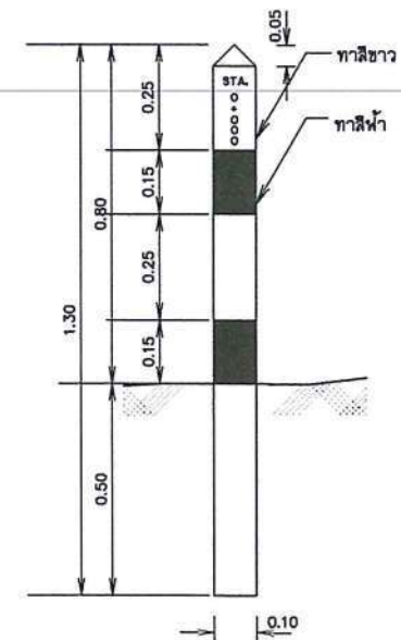
รูปตัดหลักบอกแนวท่อ
