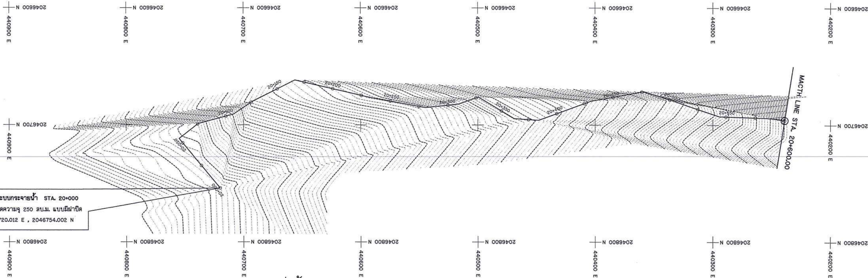
แปลนระบบส่งน้ำ STA. 20+000 - 20+600
