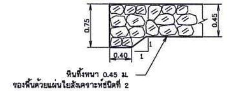
รูปขยาย 1
