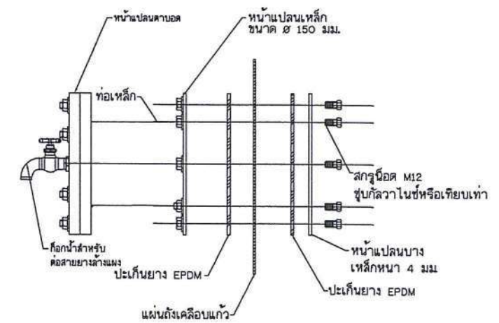
แบบขยายหน้าแปลนคาบอด scale NTC.
