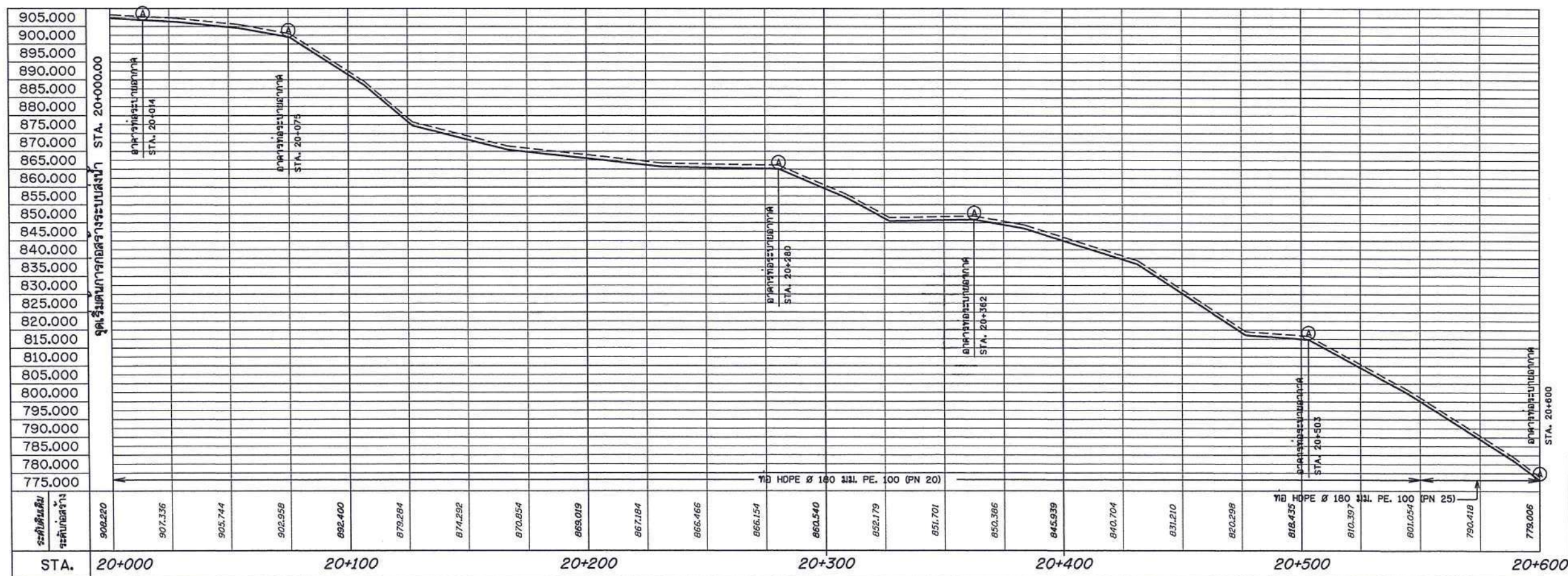
รูปตัดตามแนวยาว STA. 20+000 - 20+600
