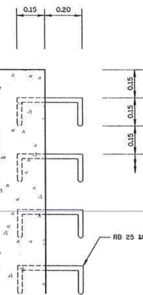
รูปขยายบันได มาตราส่วน 1:10
