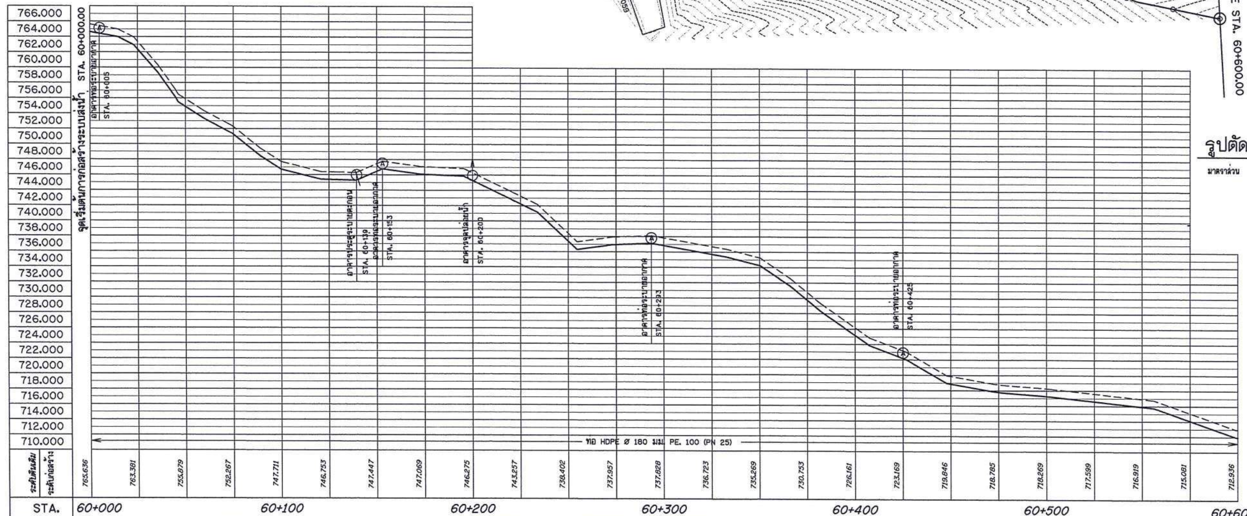
รูปตัดตามแนวยาว STA. 60+000 - 60+600
