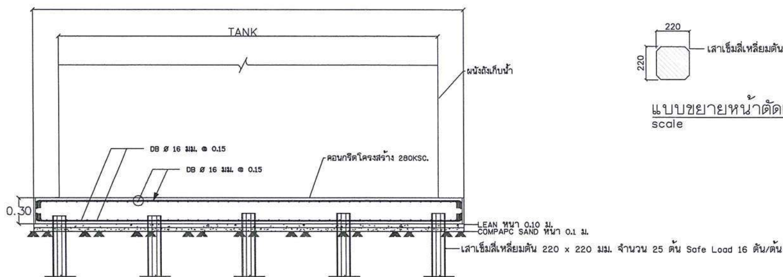
แบบตัด ก-ก scale NTC.
