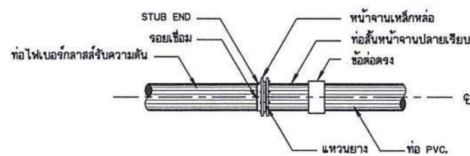
การบรรจุท่อไฟเบอร์กลาสเสริมความดัน กับท่อ PVC.
