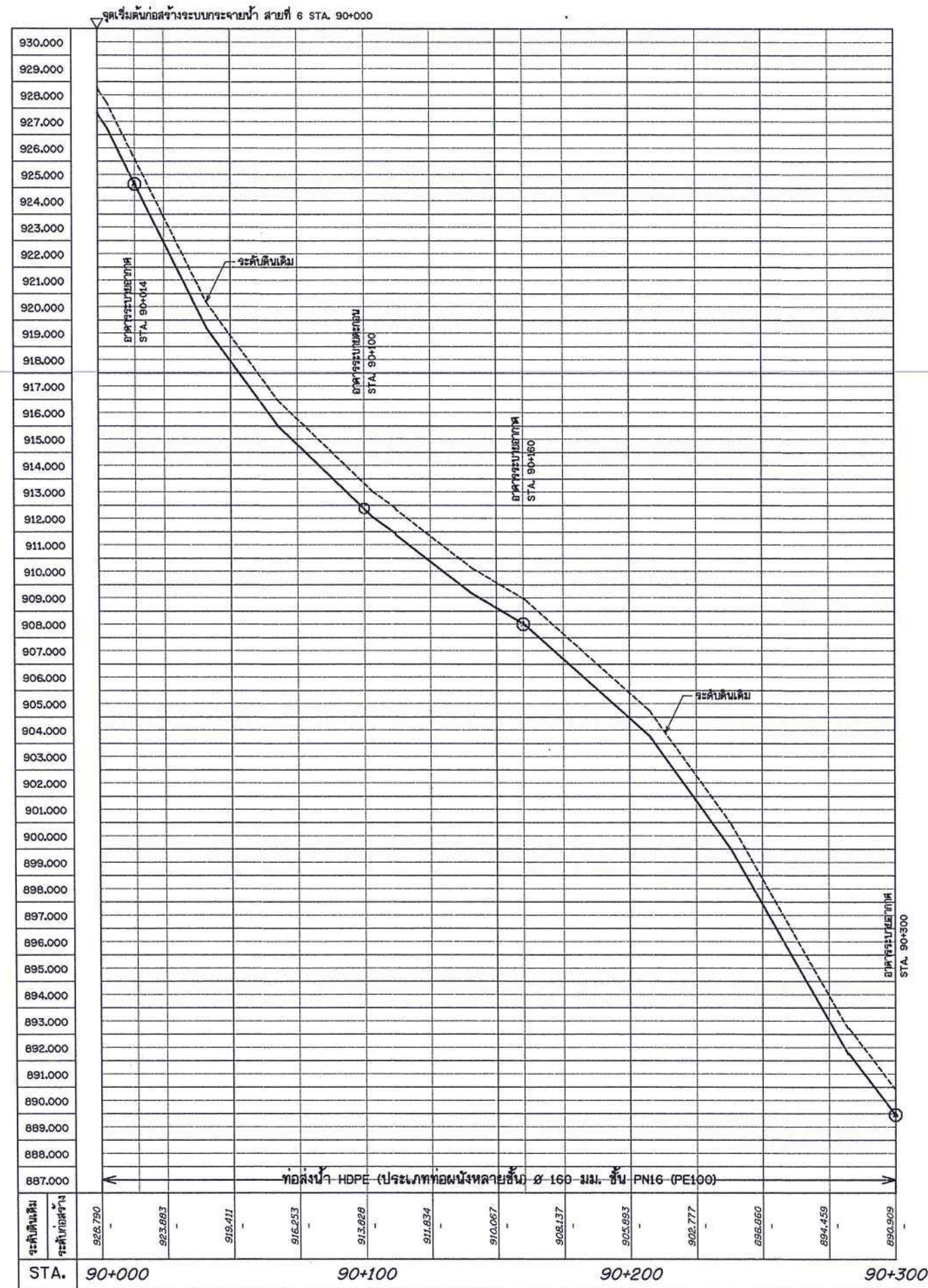
รูปตัดตามแนวยาวระบบกระจายน้ำ สายที่ 6
