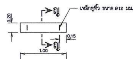
แปลนฝาบ่อดักตะกอน มาตราส่วน 1 : 10
