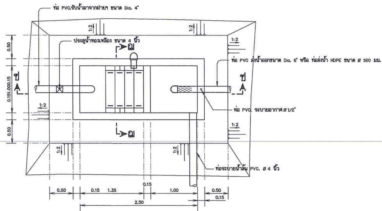
แปลนบ่อดักตะกอน มาตราส่วน 1 : 25
