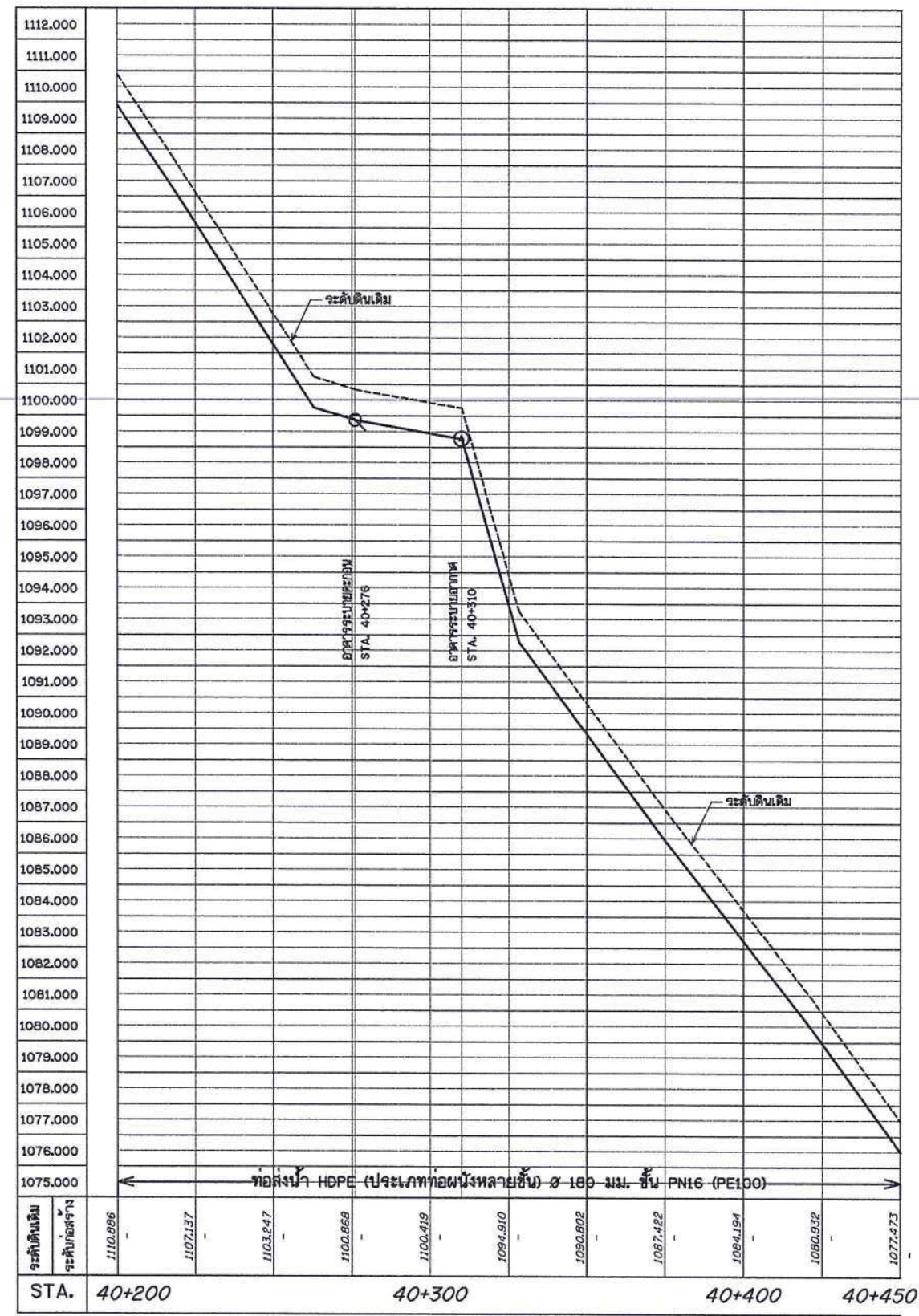
รูปตัดตามแนวยาวระบบกระจายน้ำ สายที่ 3 มาตรฐาน มาตรฐาน มาตรฐาน 1:1,000 มาตรฐาน 1:100
