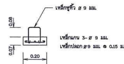
รูปตัด ญ - ญ มาตราส่วน 1 : 10
