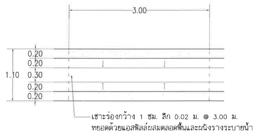
แปลนวางระบายน้ำ มาตราส่วน 1:50
