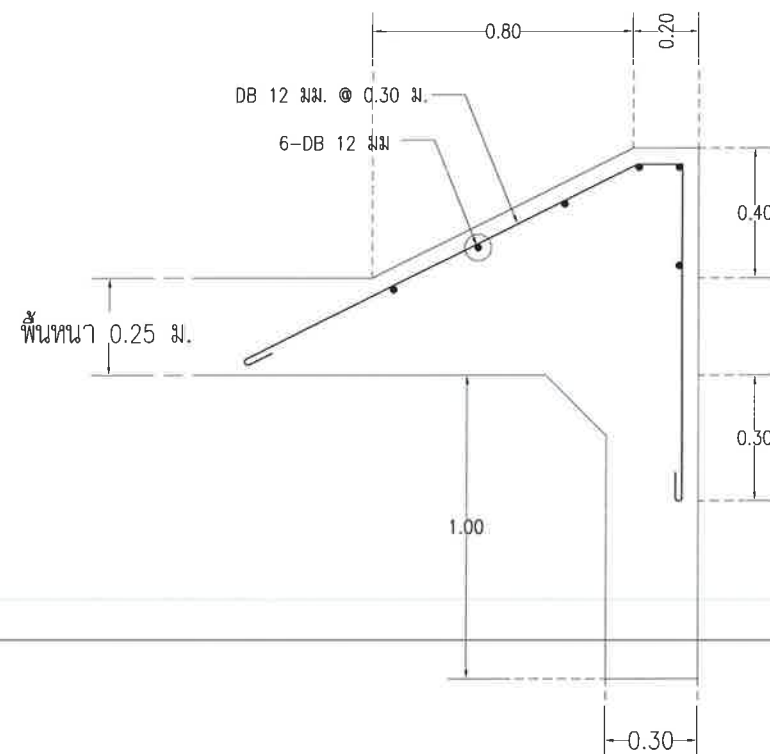
แบบขยาย End Sill มาตราส่วน 1:25
