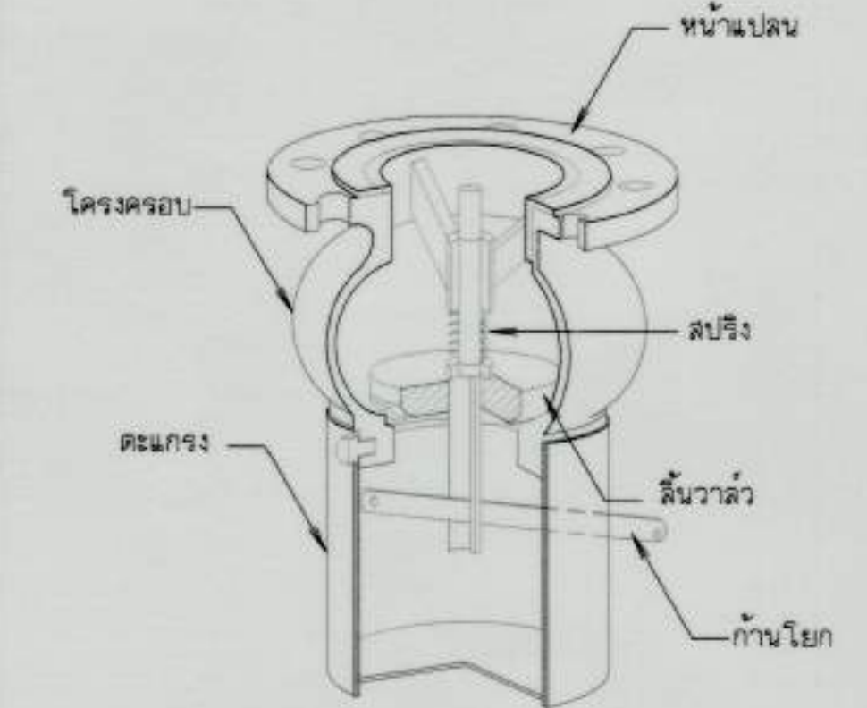
15. ฟุตวาล์ว แบบก้านโยก ไม่แสดงมาตราส่วน
