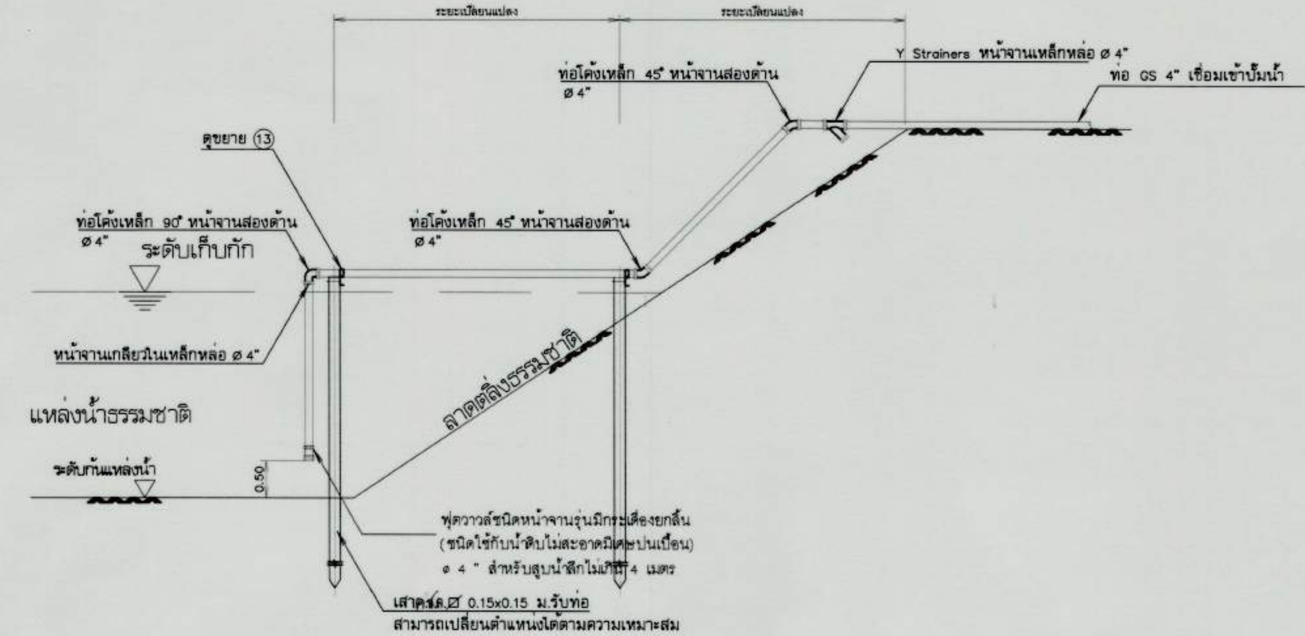
แบบขยายการเดินท่อจากแหล่งน้ำดิบ
