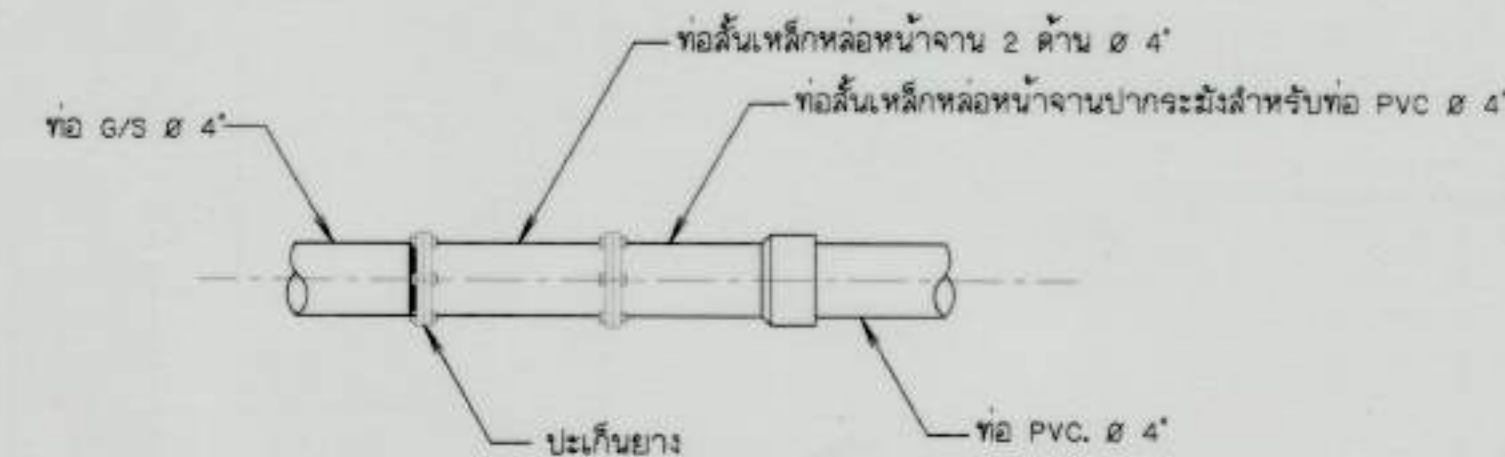
8. การบรรจบท่อเหล็กทาบสังกะสี G/S กับท่อ PVC. ไม่แสดงมาตราส่วน
