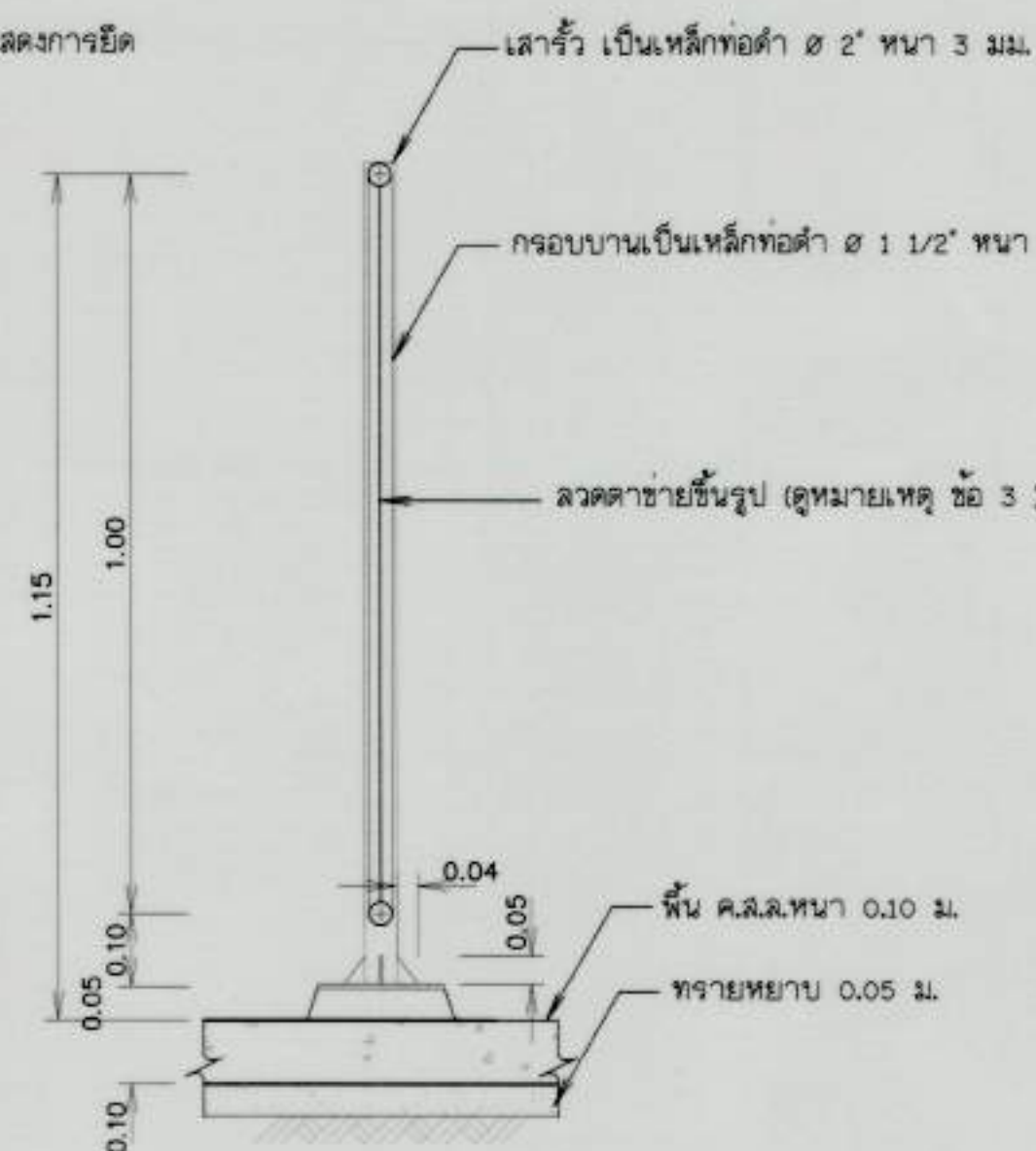
รูปตัด ก-ก
