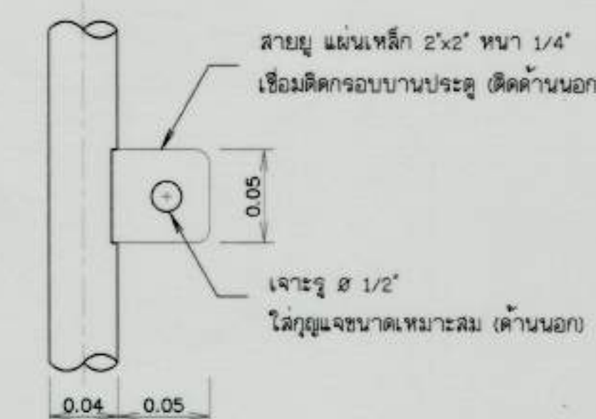
แบบขยายสายยู
