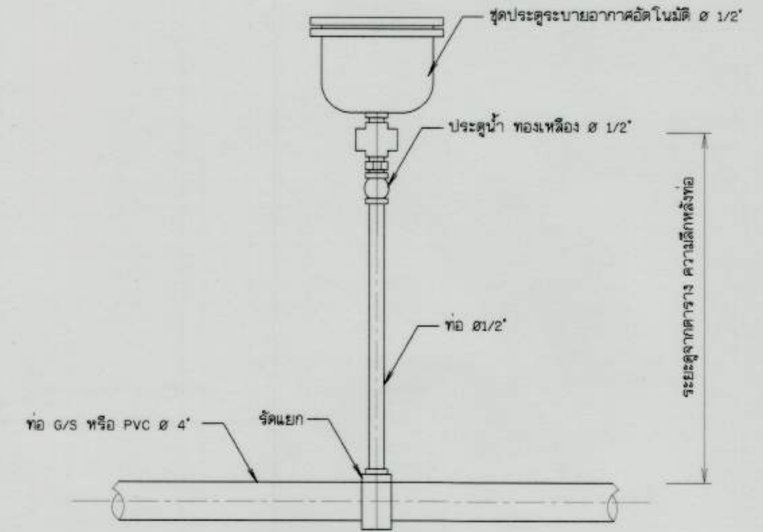
12. การติดตั้งประตูปะบายอากาศอัตโนมัติ ไม่แสดงมาตราส่วน
