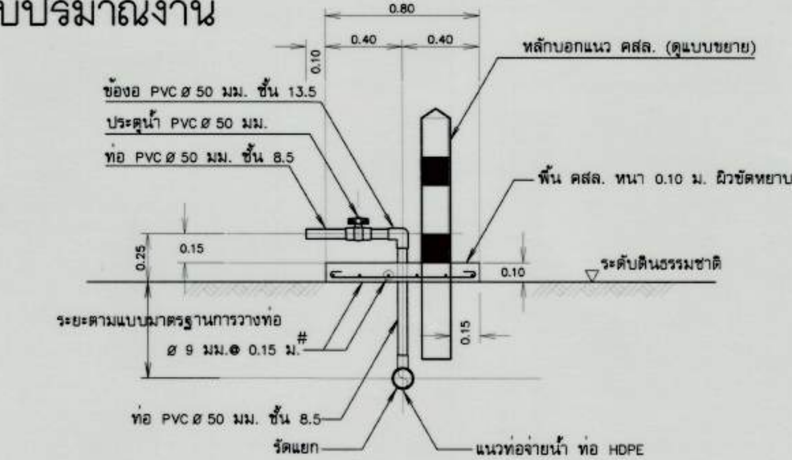
รูปตัด ก - ก แสดงการติดตั้งอาคารจุดปล่อยน้ำ
