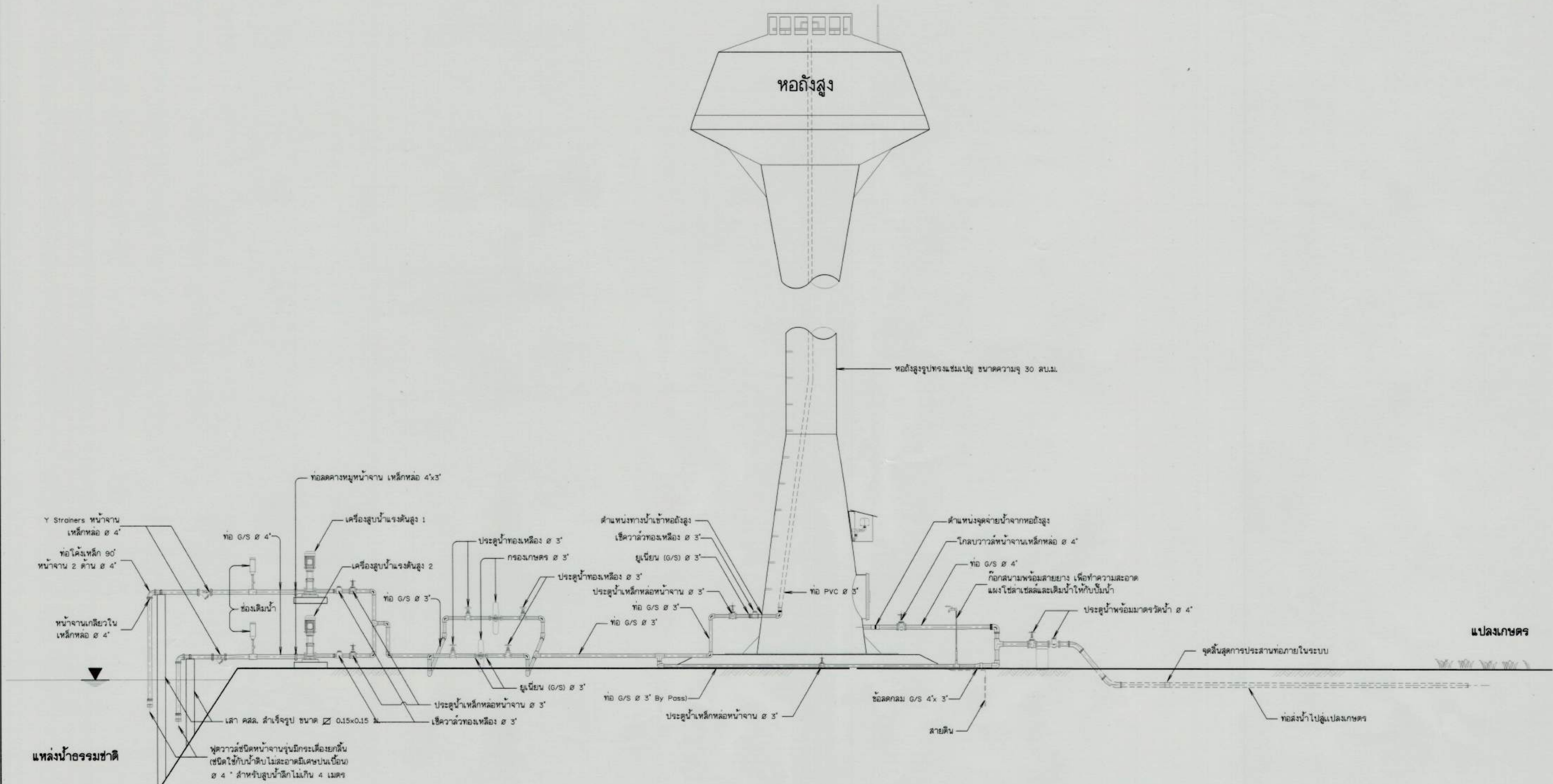
รูปแสดงรายละเอียดท่อและอุปกรณ์ระบบส่งน้ำพลังงานแสงอาทิตย์ ไม่แสดงมาตราส่วน
