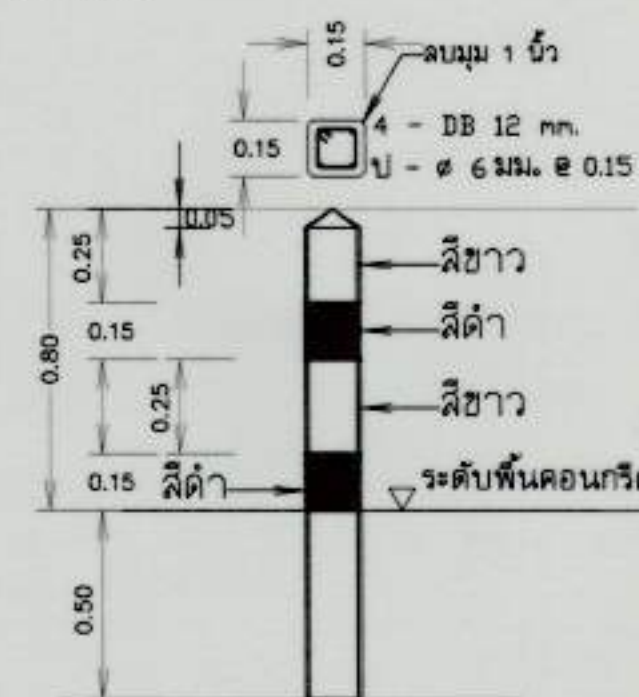
แบบขยายหลักบอกแนว
