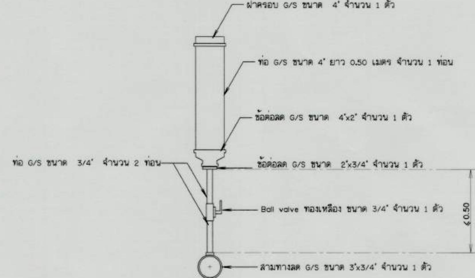
11. ชื่องัดน้ำ ไม่แสดงมาตราส่วน
