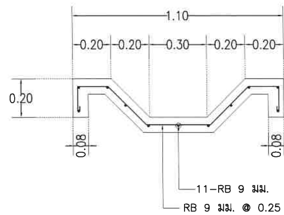
รูปตัดรางระบายน้ำ มาตราส่วน 1:20
