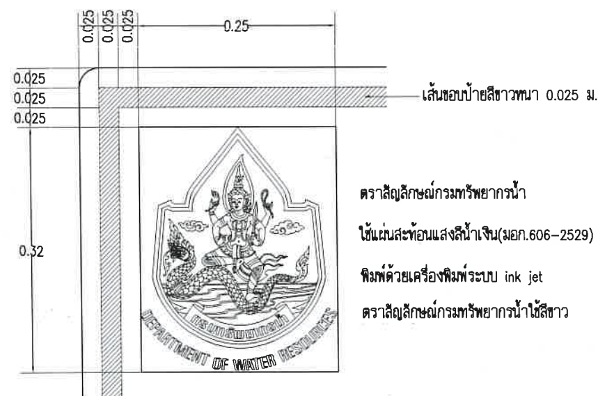
ขยายสัญลักษณ์กรมทรัพยากรน้ำ
