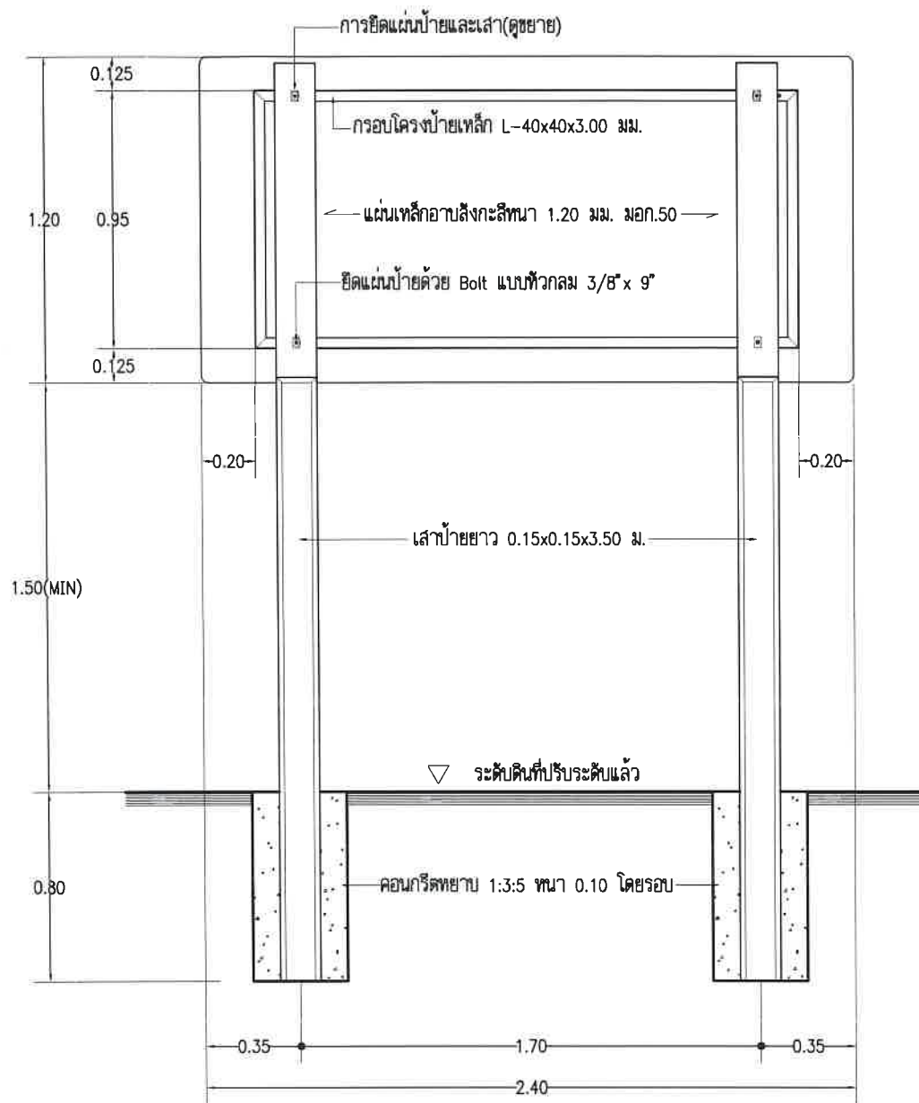
แสดงรูปด้านหลังป้ายโครงการ
