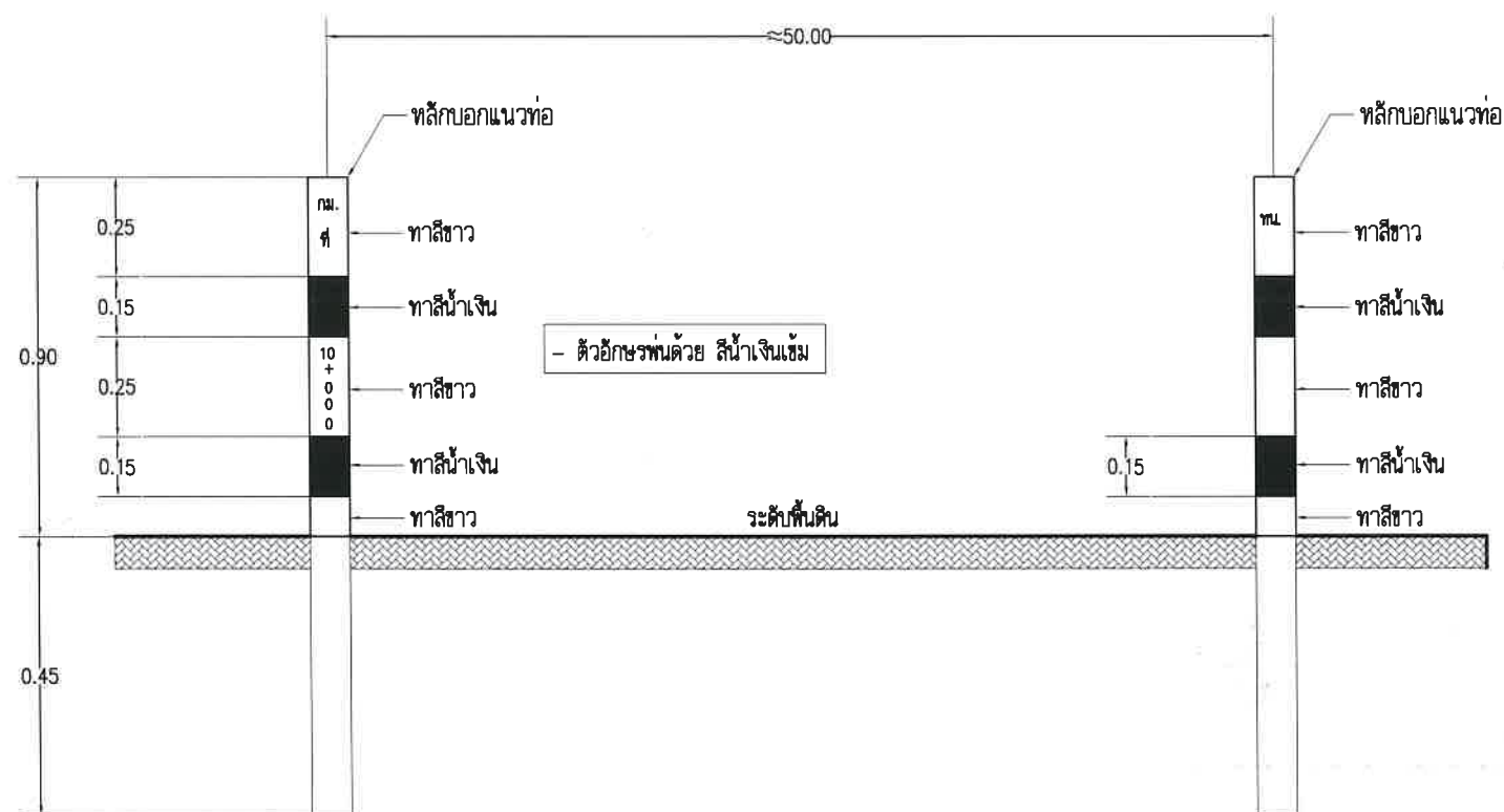
แสดงระยะบ่อแกวท่อ
