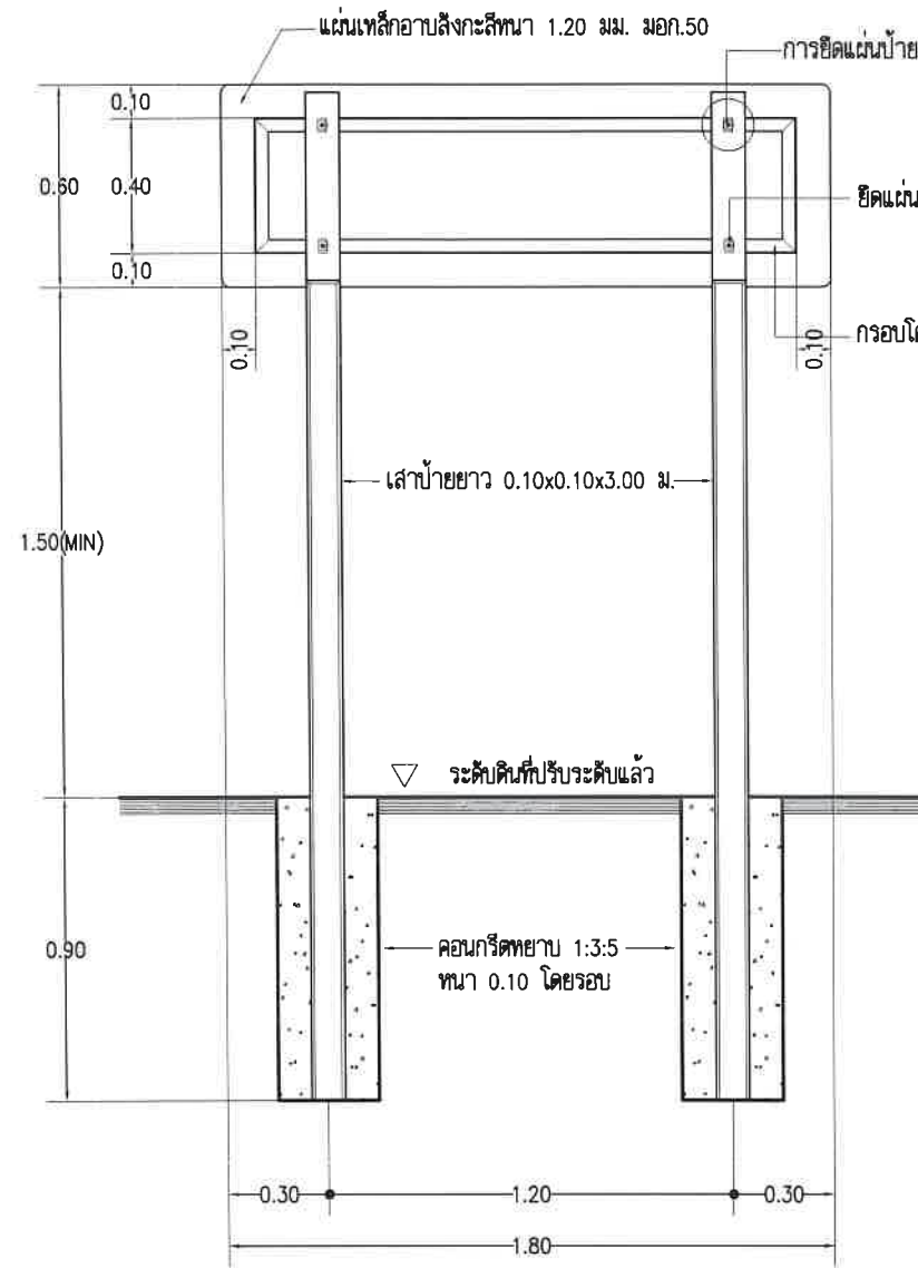
แสดงรูปด้านหลังแนะนำโครงการ SCALE 1:25
