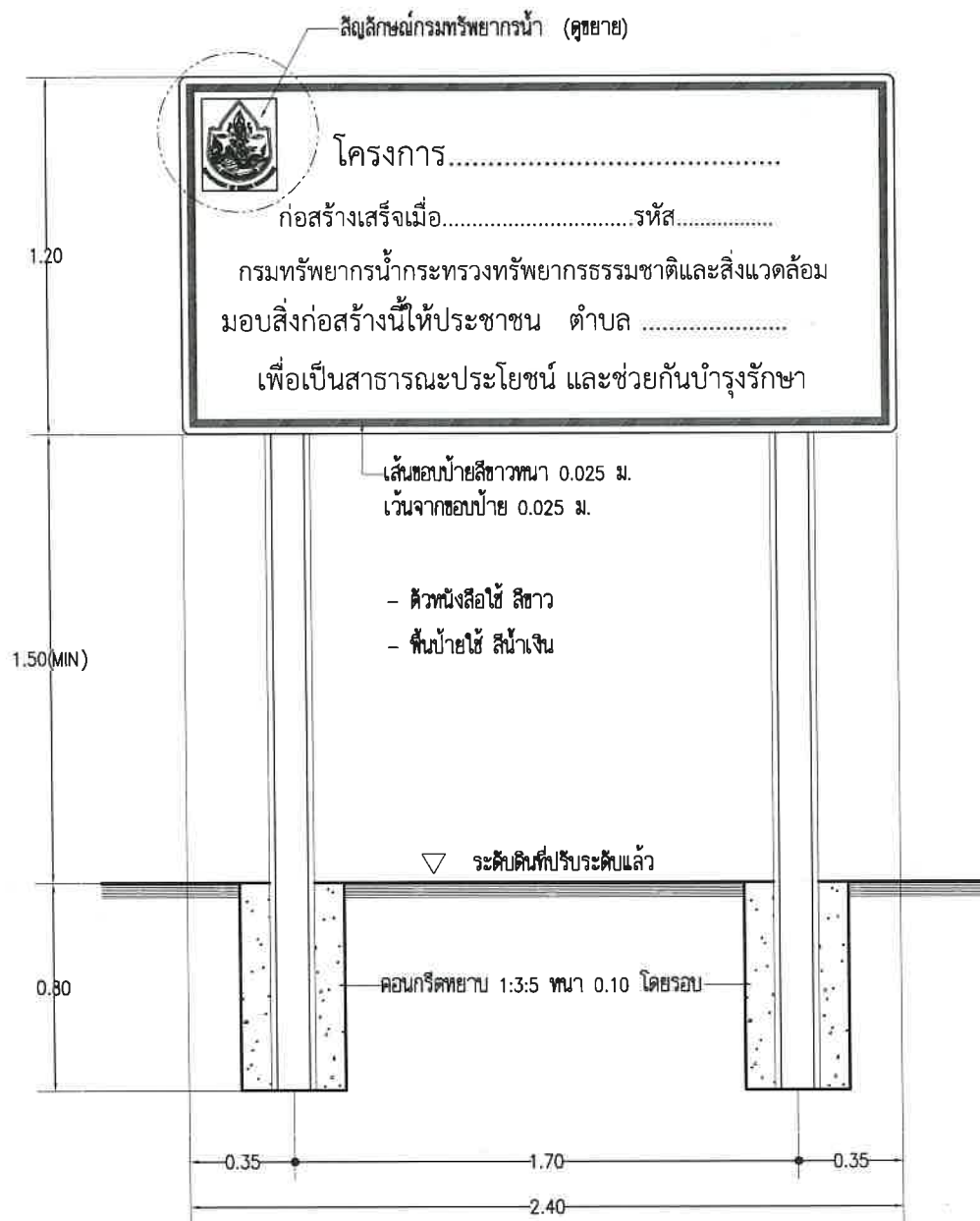
แสดงรูปด้านหน้าป้ายโครงการ
