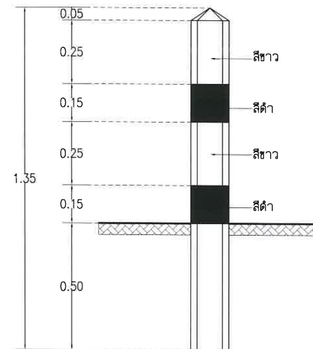
แบบขยายหลักบ่อแนว มาตราส่วน 1:15
