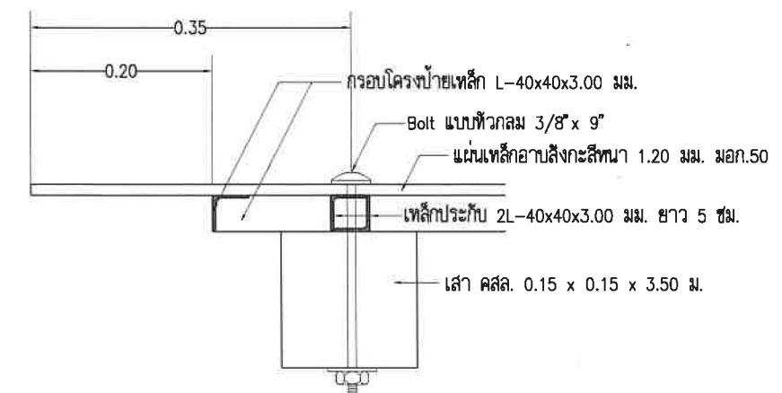
ขยายการยึดแผ่นป้ายและเสา
