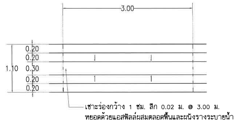
แปลนรางระบายน้ำ มาตราส่วน 1:50
