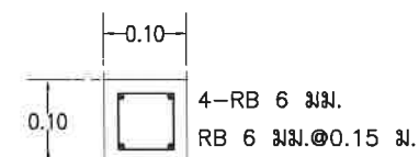
แบบขยายเหล็กเสริมหลักบ่อแกวท่อ มาตราส่วน 1:15
