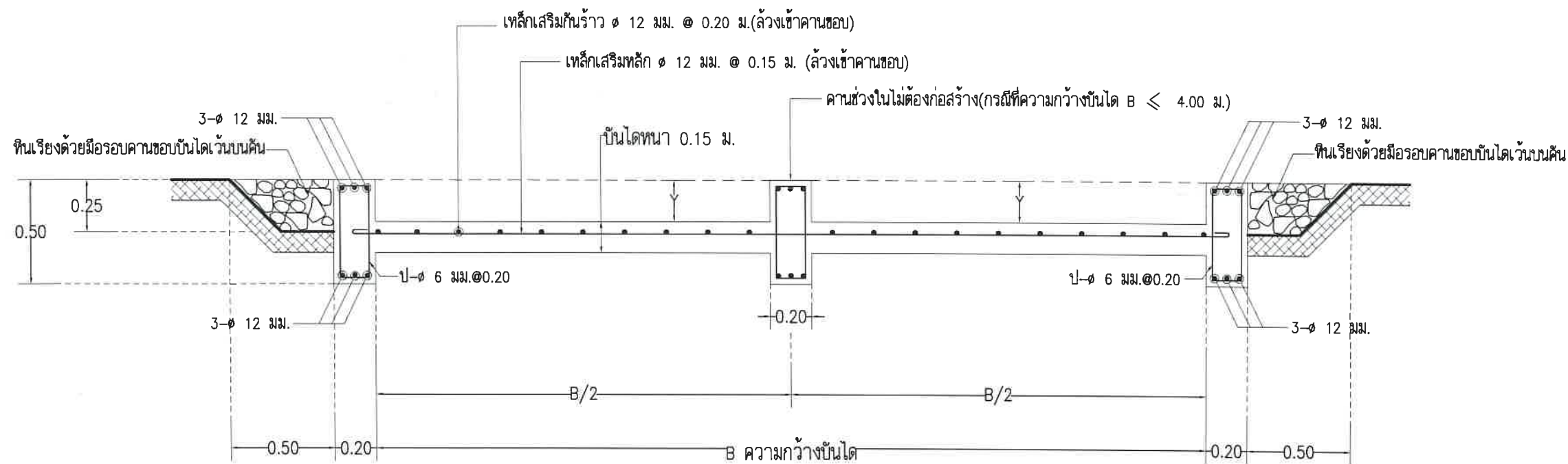
รูปตัดบันได ก - ก มาตราส่วน 1:20
