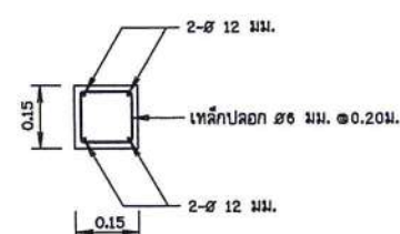
รูปตัด ก - ก ๙๙๙๙๙๙๙ 1:10
