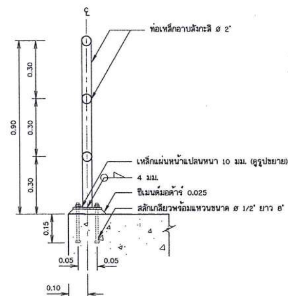
รูปตัด G-G มาตราส่วน 1:10
