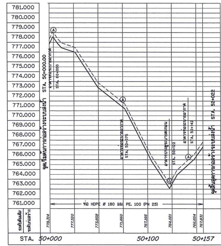
รูปตัดตามแนวยาว STA. 50+000 - 50+157
