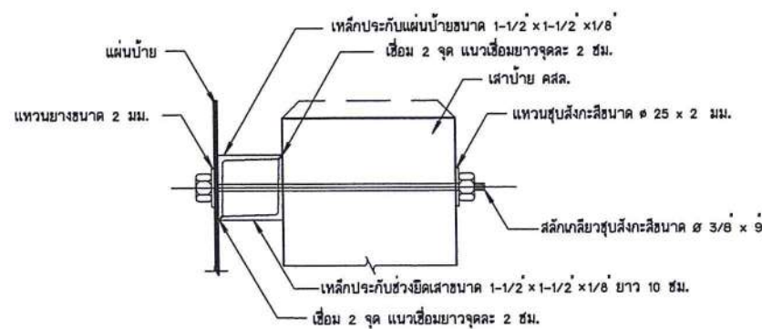
รูปตัดขยายการยึดแผ่นป้ายและเสา ๙๙๙๙๙๙๙ 1:20
