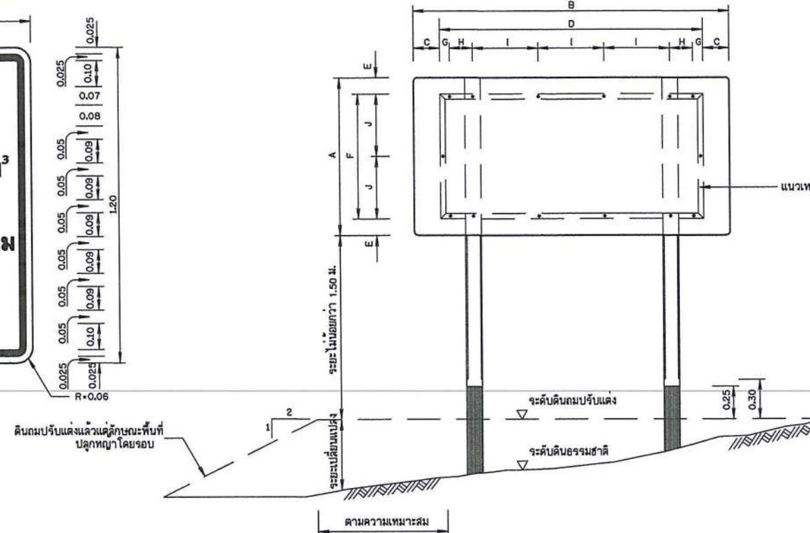
รูปแสดงการประกอบแผ่นป้าย ๙๙๙๙๙๙๙ 1:20
