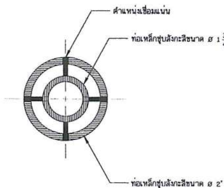
รูปตัด Y-Y มาตราส่วน 1:2.5
