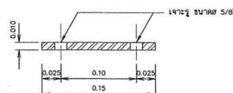
รูปตัด C-C มาตราส่วน 1:10
