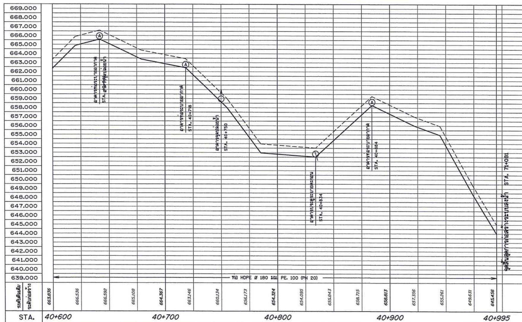
รูปตัดตามแนวยาว STA. 40+600 - 40+995
