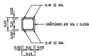
รูปตัด ข - ข ๙๙๙๙๙๙๙ 1:10
