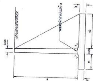
รูปตัด ก-ก ไม่แสดงขนาดจำนวน
