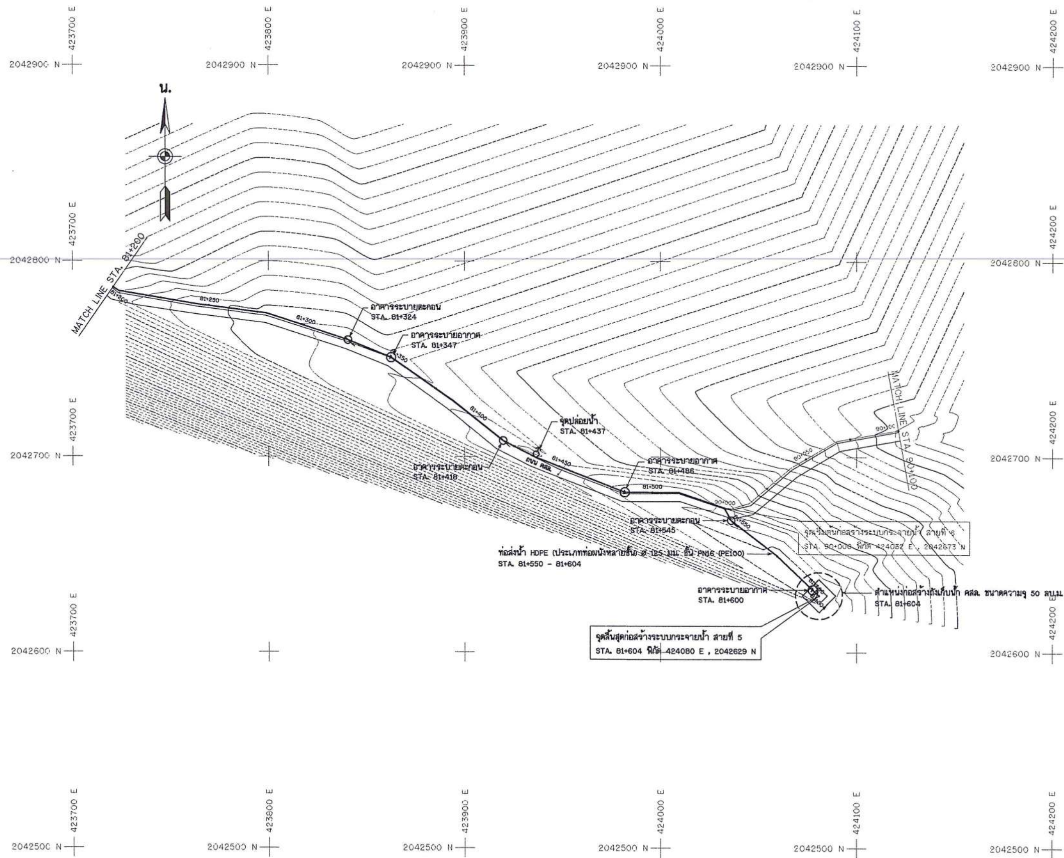
แปลนทั่วไประบบกระจายน้ำ สายที่ 5 มาตราส่วน 1:1,000
