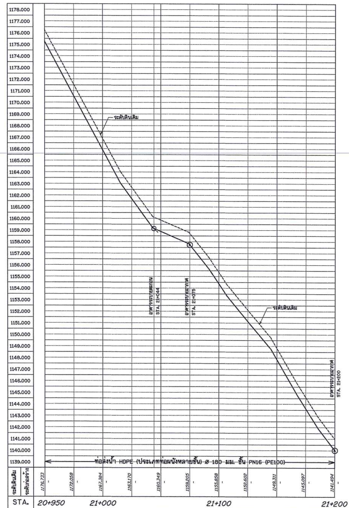
รูปตัดตามแนวยาวระบบกระจายน้ำ สายที่ 1
