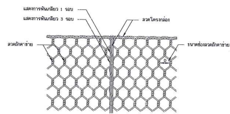
รูปแสดงการพันลวดระหว่างกล่องลวดตาข่ายและฟาด
