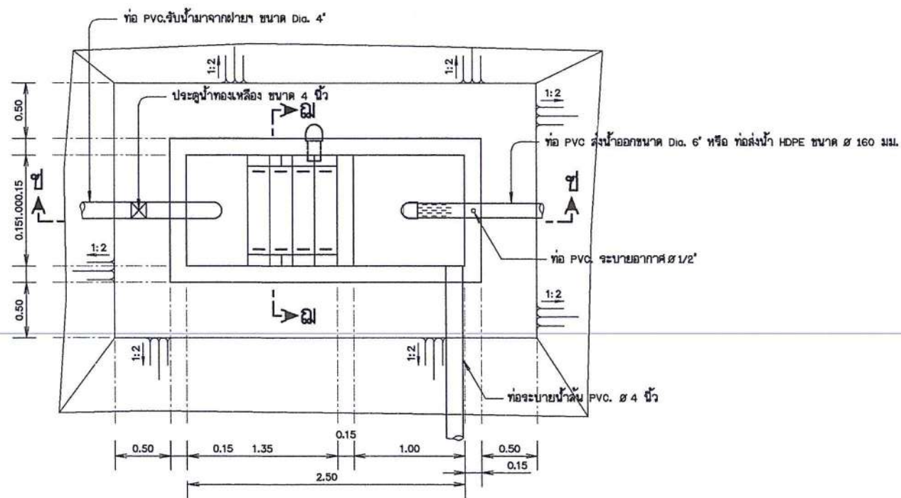
แปลนบ่อตกตะกอน
