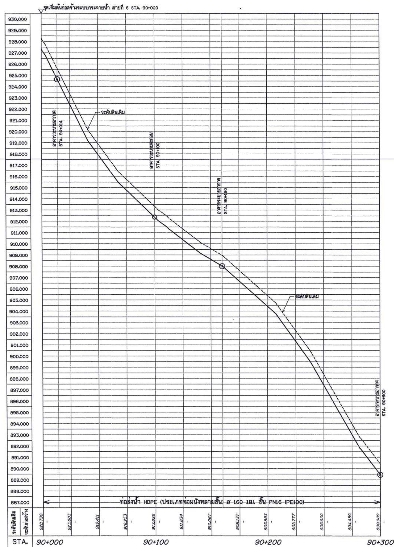
รูปตัดตามแนวยาวระบบกระจายน้ำ สายที่ 6 มาตรฐาน แนวนอน 1:1,000 แนวตั้ง 1:100
