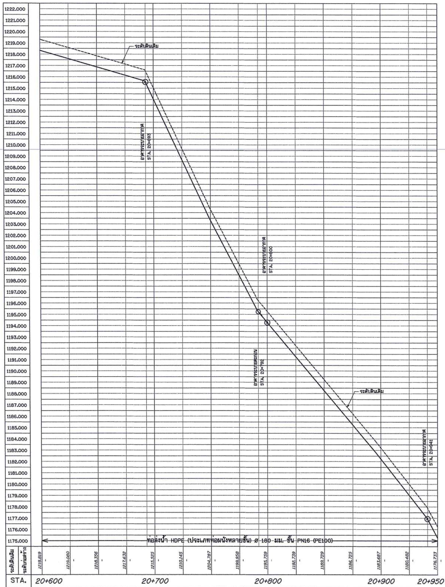
รูปตัดตามแนวยาวระบบกระจายน้ำ สายที่ 1
