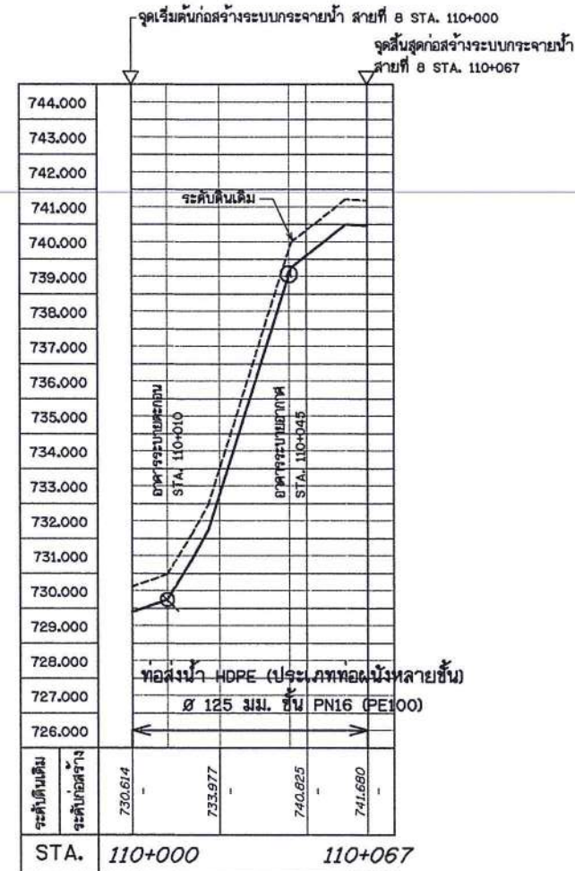
รูปตัดตามแนวยาวระบบกระจายน้ำ สายที่ 8
