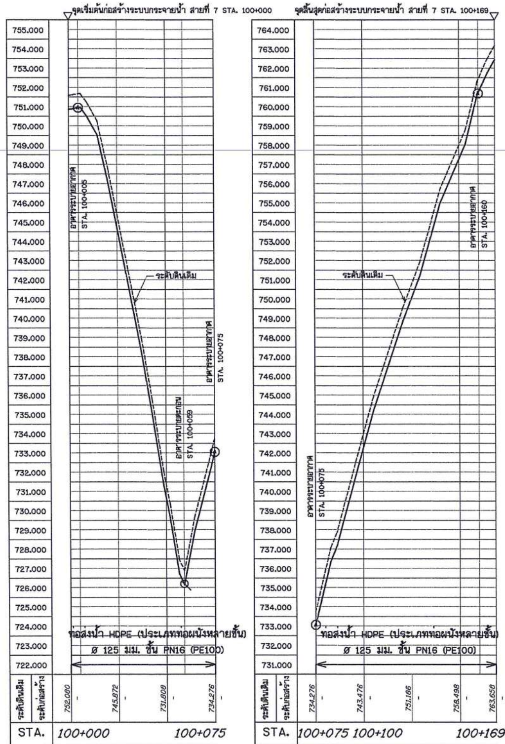
รูปตัดตามแนวยาวระบบกระจายน้ำ สายที่ 7
