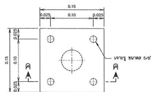
รูปขยายแผ่นเหล็กหนาแปลง มาตราส่วน 1:10
