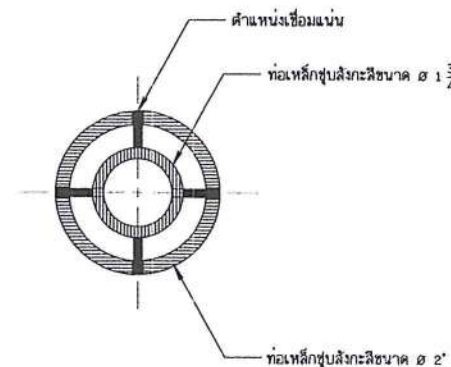
รูปตัด X-X มาตราส่วน 1:2.5
