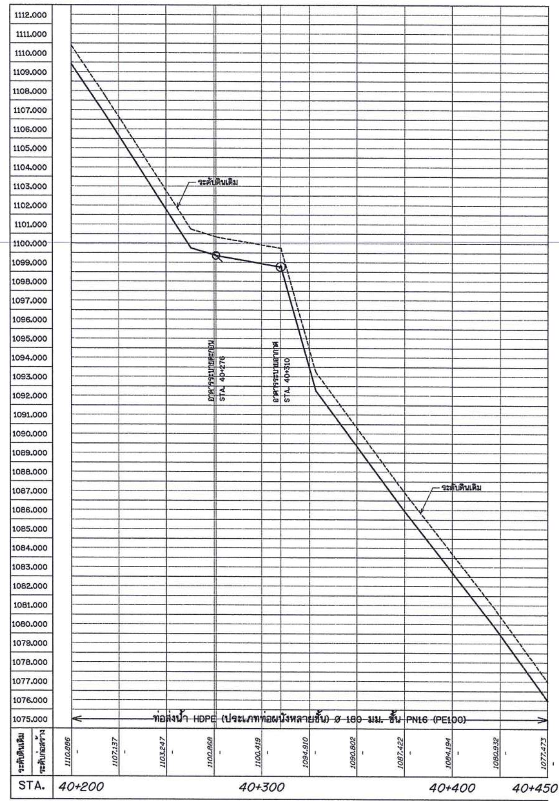
รูปตัดตามแนวยาวระบบกระจายน้ำ สายที่ 3 มาตรฐาน มาตรฐาน 1:1,000 แนวตั้ง 1:100
