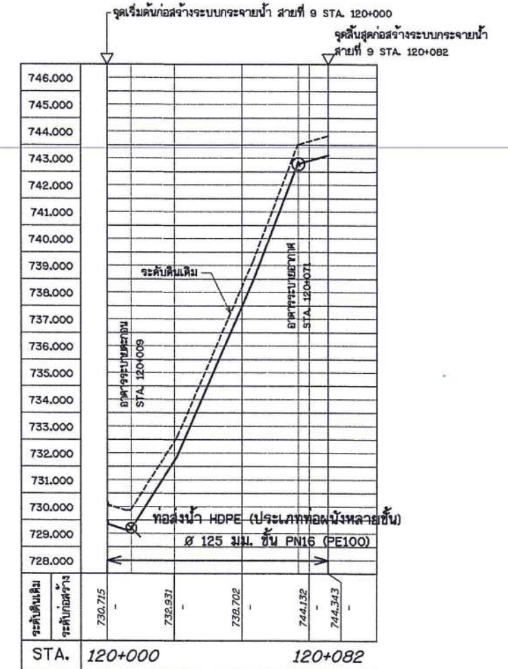
รูปตัดตามแนวยาวระบบกระจายน้ำ สายที่ 9
