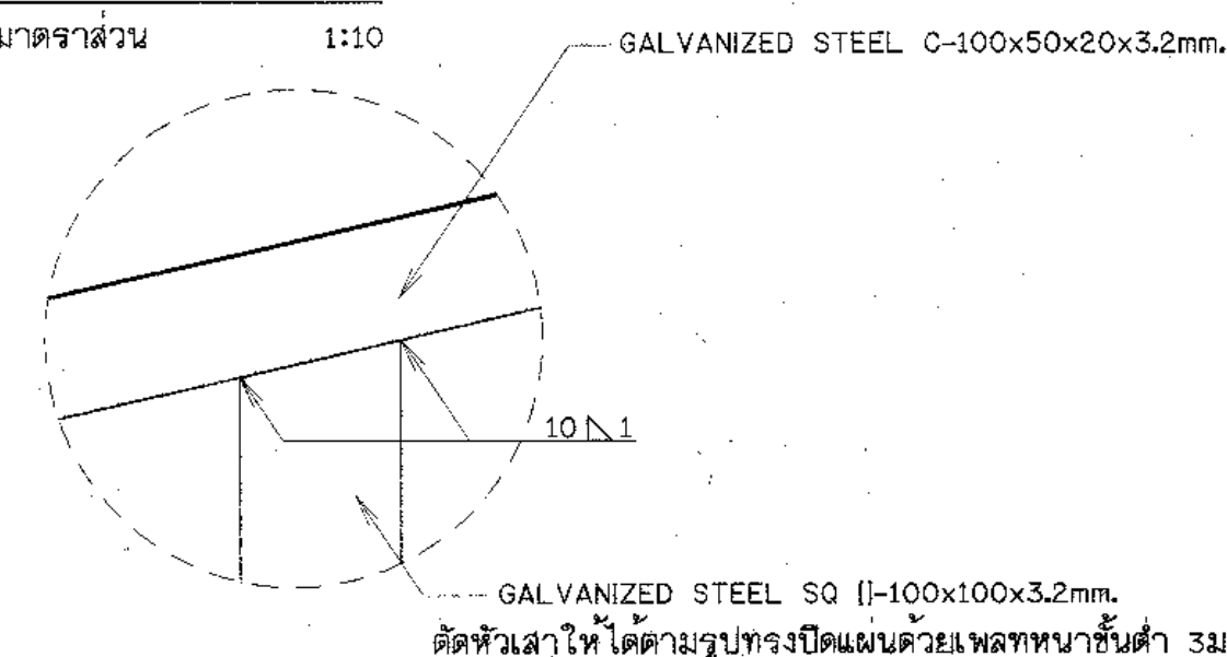
รูปขยาย 2 มาตราส่วน 1:10
