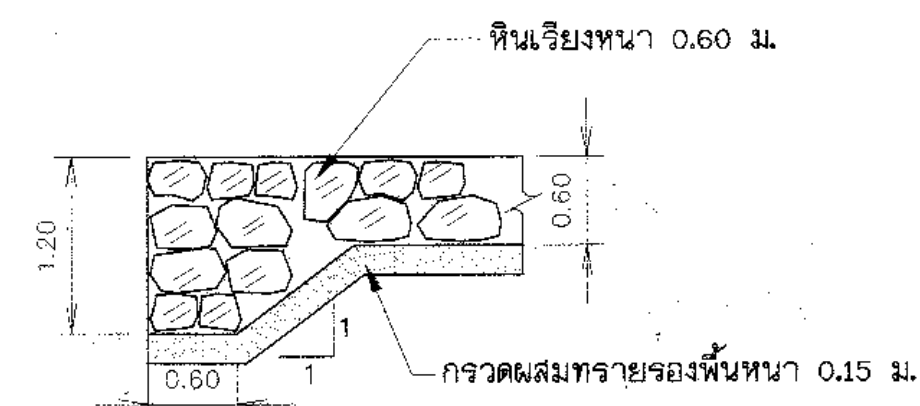
รูปตัด ค1 - ค1 ไม่แสดงมาตราส่วน
