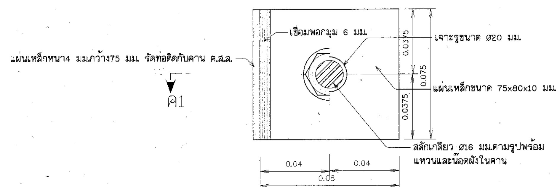
รูปตัด ฉ1 - ฉ1 ไม่แสดงมาตราส่วน
