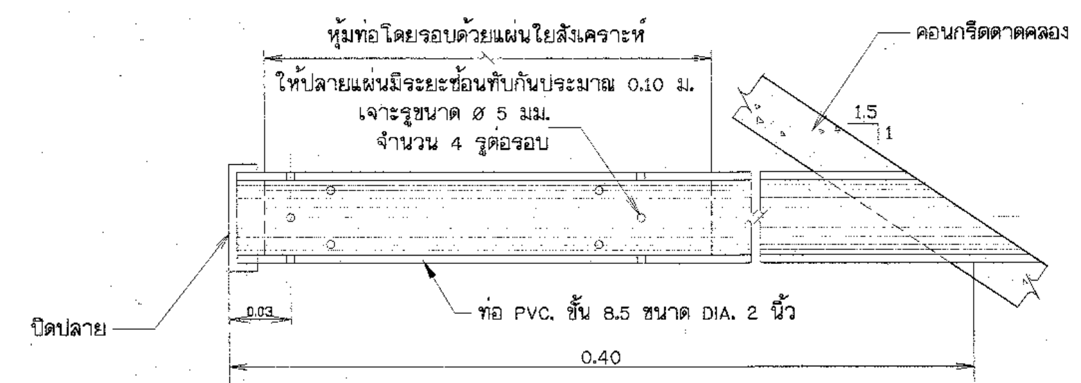
รูปตัด จ1 - จ1 ไม่แสดงมาตราส่วน
