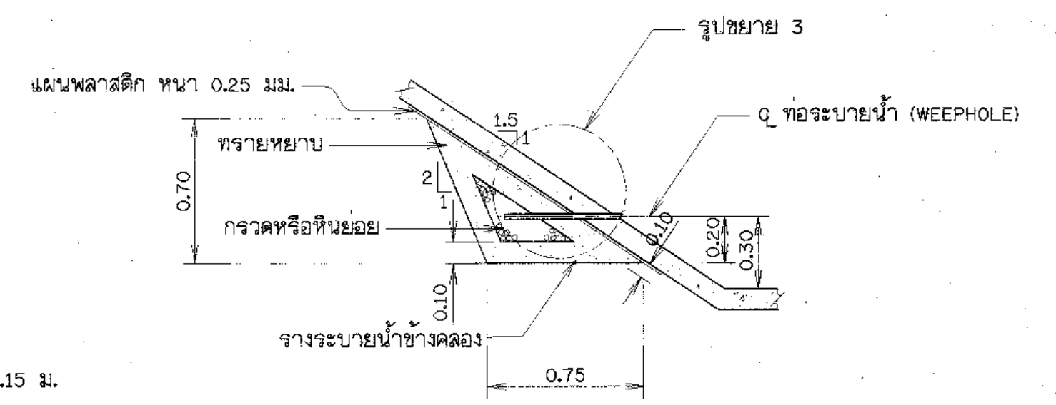
รูปตัด ง1 - ง1 ไม่แสดงมาตราส่วน
