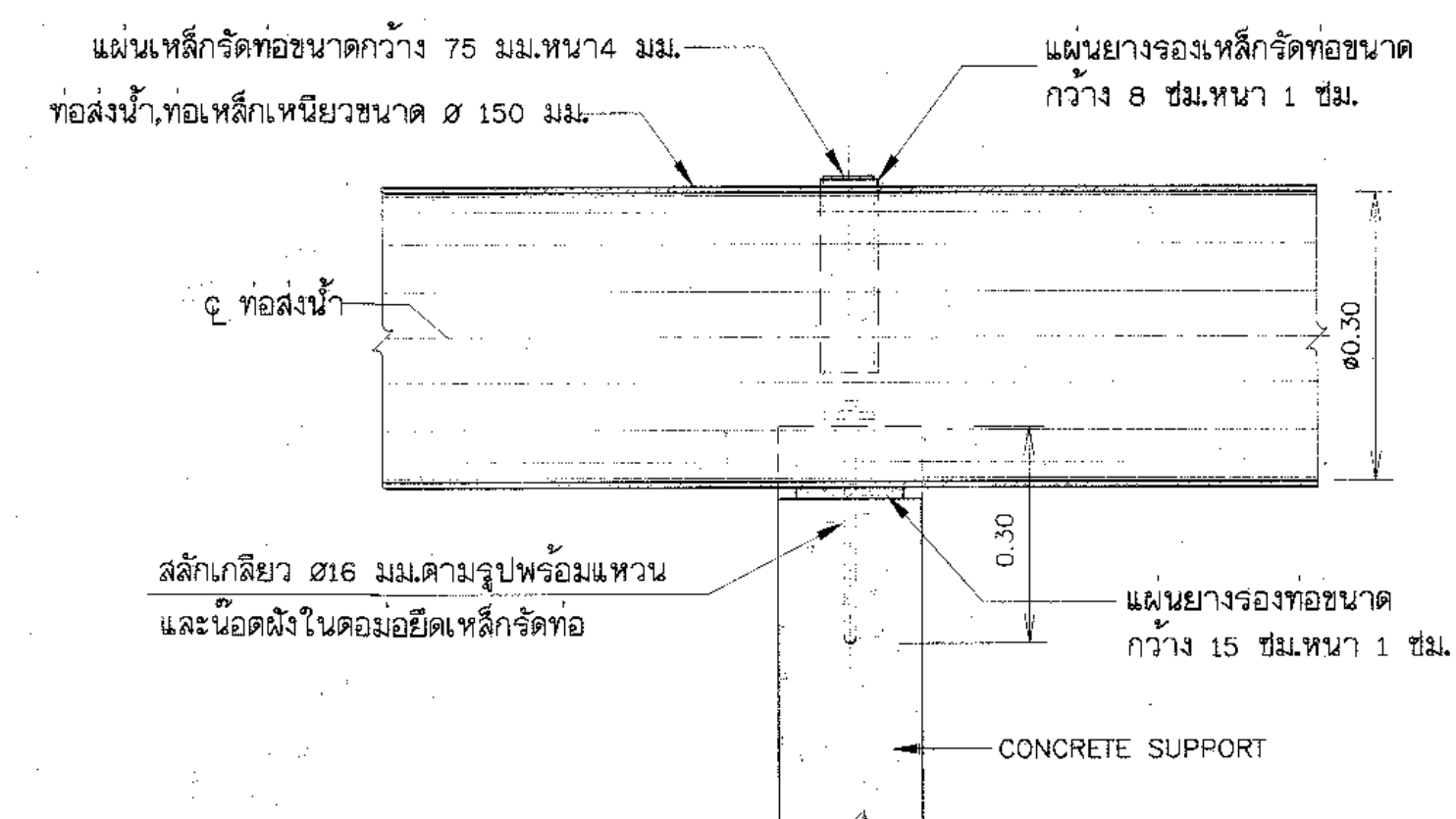
รูปตัด ก1 - ก1 ไม่แสดงมาตราส่วน
