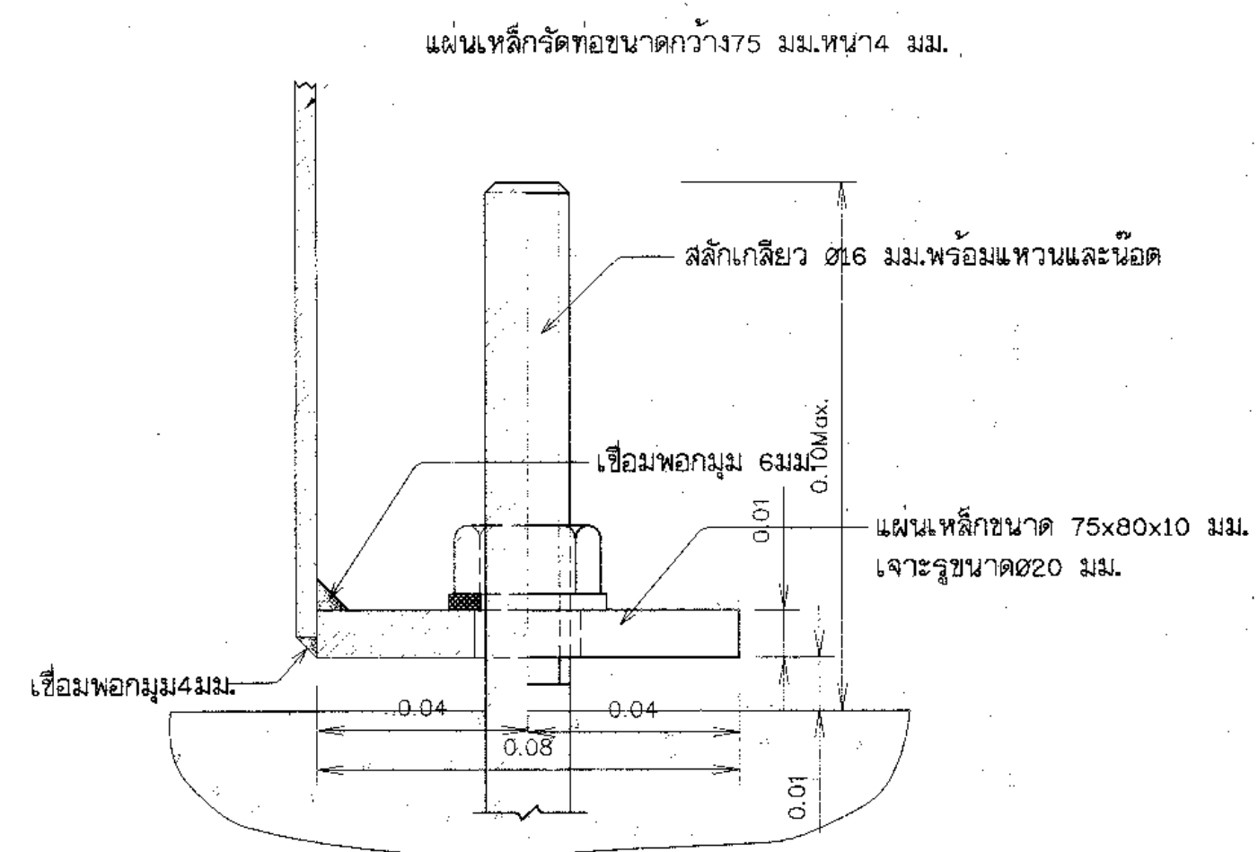
รูปตัด ซ1 - ซ1 ไม่แสดงมาตราส่วน
