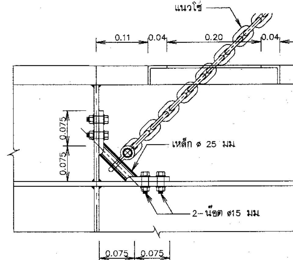
รูปขยาย ตำแหน่งจุดยึดรอกโซ่กับบานระบาย
