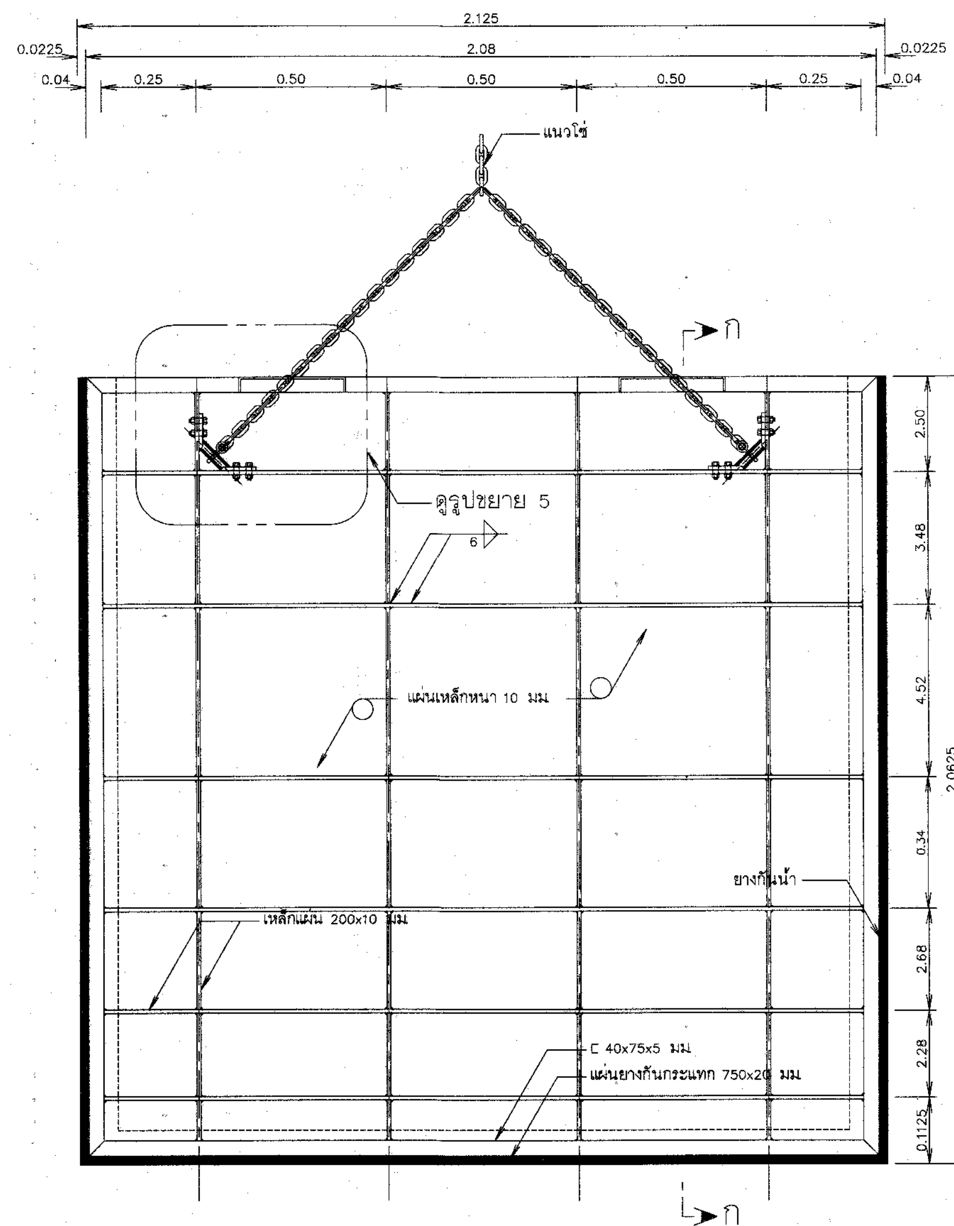
รูปด้านหลังบานประตูปรับสาย
