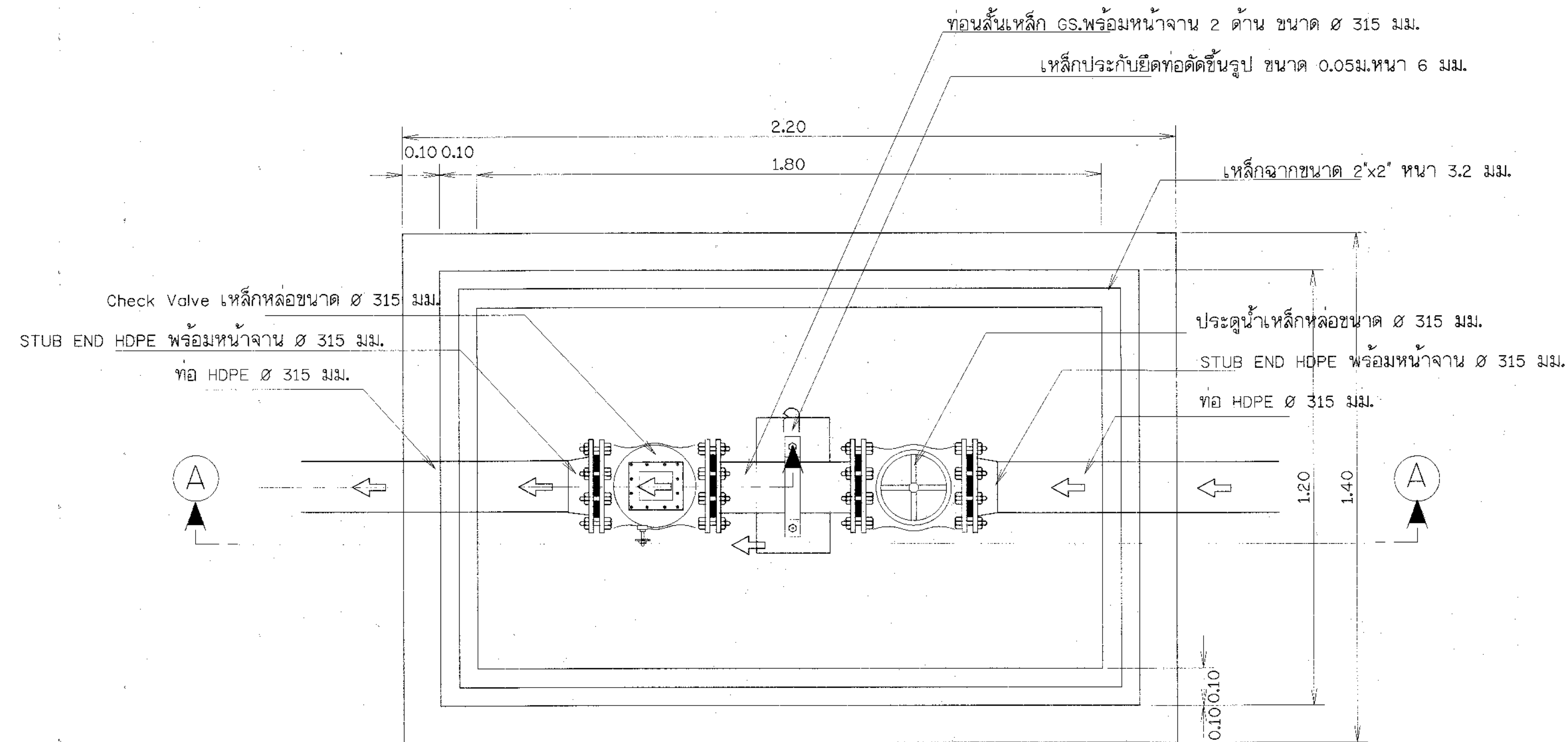
แปลนจุดประตุน้ำคุมท่อจ่ายน้ำ ขนาด 315 มม.
