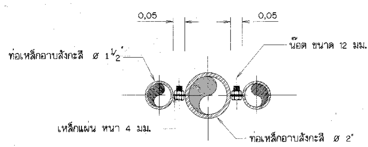
ข้อตัด ก-ก มาตราส่วน 1:10
