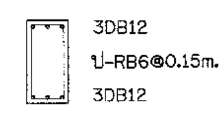
คาน Bx (0.20x0.40 m.) มาตราส่วน 1:25
