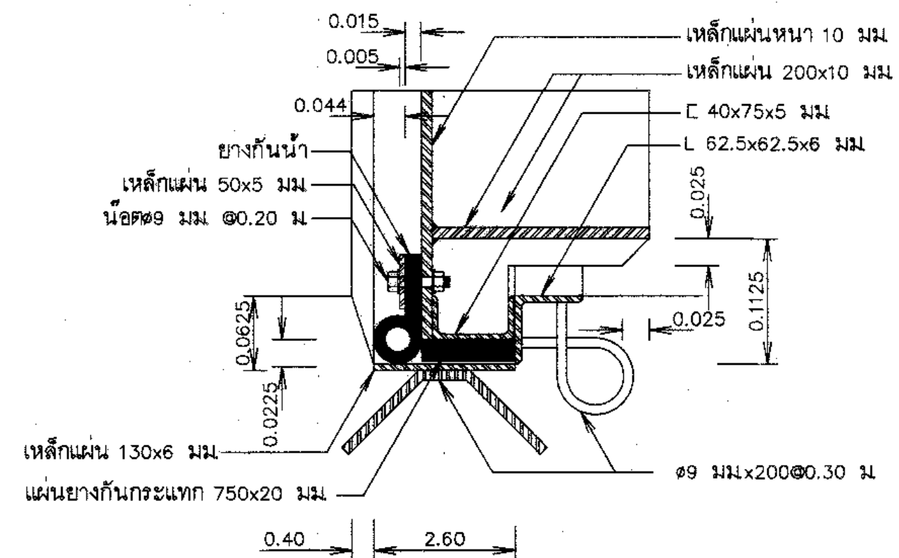
รูปขยายบานระบายด้านติดพื้น
