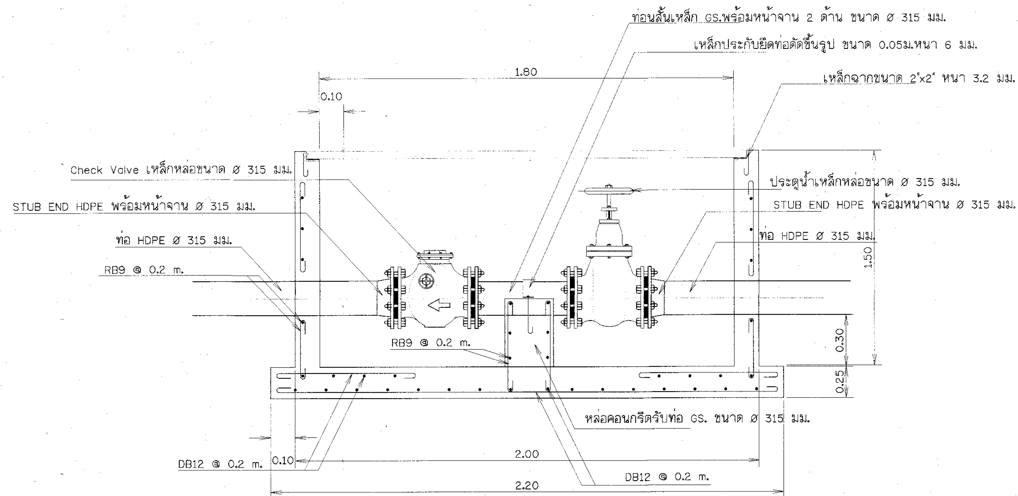
รูปตัด A - A ขยายจุดประตุน้ำคุมท่อจ่ายน้ำ ขนาด 315 มม.
