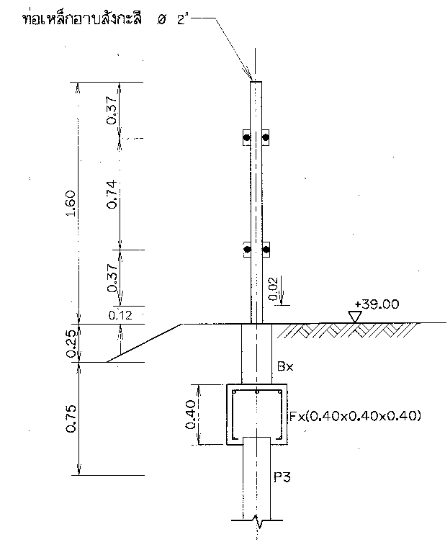
แบบขยายรั้ว (อุปด้านข้าง) มาตราส่วน 1:25
