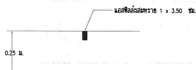
ขยาย Mastic Joint Filler
