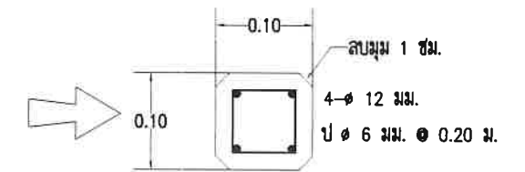
ขยายเสาป้ายฐานเสา - ได้แผ่นป้าย SCALE 1:10
