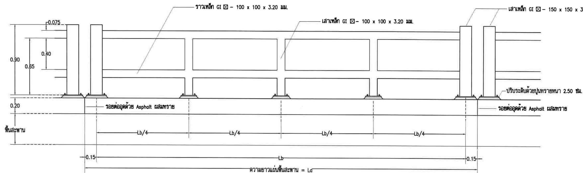
แสดงด้านข้างราวกันตกสะพาน
