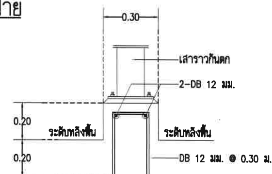
ขยายขอบฐานรับเสาแนวราวกันตก
