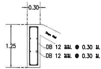
แบบขยาย Cut Off 2 SCALE 1:50
