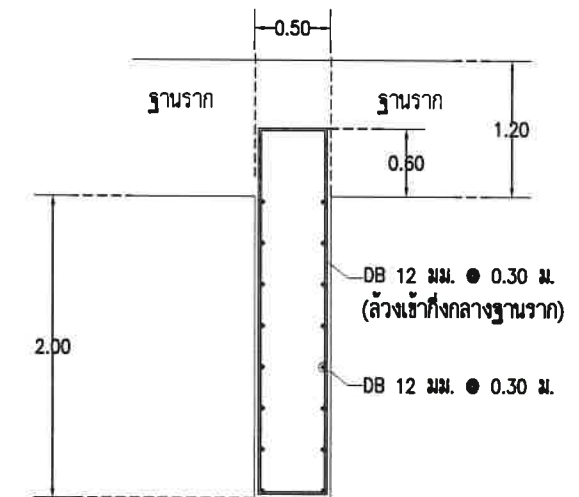
แบบขยาย Cut Off 6 SCALE 1:50
