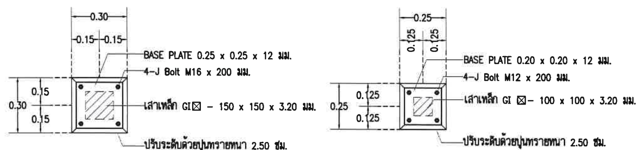
ขยายแปลนการติดตั้งเสาราวกันตก
