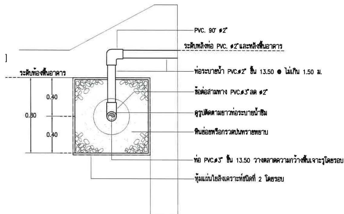
ขยายท่อลดแรงดันน้ำที่พื้นแบบที่ 1 [ท้องพื้นตรง] SCALE 1:25
