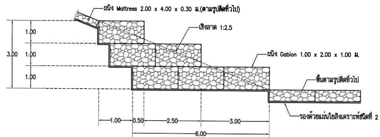
รูปแบบที่ 1 การเรียงหินผนังเชิงลาดส่วนฐาน เชิงลาด 1:2.5 SCALE 1:100
