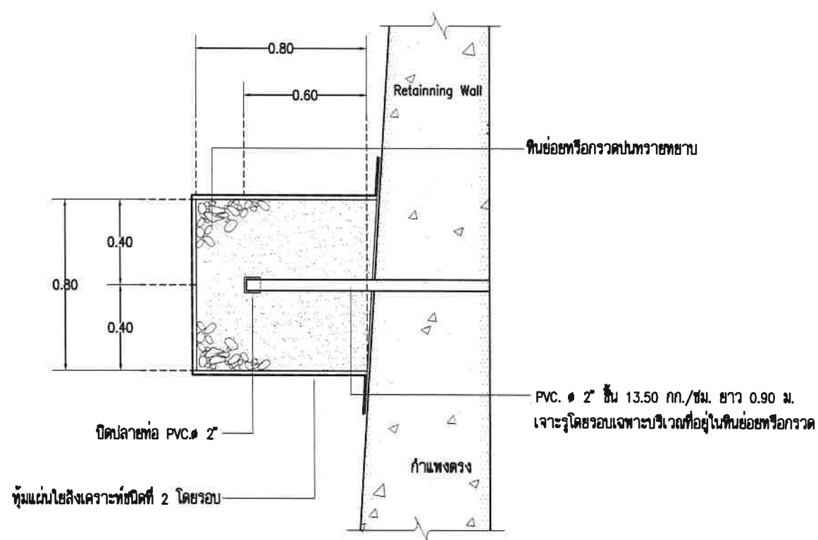
ขยายท่อลดแรงดันด้านข้างกำแพงแบบที่ 1 [กำแพงตรง] SCALE 1:25
