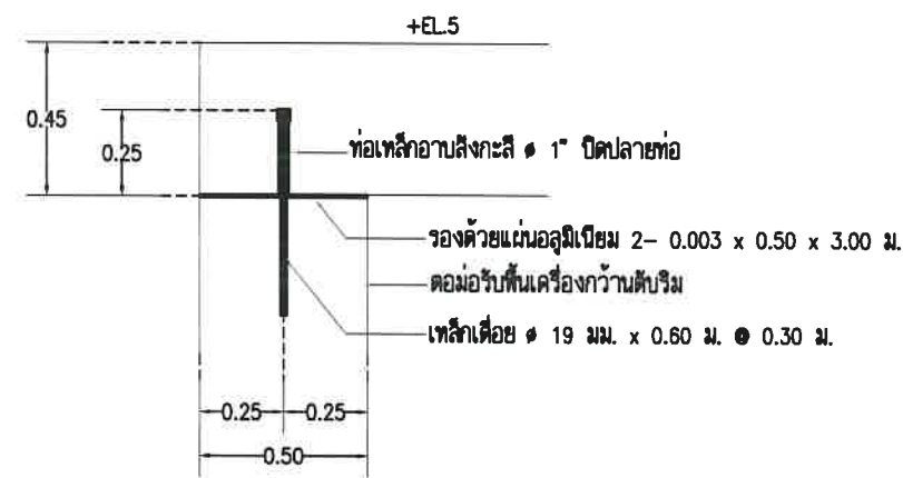
แบบขยาย 1 SCALE 1:25
