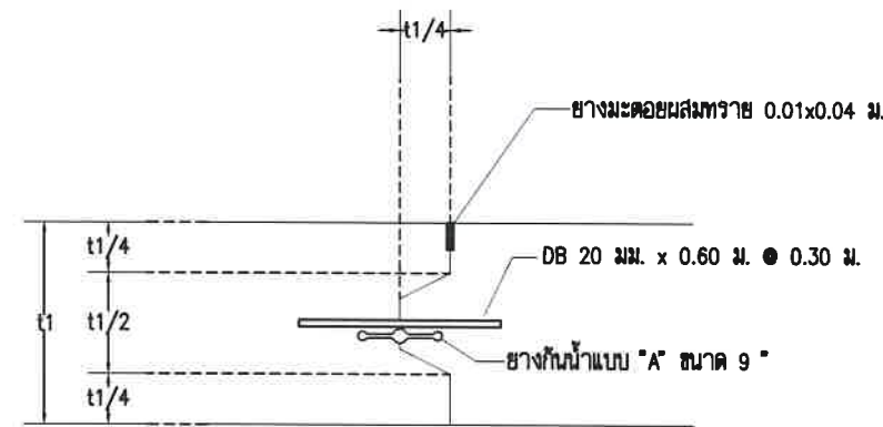
แบบขยายรอยต่อพื้น 2 SCALE 1:25
