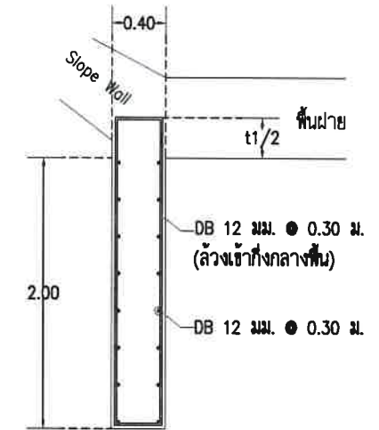
แบบขยาย Cut Off 3 SCALE 1:50
