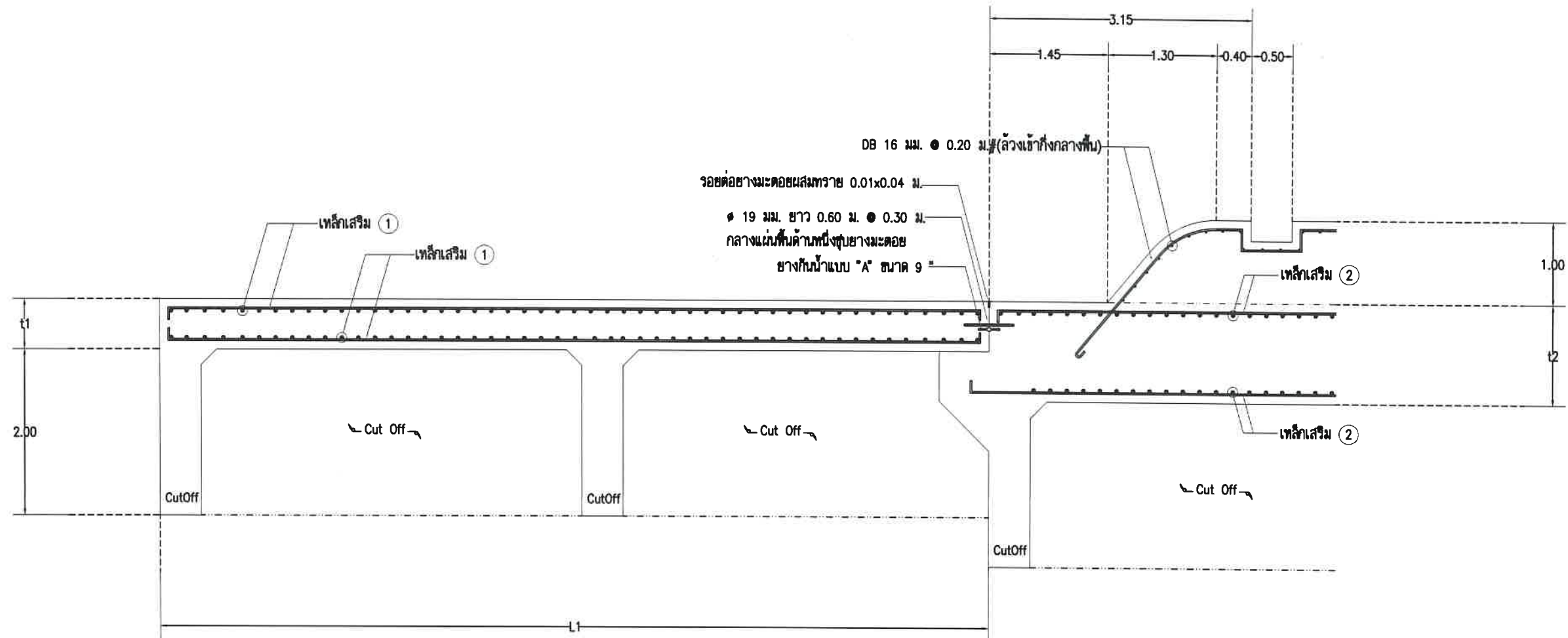
แบบขยาย 1 โครงสร้างพื้นฝาย Section C - C และ Section D - D
