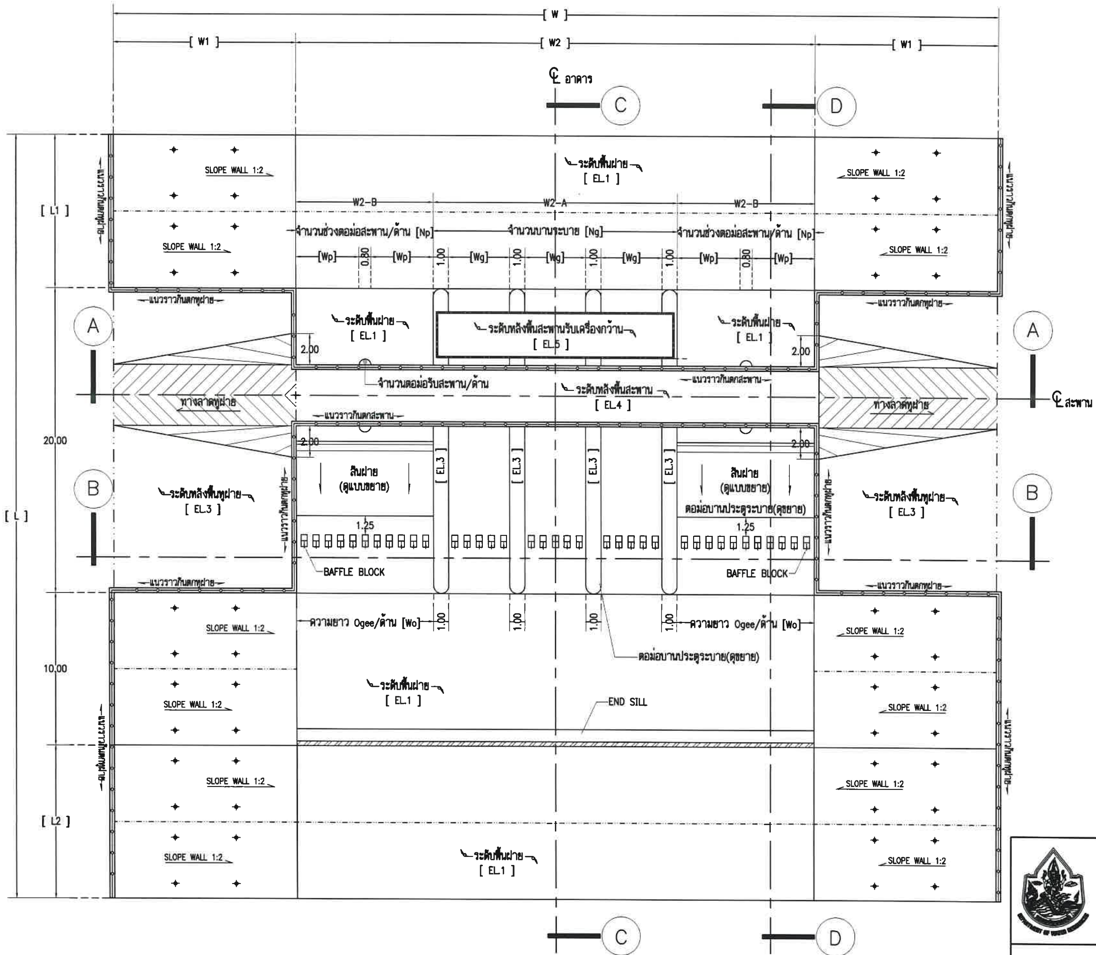
แปลนอาคารระบายน้ำ มาตราส่วน 1:250
