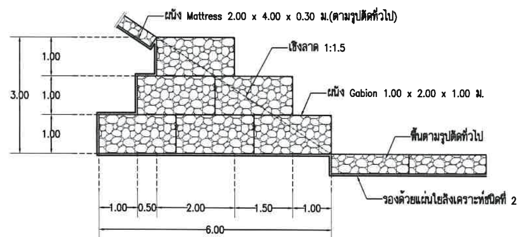
รูปแบบที่ 1 การเรียงหินผนังเชิงลาดส่วนฐาน เชิงลาด 1:1.5 SCALE 1:100
