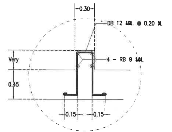
ขยายเหล็กเสริมแทนพื้นรับเครื่องกว้าน SCALE 1:25
