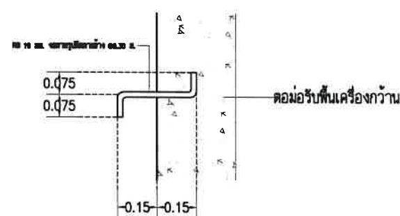
รูปตัดทางข้างบันได
