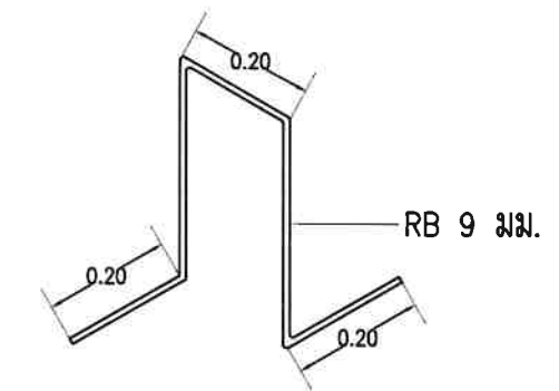
ขยายขาเก้าอี้รับเหล็กเสริม
