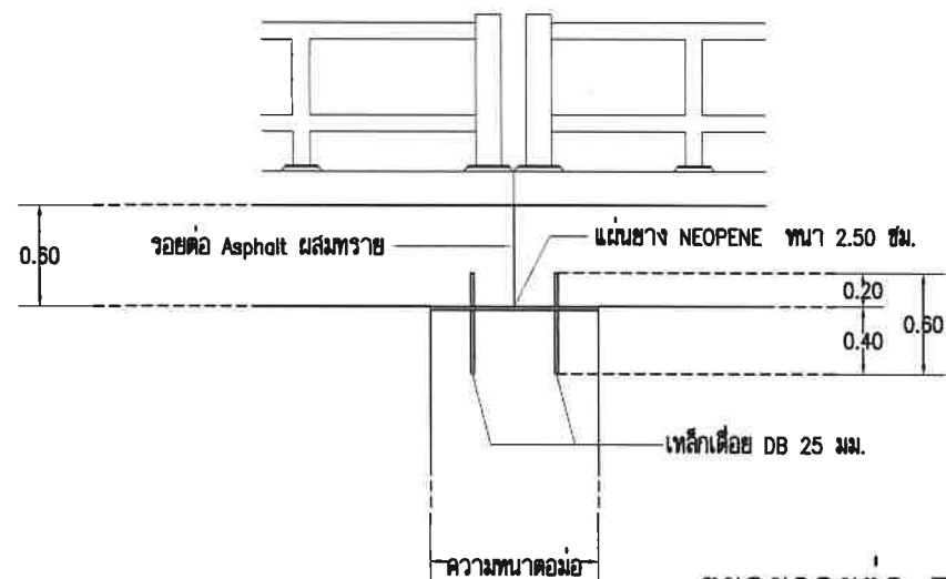
ขยายรอยต่อ FIXED BEARING
