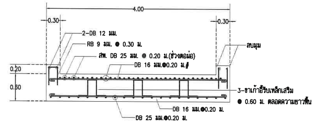
แสดงการเสริมเหล็กพื้นสะพานตามขวาง
