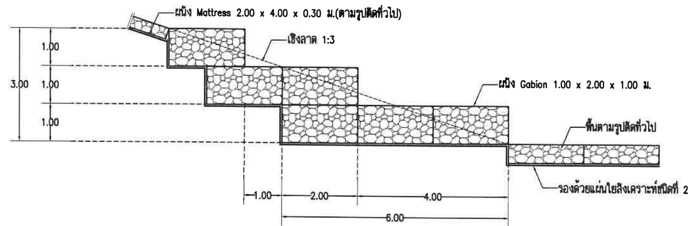
รูปแบบที่ 1 การเรียงหินผนังเชิงลาดส่วนฐาน เชิงลาด 1:3 SCALE 1:100
