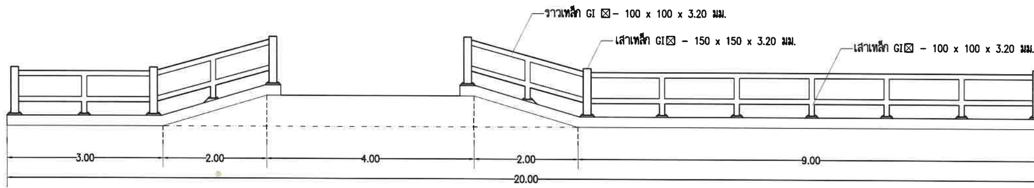
แสดงด้านข้างราวกันตกสะพาน
