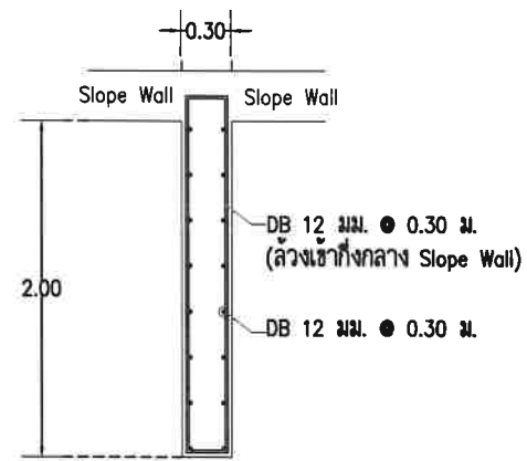
แบบขยาย Cut Off 1 SCALE 1:50
