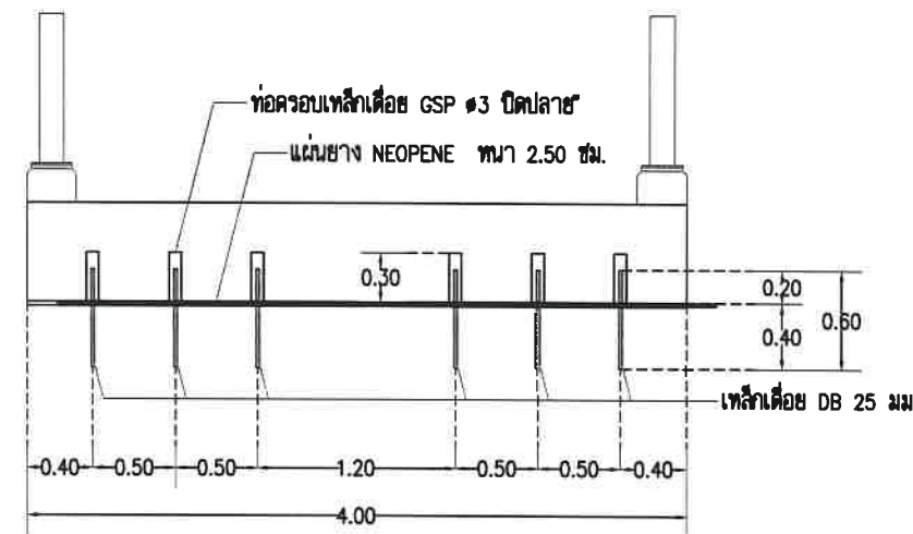
แสดงการเสริมเหล็กพื้นสะพานตามยาว
