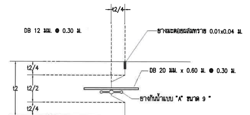
แบบขยายรอยต่อพื้น 3 SCALE 1:50
