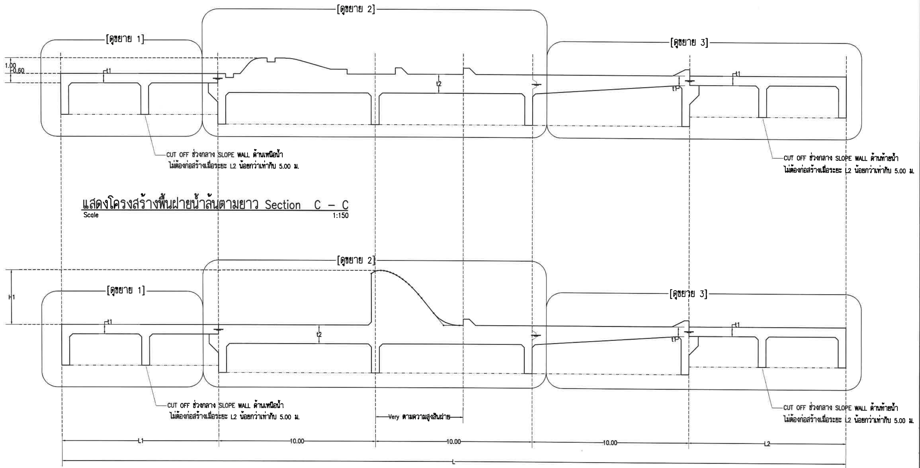
แสดงโครงสร้างพื้นฝายน้ำล้นตามยาว Section D - D Scale 1:150
