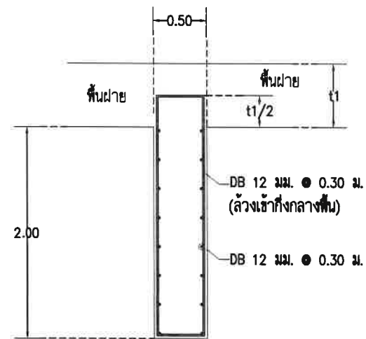
แบบขยาย Cut Off 4 SCALE 1:50
