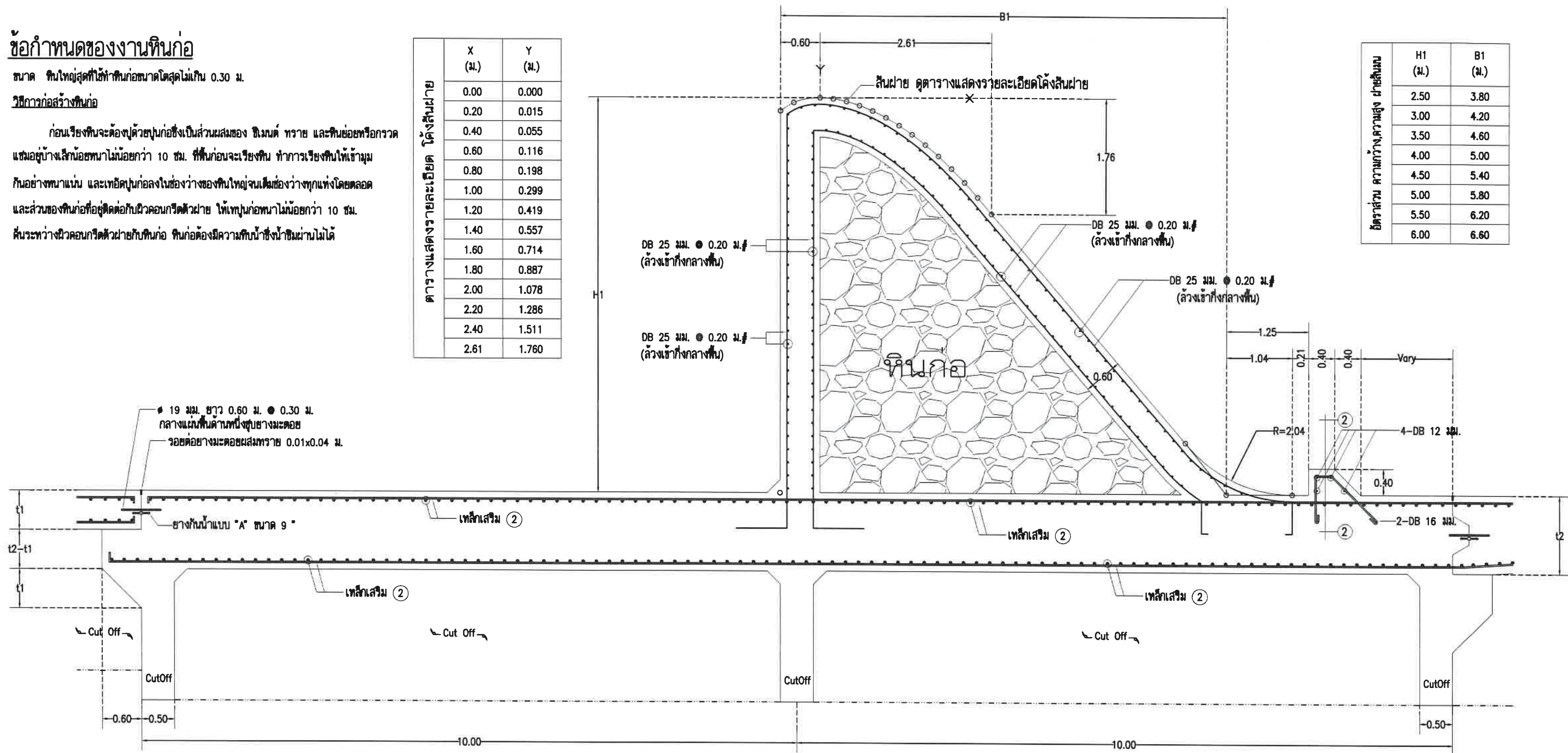
แบบขยาย 2 โครงสร้างพื้นฝ่าย Section D - D
