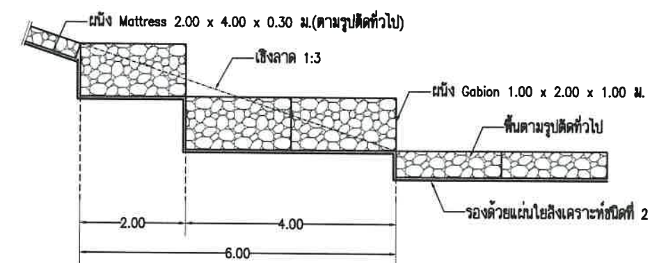
รูปแบบที่ 2 การเรียงหินผนังเชิงลาดส่วนฐาน เชิงลาด 1:3 SCALE 1:100
