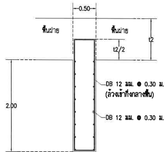
แบบขยาย Cut Off 5 SCALE 1:50
