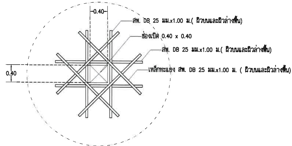
ขยายเหล็กเสริมพิเศษช่องเปิดพื้นรับเครื่องกว้าน SCALE 1:25
