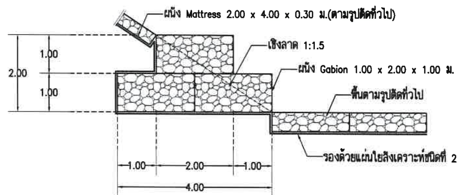
รูปแบบที่ 2 การเรียงหินผนังเชิงลาดส่วนฐาน เชิงลาด 1:1.5 SCALE 1:100
