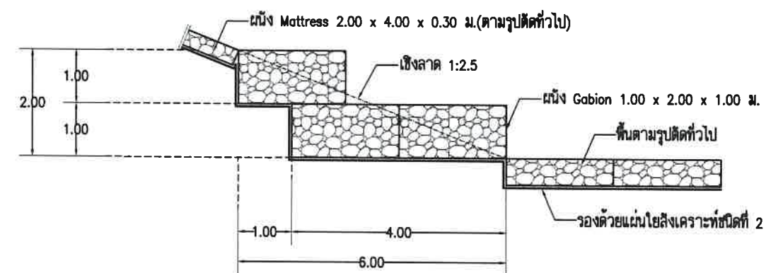
รูปแบบที่ 2 การเรียงหินผนังเชิงลาดส่วนฐาน เชิงลาด 1:2.5 SCALE 1:100
