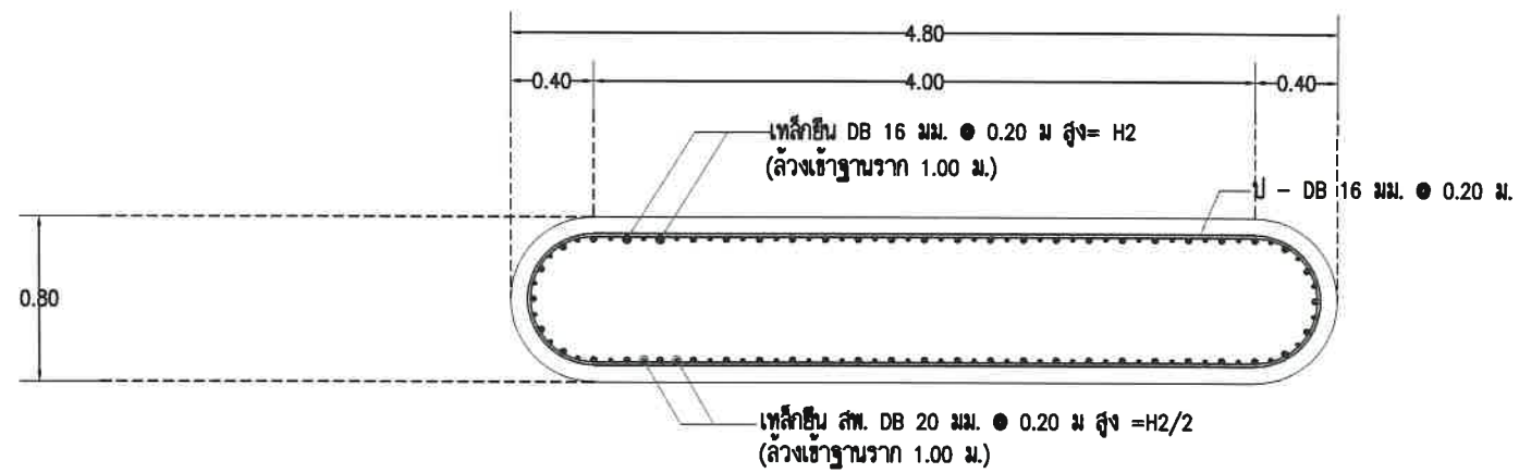
แปลนแสดงเหล็กเสริม ตอม่อรับพื้นสะพาน SCALE 1:50
