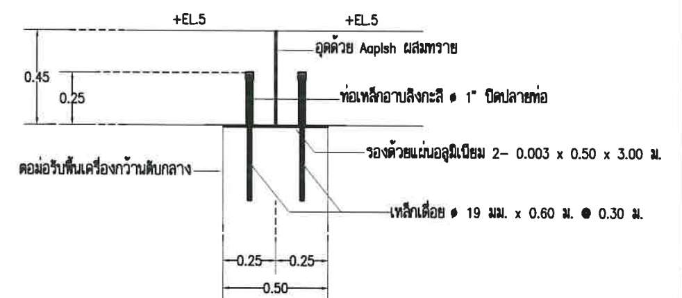
แบบขยาย 2 SCALE 1:25
