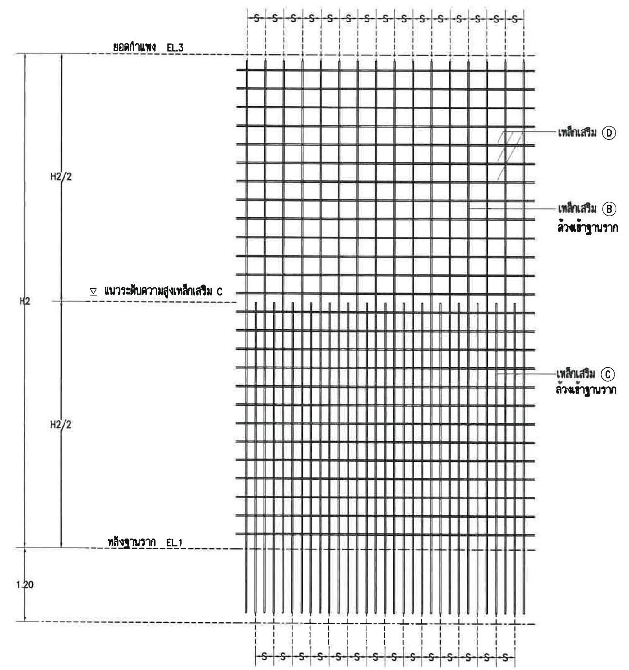
ขยายเหล็กเสริม Retaining Wall SCALE 1:60
