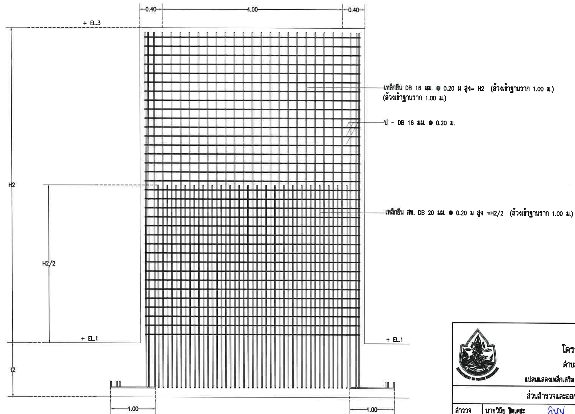
แสดงเหล็กเสริมทางช้างตอม่อรับพื้นสะพาน SCALE 1:50
