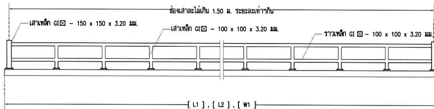
แสดงด้านข้างราวกันตกห้วย
