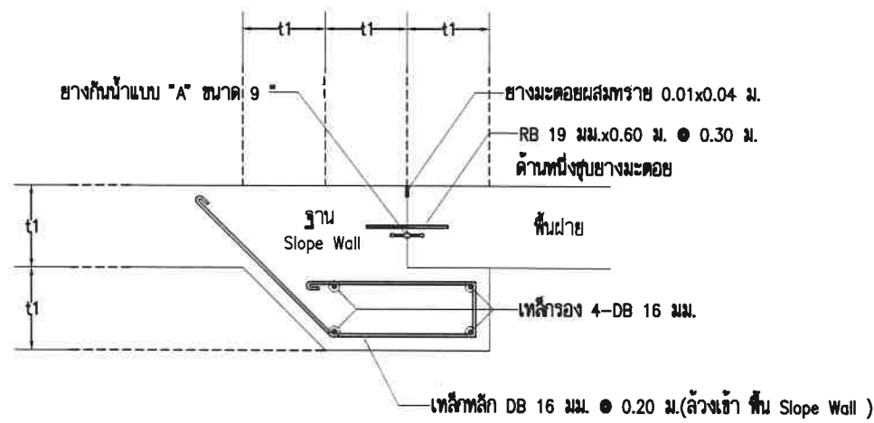
แบบขยายรอยต่อพื้น 1 SCALE 1:50
