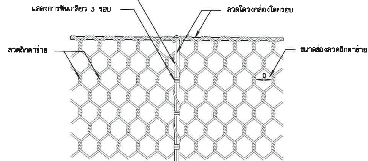
รูปแสดงการพันลวดระหว่างกล่องลวดตาข่ายและฝาปิด
