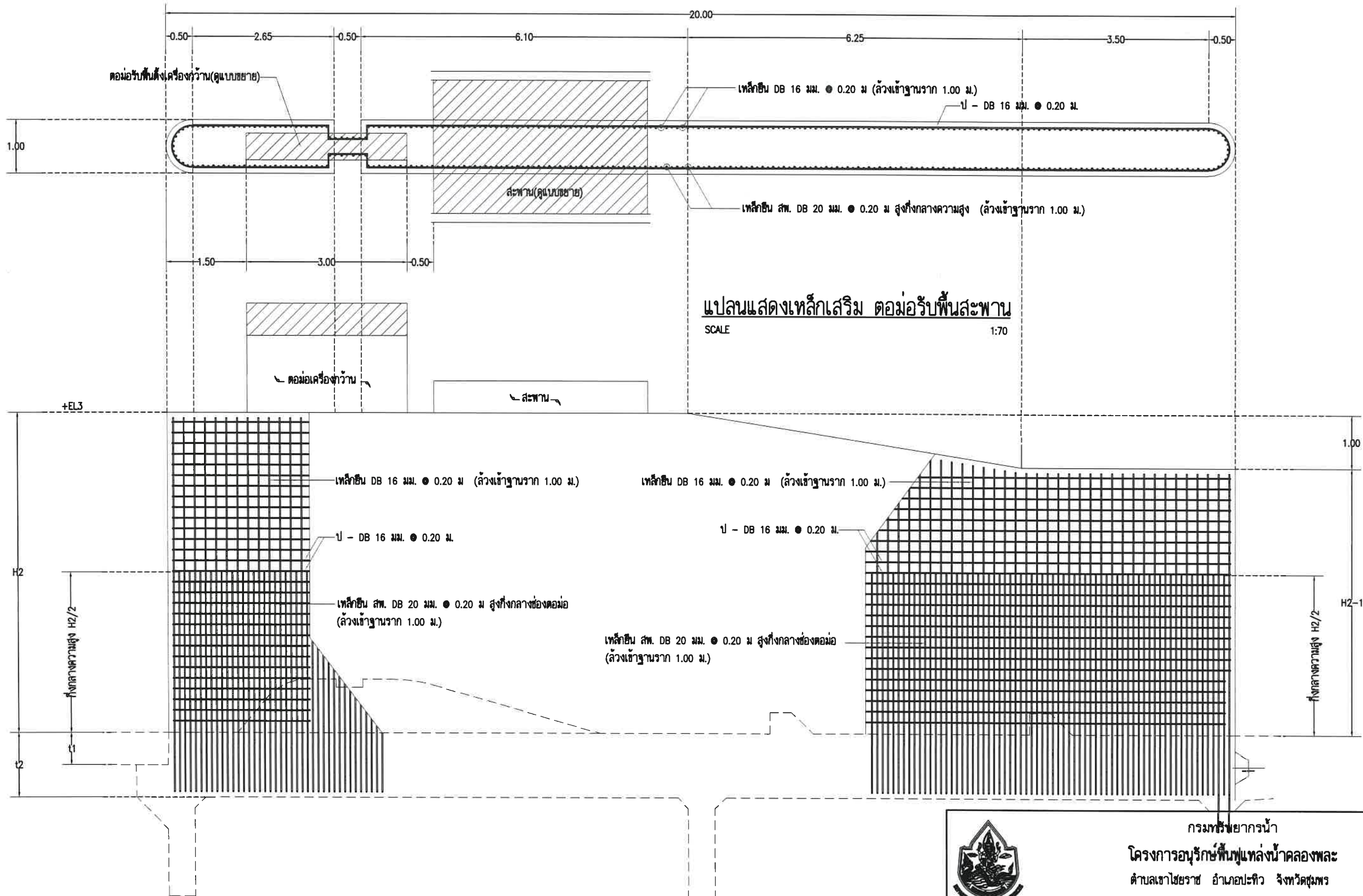
แสดงเหล็กเสริมทางช้างตอม่อรับช่องประตูระบายน้ำ SCALE 1:70
