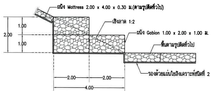
รูปแบบที่ 2 การเรียงหินผนังเชิงลาดส่วนฐาน เชิงลาด 1:2 SCALE 1:100
