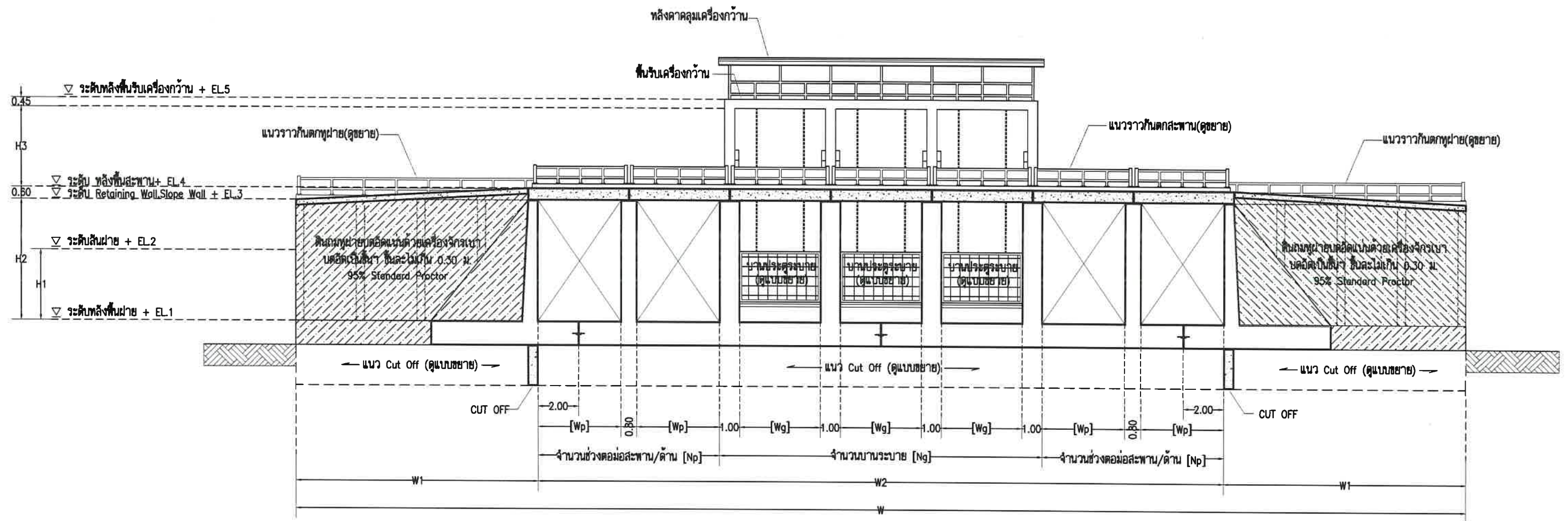
รูปตัดอาคารระบายน้ำตามขวาง A - A มาตราส่วน 1:200
