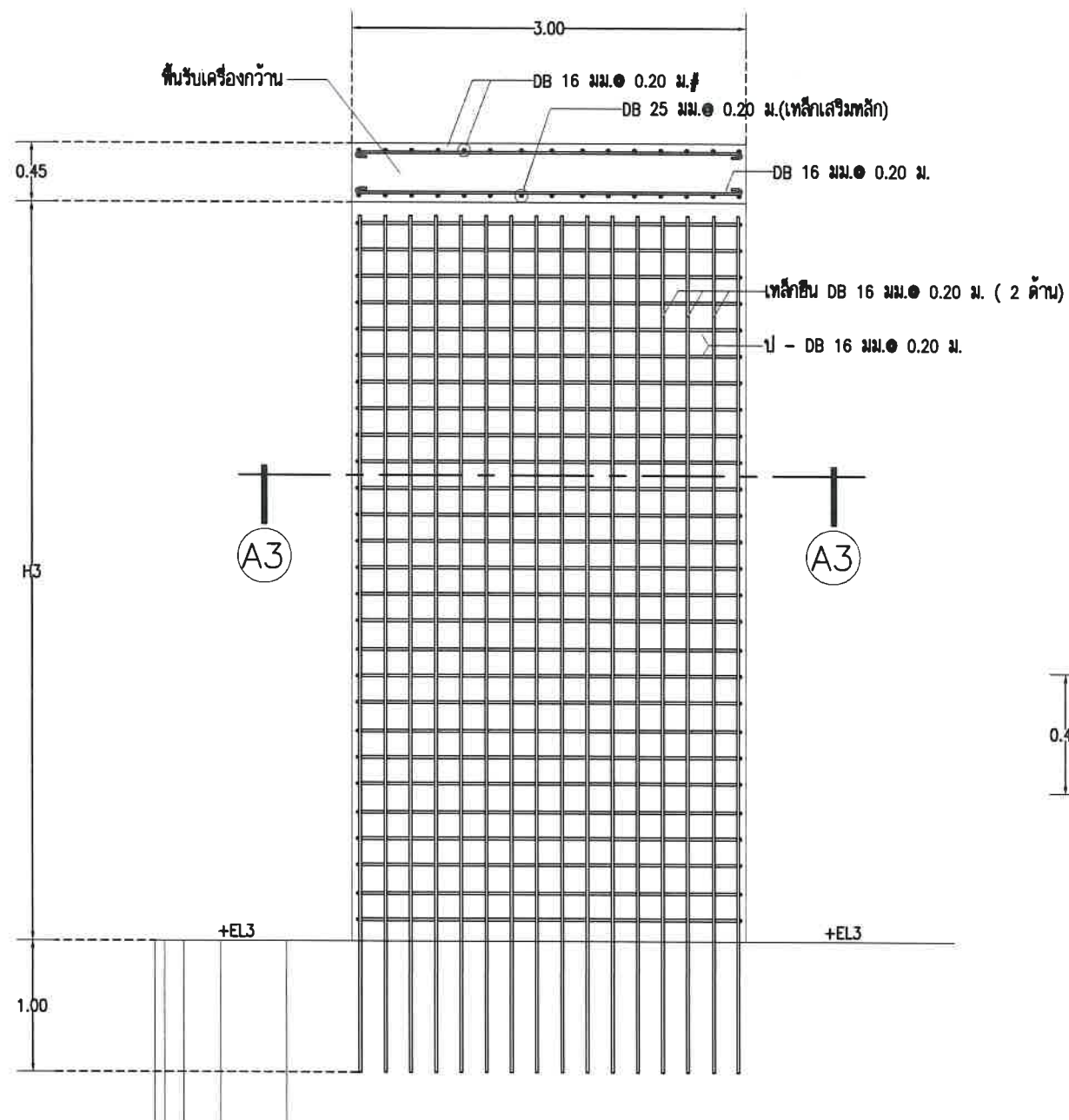
ขยายเหล็กเสริมพิเศษช่องเปิดพื้นรับเครื่องกว้าน SCALE 1:25
