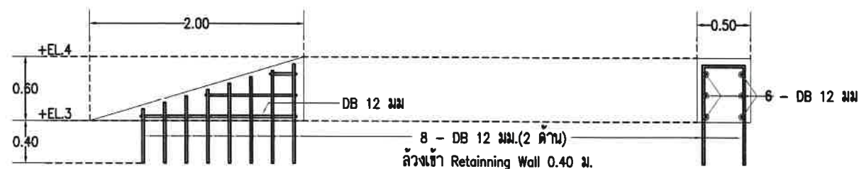
ขยายกำแพงลาด(คอสะพาน)
