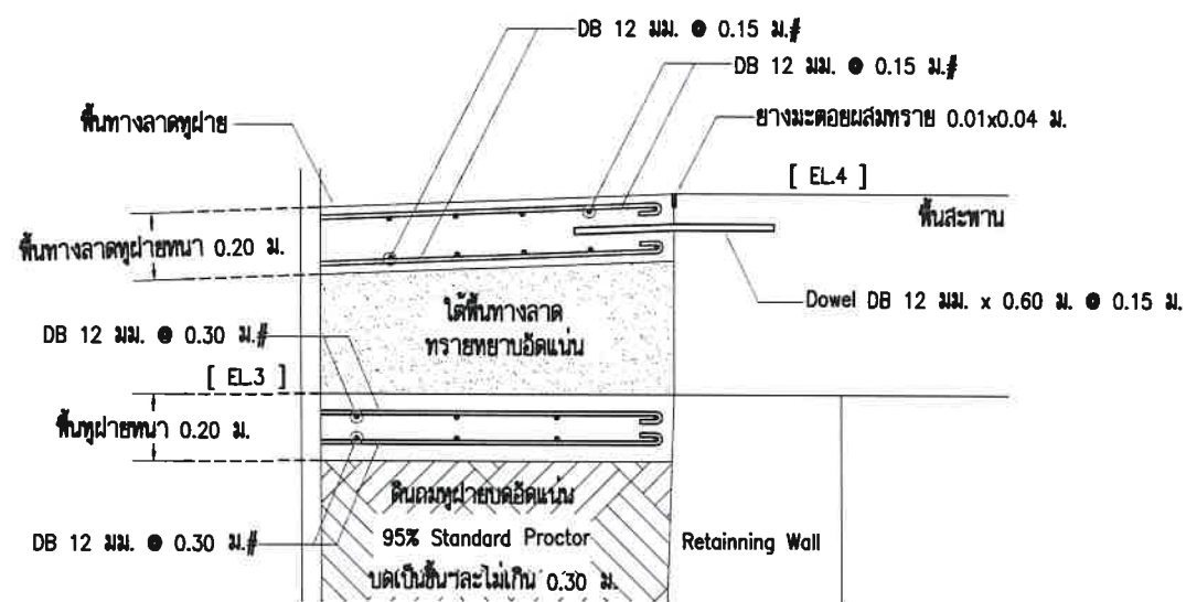
แบบขยายเหล็กเสริม พื้นทางลาดฝาย & พื้นฝาย SCALE 1:25
