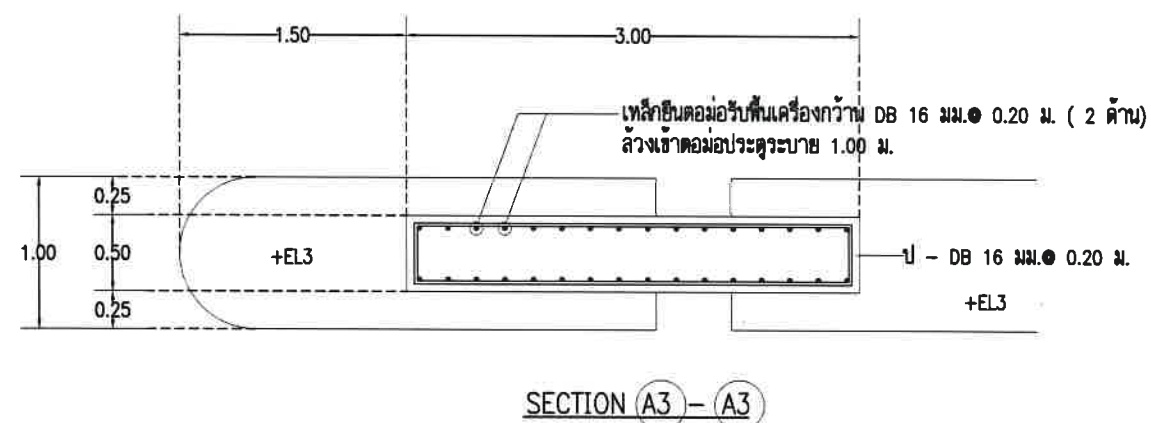
ขยายเหล็กเสริมพื้นรับเครื่องกว้าน ต่อม่อรับพื้น SCALE 1:50
