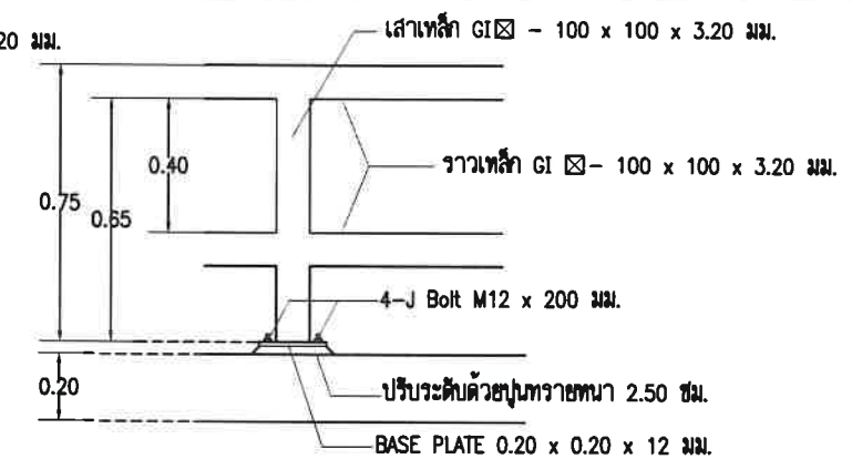
ขยายรูปตัด เสา 100 x 100 มม.
