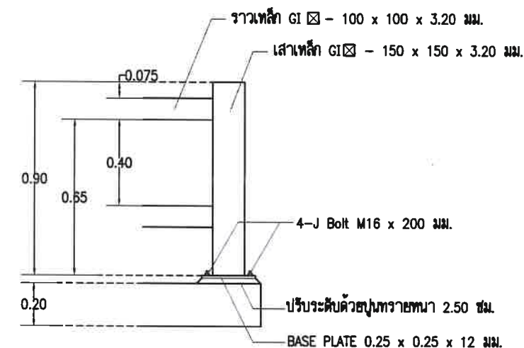
ขยายรูปตัดเสา 150 x 150 มม.
