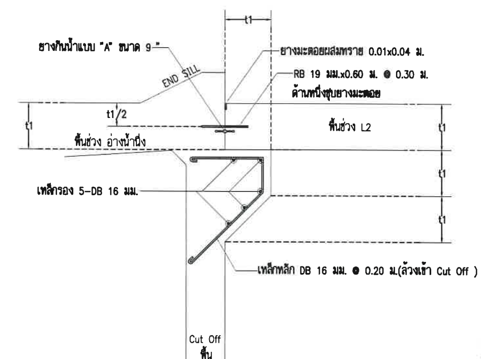
แบบขยายรอยต่อพื้น 3 SCALE 1:50
