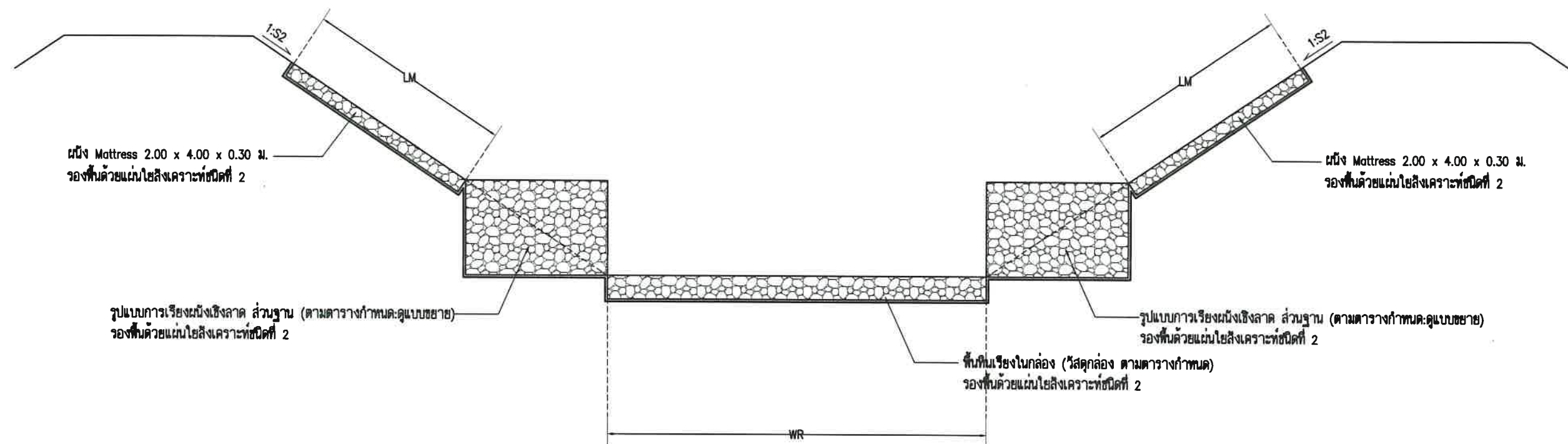
แสดงหน้าตัดการเรียงหินป้องกันการกัดเซาะ ด้านเหนือน้ำ และ ด้านท้ายน้ำ
