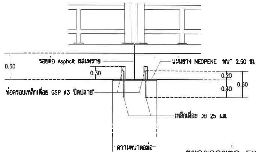
ขยายรอยต่อ FREE BEARING
