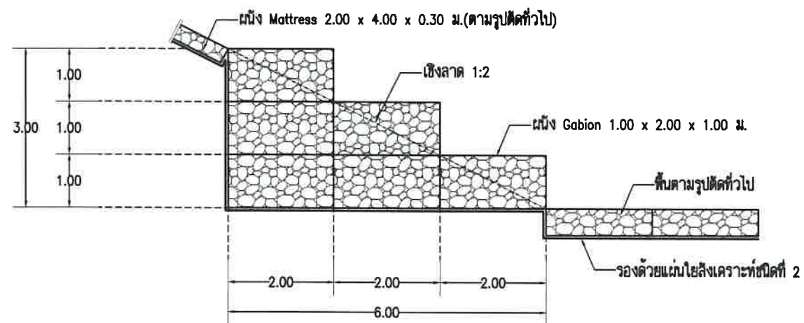
รูปแบบที่ 1 การเรียงหินผนังเชิงลาดส่วนฐาน เชิงลาด 1:2 SCALE 1:100
