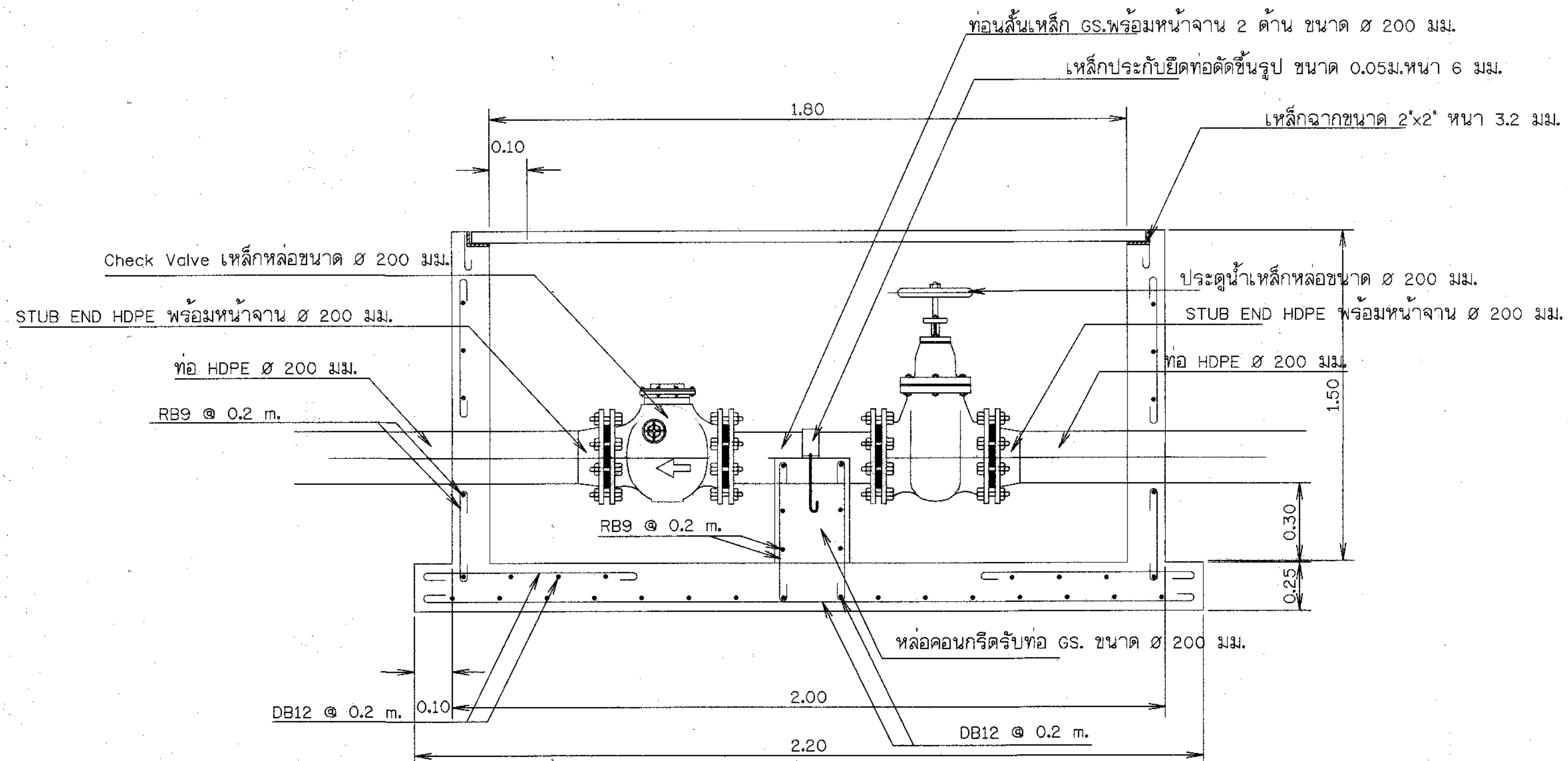
รูปตัด A - A ขยายจุดประตุน้ำคุมท่อจ่ายน้ำ ขนาด 200 มม.
