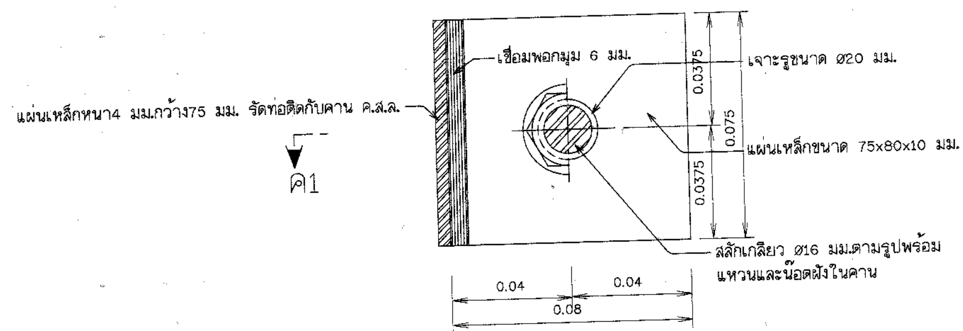
แบบแผ่นเหล็กยึดท่อ ไม่แสดงมาตราส่วน
