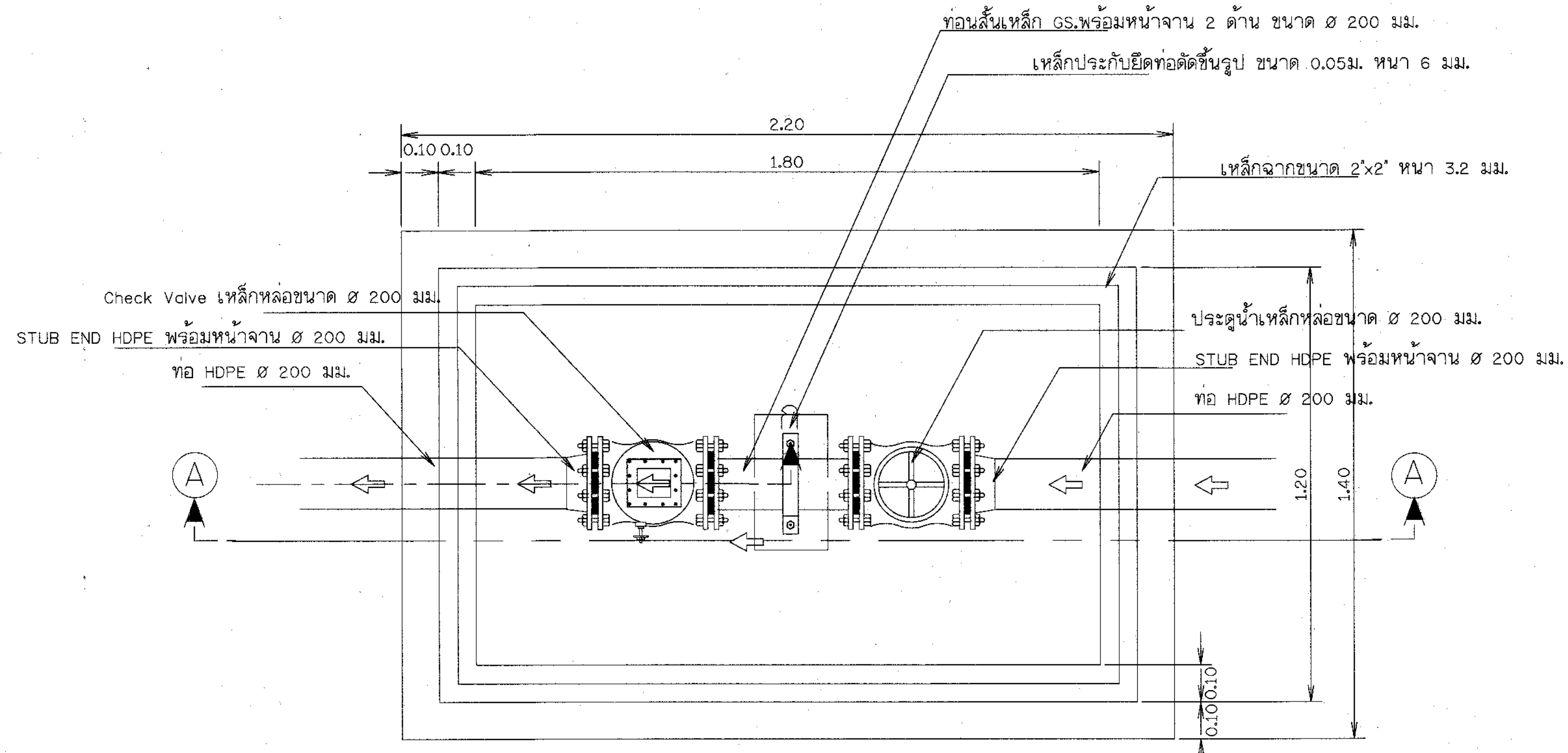
แปลนจุดประตุน้ำคุมท่อจ่ายน้ำ ขนาด 200 มม.
