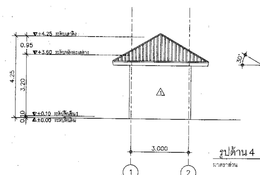
รูปด้าน 3 มาตราส่วน 1:100
