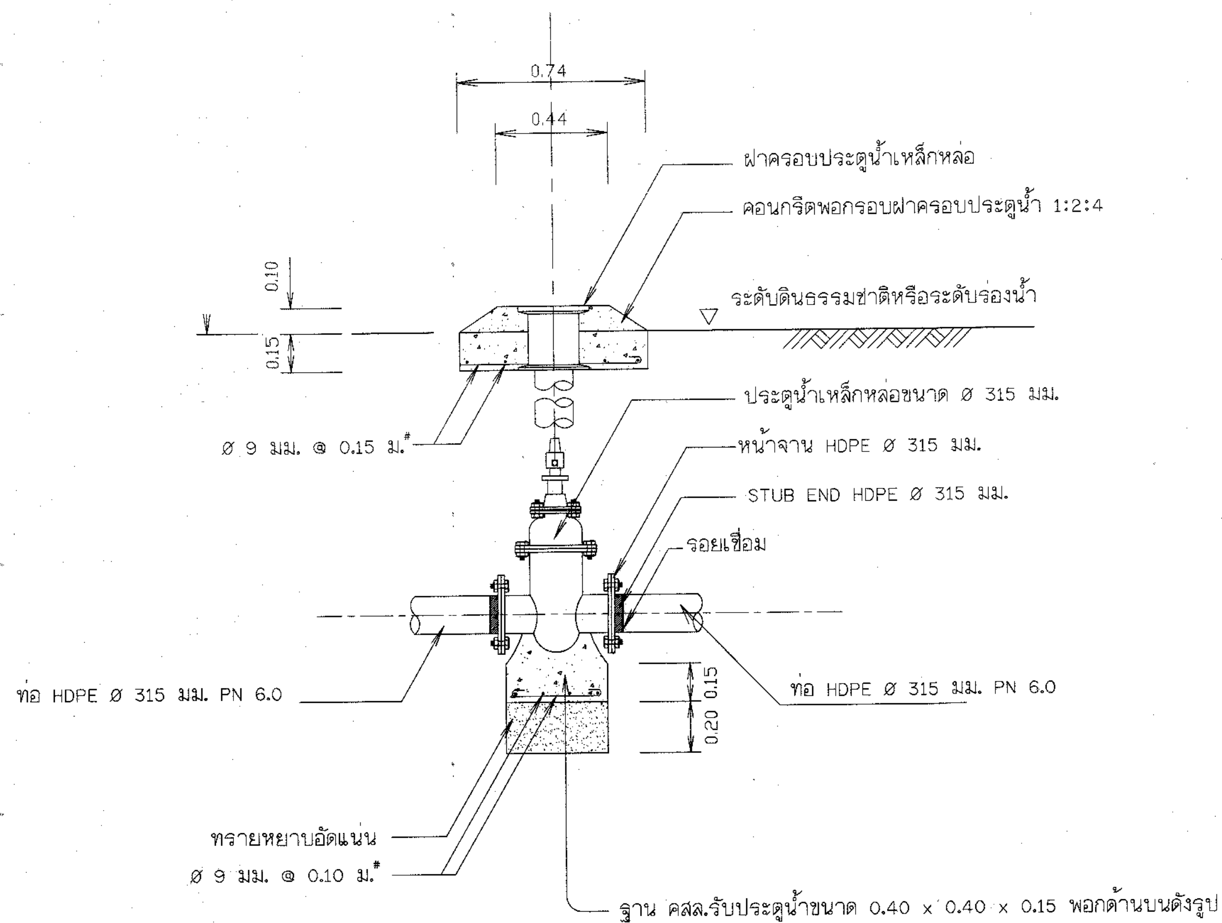
รูปตัด ก - ก แสดงการติดตั้งประตูกวควบคุมท่อยาน้ำ ขนาด 315 มม.
