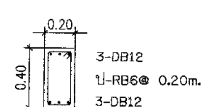
แบบขยายโครงสร้างคาน SCALE 1:100
