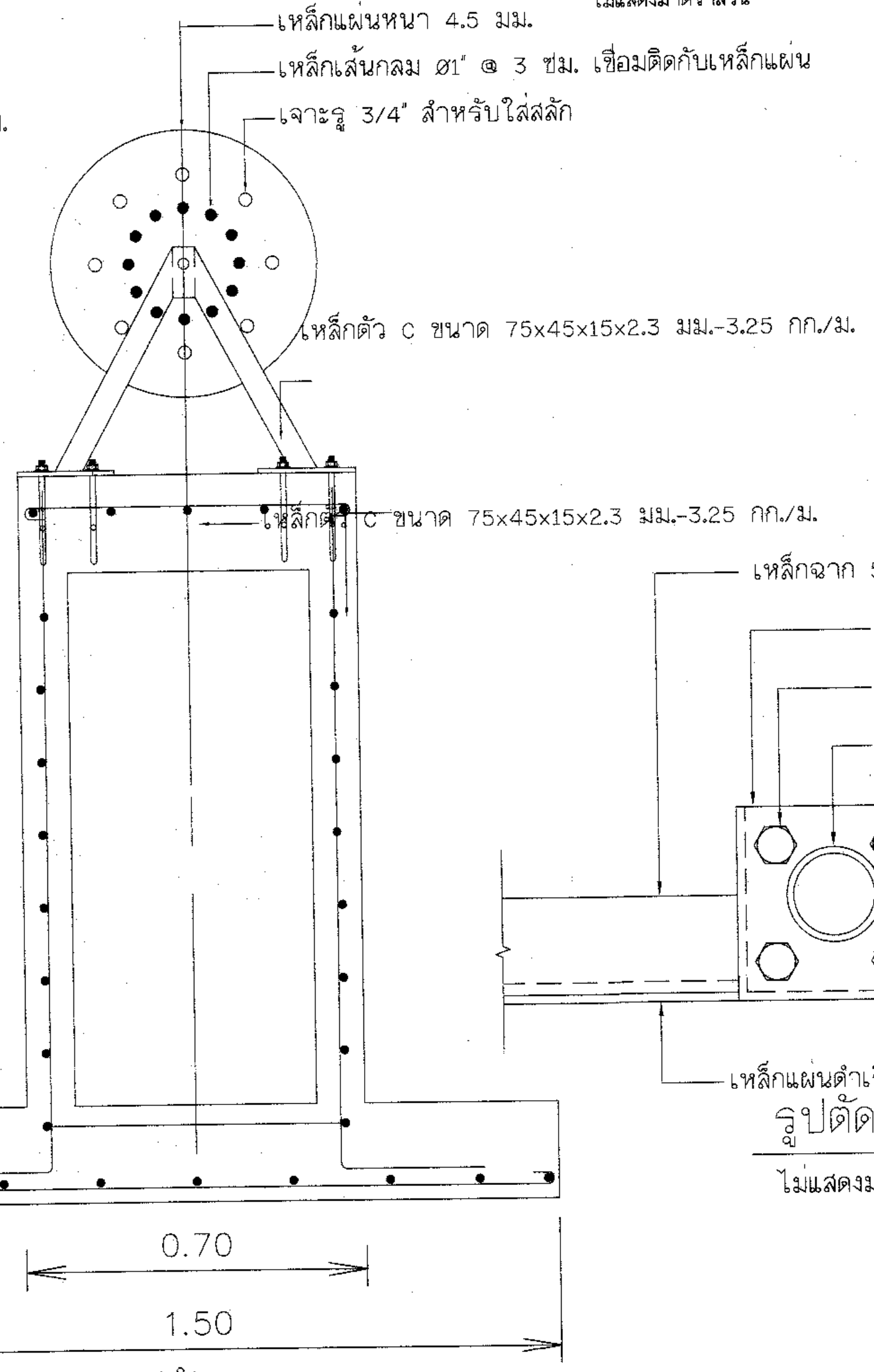
รูปตัด 2-2
