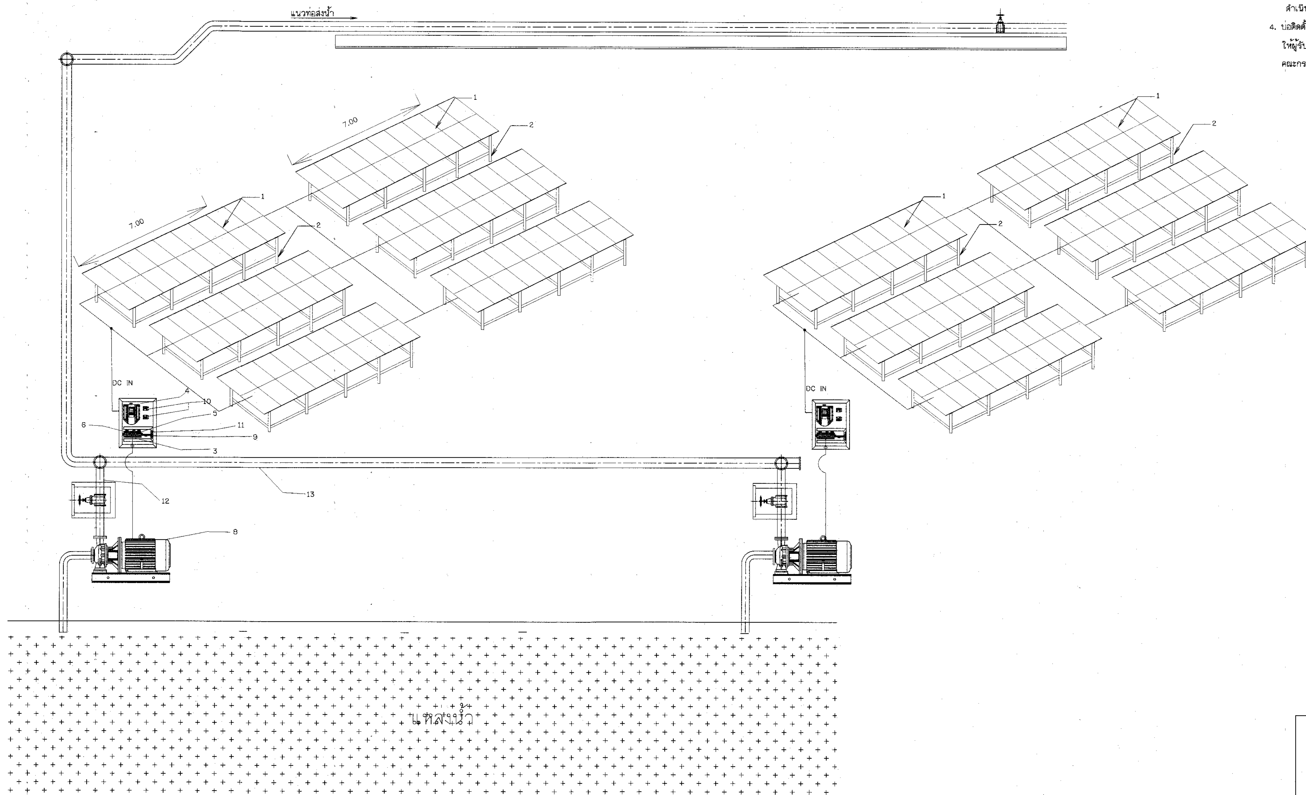
แบบระบบกระจายน้ำด้วยพลังงานแสงอาทิตย์ มาตราส่วน ไม่แสดงมาตราส่วน
