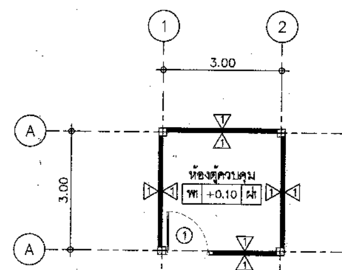
แปลนพื้นชั้น 1 มาตราส่วน 1:100
