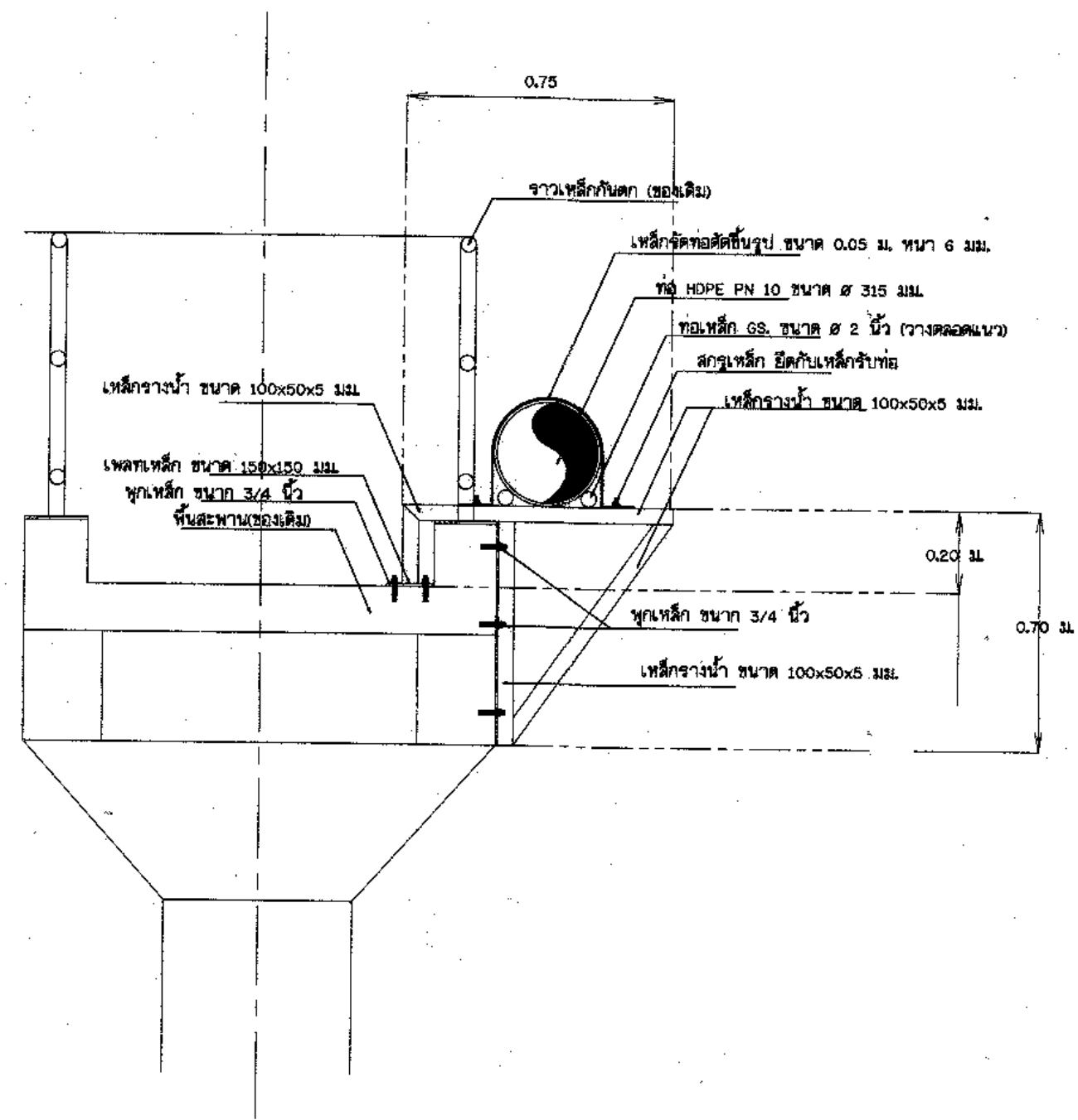
รูปตัดขยายการวางท่อจ่ายข้างสะพาน ขนาด 315 มม. มาตราส่วน No Scale
