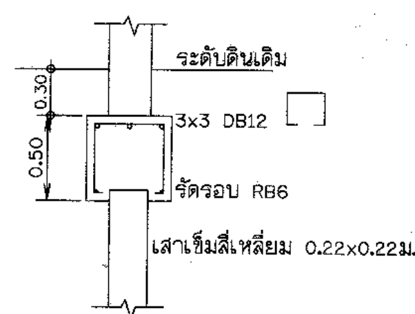
แบบขยายฐานราก มาตราส่วน 1:100
