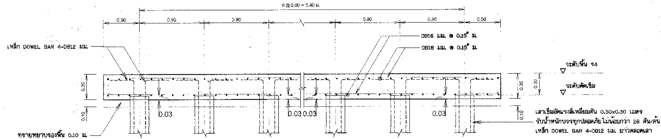
รูปตัด ก1 - ก1
