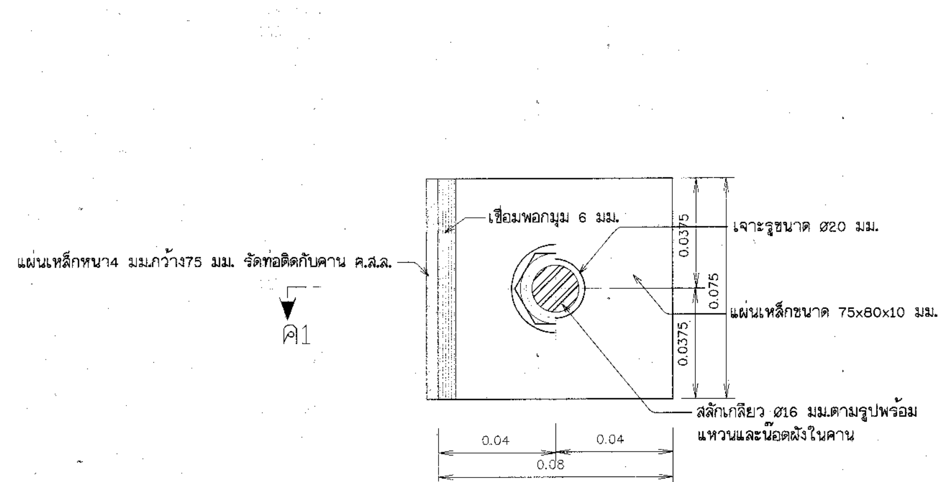
แปลนแผ่นเหล็กยึดท่อ ไม่แสดงมาตราส่วน
