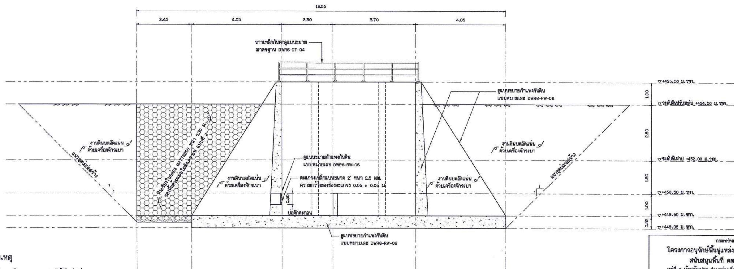
รูปตัดแนว ค - ค
