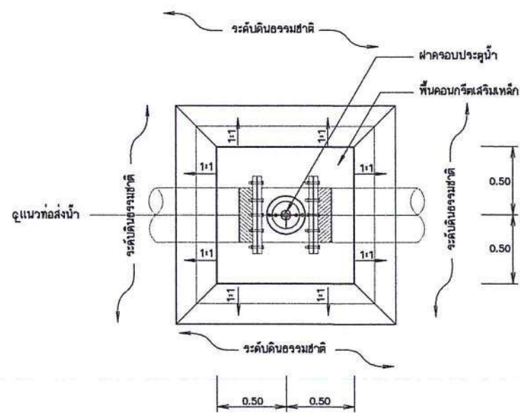
แปลนอาคารควบคุมพลังงาน มาตราส่วน 1:20
