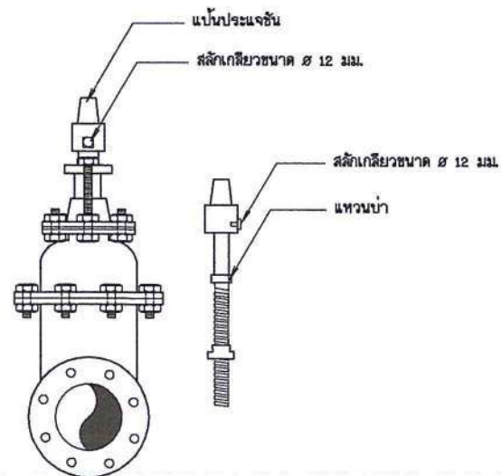
รายละเอียดประตุน้ำเหล็กหล่อ มาตราส่วน ไม่แสดงมาตราส่วน
