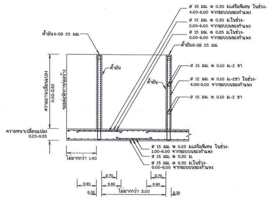
รูปตัด ง - ง
