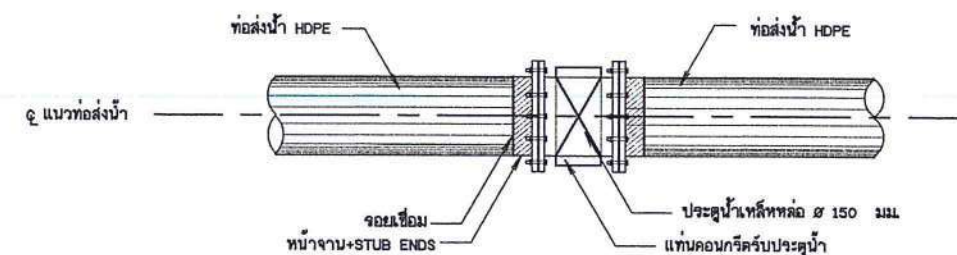
รูปขยายการติดตั้งอาคารควบคุมพลังงาน มาตราส่วน 1:20
