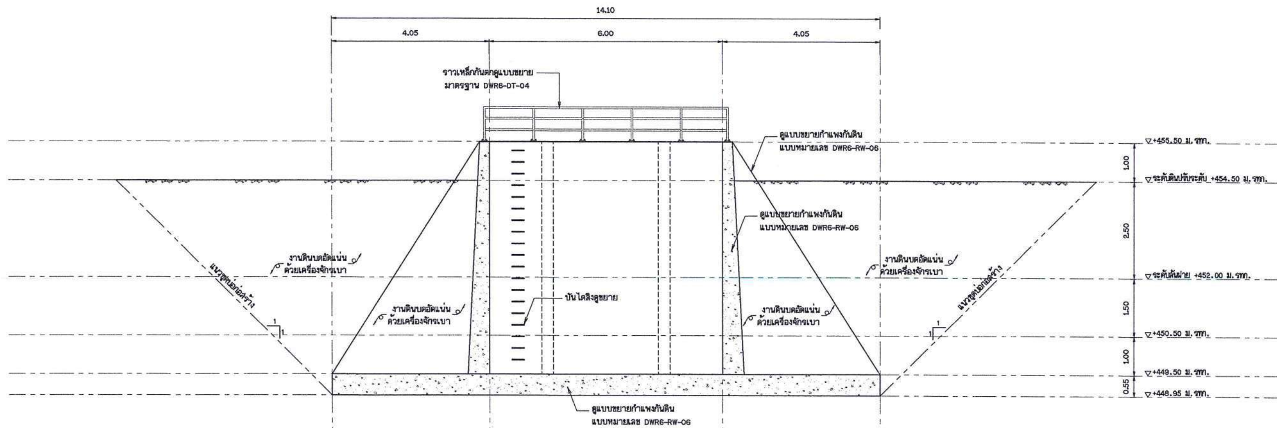
รูปตัดแนว ข - ข
