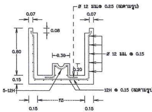
เหล็กเสริมบ่อประตูปรับน้ำ
