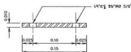
รูปตัด ค-ค
