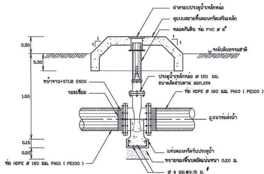
รูปตัดอาคารควบคุมพลังงาน มาตราส่วน 1:20
