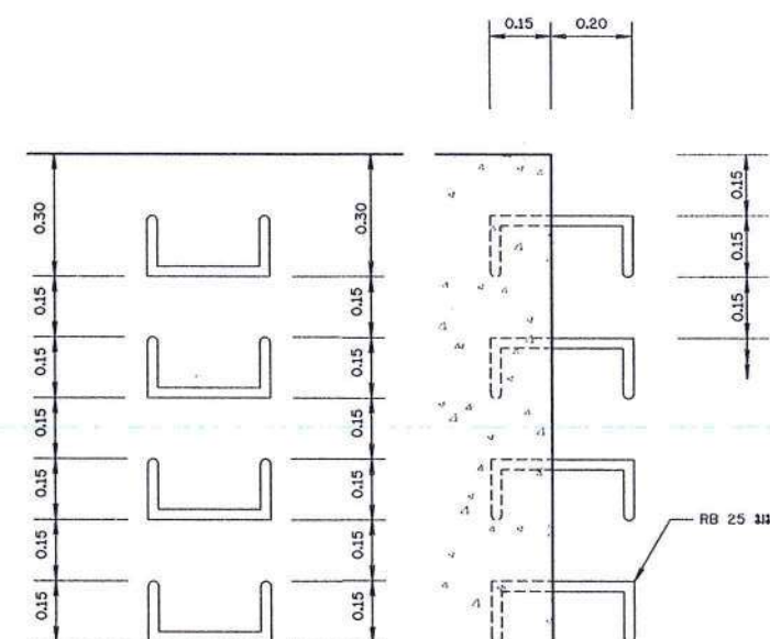
รูปขยายบันไดลิง
