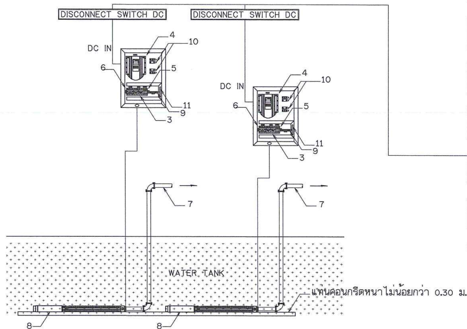
แบบระบบกระจายน้ำด้วยพลังงานแสงอาทิตย์ มาตราส่วน ไม่แสดงมาตราส่วน
