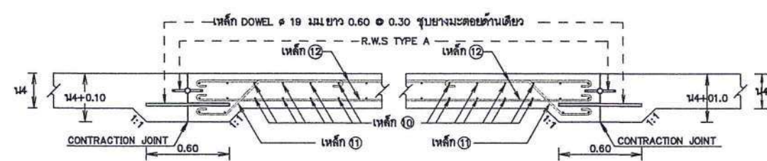
รูปตัดแสดงการเสริมเหล็กพื้นสระ มาตราส่วน 1:20
