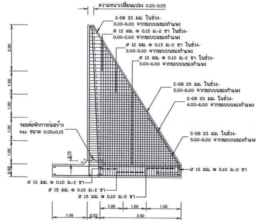
การเสริมเหล็กกำแพงค้ำยัน
