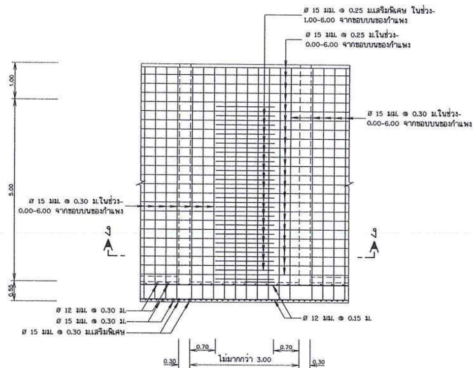
รูปตัดตามยาวของกำแพงบานไม่ติดดิน
