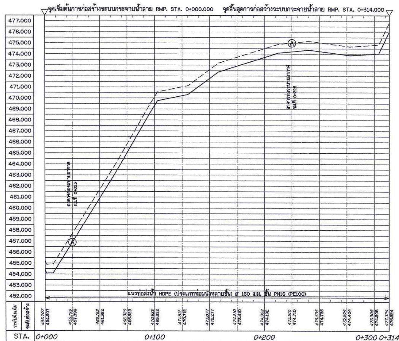
รูปตัดตามแนวยาว มาตราส่วน 1:500 แนวราบ 1:1,000
