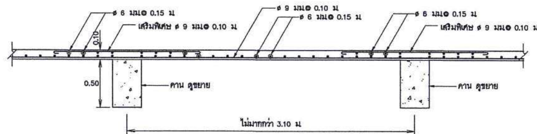
ขยายการเสริมเหล็กพื้นปิดสระ มาตราส่วน 1:20
