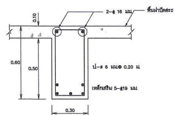
เสริมเหล็กคานแบบที่ ① มาตราส่วน 1:10
