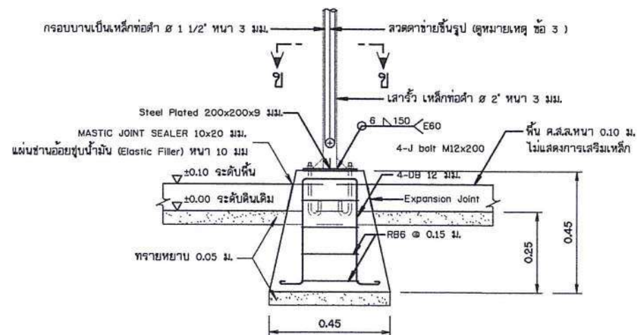
รูปขยายฐานรากโครงสร้างรับแผง F2 (ต่อม่อ คสล. หล่อเสาเชิงรูปพร้อมติดตั้ง)
