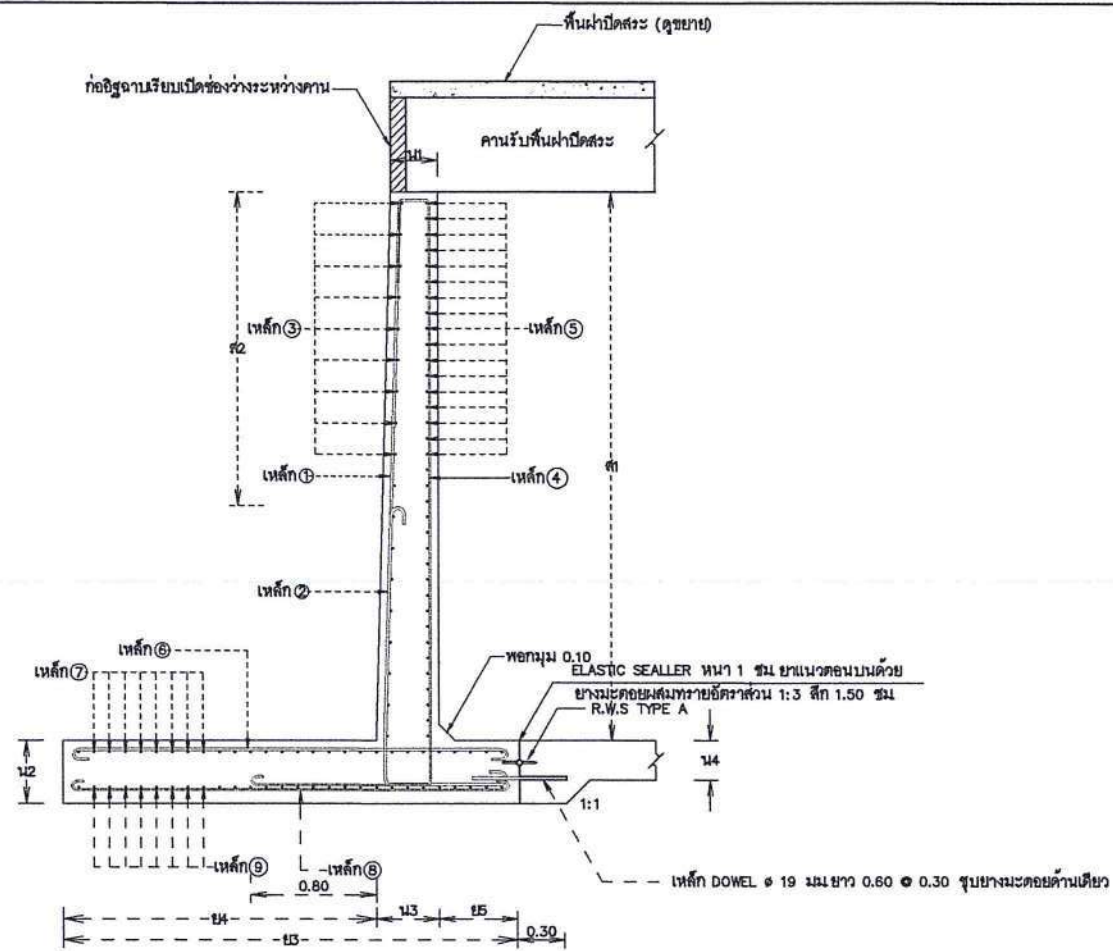
รูปตัดแนว ค - ค มาตราส่วน 1:25
