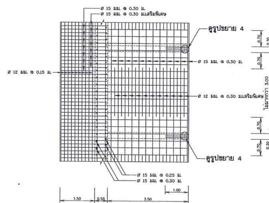
รูปตัดตามยาวของพื้นด้านล่าง
