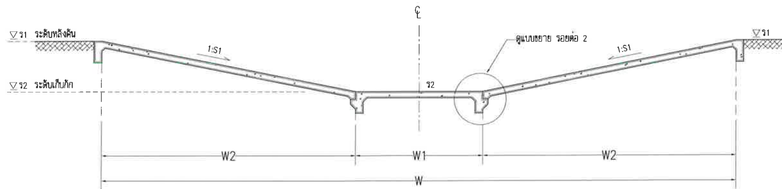
รูปตัดตามยาวอาคารระบายน้ำ ข - ข มาตราส่วน 1:150
