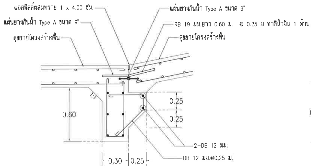
ขยายรอยต่อคอนกรีต 2 มาตราส่วน 1:25
