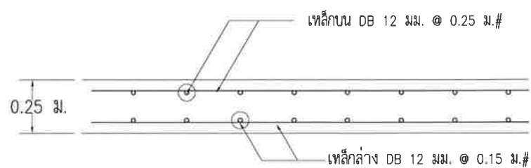
ขยายโครงสร้างพื้นอาคารระบายน้ำ(ทุกชั้น) มาตราส่วน 1:25
