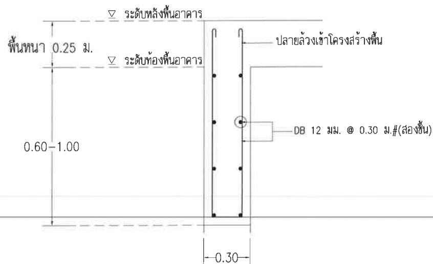
ขยายโครงสร้าง CutOff 0.60-1.00 ม. มาตราส่วน 1:25
