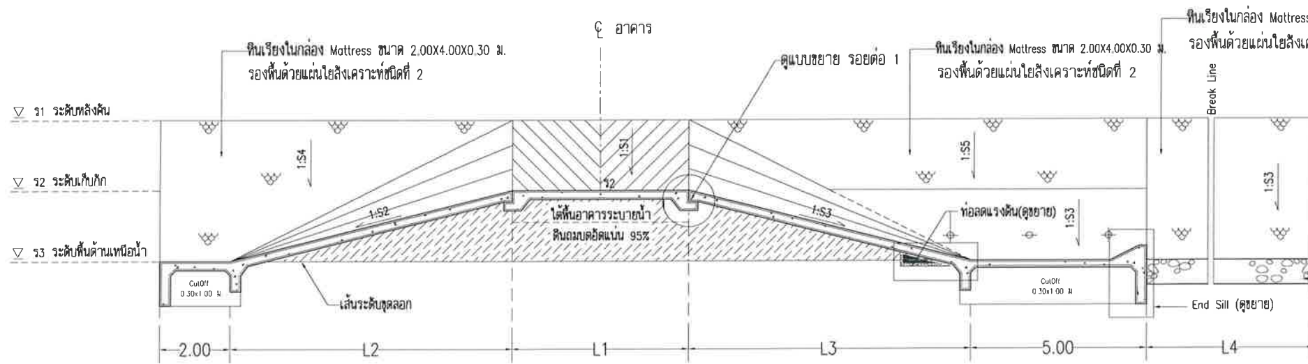
รูปตัดตามยาวอาคารระบายน้ำ ก - ก มาตราส่วน 1:150
