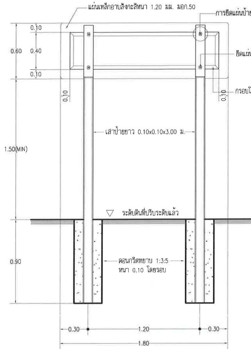
แสดงรูปด้านหลังแนะนำโครงการ SCALE 1:25
