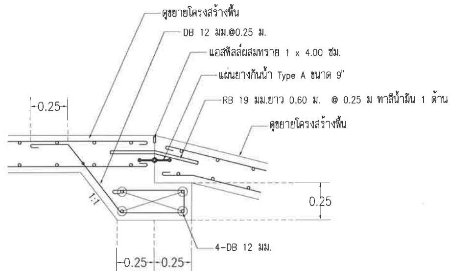
ขยายรอยต่อคอนกรีต 1 มาตราส่วน 1:25
