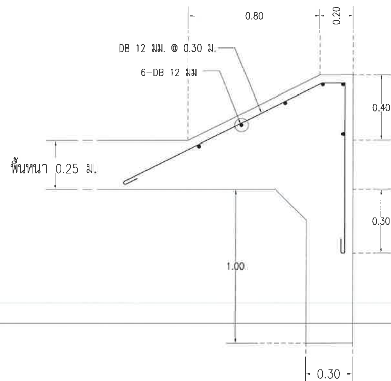
แบบขยาย End Sill มาตราส่วน 1:25
