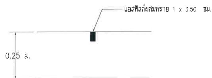
ขยาย Mastic Joint Filler
