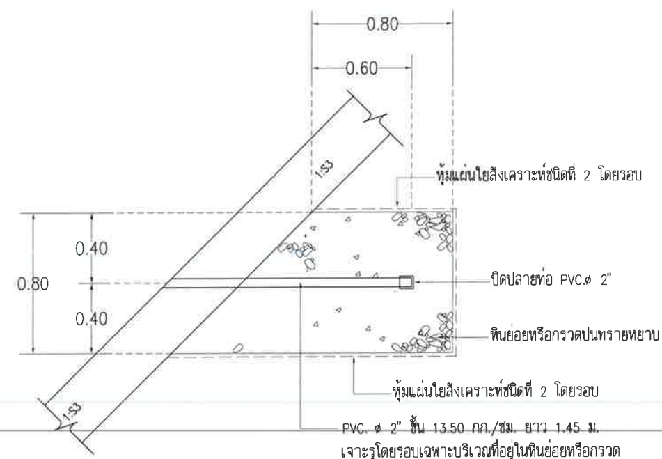
ขยายท่อลอดแรงดัน SCALE 1:30
