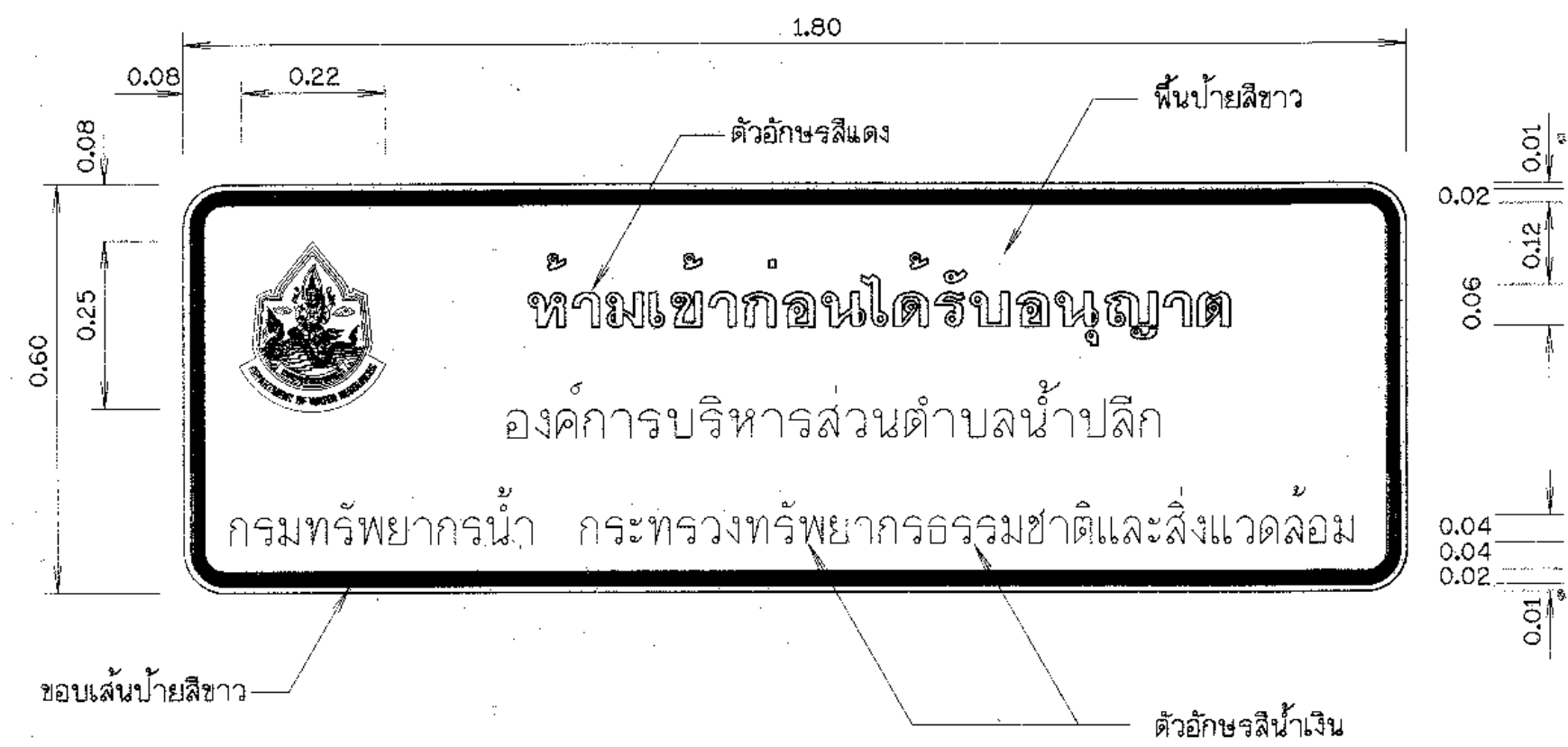
แบบขยาย 1 มาตราส่วน 1:10
