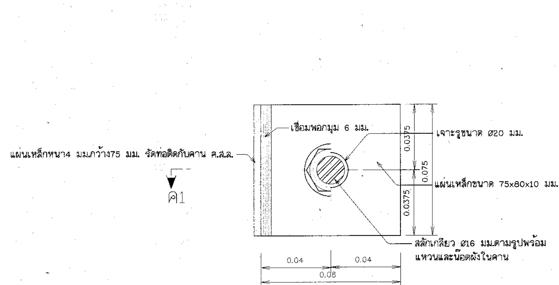
แผนแผ่นเหล็กยึดท่อ ไม่แสดงมาตราส่วน
