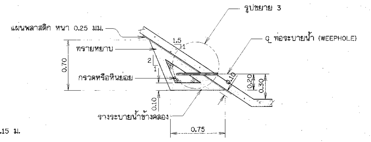
รูปขยาย 2 ระบบระบายน้ำข้างคลอง ไม่แสดงมาตราส่วน
