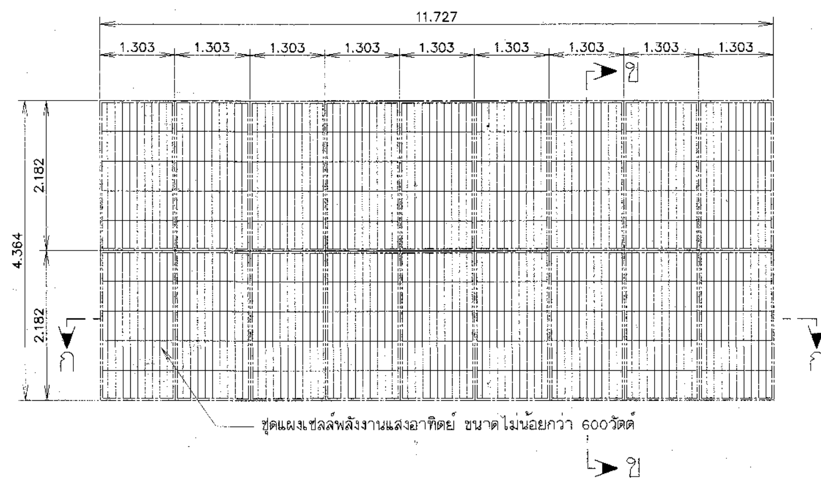
แปลนแผงเซลล์พลังงานแสงอาทิตย์ขนาดไม่น้อยกว่า 600 วัตต์
