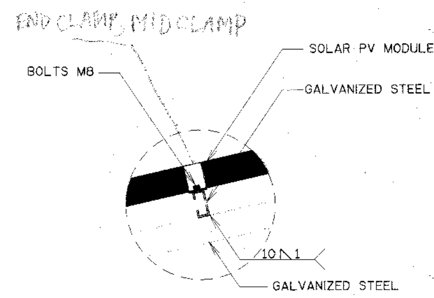
รูปขยายเสา มาตราส่วน 1:10
