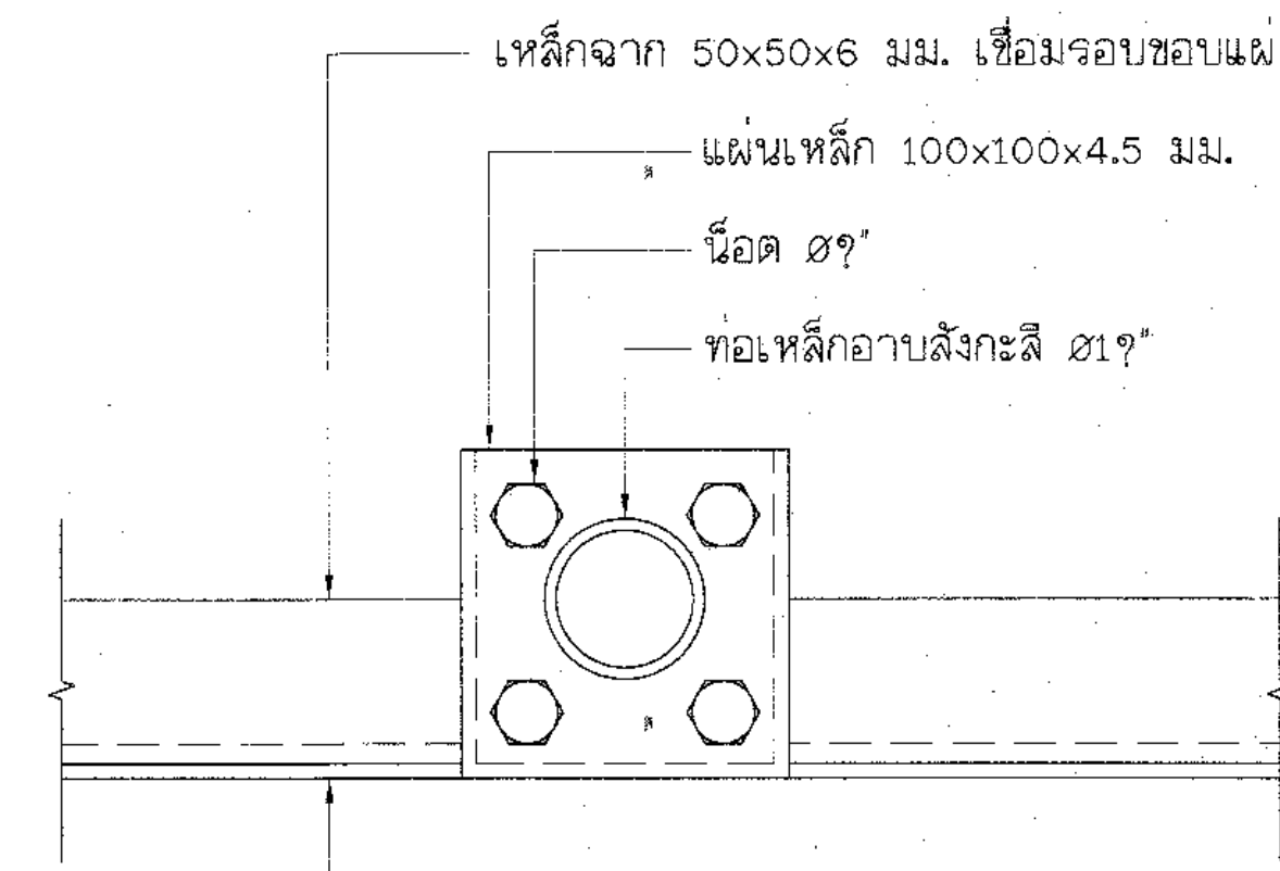
แบบขยาย "ช"
