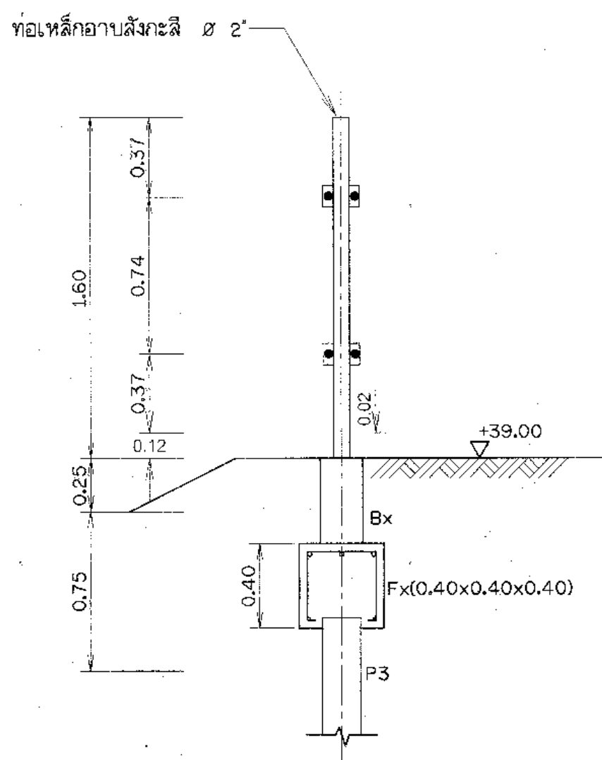
แบบขยายรั้ว (รูปด้านข้าง) มาตราส่วน 1:25
