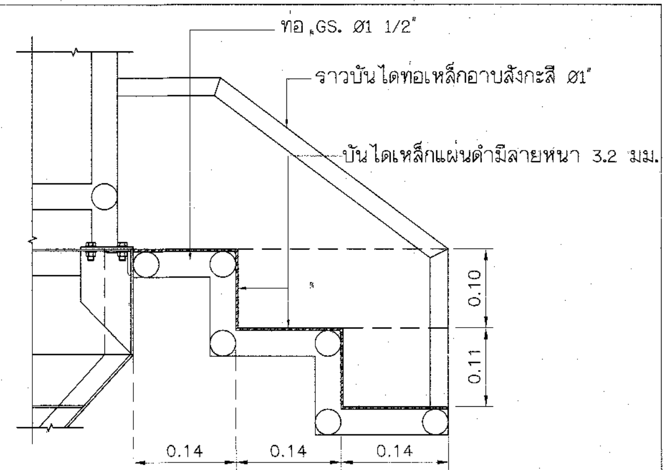
แบบขยาย "ง"
