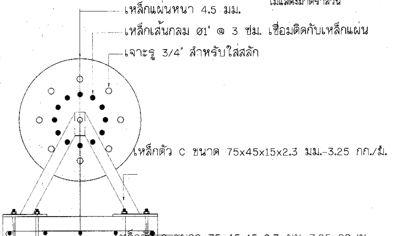
แบบขยาย "ง"
