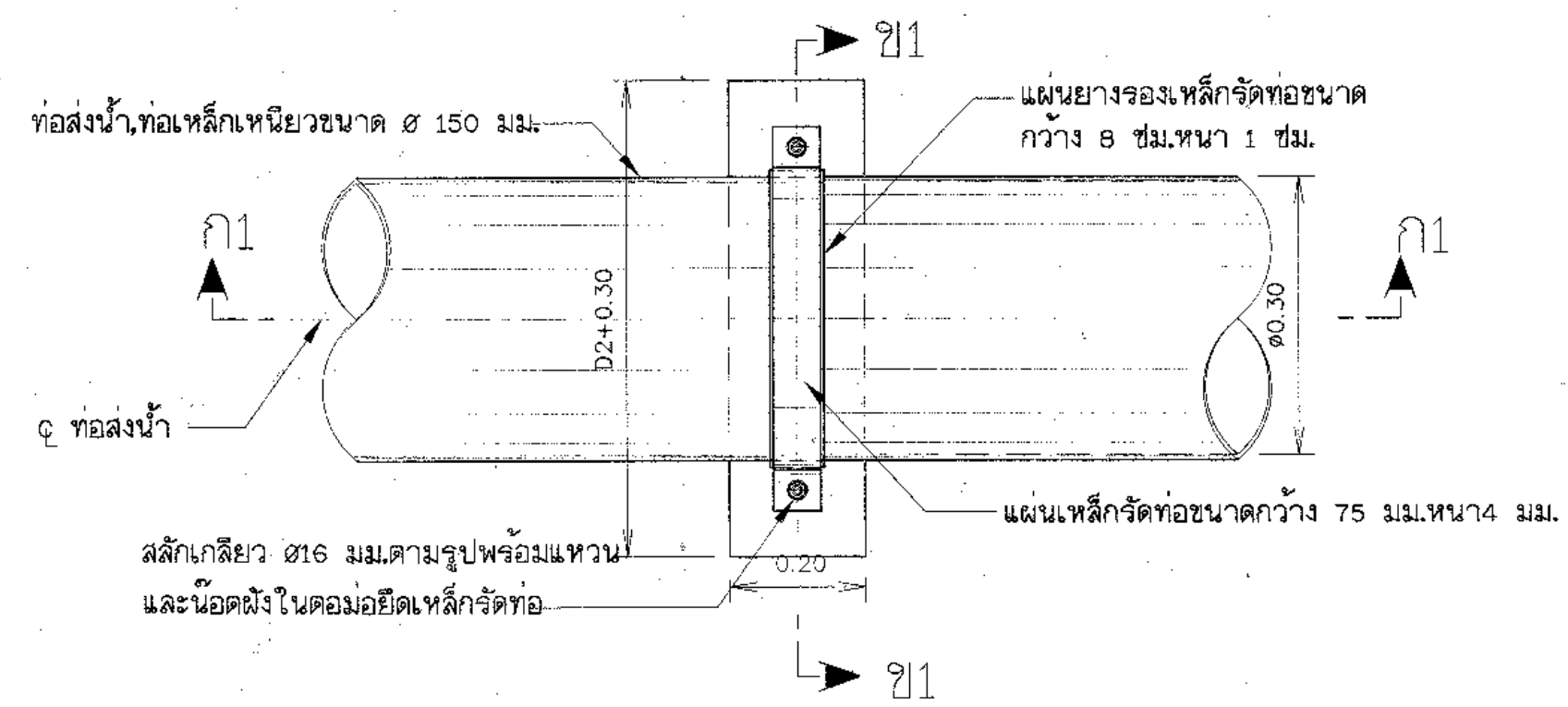
แผนการยึดท่อ ไม่แสดงมาตราส่วน
