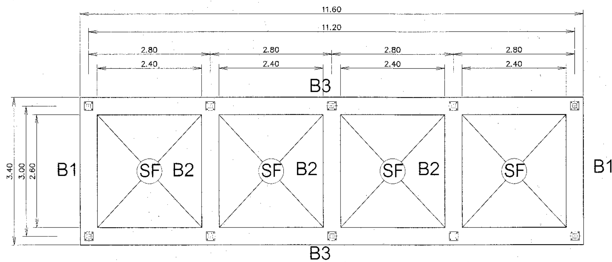
แปลนคานาคอนดิน
