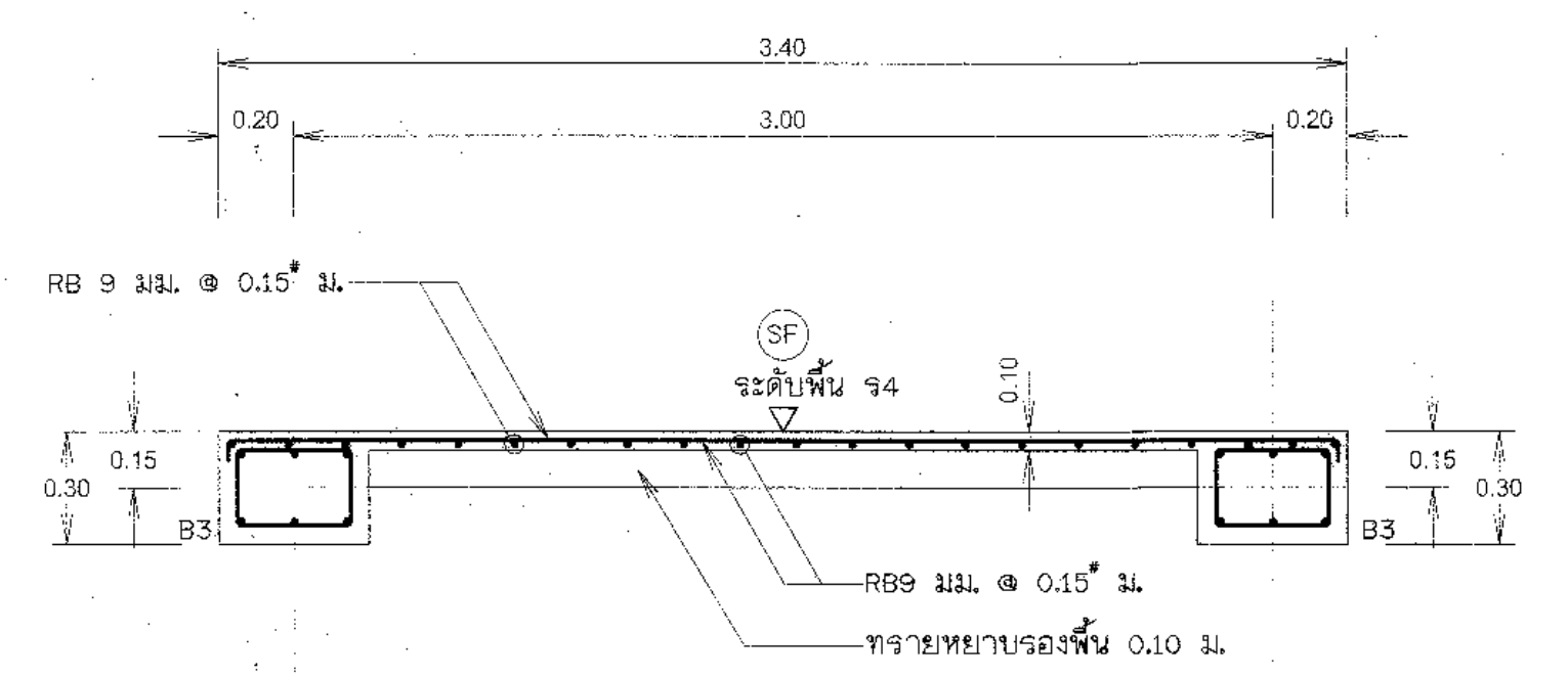
รูปตัด ก1 - ก1
