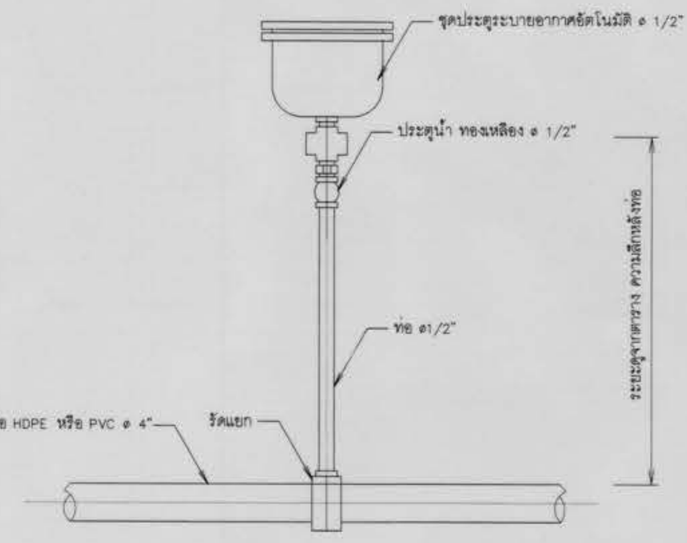
12. การติดตั้งประตูละบายอากาศอัด โนมิตี ไม่แสดงขนาดจาวส่วน
