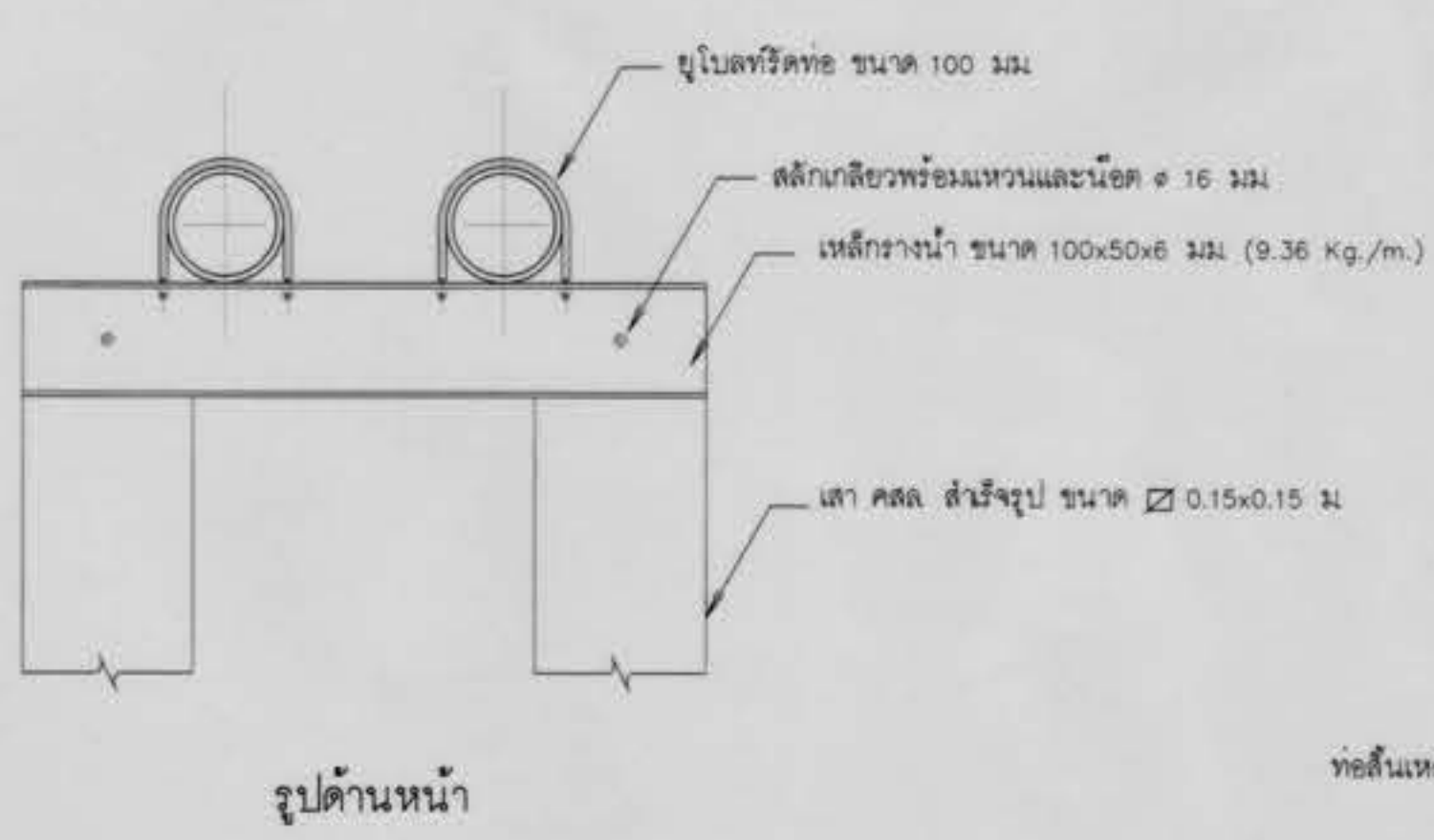
13. เสาต่อม่อรับท่อชุด และแบบขยายอุปกรณ์รีดท่อ ไม่แสดงขนาดจาวส่วน
