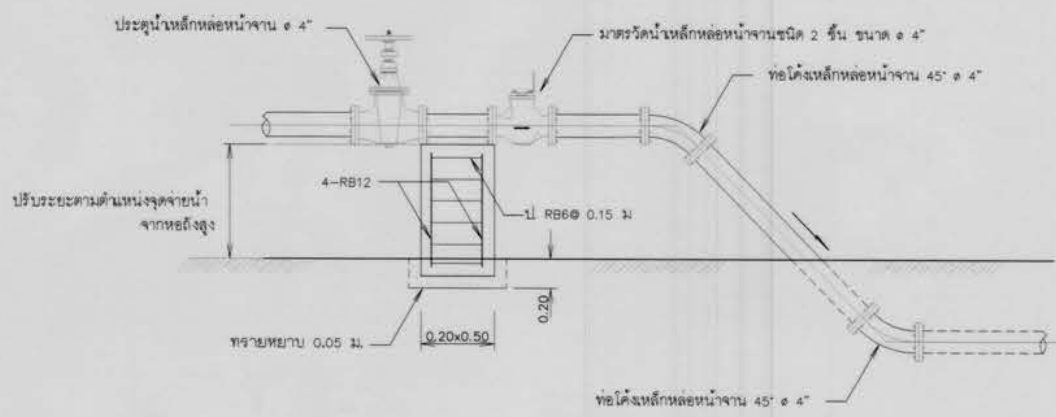
14. การติดตั้งมาตรวัดน้ำบนพื้นดิน ๑ 4" ไม่แสดงขนาดจาวส่วน
