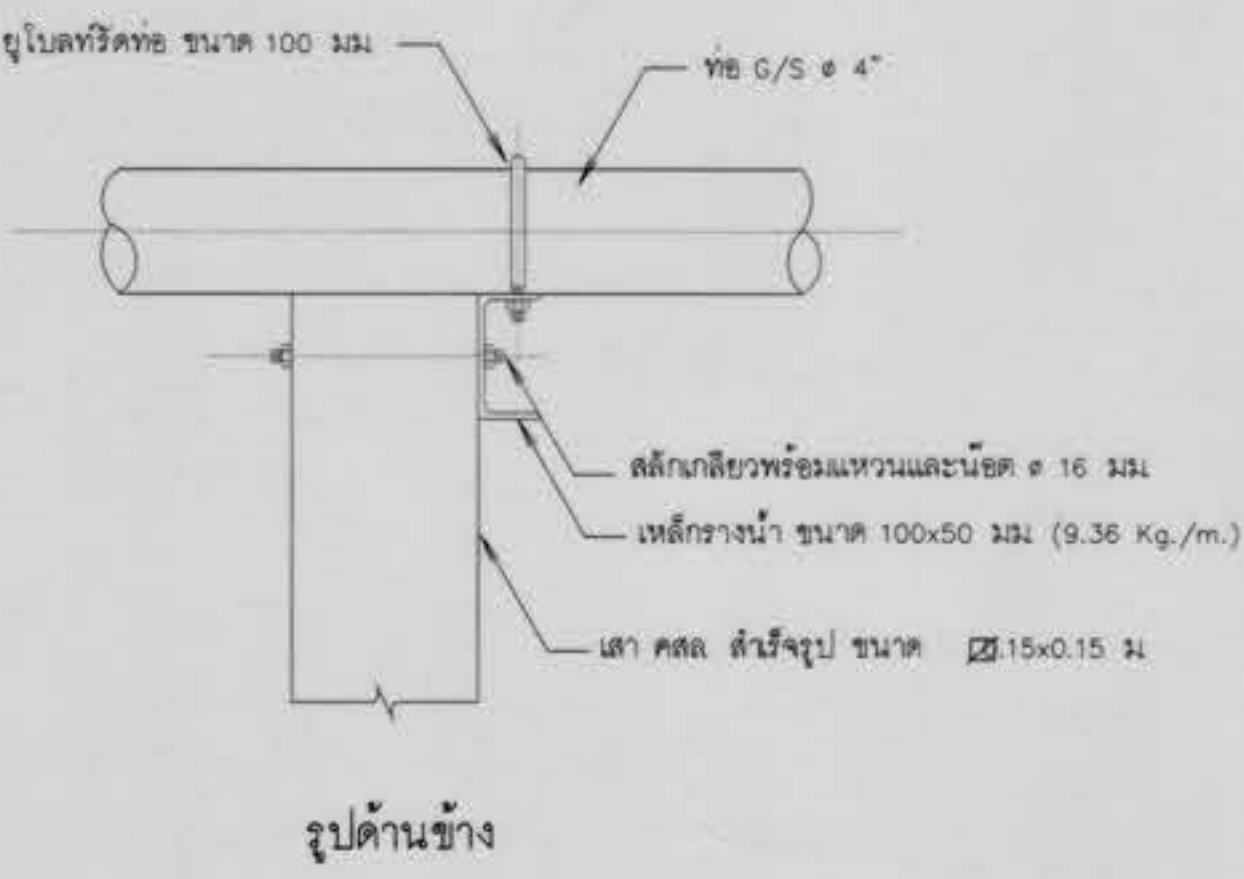
13. เสาต่อม่อรับท่อชุด และแบบขยายอุปกรณ์รีดท่อ ไม่แสดงขนาดจาวส่วน
