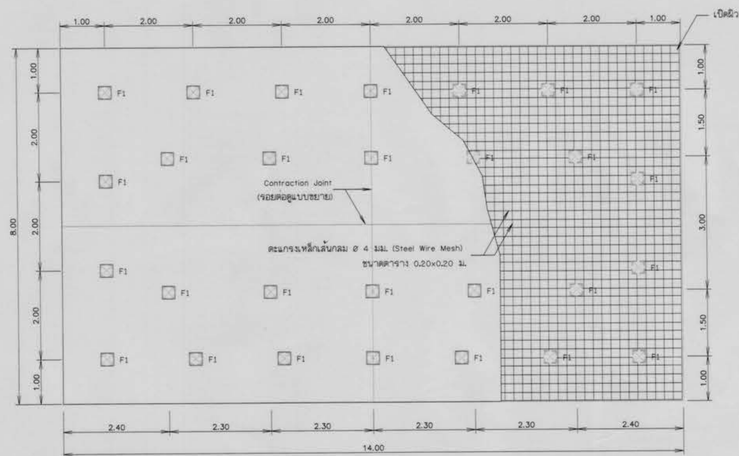
แผนฐานรากและโครงหลังคา โมเมนต์ตามราส่วน
