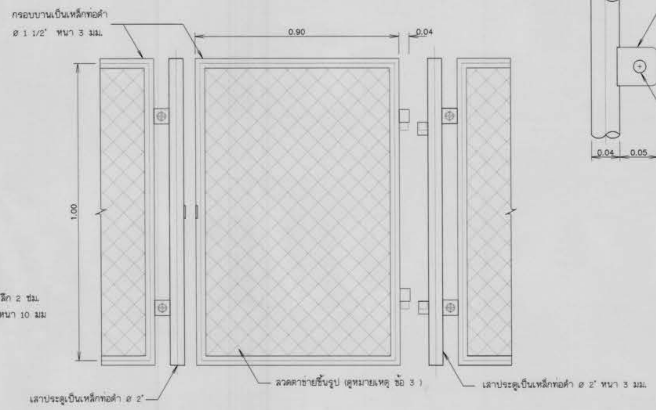
แบบขยายรายละเอียดประตู ไม่แสดงขนาดจาล้วน
