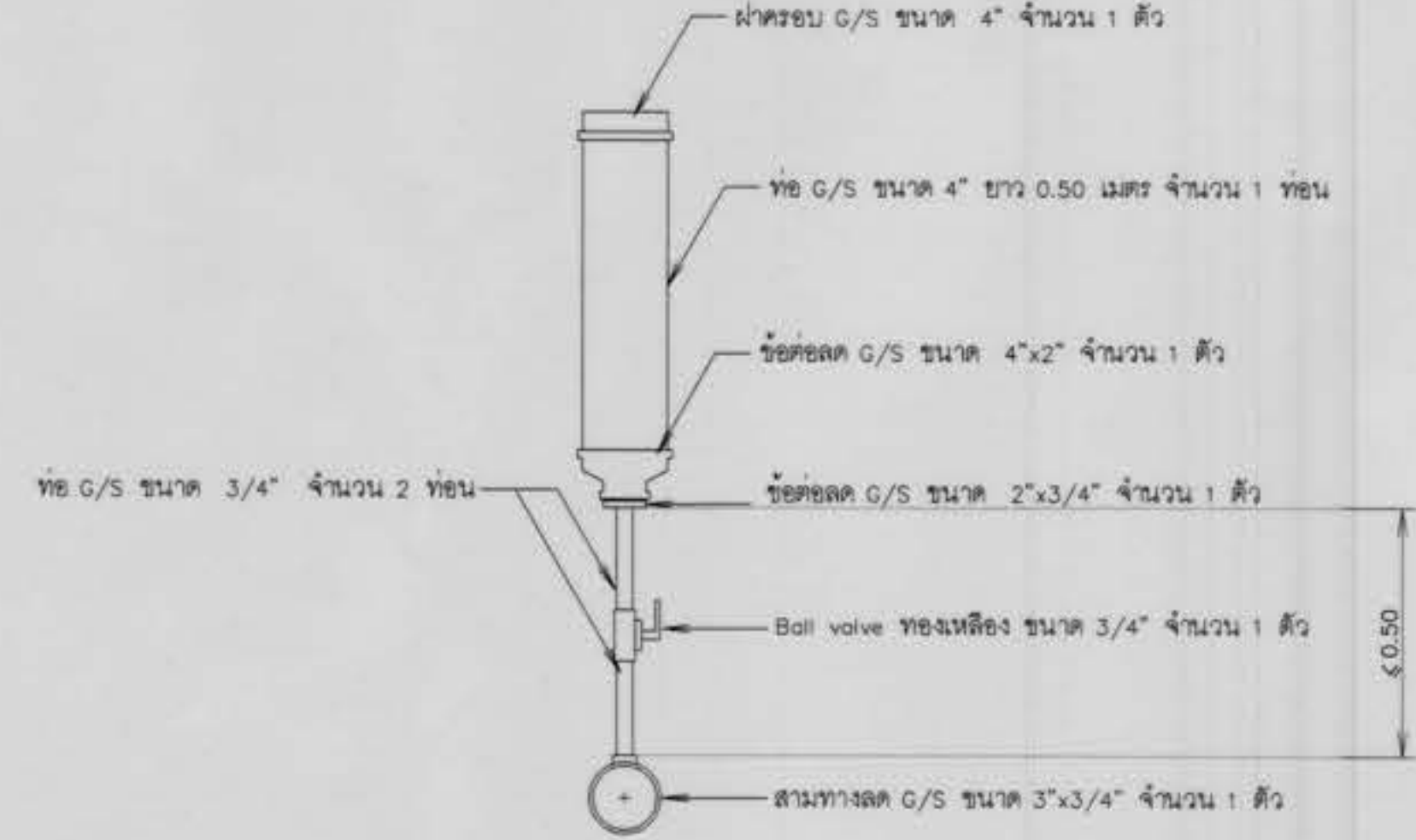
11. ช่องเติมน้ำ ไม่แสดงขนาดจาวส่วน
