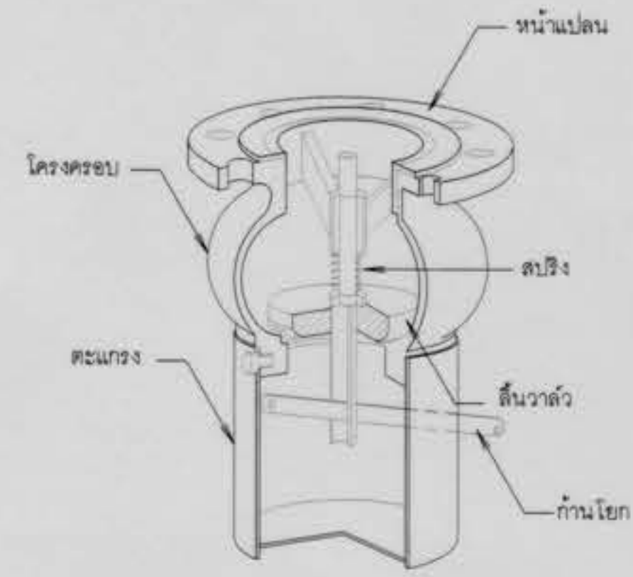
15. พู่ตวลั่ว แบบก้านโยก ไม่แสดงขนาดจาวส่วน
