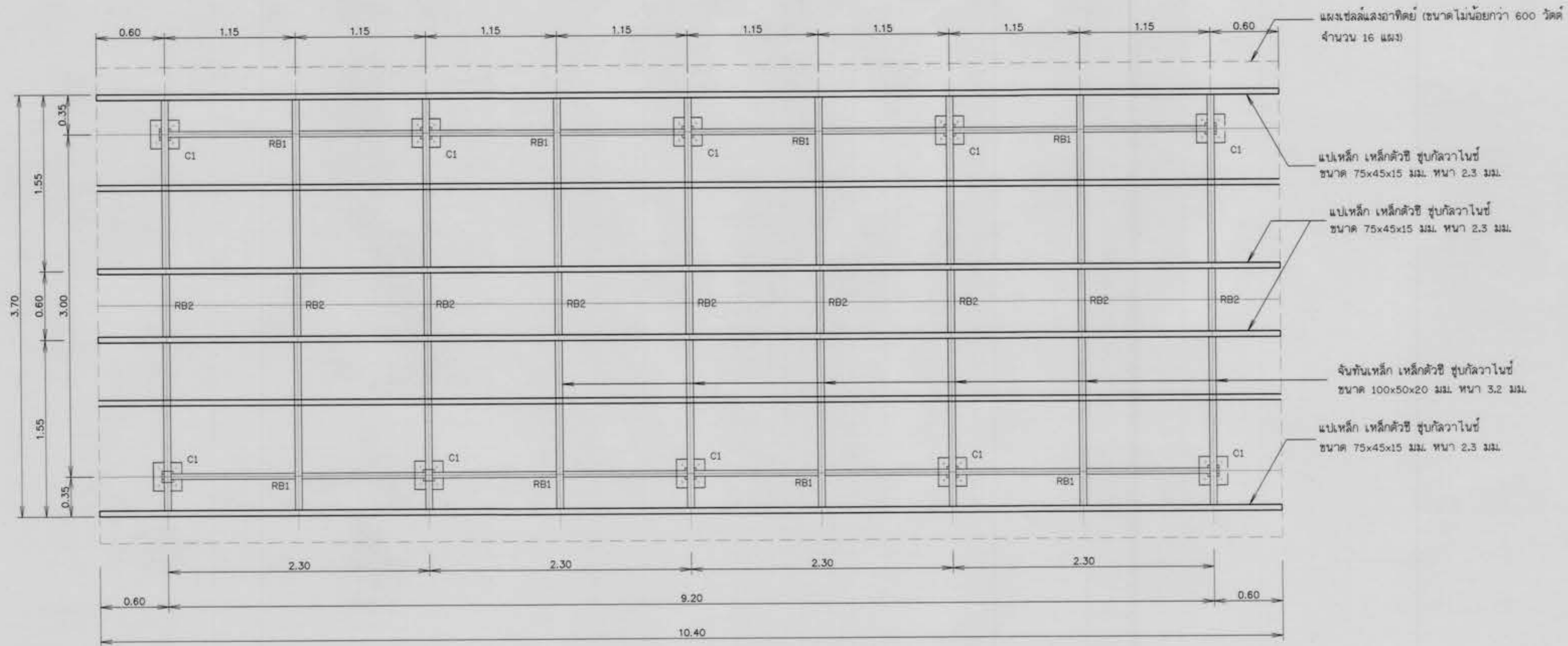
แผนฐานรากและโครงหลังคา โมเมนต์ตามราส่วน
