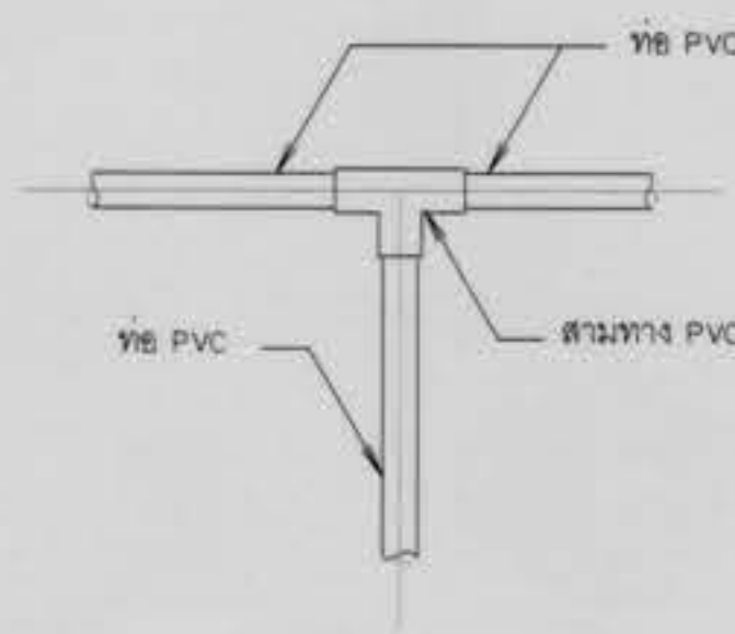
10. แบบการต่อสามทาง PVC ไม่แสดงขนาดจาวส่วน
