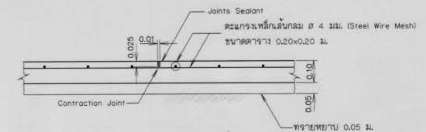
แบบขยายรอยต่อพื้น (Contraction Joint) โมเมนต์ตามราส่วน
