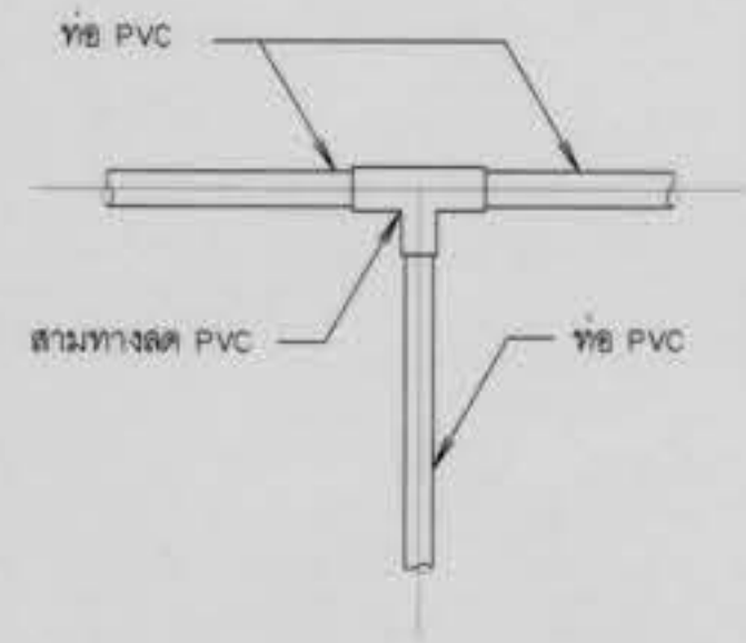
9. แบบการต่อสามทางลด PVC ไม่แสดงขนาดจาวส่วน
