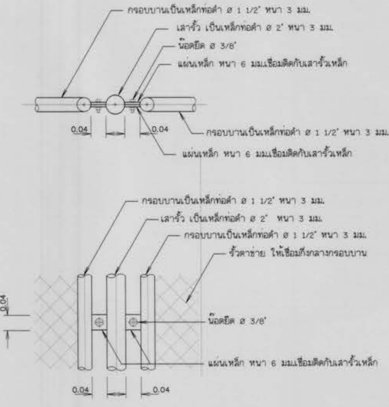
แบบขยายรายละเอียดแสดงการยึดระหว่างรั้วกับเล้า ไม่แสดงขนาดจาล้วน
