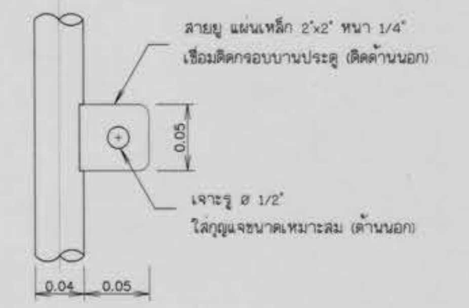
แบบขยายสายยู ไม่แสดงขนาดจาล้วน
