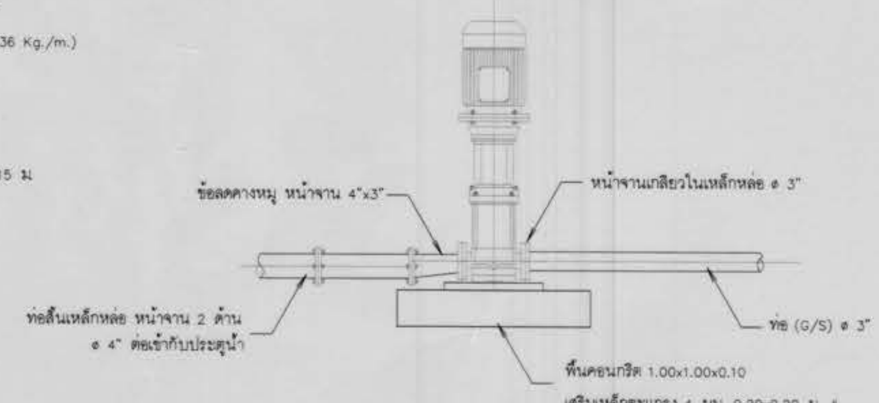
15. การต่อท่อเครื่องสูบน้ำ ไม่แสดงขนาดจาวส่วน
