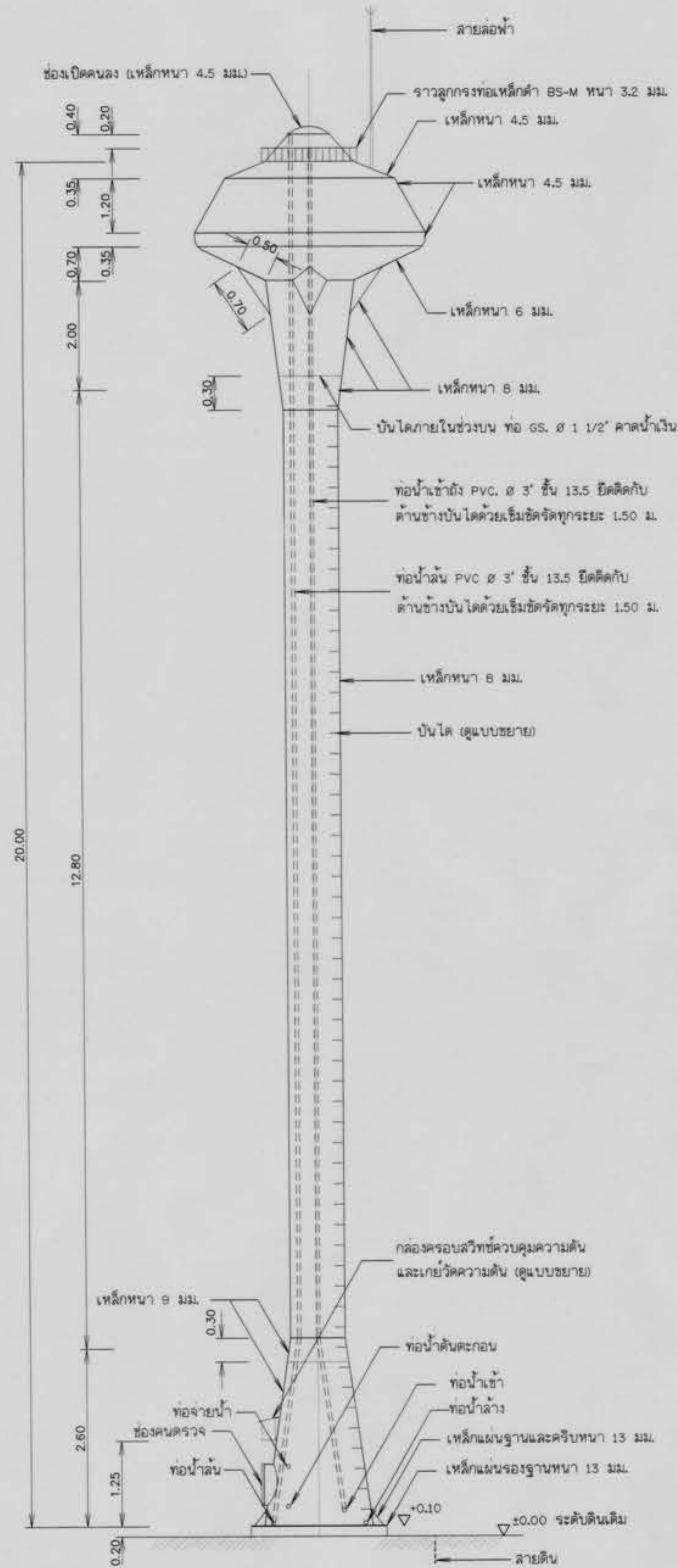
รูปด้านข้างของถังเหล็กแบบถังแชมเปญ
